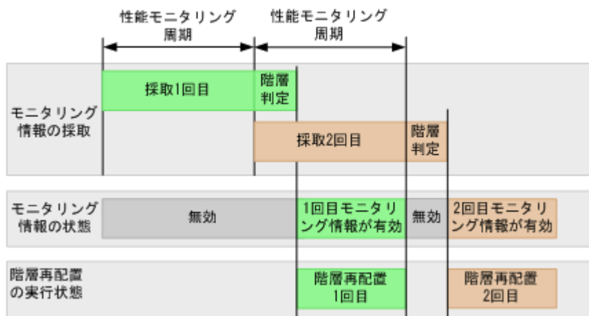
図 13 自動実行モードでのモニタリング情報の採取から階層再配置までの流れ
