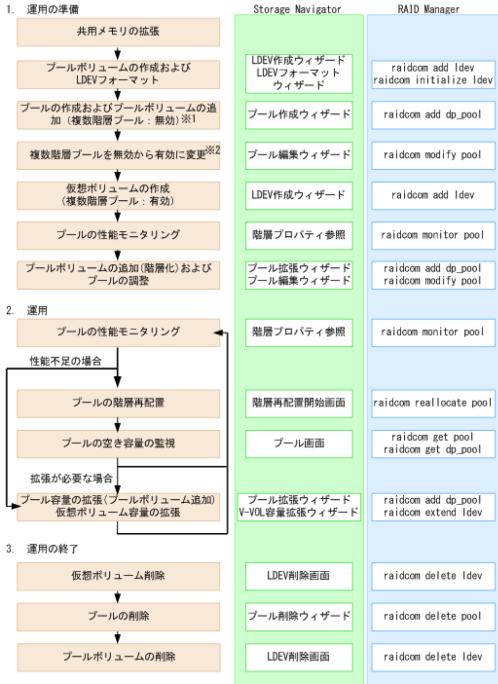
図 38 Dynamic Tiering for Mainframe 運用の流れ
