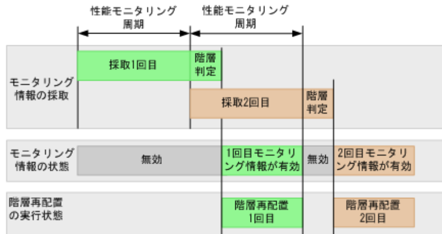
図 18 自動実行モードによる階層再配置の流れ
