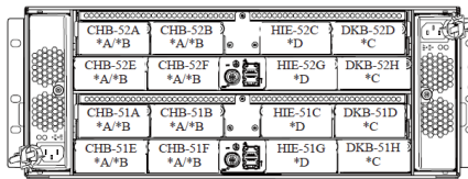
DKC-5 後面
