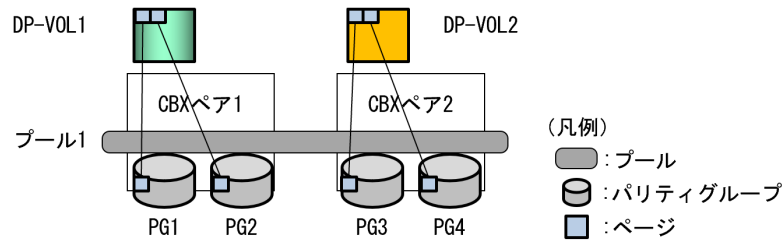
図 50 SCM、SSD、または FMD のパリティグループを含むプールの、性能を重視する場合の推奨構成と非推奨構成
