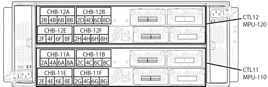
DKC-2 後面の CHB ポート番号
