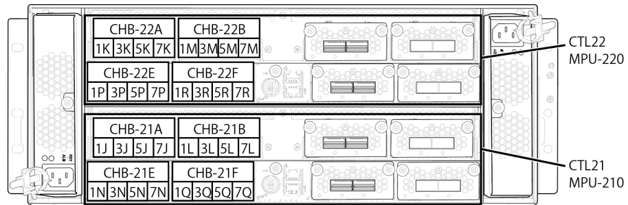
DKC-3 後面の CHB ポート番号
