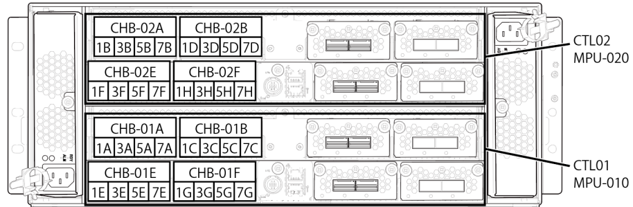
DKC-1 後面の CHB ポート番号
