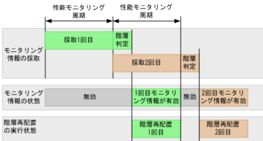
図 19 自動実行モードによる階層再配置の流れ
