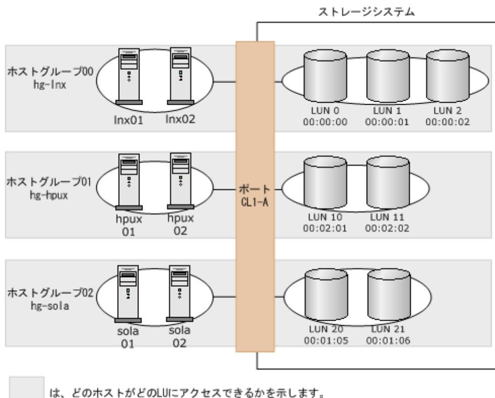
図 33 LUN セキュリティが有効な場合
