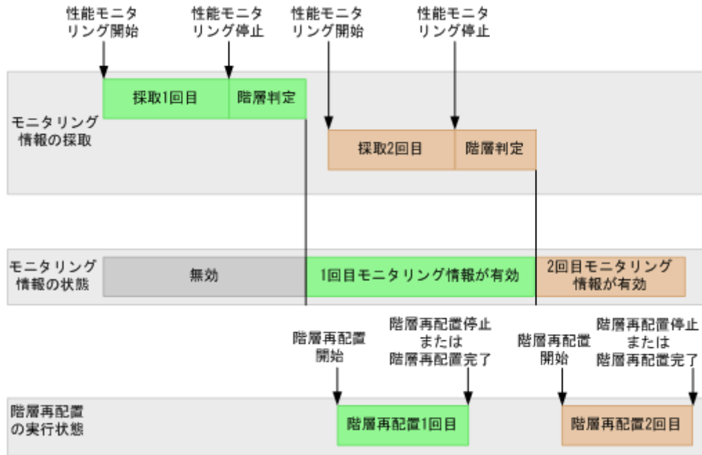
図 15 手動実行モードでのモニタリング情報の採取から階層再配置までの流れ
