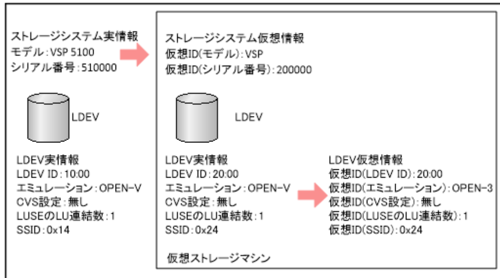
図 43 仮想 ID 設定の例
