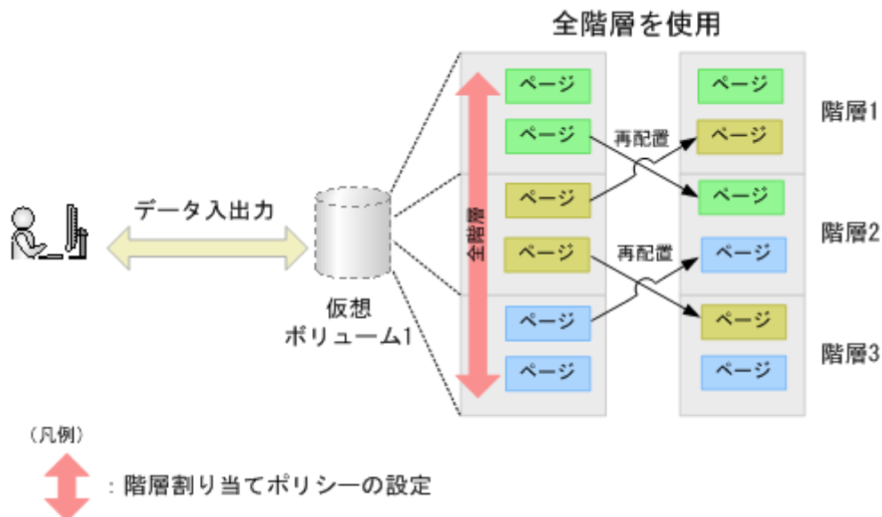
図 23 階層割り当てポリシーが全階層の場合のデータの配置
