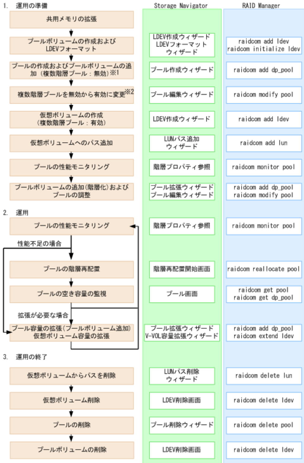
図 48 Dynamic Tiering 運用の流れ
