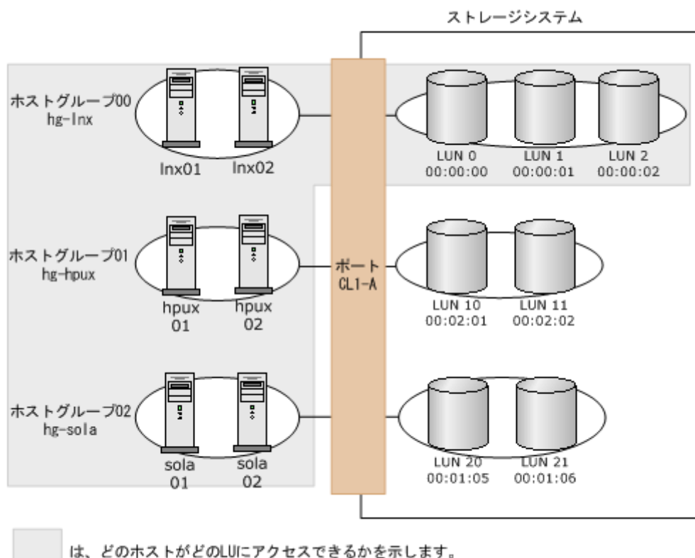
図 34 LUN セキュリティが無効な場合
