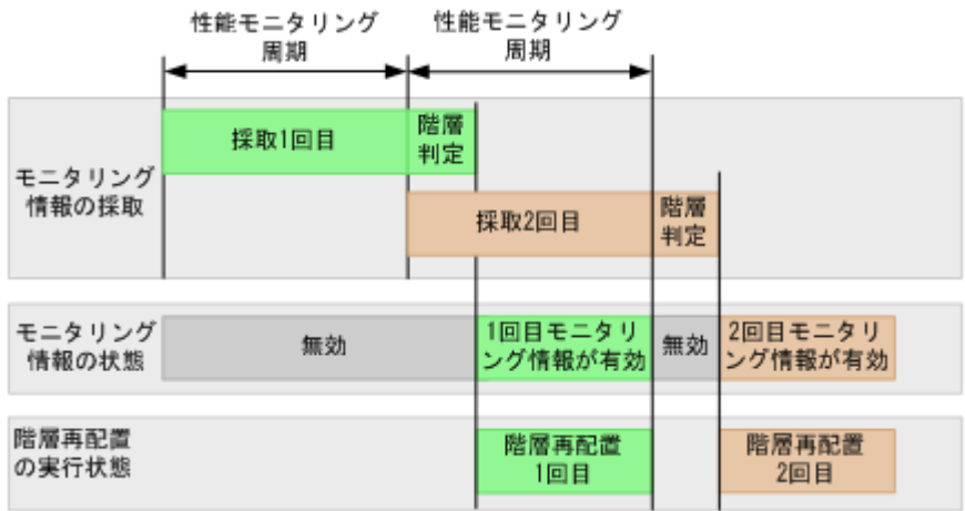
図 14 自動実行モードでのモニタリング情報の採取から階層再配置までの流れ
