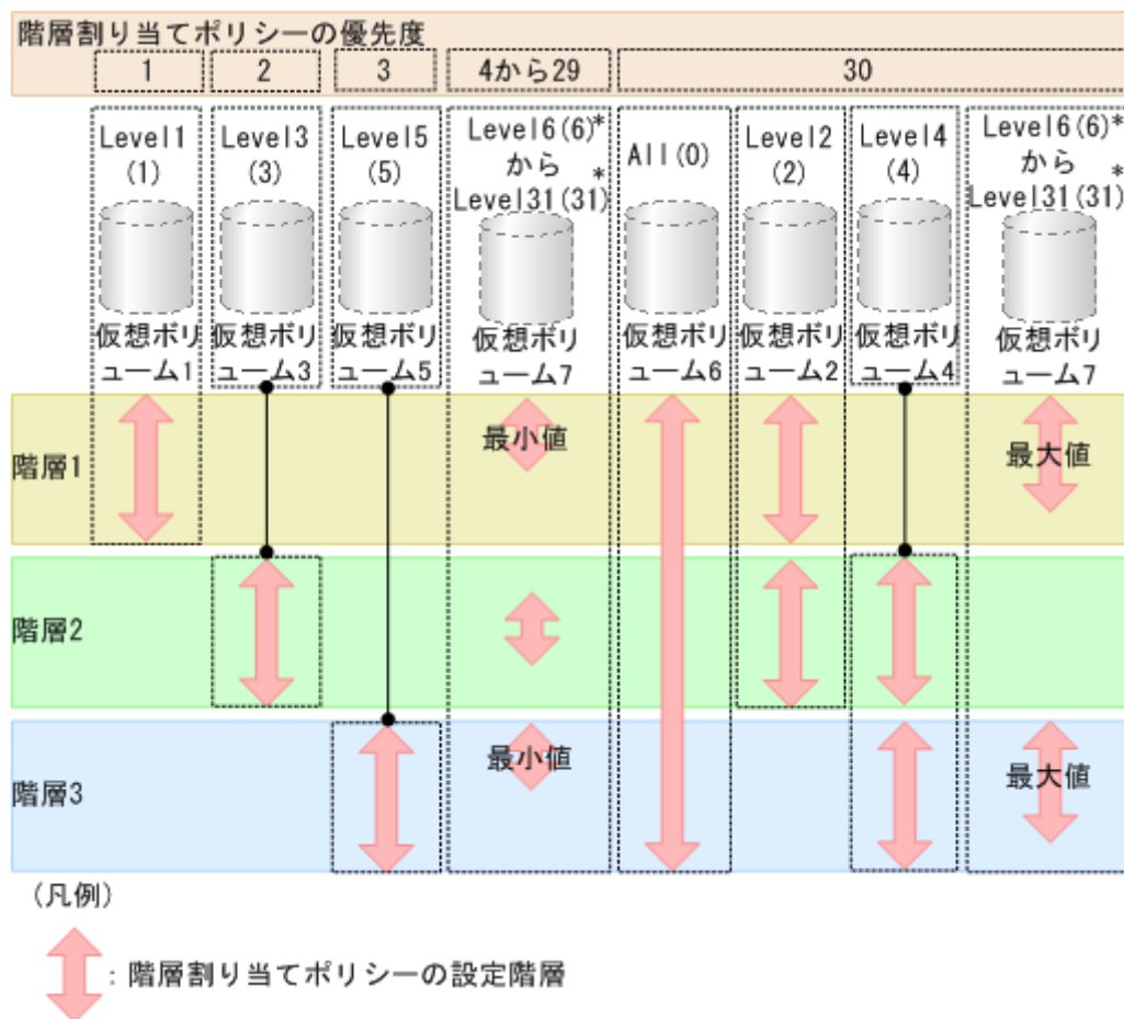
図 28 階層割り当てポリシーの優先度と予約される階層
