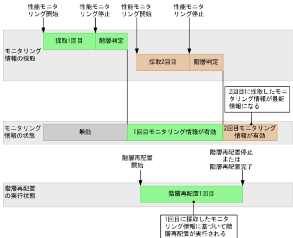
図 16 階層再配置の実行中に 2 回目のモニタリング情報の採取が完了した場合
