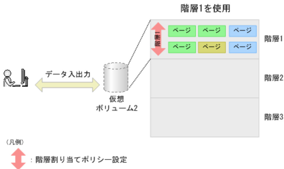
図 24 階層割り当てポリシーを階層 1 に設定した場合のデータの配置
