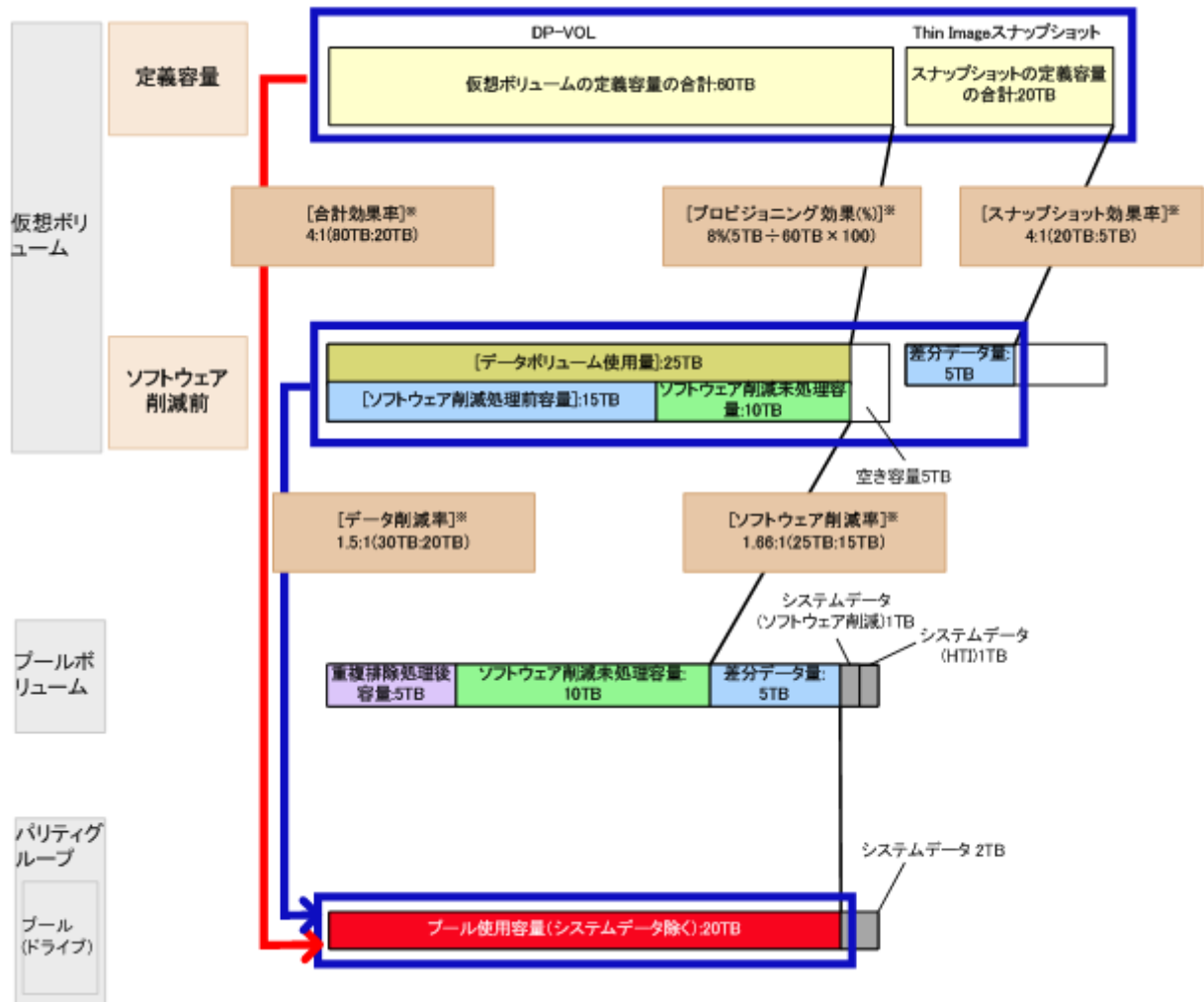
図 31 容量削減機能の重複排除機能と圧縮機能を適用する場合の合計効果とその内訳
