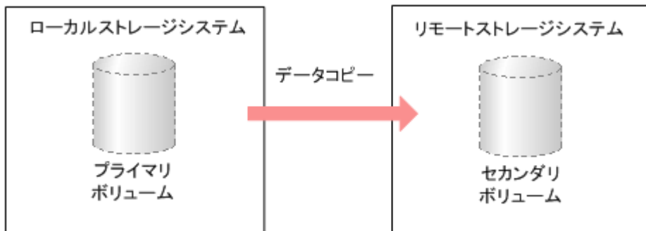
図 37 Dynamic Provisioning、Dynamic Tiering、または active flash と TrueCopy との併用の例
