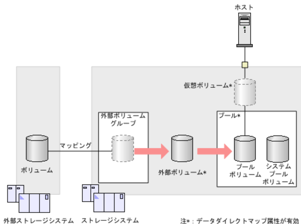
図 5 データダイレクトマップ属性の仮想ボリューム
