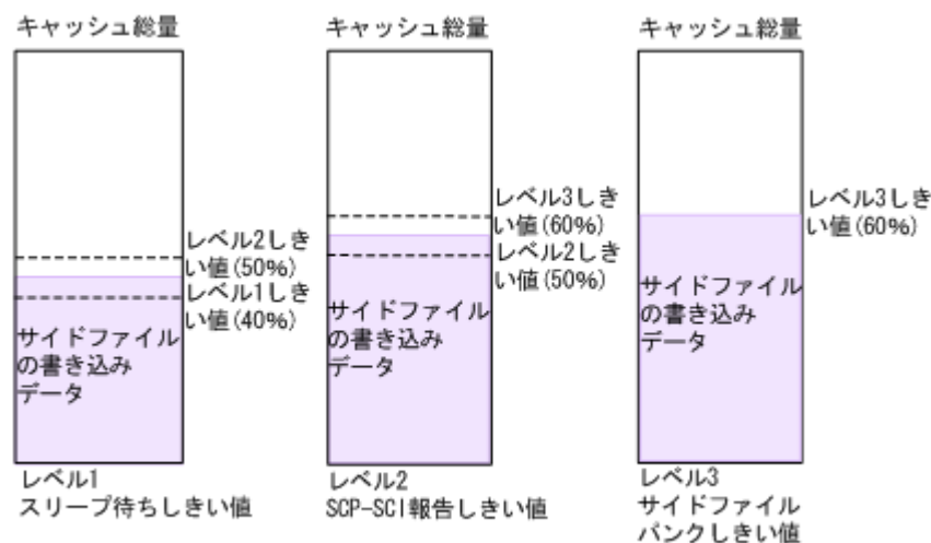
図 16 書き込みデータ量の制御 (1)
