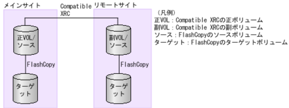
図 11 Compatible XRC の正ボリュームと FlashCopy のソースボリューム、Compatible XRC の副ボリュームと FlashCopy のソースボリュームを共用する構成
