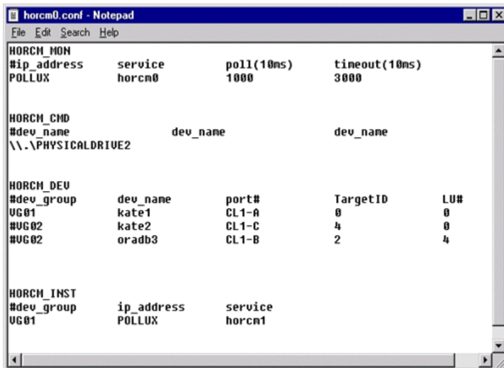
図 7 構成定義ファイル例 - Windows サーバ
