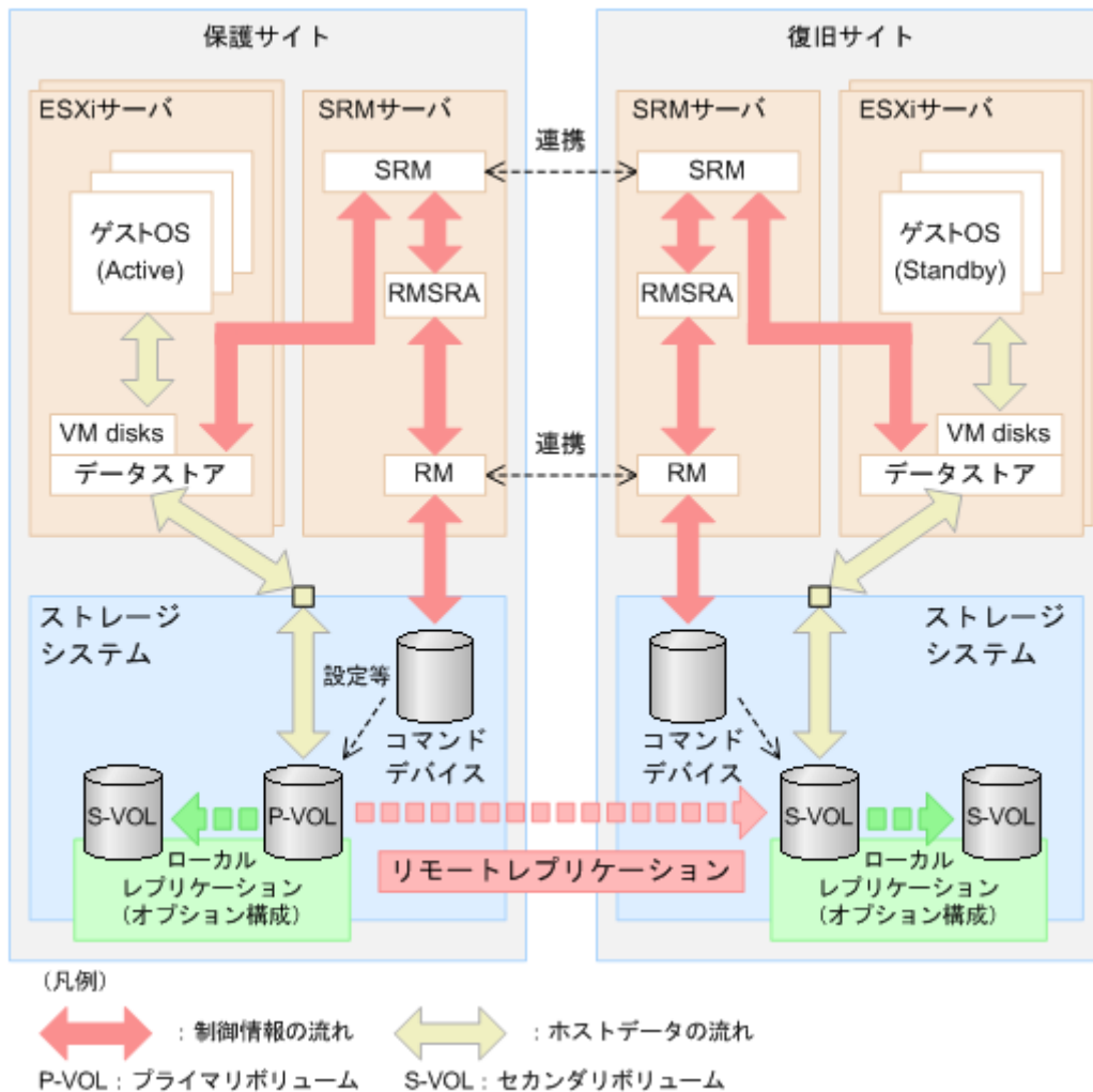
図 B-1：Windows 版 SRM-RMSRA および日立ストレージシステムの構成図 (SRM サーバに RAID Manager をインストールする構成)
