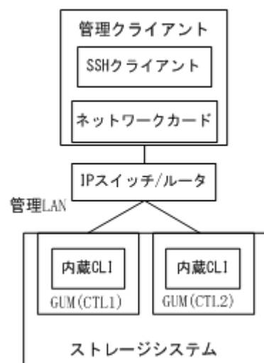
図 A-1 : 内蔵 CLI を使用する場合のシステム構成
