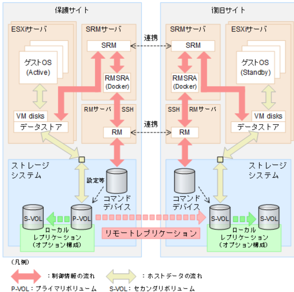
図 B-3 : Virtual Appliance 版 SRM-RMSRA および日立ストレージシステムの構成図
