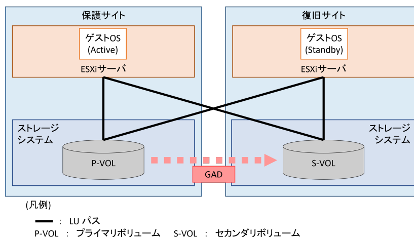
図 B-5 : GAD を使用する構成
