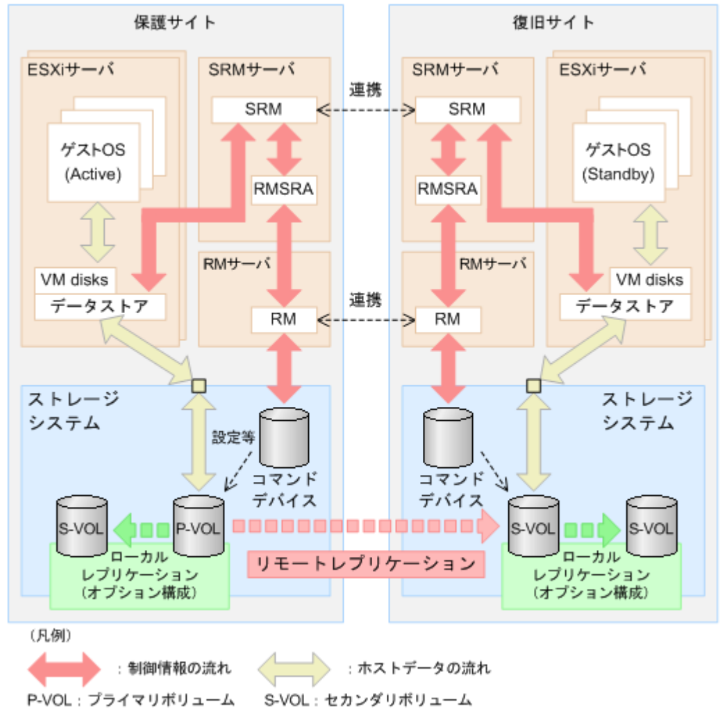
図 B-2 : Windows 版 SRM-RMSRA および日立ストレージシステムの構成図 (SRM サーバとは別に RAID Manager サーバを使用する構成)
