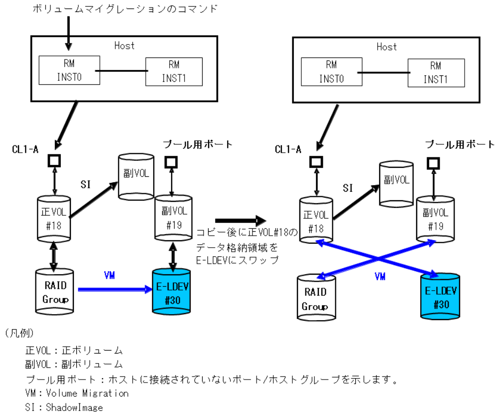
図 6-13 : Volume Migration 構成
