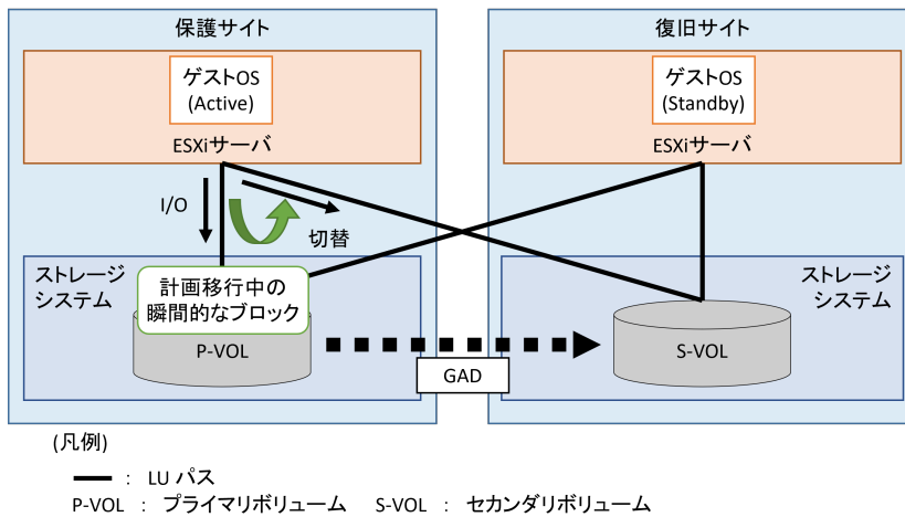
図 B-6 : マルチパスソフトウェアによる I/O 切替の設定例
