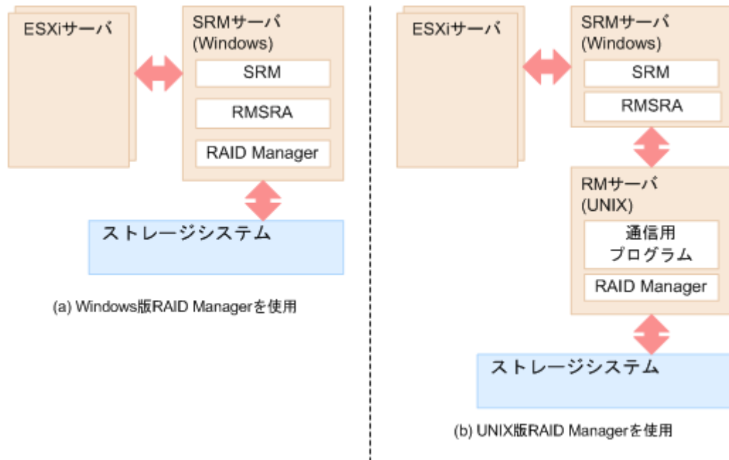
図 B-4 : RAID Manager ホストの OS による構成の違い
