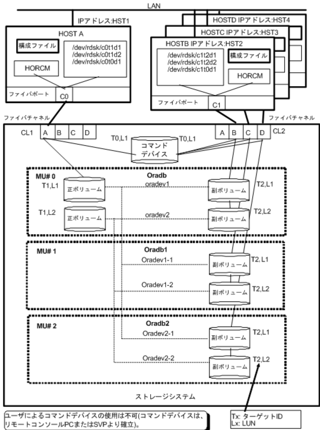
図 24 ShadowImage 構成例 (次ページに続く)
