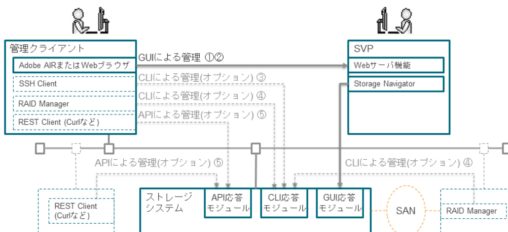
図 2 Storage Navigator 利用の構成
