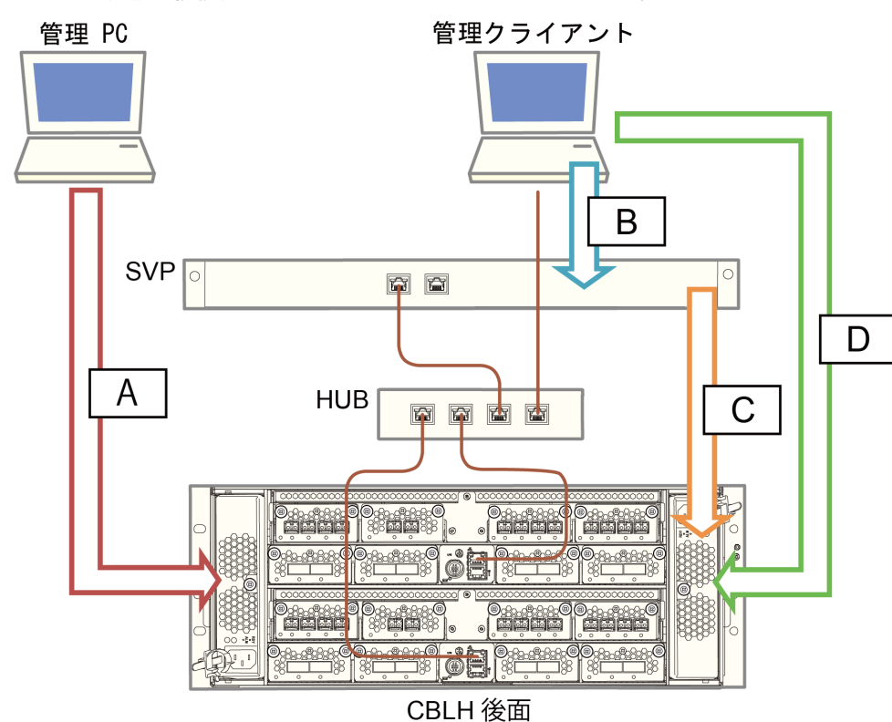
図 4 SSL 通信の接続経路（VSP E590 および VSP E790 以外の場合）
