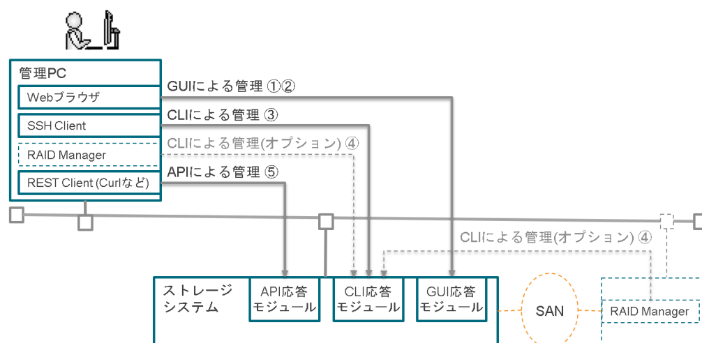
図 1 Hitachi Storage Advisor Embedded 利用の構成
