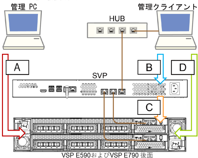
図 3 SSL 通信の接続経路（VSP E590 および VSP E790 の場合）
