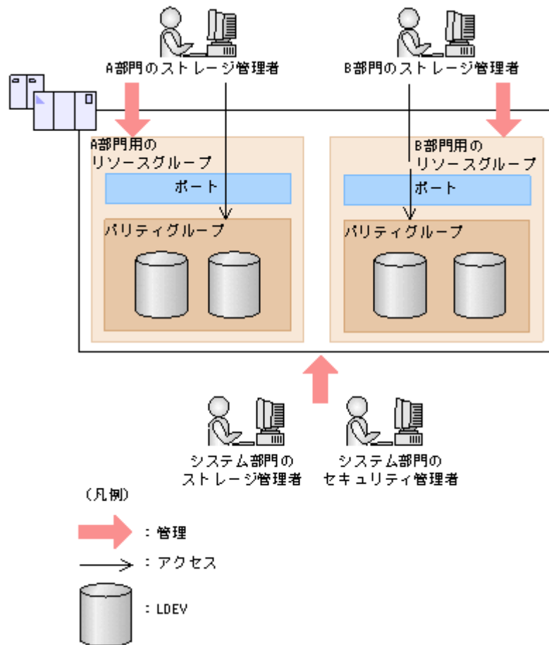
図 8 Resource Partition Manager を使用したシステム構成例（ポートを共有しない場合）
