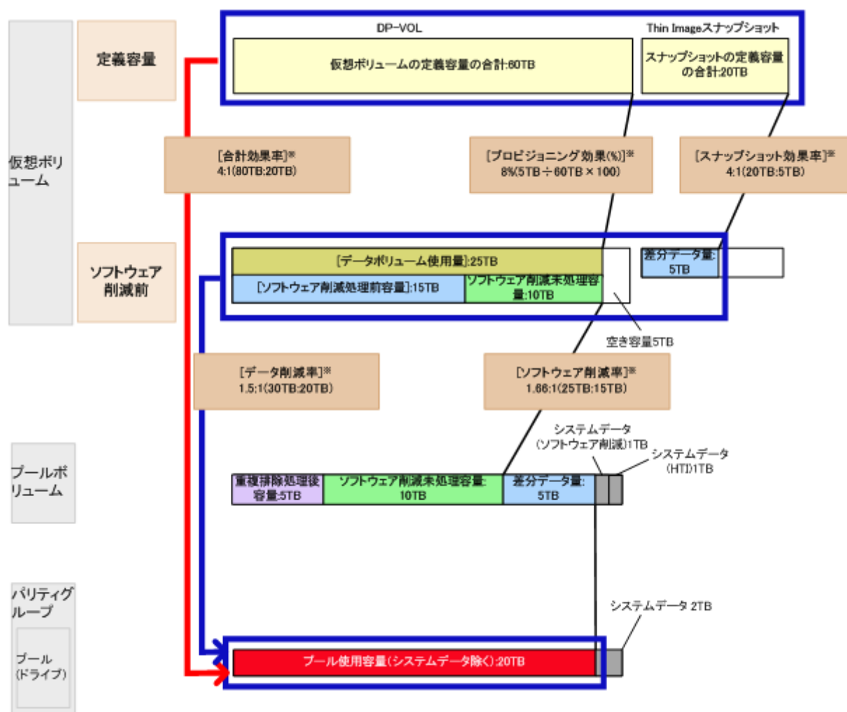
図 6 容量削減機能の重複排除機能と圧縮機能を適用する場合の合計効果とその内訳
