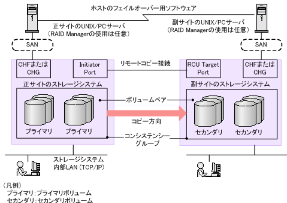
図 1 TrueCopy の構成要素（ファイバチャネルインタフェースまたは iSCSI インタフェース）
