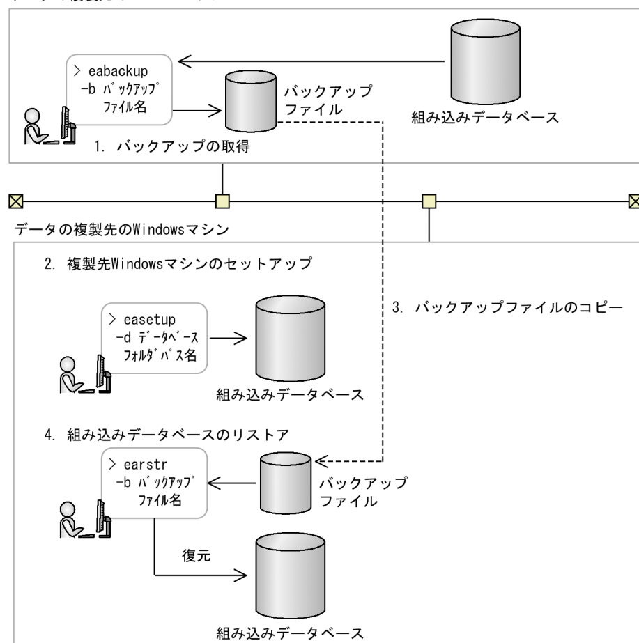
図 4-2 解析環境の複製
