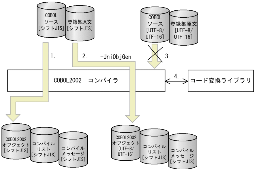
図 24-1 コンパイルでの Unicode 機能（シフト JIS 環境下）
