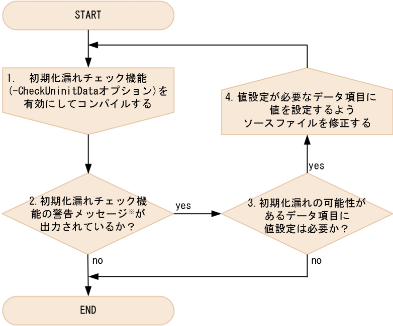
図 29-5 初期化漏れチェック機能を使用するときの作業の流れ
