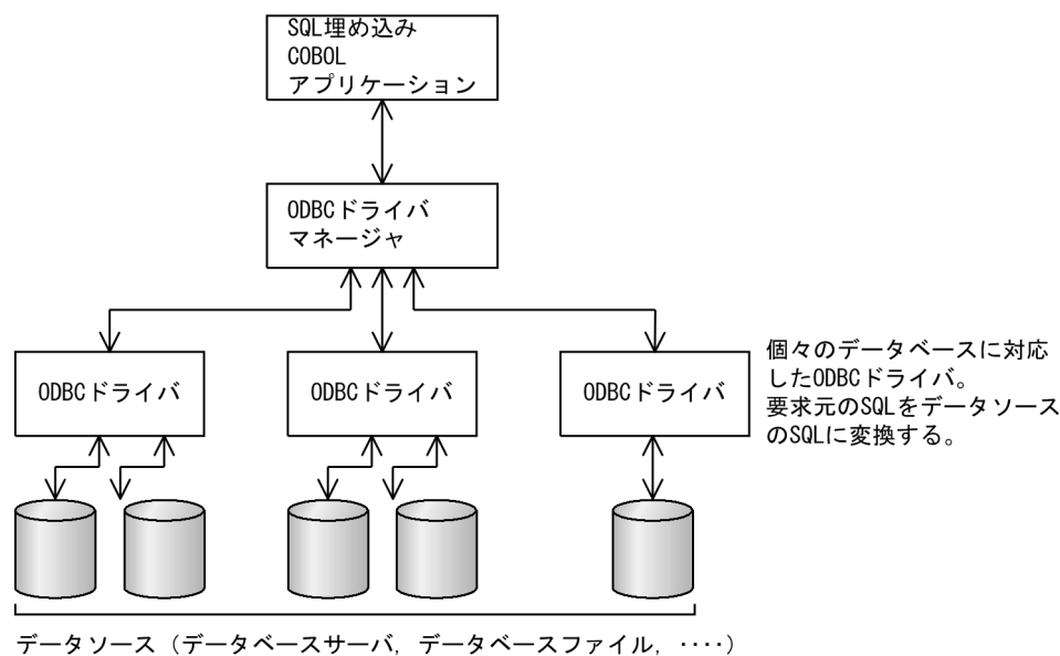
図 21-3 ODBC インタフェース機能の概要
