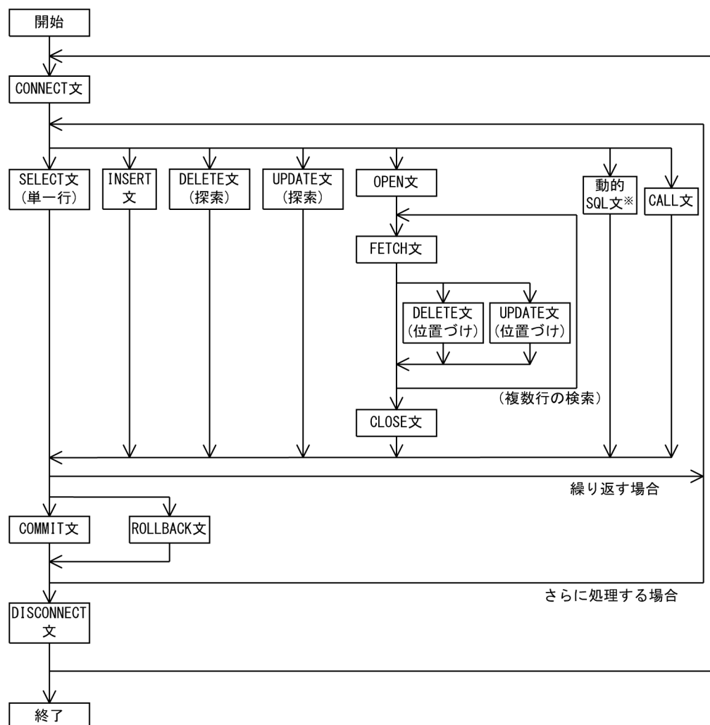
図 21-1 SQL 文の実行順序
