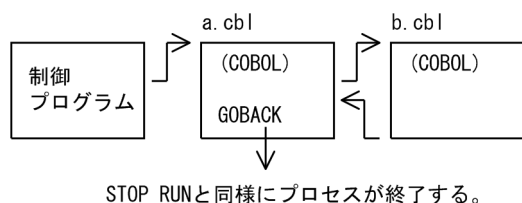
図 14-2 GOBACK 文による終了の例
