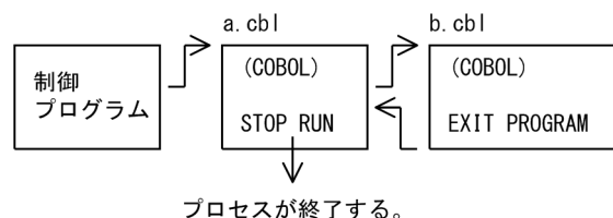
図 14-1 STOP RUN 文による終了の例
