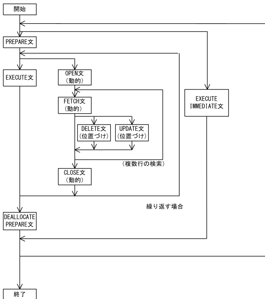
図 21-2 動的 SQL 文の実行順序
