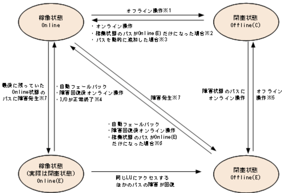
図 2-11 パスの状態遷移
