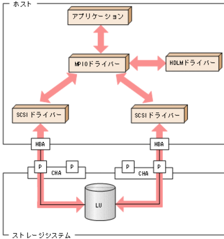
図 2-6 HDLM ドライバーと MPIO ドライバーの位置づけ
