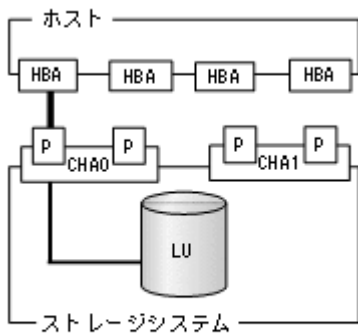
図 3-3 シングルパス構成およびマルチパス構成
