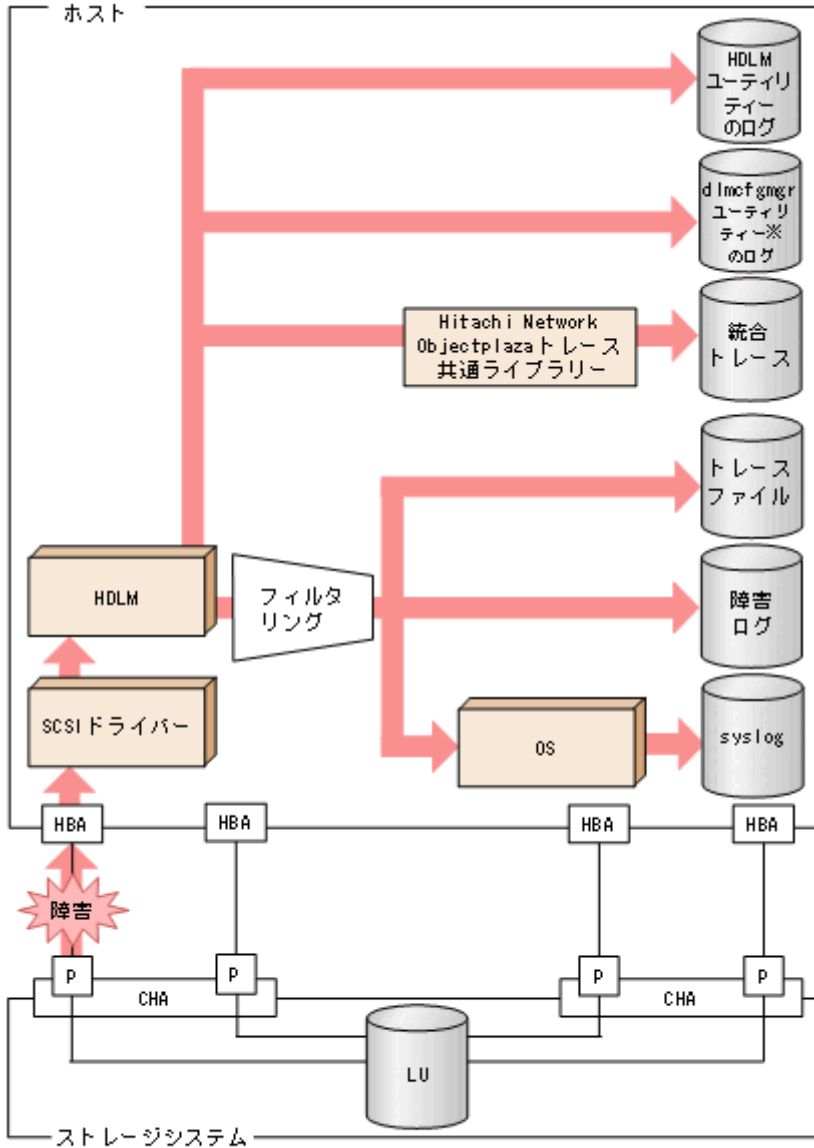
図 2-13 障害情報を採取するときのデータの流
