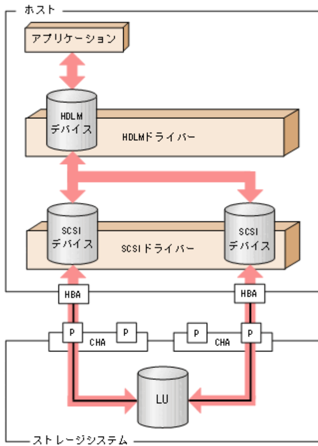
図 2-4 HDLM ドライバーと HDLM デバイスの位置づけ
