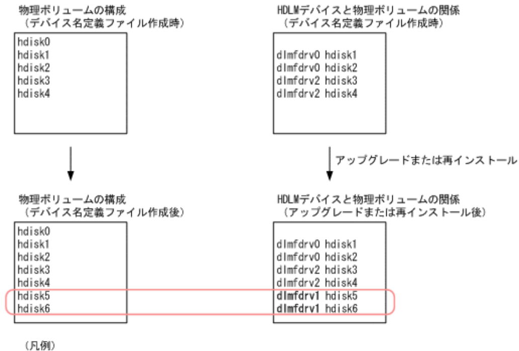
図 7-2 HDLM が HDLM デバイスの名称を定義する例
