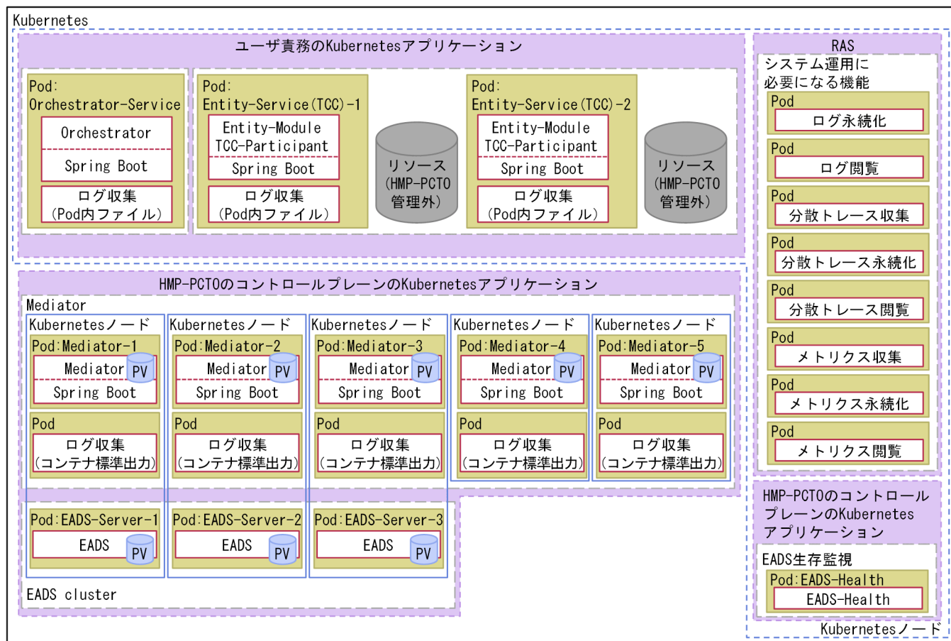
図 1-6 TCC-Participant を使用する場合の最小機器構成（ThreeQuarters 合意方式（通常版））
