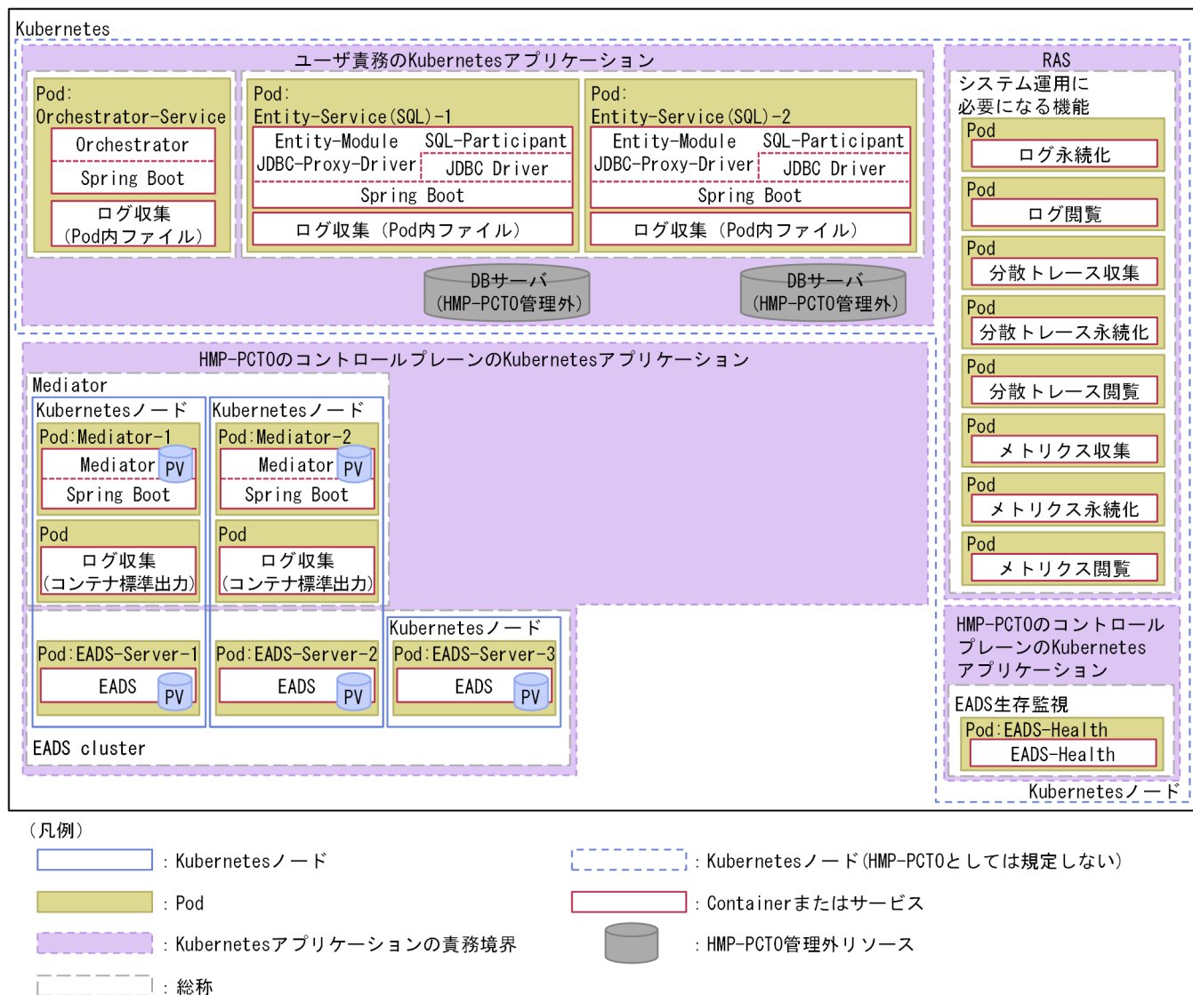
図 1-3 SQL-Participant を使用する場合の最小機器構成 (PrivilegedValue 合意方式 (通常版))
