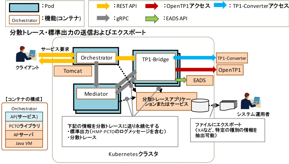
図 11-6 HMP-PCTO 分散トレース・標準出力の送信およびエクスポート (TP1-Bridge を使用する場合)
