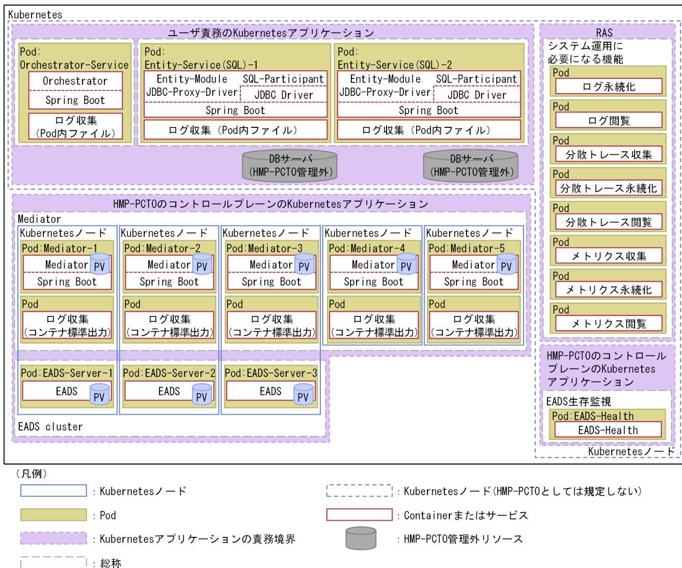
図 1-2 SQL-Participant を使用する場合の最小機器構成（ThreeQuarters 合意方式（通常版））
