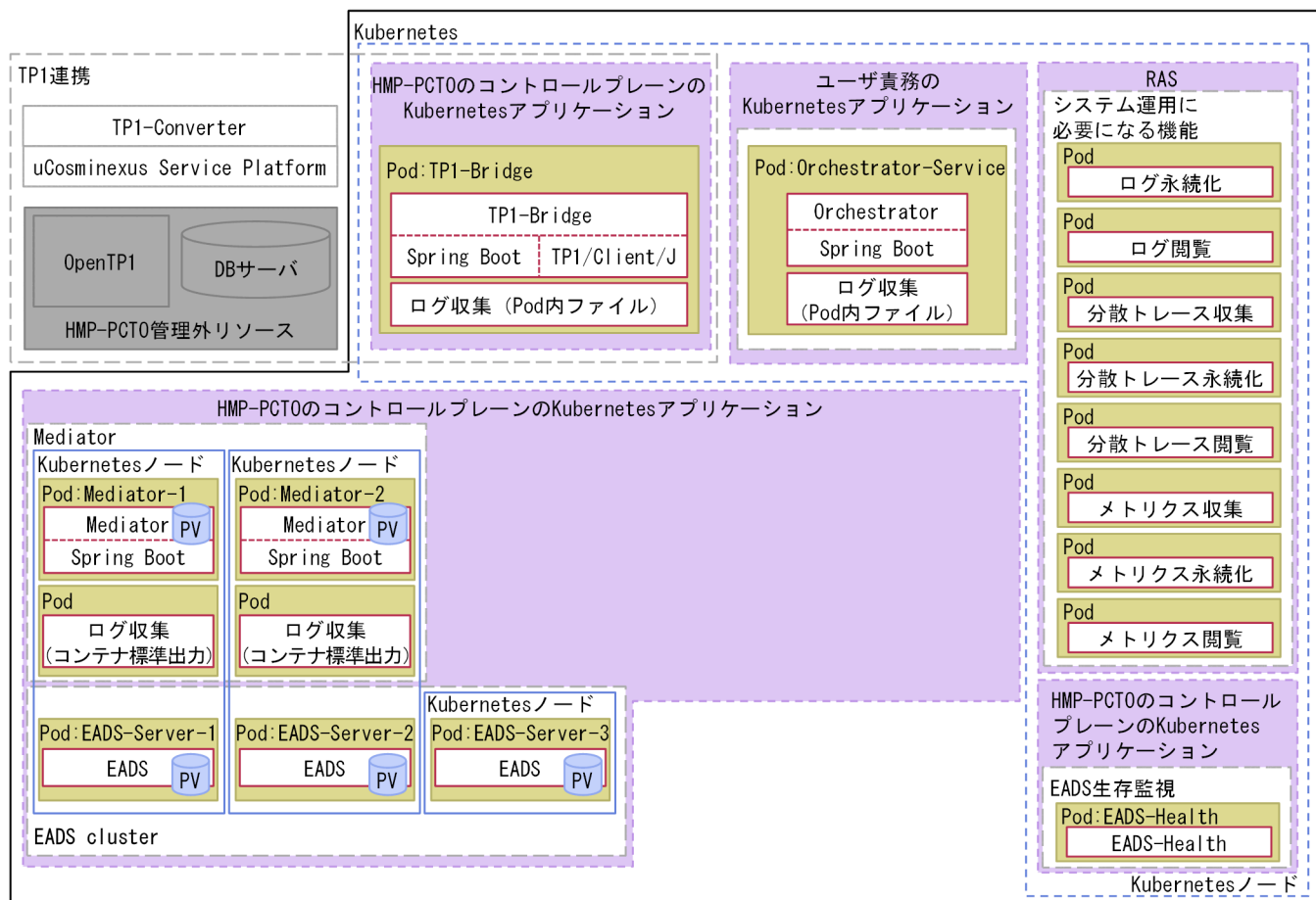
図 1-11 TP1-Bridge を使用する場合の最小機器構成 (PrivilegedValue 合意方式 (通常版))
