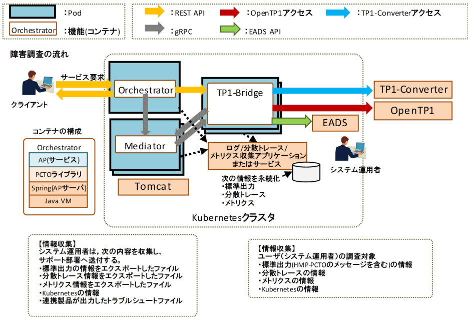
図 11-45 HMP-PCTO 障害発生時の流れ (TP1-Bridge を使用する場合)
