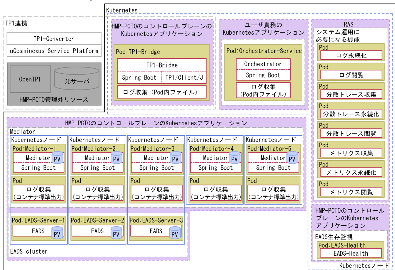
図 1-10 TP1-Bridge を使用する場合の最小機器構成（ThreeQuarters 合意方式（通常版））
