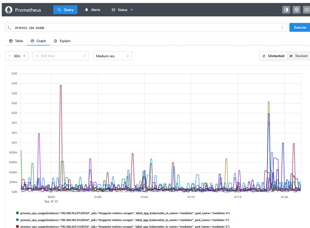
図 11-41 Prometheus サーバの標準の Web UI
