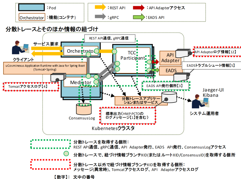
図 11-8 HMP-PCTO 各情報の紐づけのイメージ (TCC-Participant を使用する場合)
