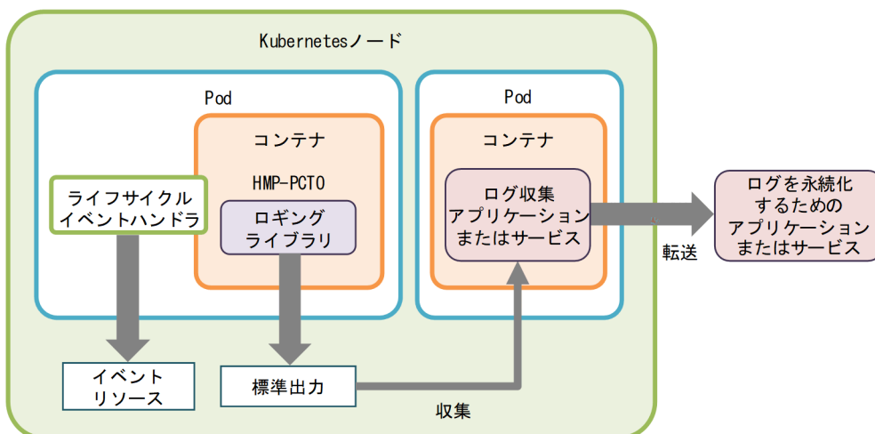
図 11-10 メッセージログの構成
