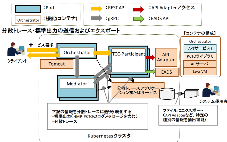
図 11-5 HMP-PCTO 分散トレース・標準出力の送信およびエクスポート（TCC-Participant を使用する場合）
