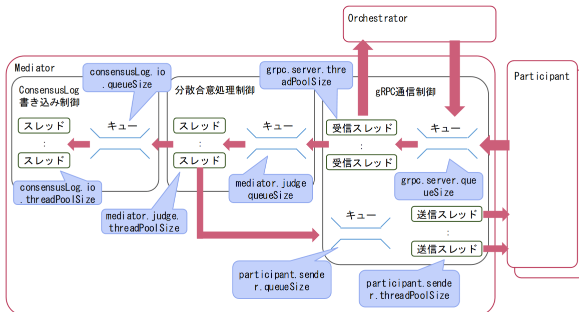
図 3-14 同時実行スレッド数制御
