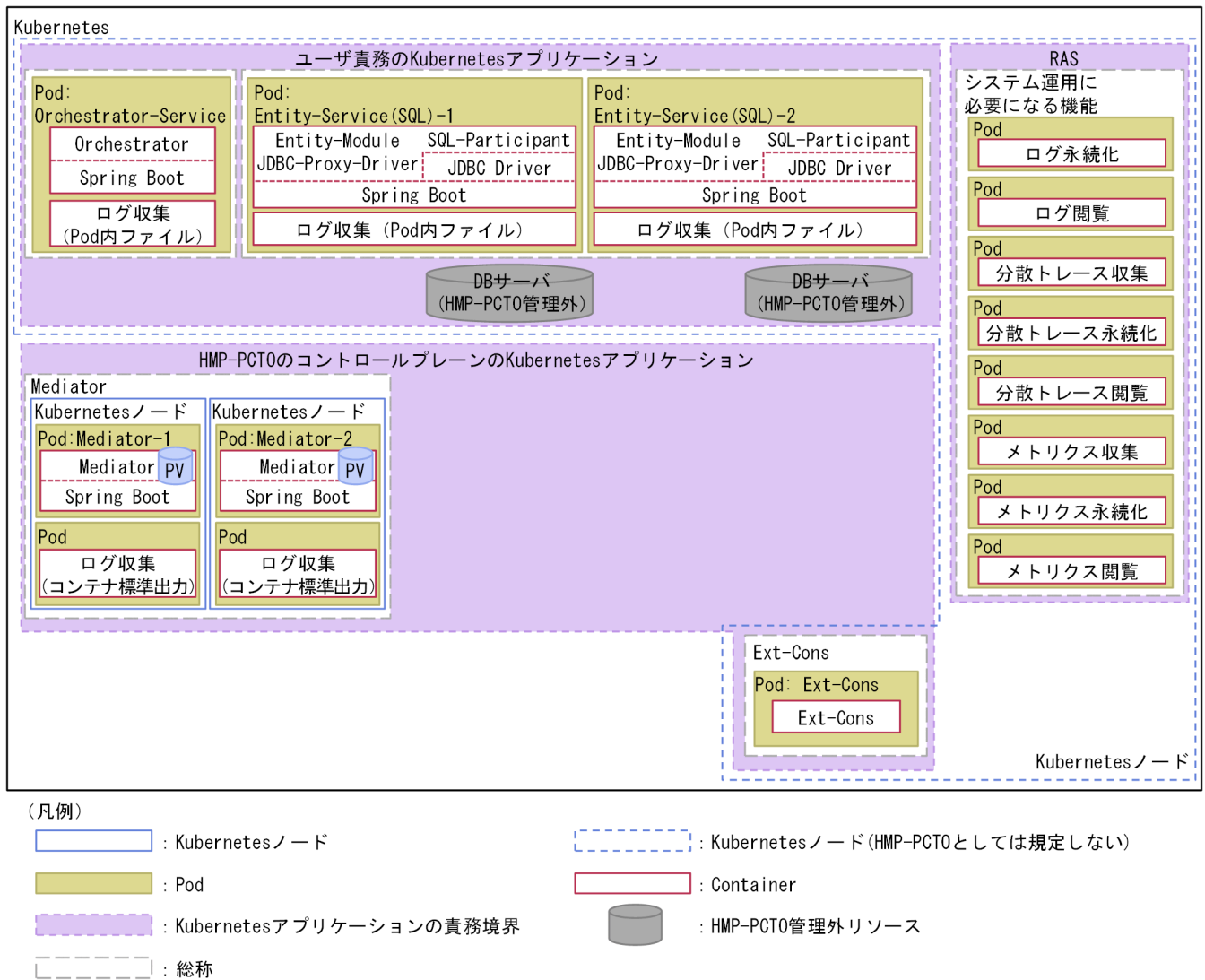
図 1-5 SQL-Participant を使用する場合の最小機器構成（PrivilegedValue 合意方式（トライアル版））
