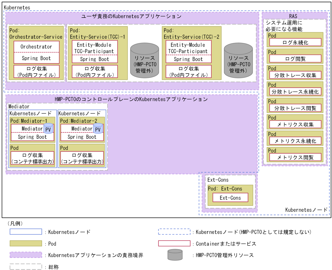
図 1-9 TCC-Participant を使用する場合の最小機器構成（PrivilegedValue 合意方式（トライアル版））
