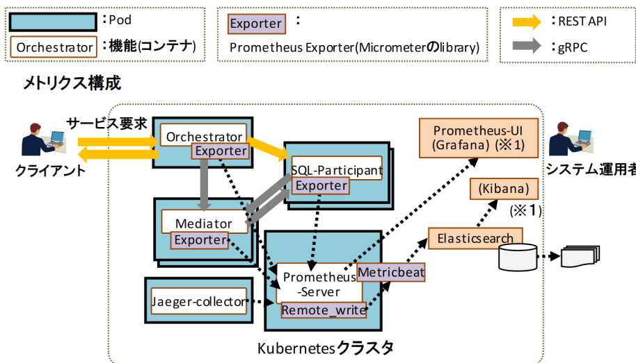
図 11-35 HMP-PCTO メトリクスの構成 (SQL-Participant の場合)
