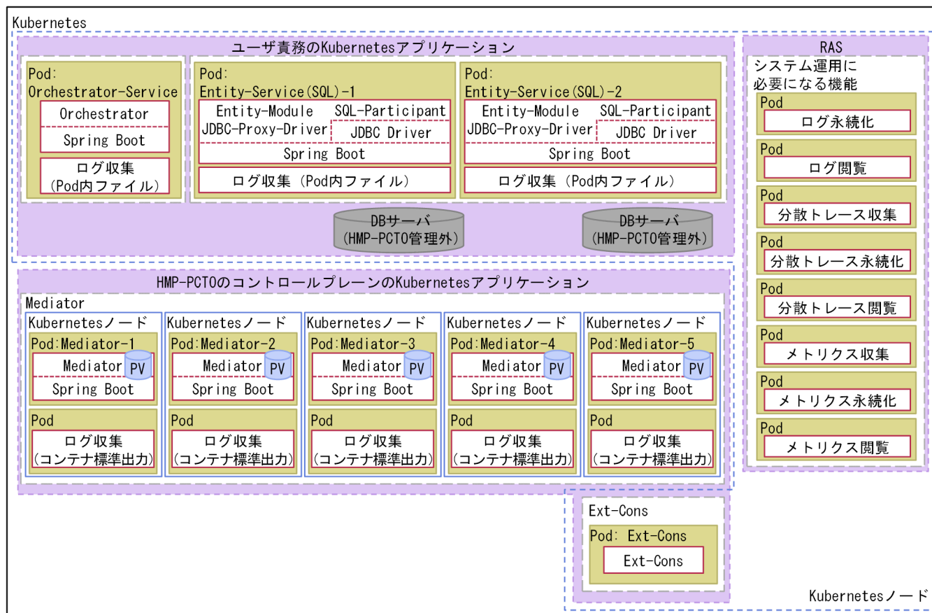
図 1-4 SQL-Participant を使用する場合の最小機器構成（ThreeQuarters 合意方式（トライアル版））
