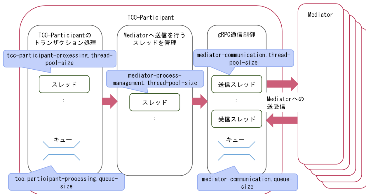
図 3-10 TCC-Participant の同時実行スレッド数制御
