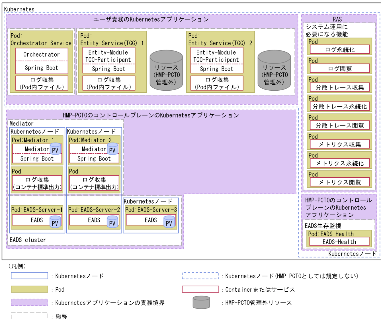
図 1-7 TCC-Participant を使用する場合の最小機器構成 (PrivilegedValue 合意方式 (通常版))
