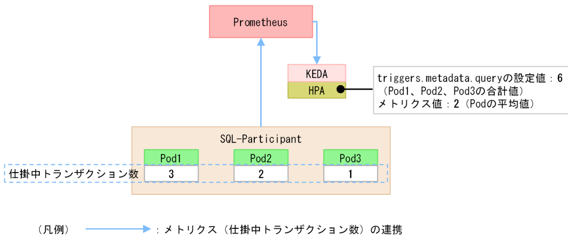
図 4-4 triggers.metadata.query の設定例イメージ図
