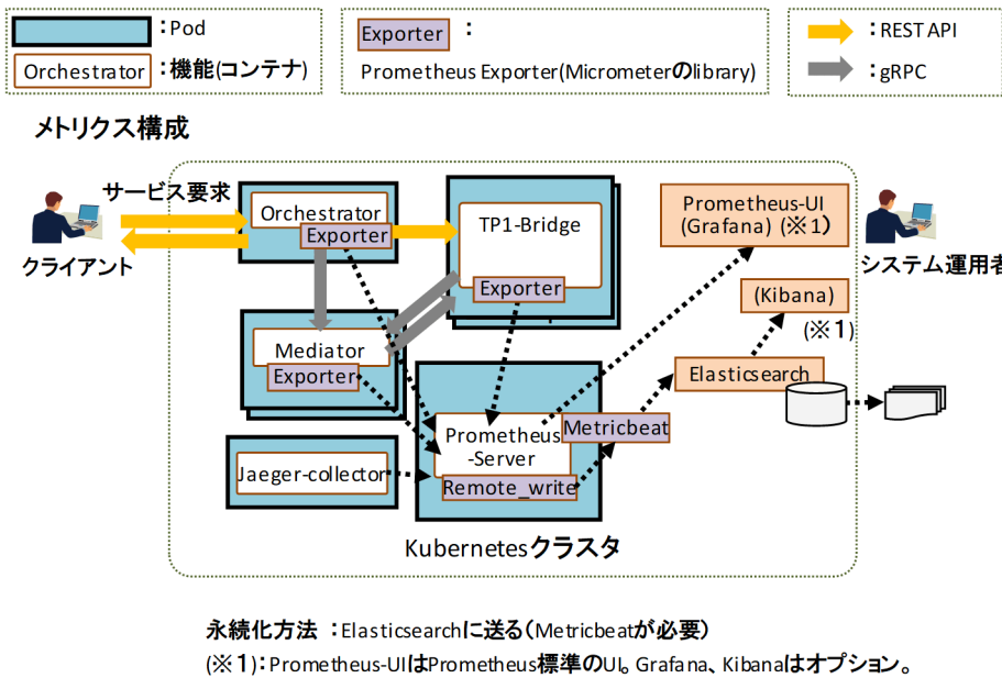
図 11-37 HMP-PCTO メトリクスの構成 (TP1-Bridge の場合)
