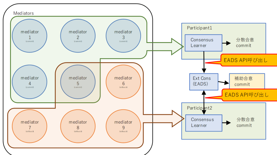
図 11-32 EADS 向けトレース
