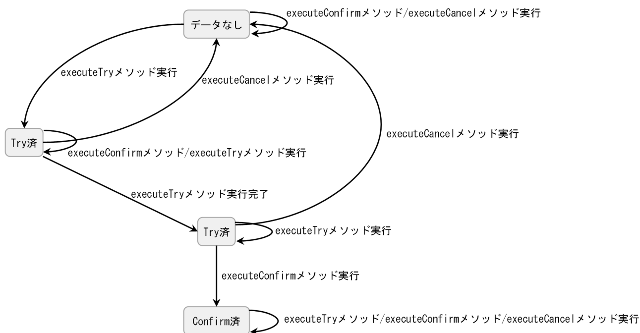
図 2-1 データのステートマシン図
