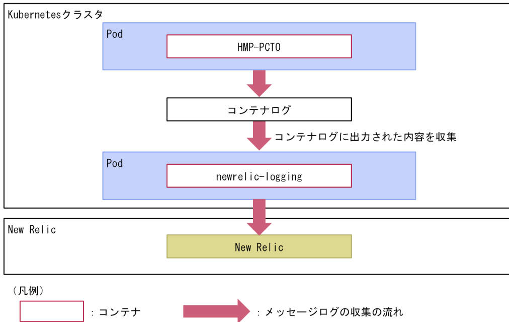
図 11-11 New Relic 使用時の構成図
