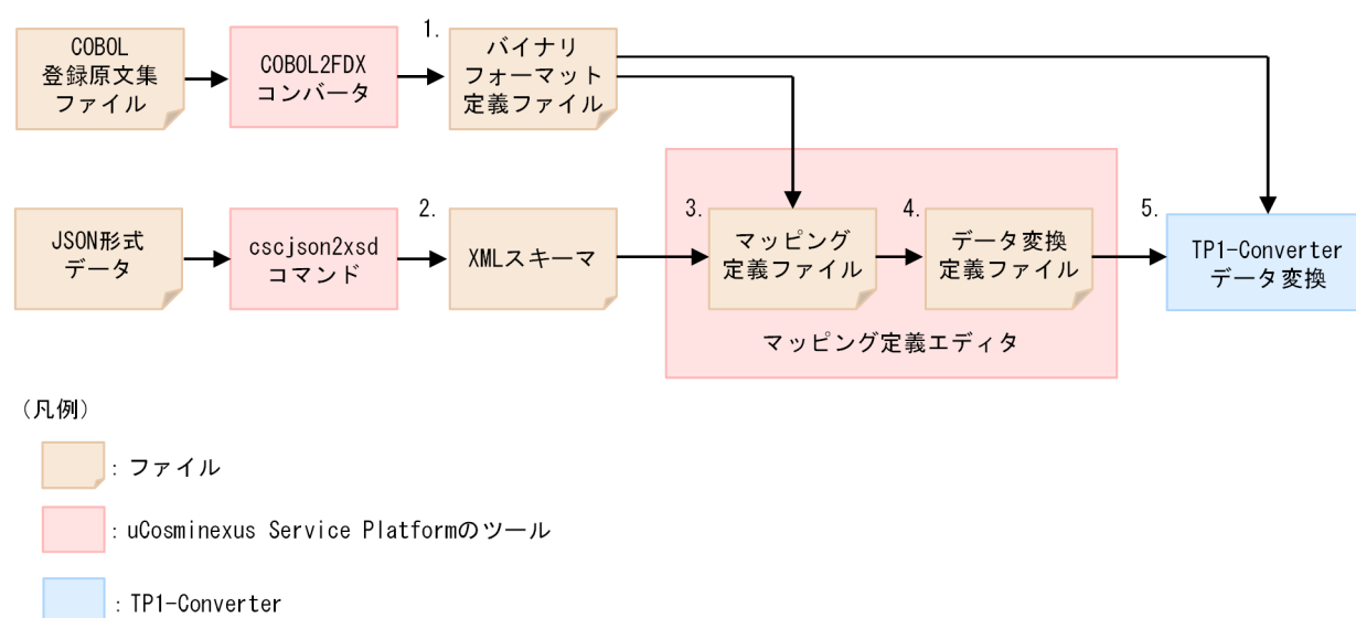
図 5-2 データ変換で使用するファイルを作成する流れ
