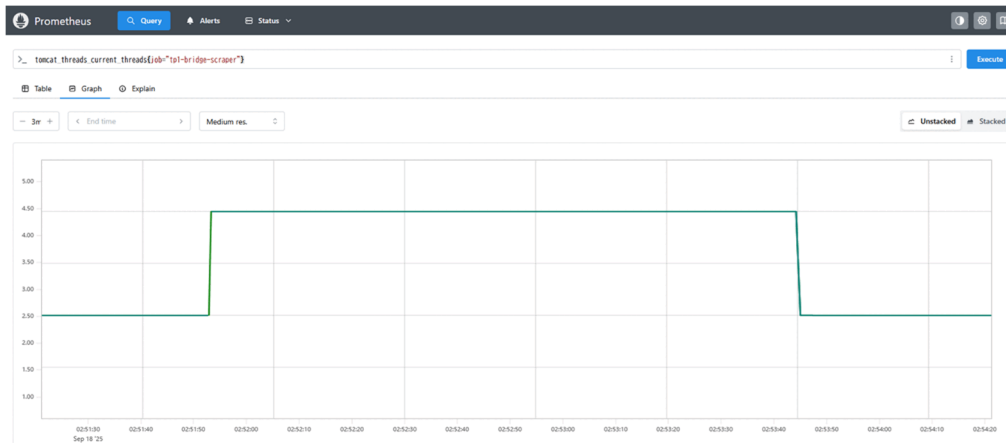
図 3-17 Prometheus の Web UI
