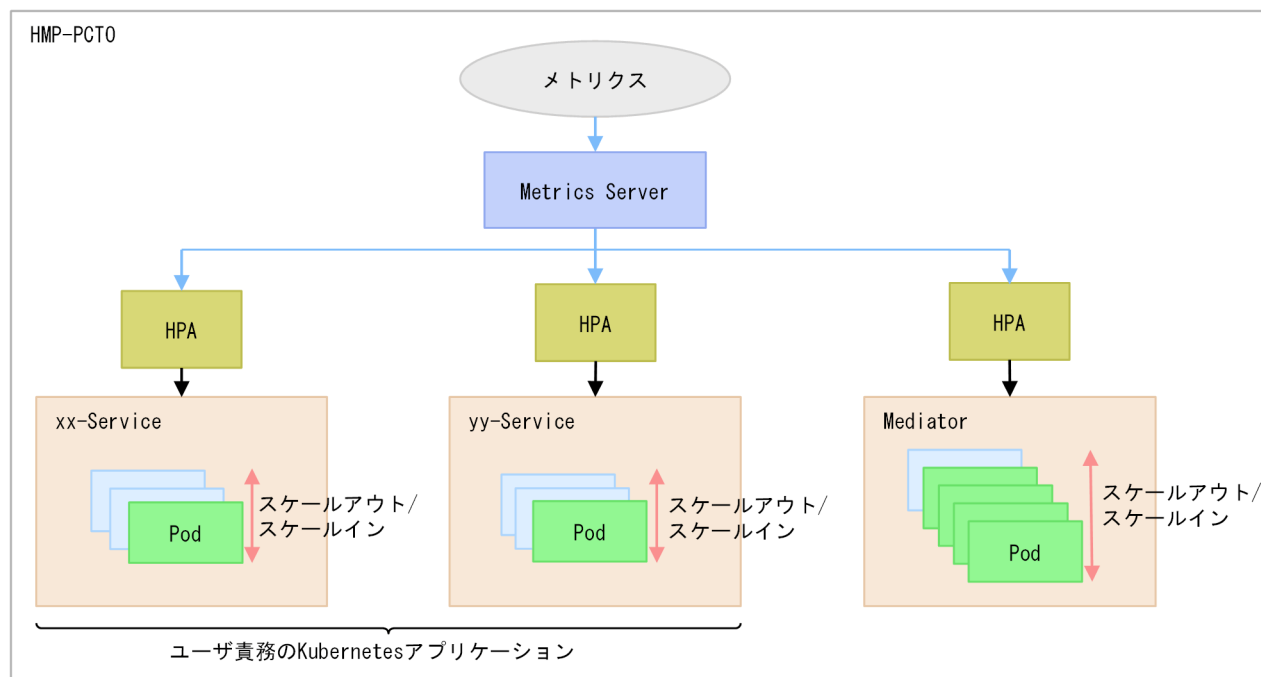
図 4-2 オートスケールの設定後の Kubernetes アプリケーションと Pod の構成図 (Metrics Server でメトリクスを監視する方法)
