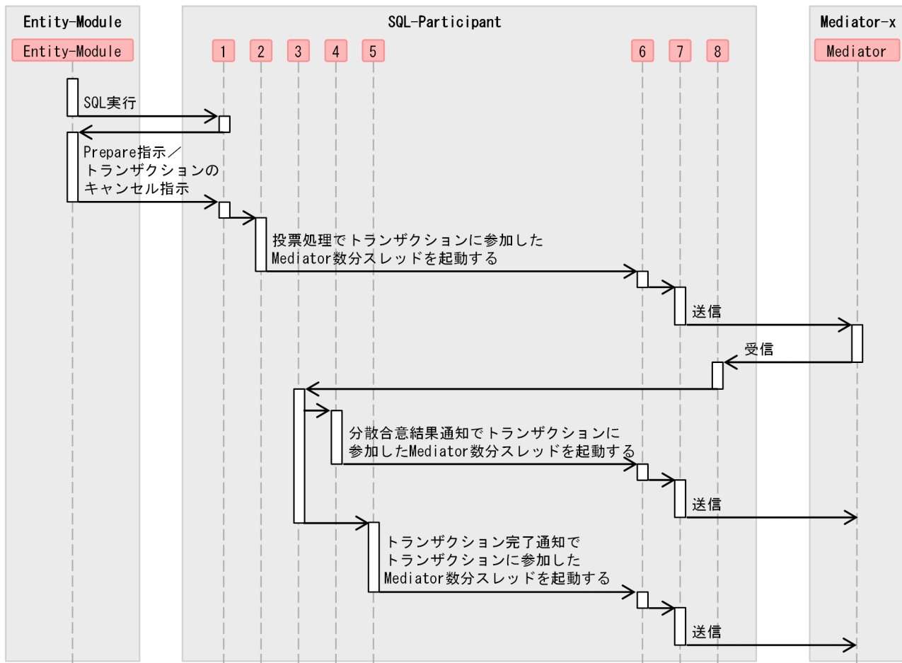
図 3-7 SQL-Participant のスレッド占有期間
