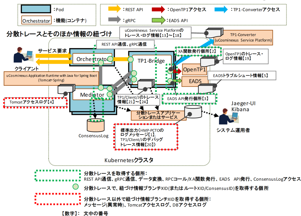
図 11-9 HMP-PCTO 各情報の紐づけのイメージ (TP1-Bridge を使用する場合)
