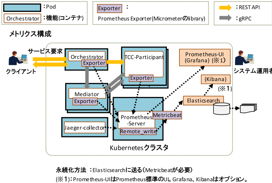
図 11-36 HMP-PCTO メトリクスの構成 (TCC-Participant の場合)
