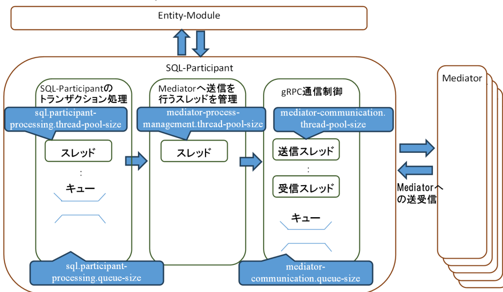
図 3-6 SQL-Participant の同時実行スレッド数制御
