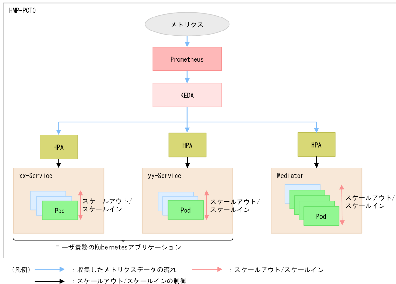
図 4-3 オートスケールの設定後の Kubernetes アプリケーションと Pod の構成図 (Prometheus でメトリクスを監視する方法)
