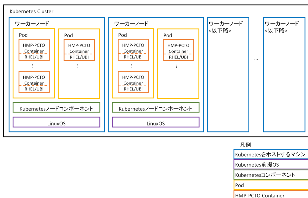
図 1-1 HMP-PCTO の Kubernetes クラスタの構成要素
