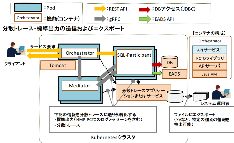
図 11-4 HMP-PCTO 分散トレース・標準出力の送信およびエクスポート（SQL-Participant を使用する場合）
