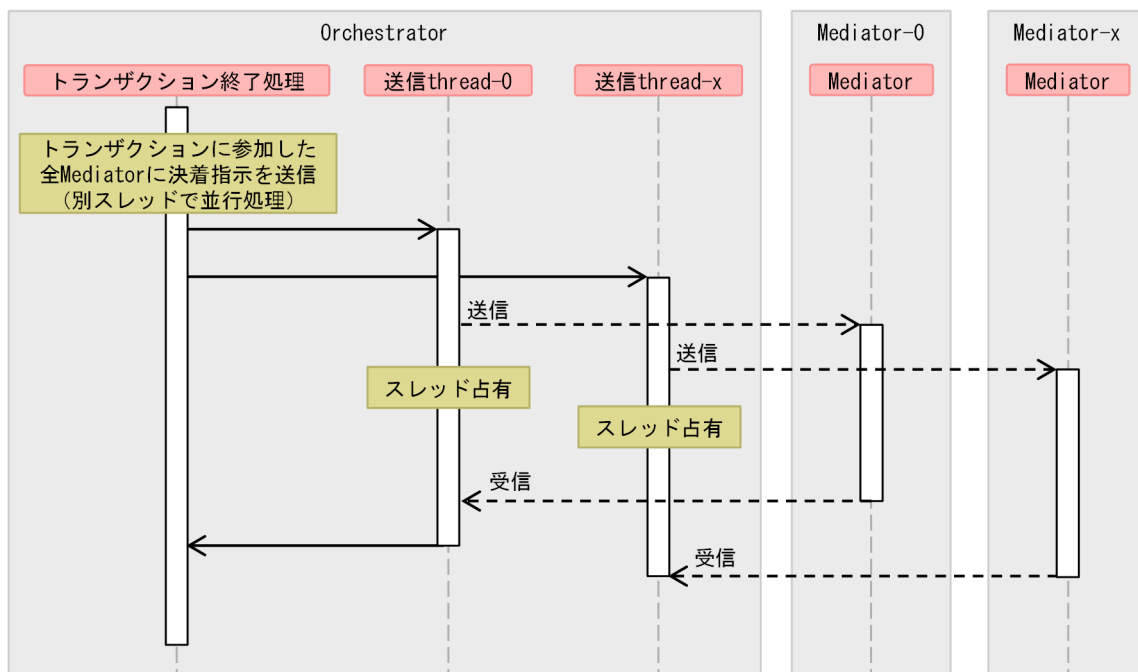
図 3-2 スレッド占有期間
