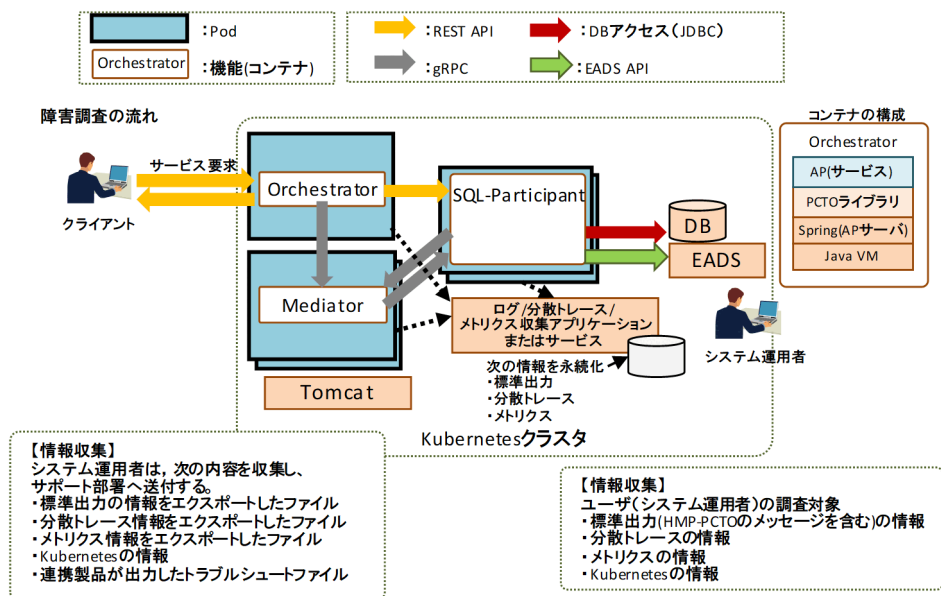
図 11-43 HMP-PCTO 障害発生時の流れ (SQL-Participant を使用する場合)
