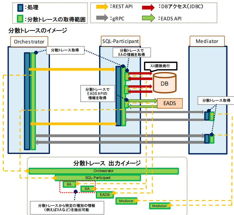
図 11-1 分散トレースのイメージ (SQL-Participant を使用する場合)
