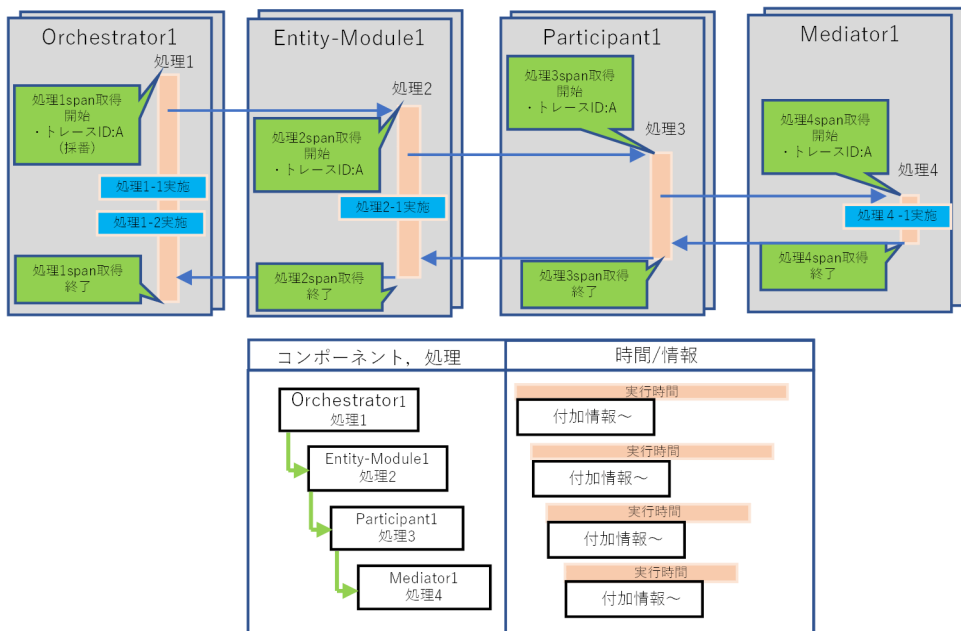
特定トレースIDのspan情報表示イメージ図
