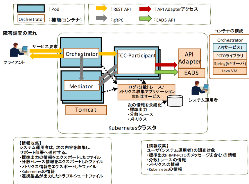
図 11-44 HMP-PCTO 障害発生時の流れ (TCC-Participant を使用する場合)
