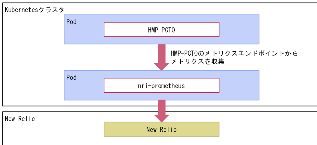
図 11-34 New Relic 使用時の構成図
