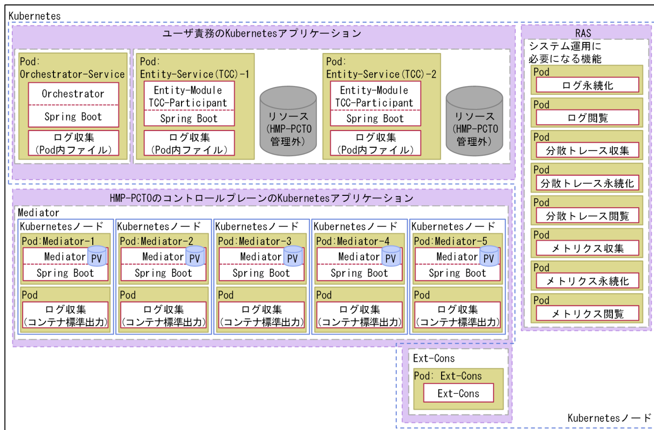
図 1-8 TCC-Participant を使用する場合の最小機器構成（ThreeQuarters 合意方式（トライアル版））
