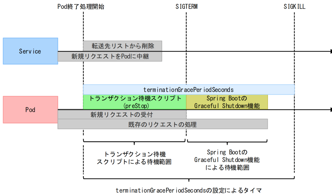
図 7-1 Pod 終了処理時に、未決着トランザクション件数および処理中リクエスト件数が 0 件になるまでの待機範囲
