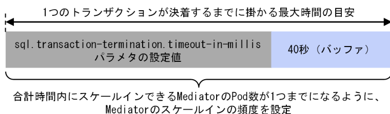
図 4-5 Mediator のスケールインの頻度
