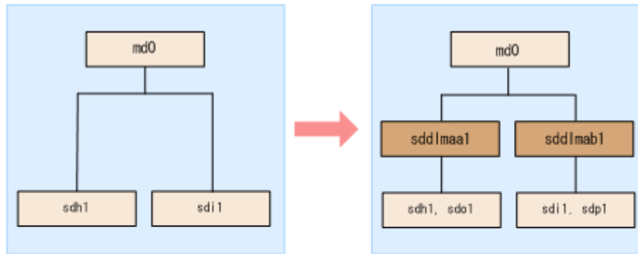
図 3-13 SCSI デバイス上にある md デバイスを HDLM デバイス上に移行した場合のデバイス構成 (md デバイスの RAID 機能を使用した環境)
