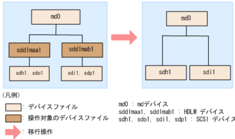
図 3-23 HDLM デバイス上にある md デバイスを SCSI デバイス上に移行する場合のデバイス構成 (md デバイスの RAID 機能を使用した環境)
