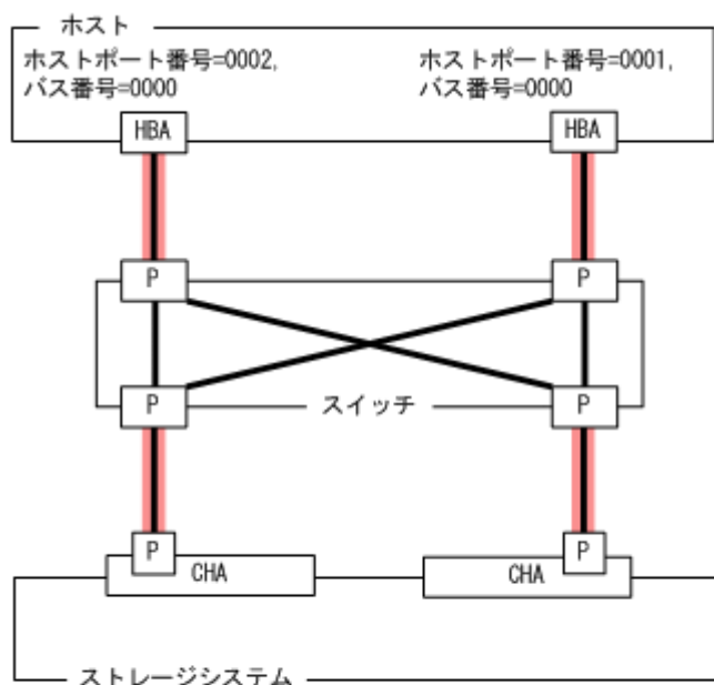
図 4-2 ファイバケーブルを交換する手順説明の前提となるシステム構成
