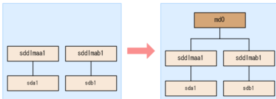
図 3-12 HDLM デバイス上に md デバイスを作成した場合のデバイス構成
