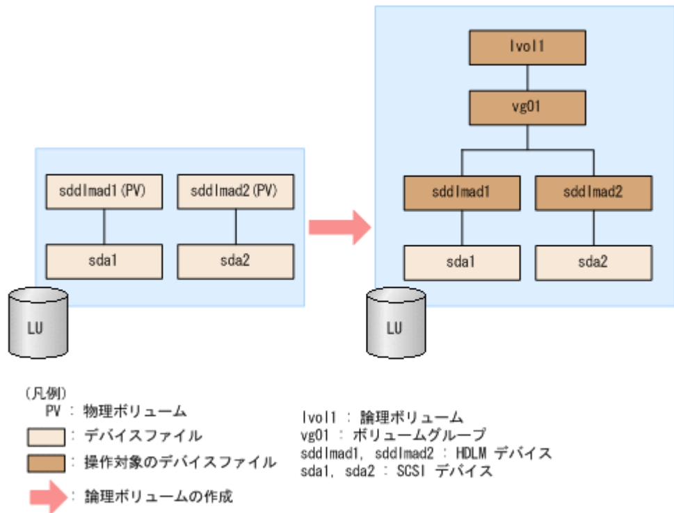
図 3-15 HDLM デバイス上に論理ボリュームを作成した場合のデバイス構成
