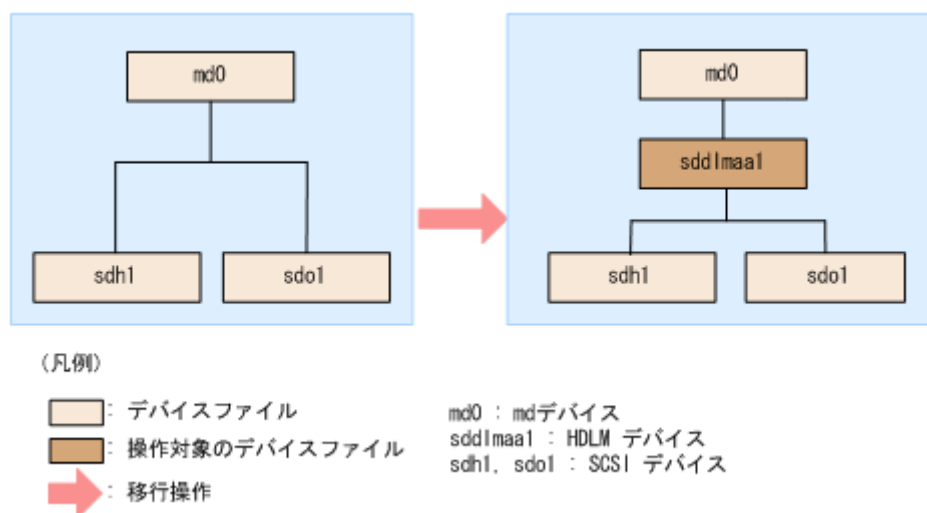
図 3-14 SCSI デバイス上にある md デバイス (md デバイスの MULTIPATH 機能を使用した環境) から HDLM デバイス上に移行した場合のデバイス構成
