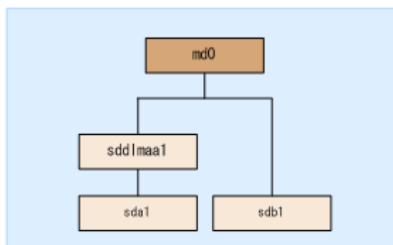
図 3-10 誤った md デバイスの構成例
