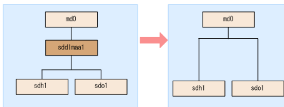
図 3-24 HDLM デバイス上にある md デバイスを SCSI デバイス上に移行する場合のデバイス構成 (md デバイスの MULTIPATH 機能を使用した環境)
