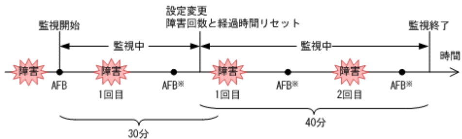
図 13 間欠障害の監視中に間欠障害と見なす条件を変更した場合の動作
