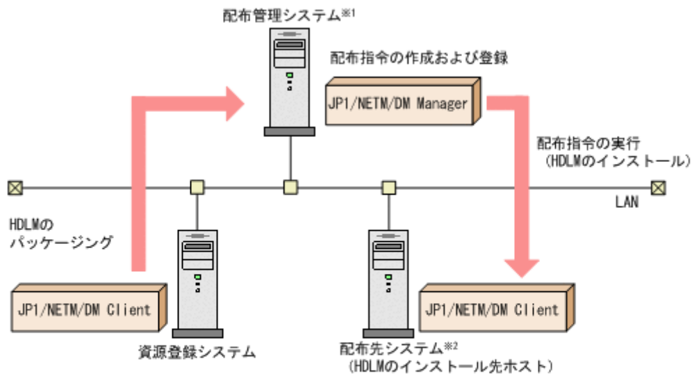
図 19 JP1/NETM/DM を使用して HDLM をリモートインストールする場合のシステム構成
