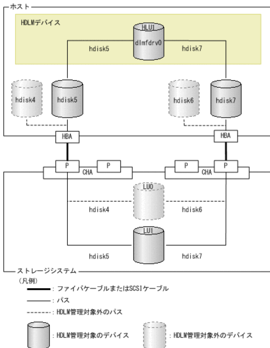
図 21 HDLM デバイス構成後のシステム構成例
