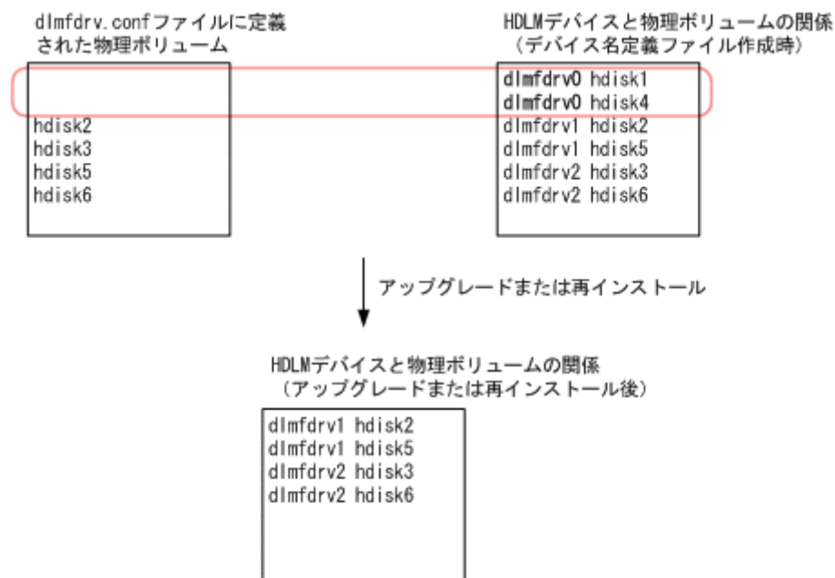
図 29 dlmfdrv.conf ファイルの内容が優先される例
