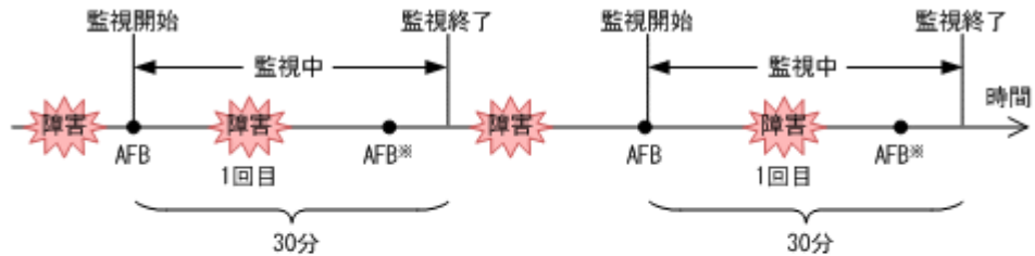
図 12 パスに間欠障害が発生していないと見なす場合の動作
