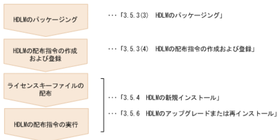
図 18 リモートインストールの流れ
