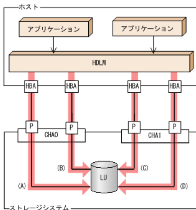
図7 ロードバランス機能を使用している場合の I/O の流れ
