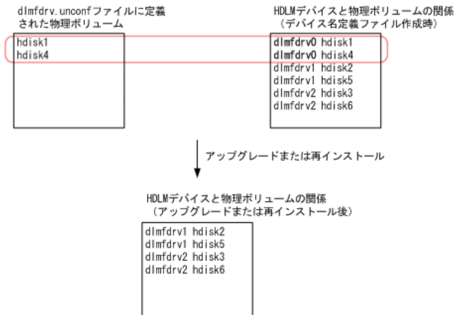
図 30 dlmfdrv.unconf ファイルの内容が優先される例
