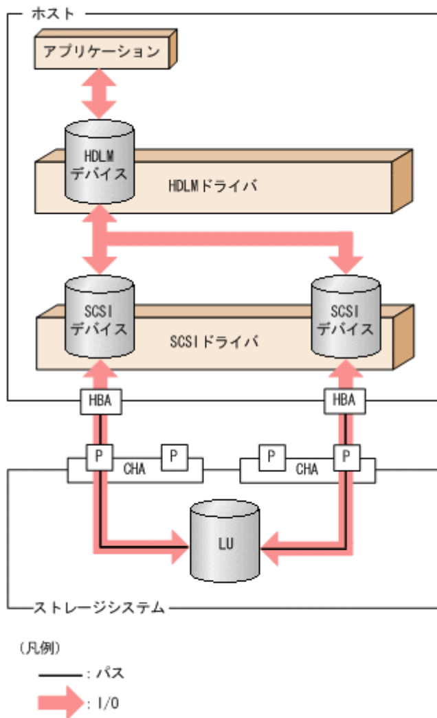
図 5 HDLM ドライバと HDLM デバイスの位置づけ
