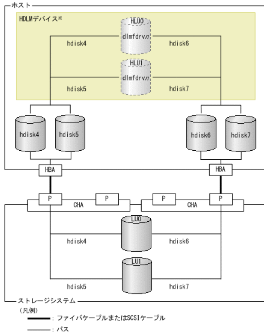
図 20 システム構成例
