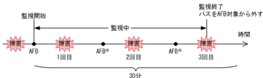
図 11 パスに間欠障害が発生していると思なす場合の動作
