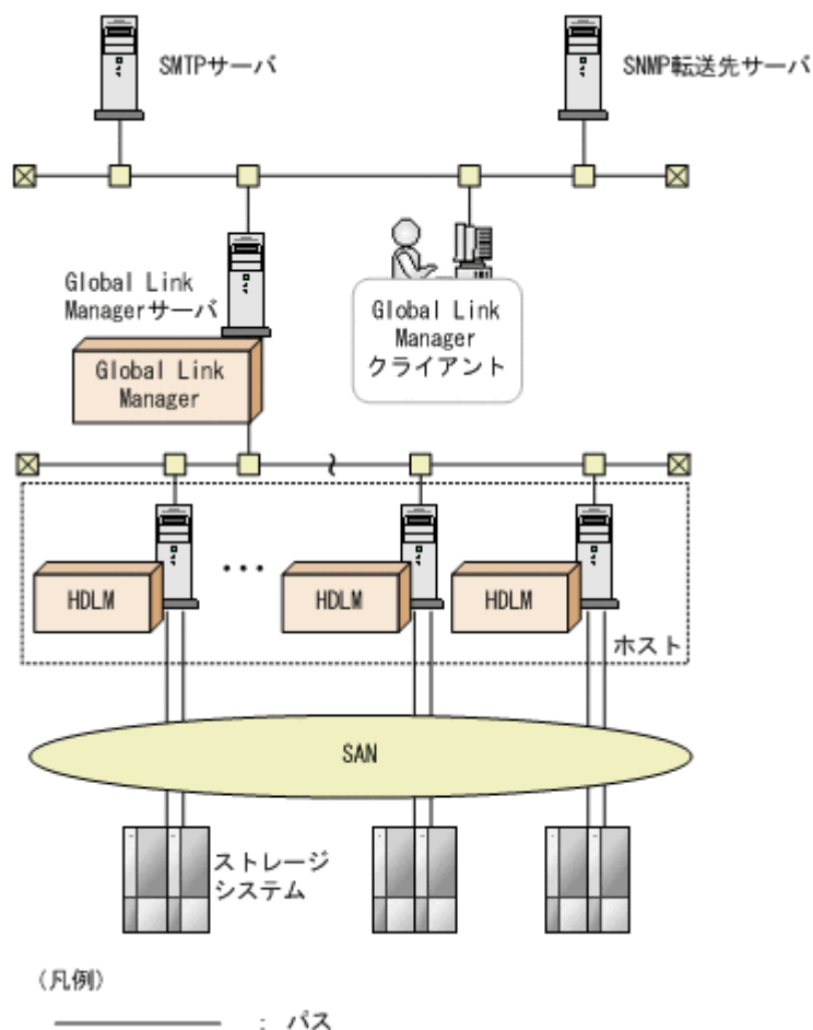
図 15 HDLM と Global Link Manager を使用したシステム構成例
