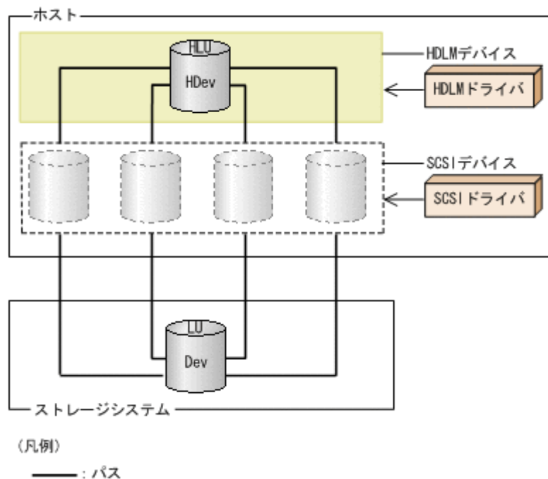
図 3 HDLM をインストールしたあとにホスト側で認識される LU の構成
