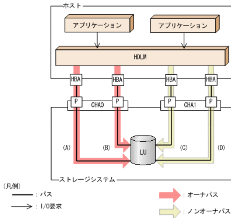
図 8 オーナパスとノンオーナパスがある場合のロードバランス
