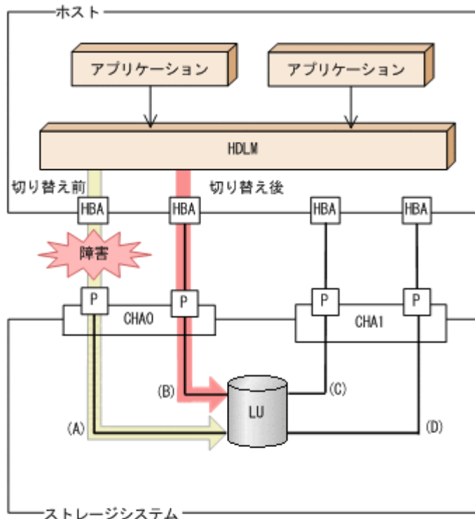
図9 パスの切り替え
