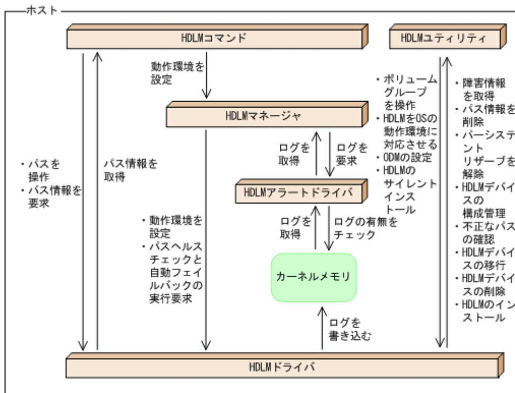
図 4 HDLM のプログラム構成
