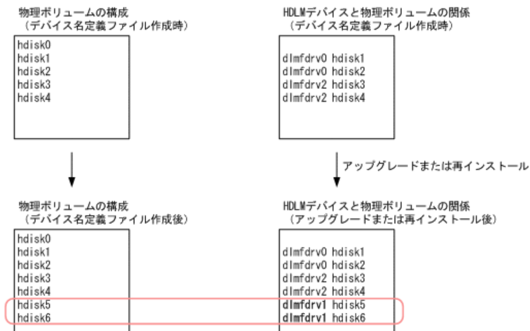
図 28 HDLM が HDLM デバイスの名称を定義する例
