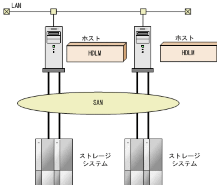
図 1 ホストとストレージシステムとの接続形態
