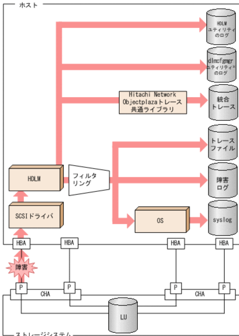
図 14 障害情報を採取するときのデータの流れ
