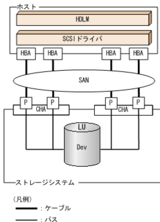
図 2 HDLM のシステム構成
