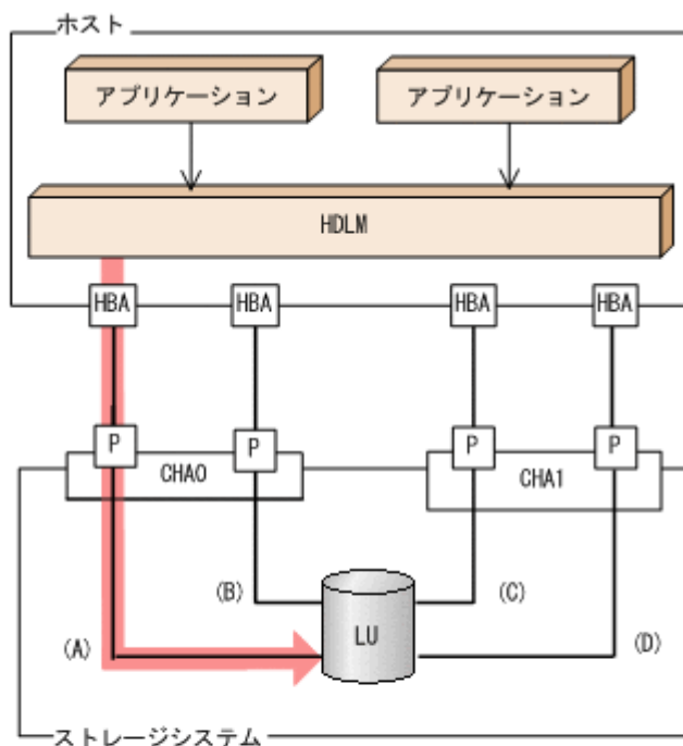
図 6 ロードバランス機能を使用していない場合の I/O の流れ
