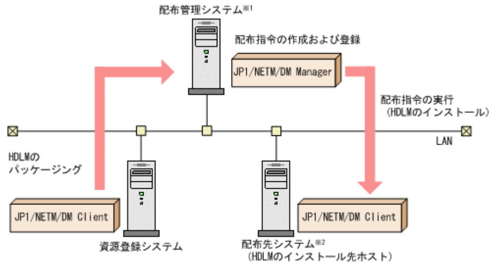
図 3-4 JP1/NETM/DM を使用して HDLM をリモートインストールする場合のシステム構成
