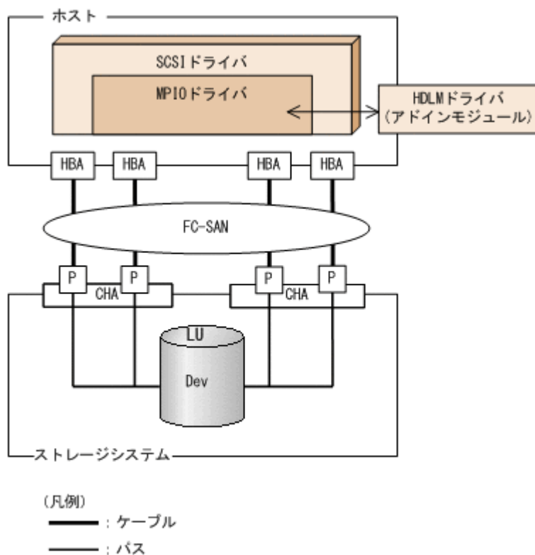
図 2-1 HDLM のシステム構成
