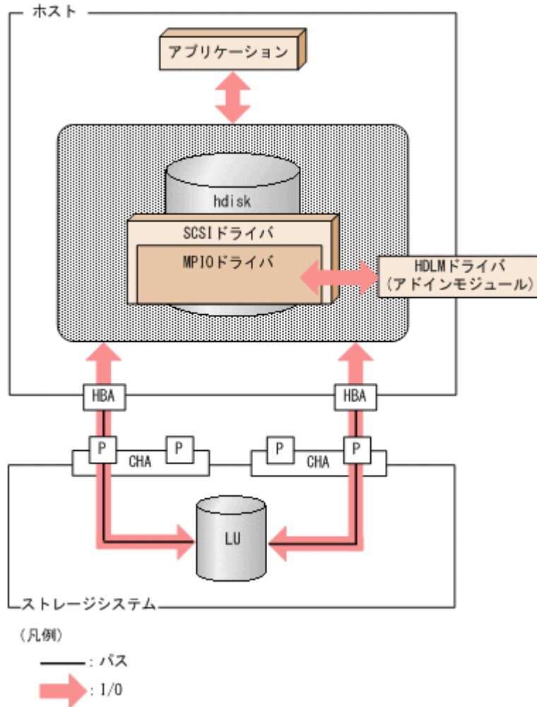
図 2-4 HDLM ドライバと hdisk の位置づけ
