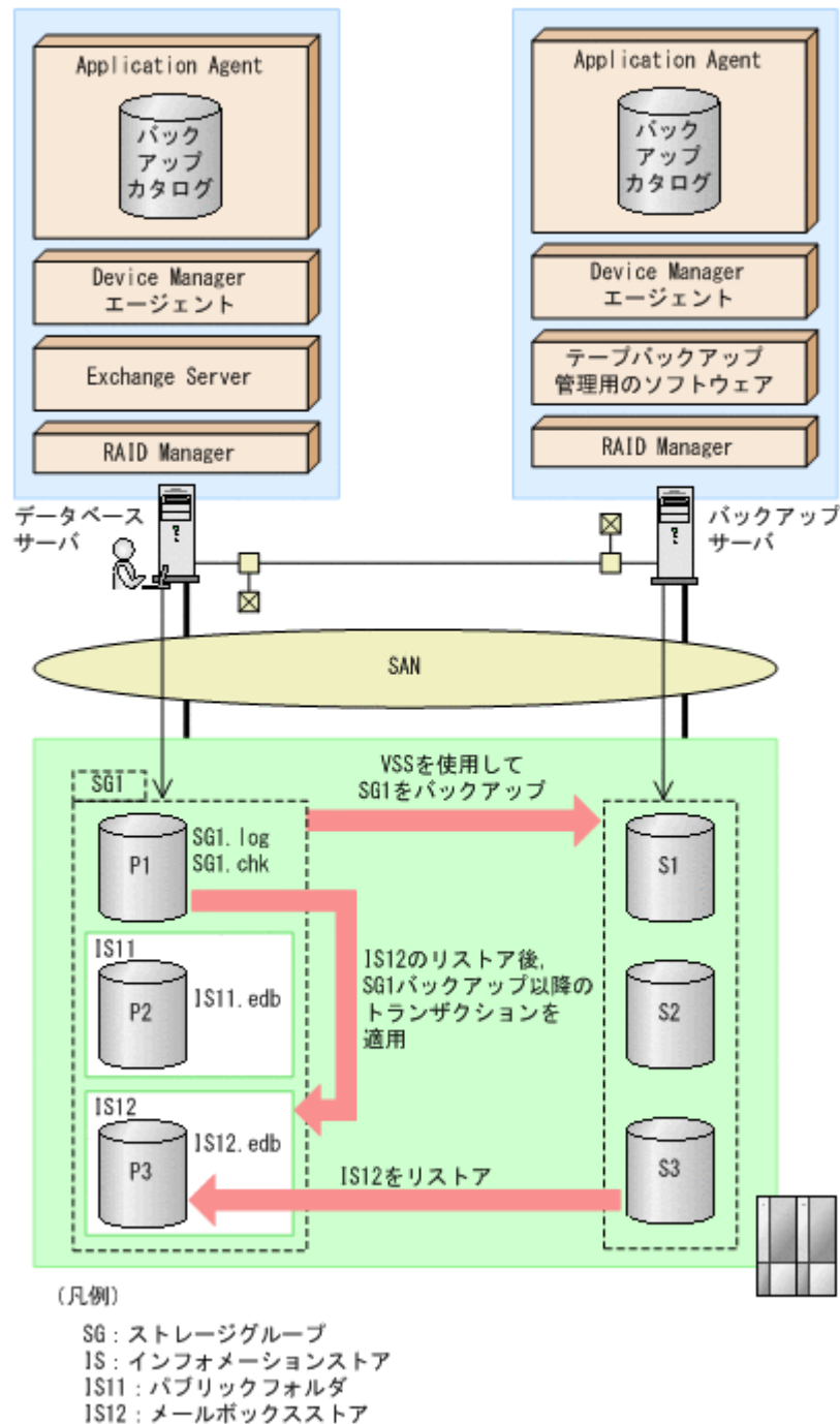
図 7-10 トランザクションログを適用してインフォメーションストア単位でリストアするシステム構成
