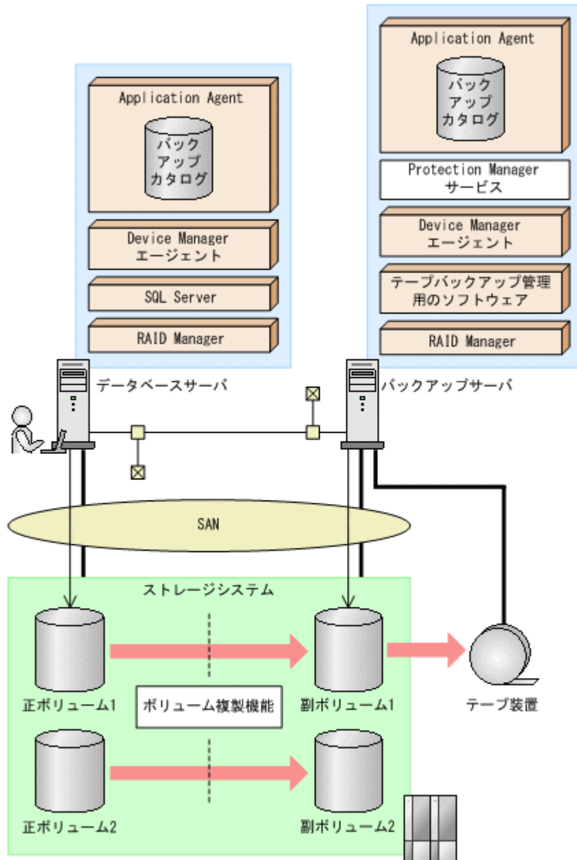
図 6-16 SQL Server データベースをテープへバックアップするためのシステム構成
