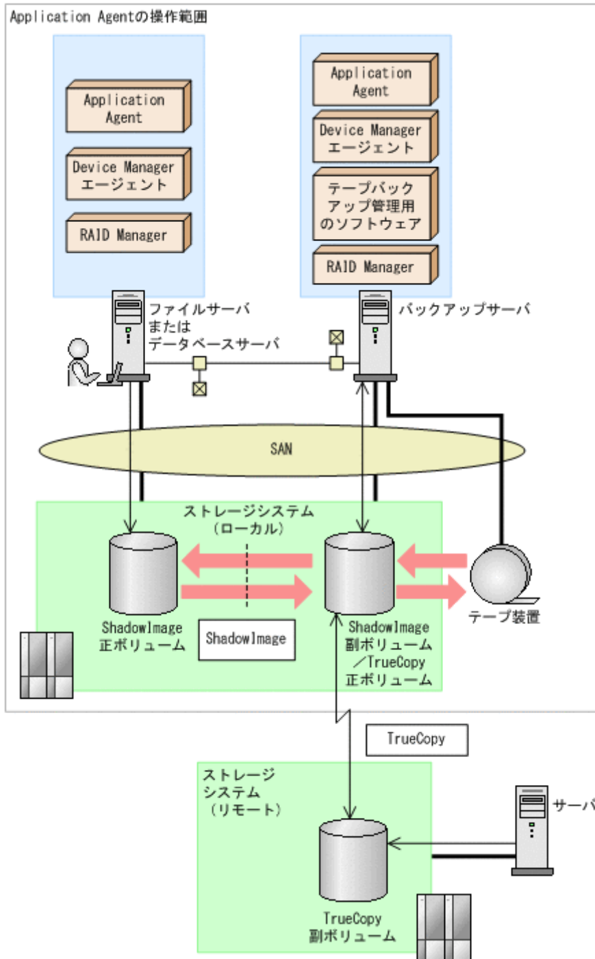
図 2-31 システム構成 (ShadowImage の副ボリュームと TrueCopy の正ボリュームが同じ LDEV の場合)で Application Agent が ShadowImage のペアボリュームをバックアップまたはリストアする場合、TrueCopy のペアボリュームの状態は SMPL または PSUS (SSUS) にしてください。TrueCopy のペアボリュームの状態が PAIR のままで ShadowImage のペアボリュームをバックアップまたはリストアすると、コピーグループの状態が不正であることを表すエラーメッセージが出力され、バックアップまたはリストアが失敗します。
