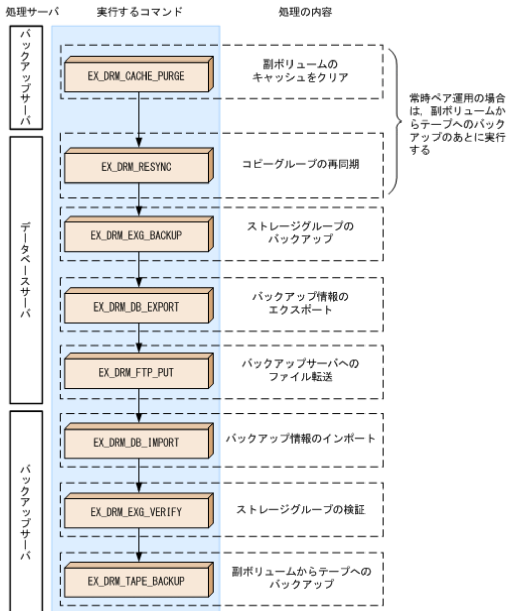
図 7-5 ストレージグループをテープにバックアップする処理の流れ
