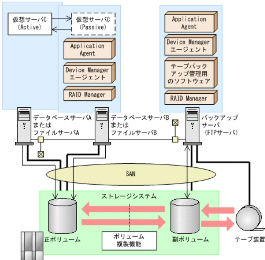
図 2-9 運用待機型のクラスタ構成例 (Active-Passive)
