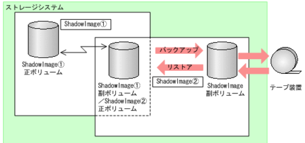
図 2-32 システム構成 (ShadowImage のカスケード構成で、バックアップ対象のボリュームが正ボリュームと副ボリュームを兼ねている場合)
