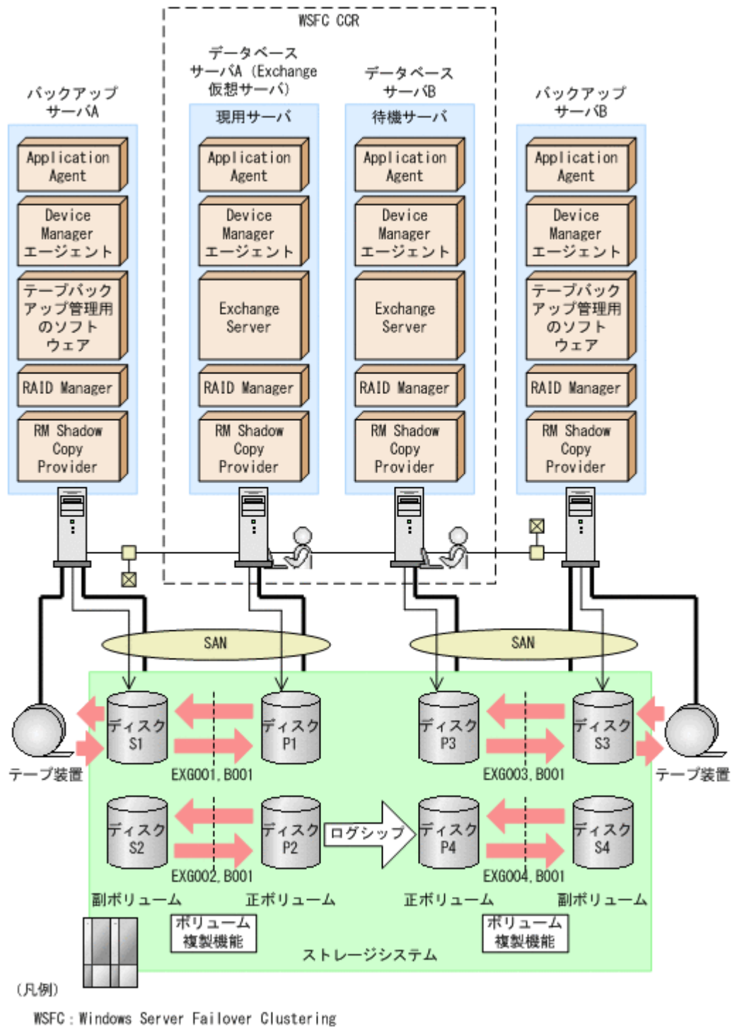
図 7-12 CCR 構成でバックアップおよびリストアする場合のシステム構成例
