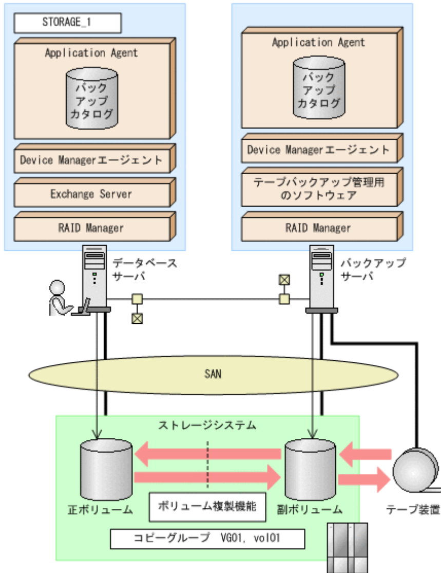
図 7-4 ストレージグループをテープへバックアップ，リストアするためのシステム構成
