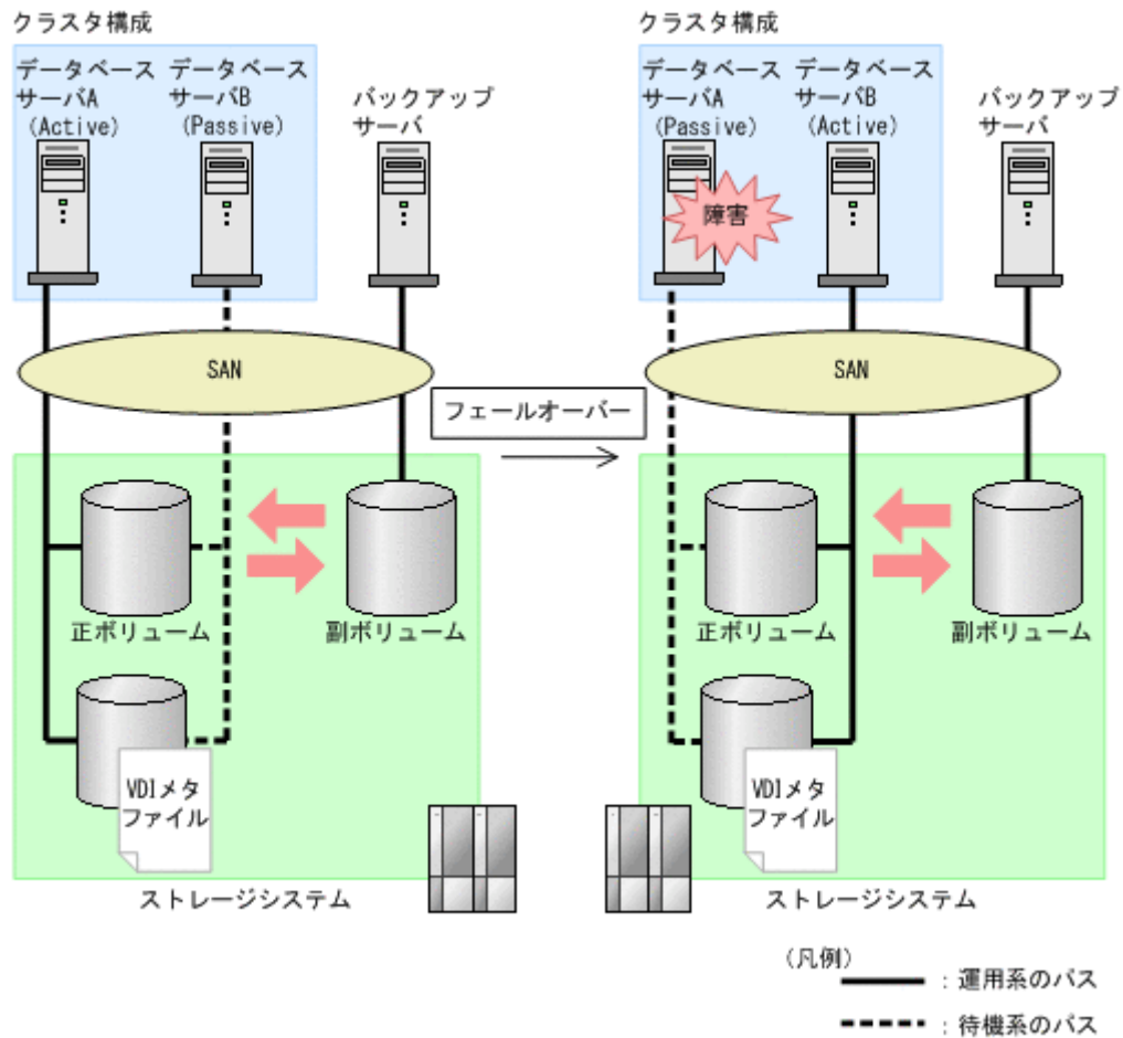
図 2-18 VDI メタファイルの配置 (クラスタ構成の場合)
