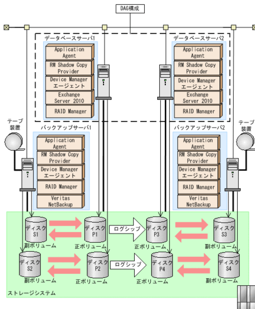
図 7-14 DAG 構成でバックアップおよびリストアする場合のシステム構成
