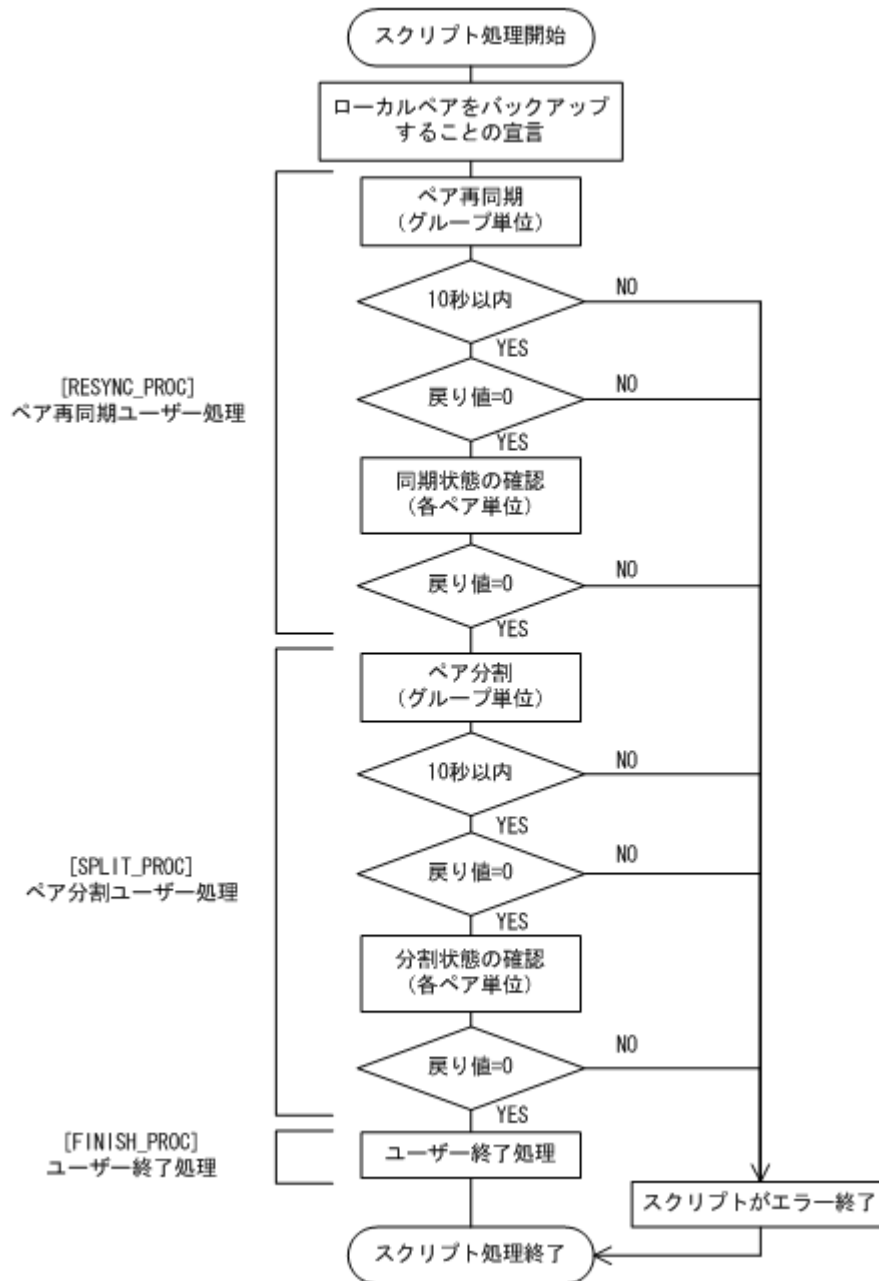
図 6-33 ローカルバックアップする場合のスクリプト内の処理フロー図
