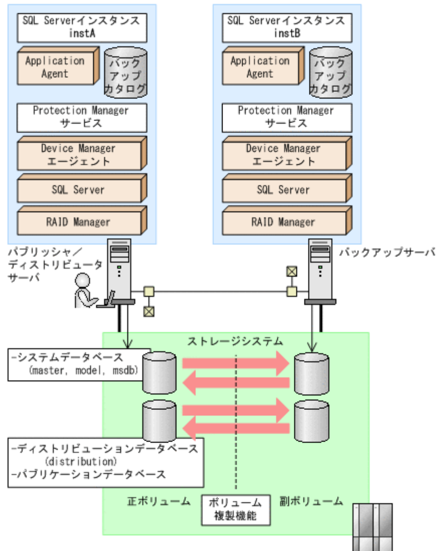
図 6-38 パブリッシャ/ディストリビュータサーバと対応するバックアップサーバの構成
