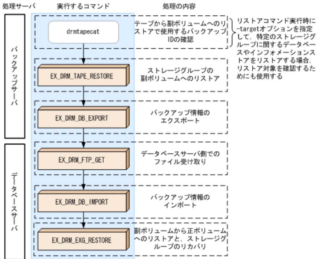
図 7-6 ストレージグループをテープからリストアする処理の流れ
