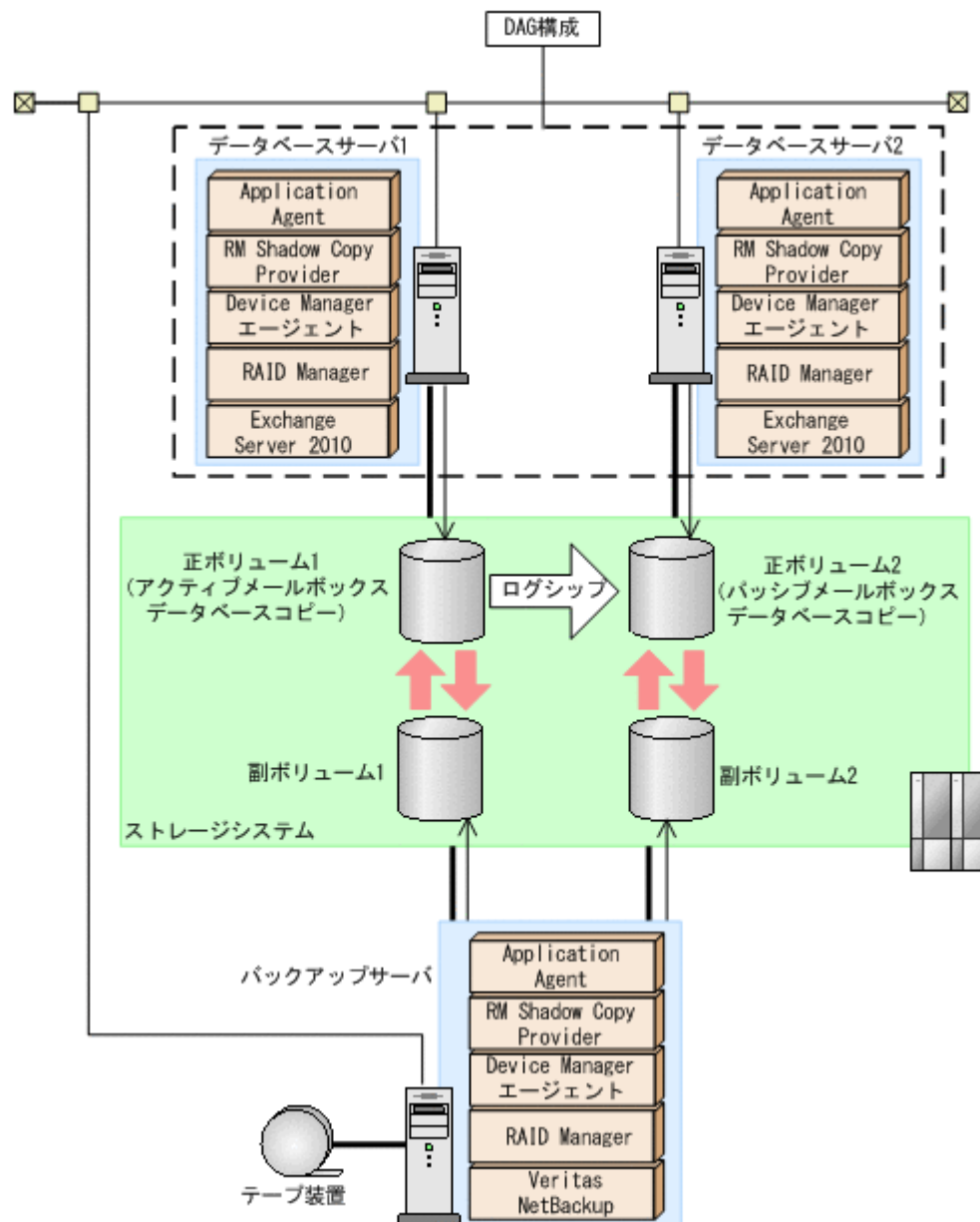
図 2-27 アクティブメールボックスデータベースコピーとパッシブメールボックスデータベースコピーで同じバックアップサーバを使用した構成
