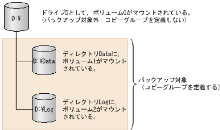
図 2-35 バックアップ対象となるディレクトリマウントの構成例
