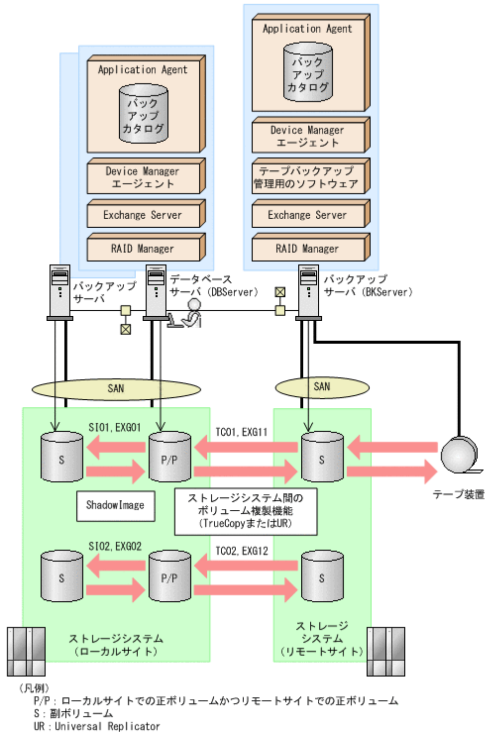
図 7-11 ローカルサイトとリモートサイトの間でストレージグループをバックアップおよびリストアする場合はシステム構成例
