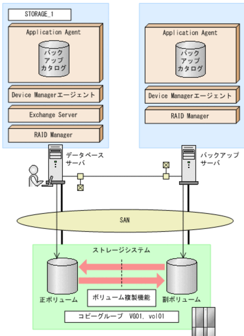
図 7-1 VSS を使用してボリューム間でデータをバックアップおよびリストアする場合のシステム構成（バックアップ対象が Exchange データベースの場合）
