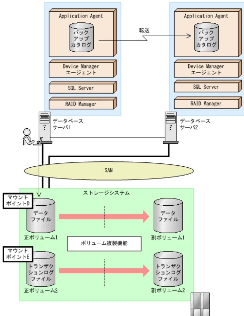
図 6-25 バックアップ時のシステム構成例
