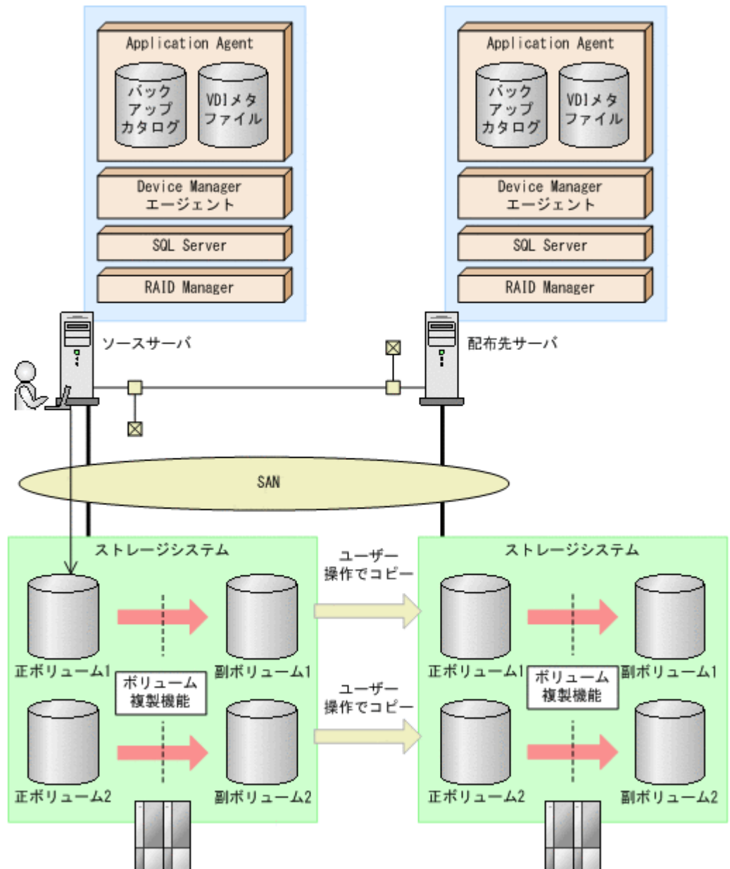
図 6-27 ログ配布機能を使用するためのシステム構成例
