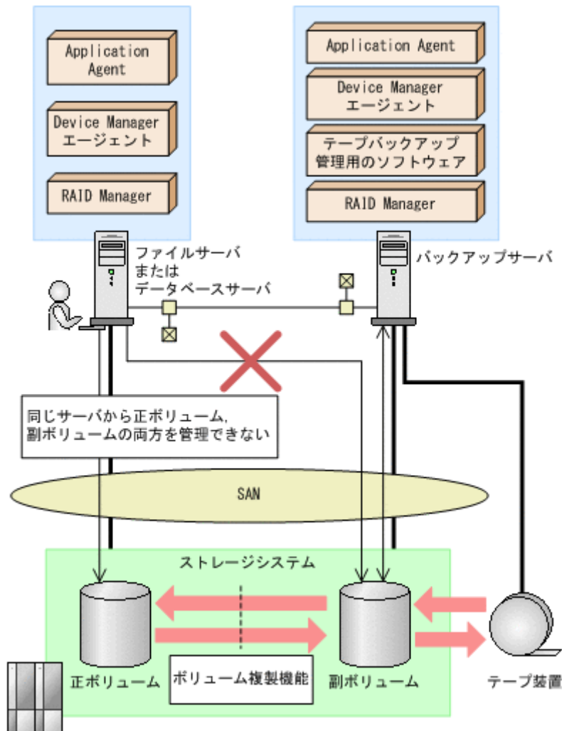
図 2-29 同じサーバから正ボリューム、副ボリュームを管理する構成（Application Agent 適用外）
