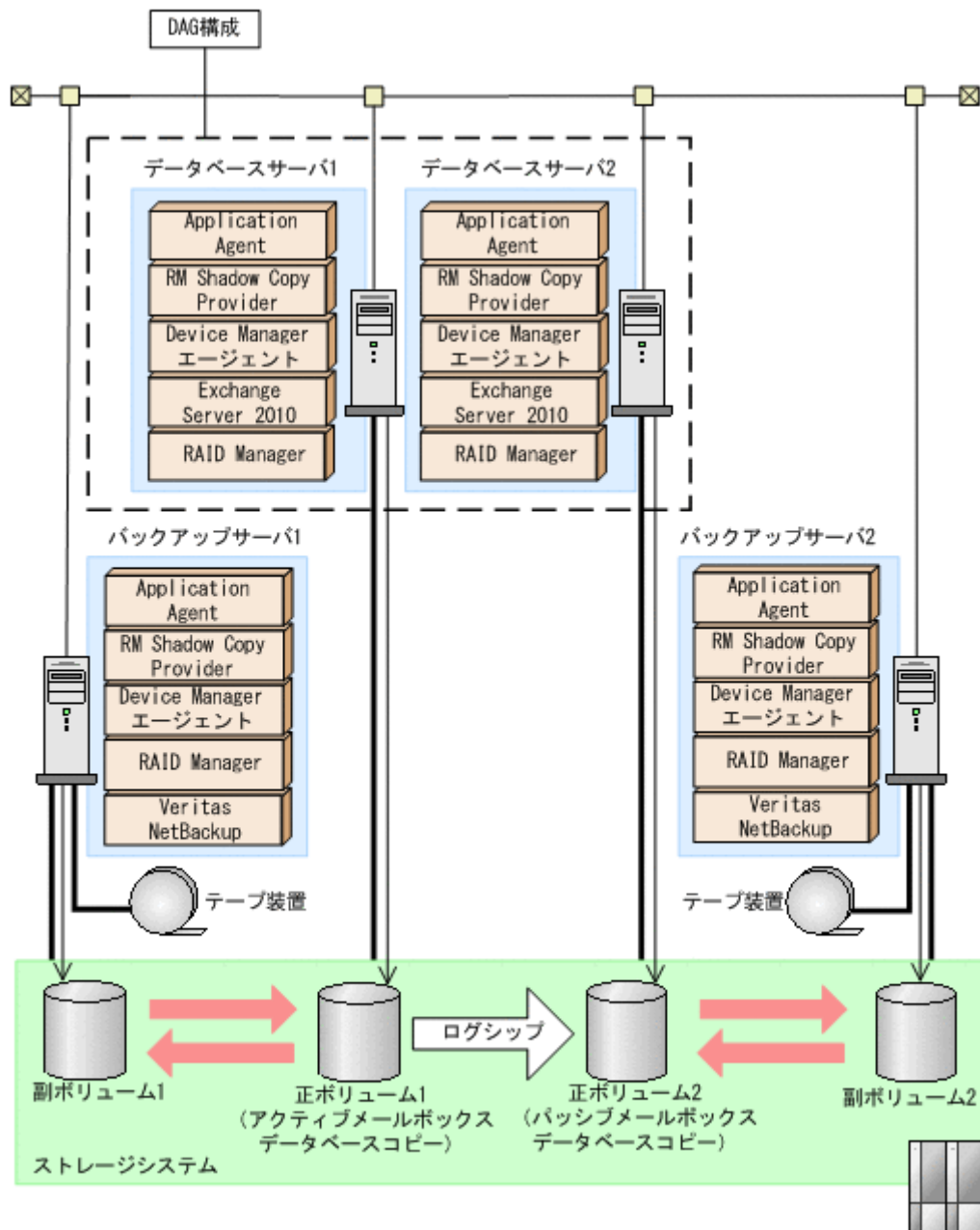
図 2-26 アクティブメールボックスデータベースコピーとパッシブメールボックスデータベースコピーで異なるバックアップサーバを使用した構成
