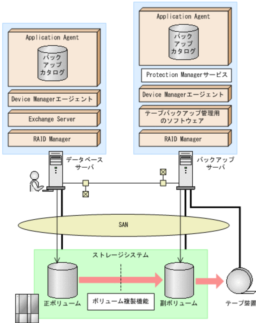
図 7-7 ストレージグループをテープへバックアップするためのシステム構成
