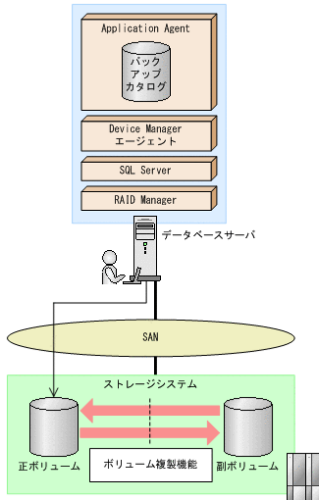
図 6-10 ボリューム間でデータをバックアップおよびリストアする場合のシステム構成 (バックアップ対象が SQL Server データベースの場合)
