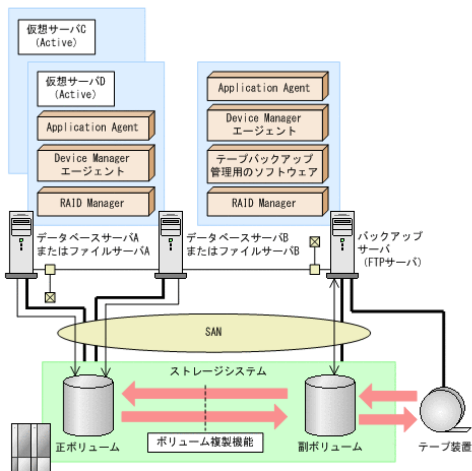
図 2-10 相互待機型のクラスタ構成例 (Active-Active)
