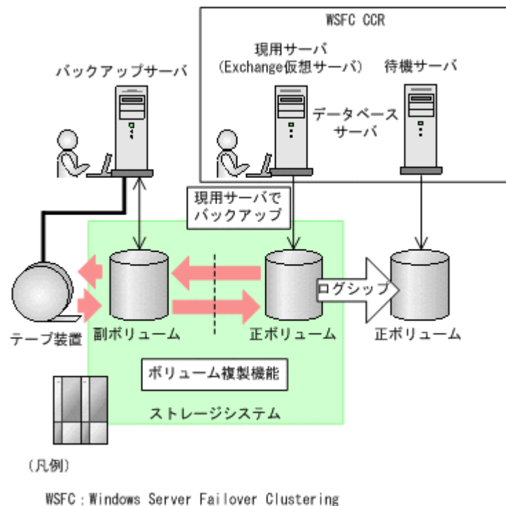
図 2-19 CCR 構成例 (現用サーバだけを使用した場合)
