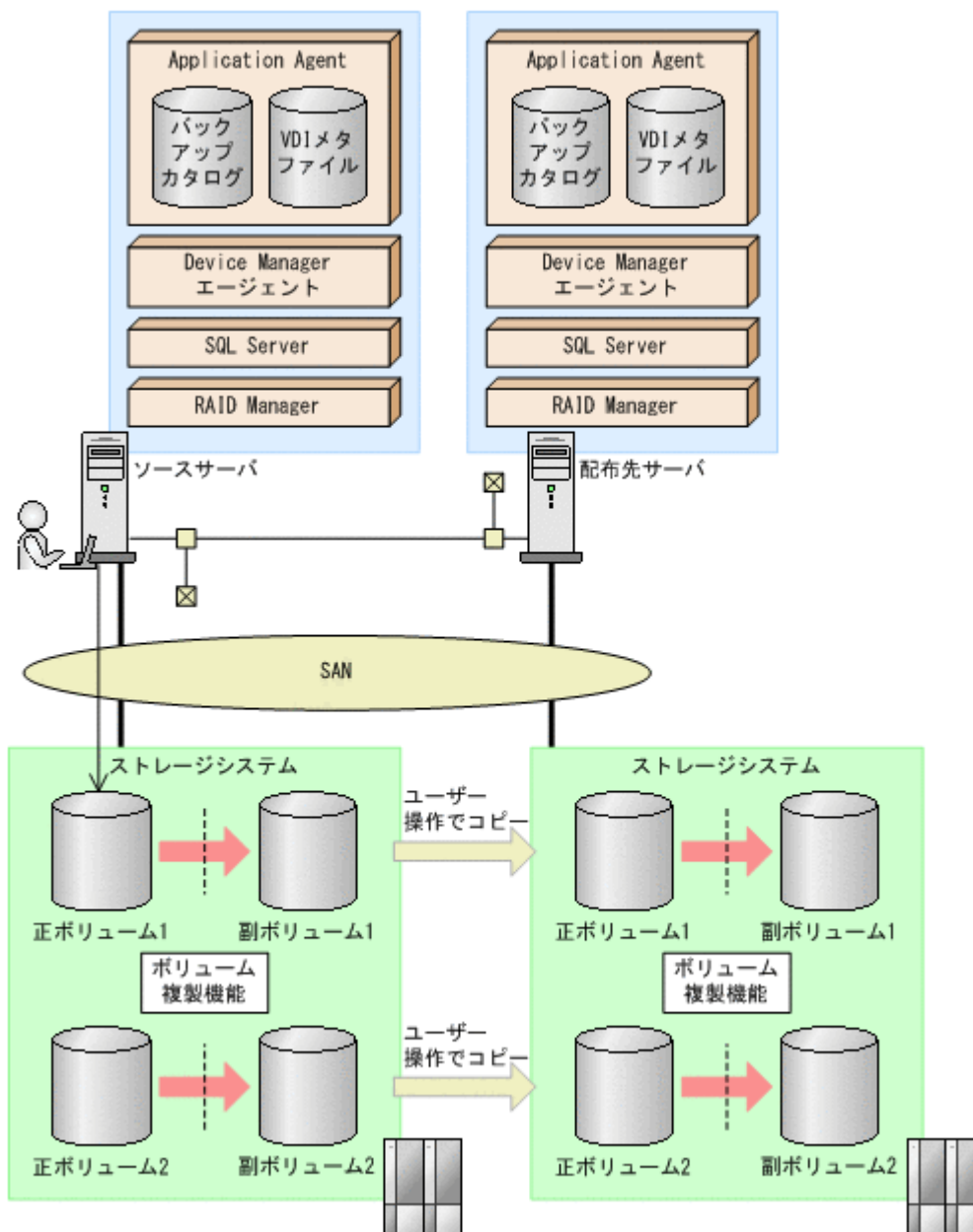
図 2-13 ログ配布機能を使用する場合のシステム構成例
