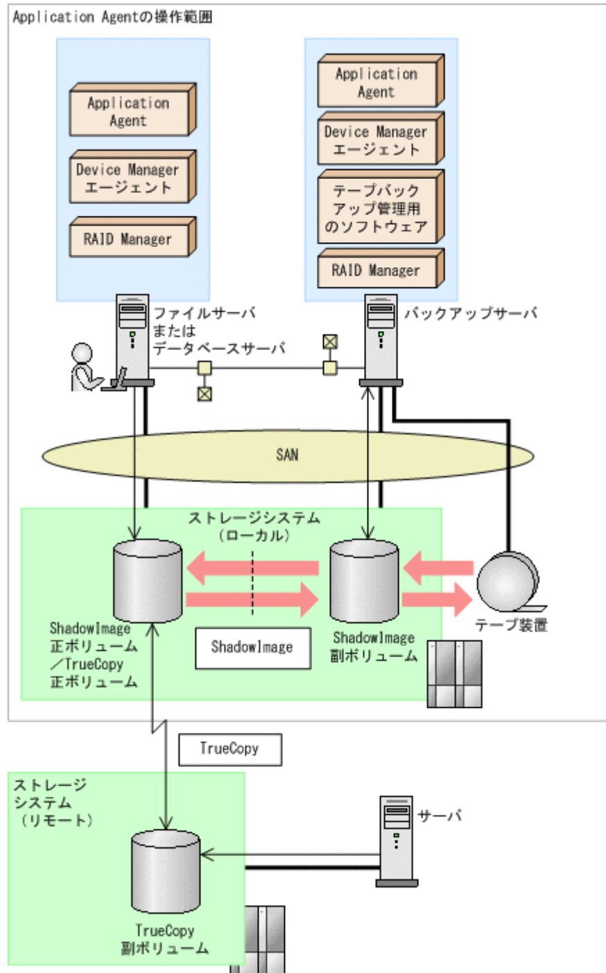
図 2-30 システム構成 (ShadowImage のペアボリュームと TrueCopy のペアボリュームが同じ LDEV の場合) で Application Agent が ShadowImage のペアボリュームをリストアする場合、TrueCopy のペアボリュームの状態は SMPL または PSUS (SSUS) にしてください。TrueCopy のペアボリュームの状態が PAIR のままで ShadowImage のペアボリュームをリストアすると、コピーグループの状態が不正であることを表すエラーメッセージが出力され、リストアが失敗します。
