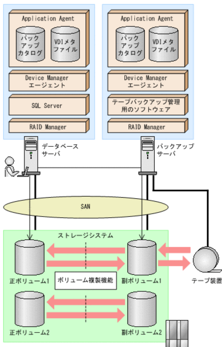
図 6-13 SQL Server データベースをテープへバックアップ、リストアするためのシステム構成
