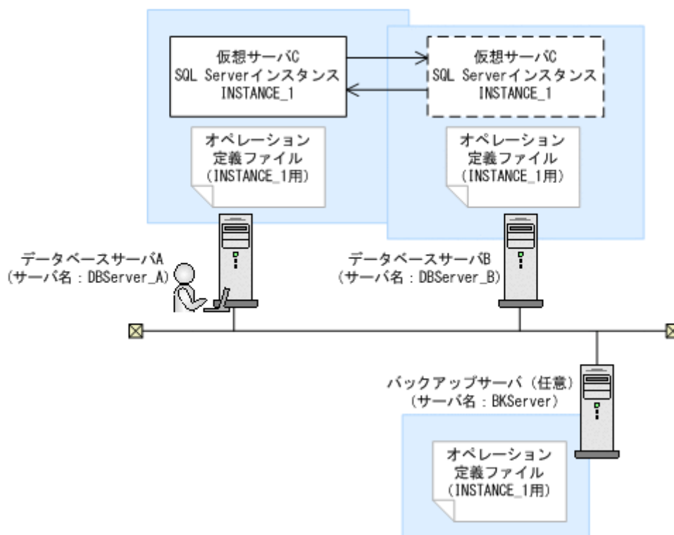
図 3-12 オペレーション定義ファイルの配置例（バックアップ対象が SQL Server データベースの場合）
