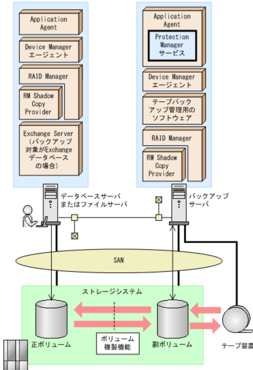
図 2-11 VSS を使用した場合のシステム構成例
