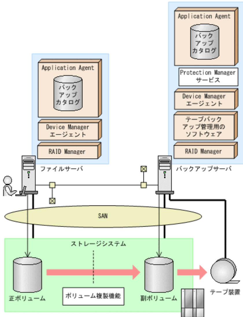
図 5-7 ファイルシステムをテープへバックアップするためのシステム構成
