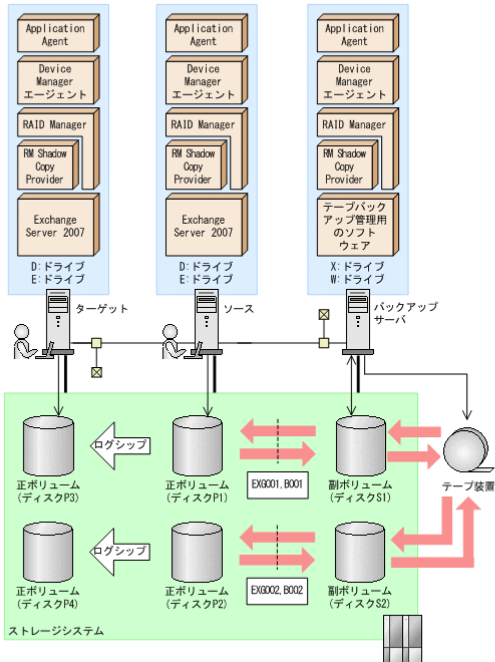
図 7-13 SCR のシステム構成
