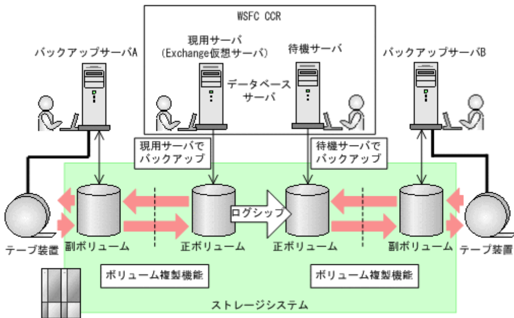
図 2-21 CCR 構成例（現用サーバと待機サーバで異なるバックアップサーバを使用する場合）
