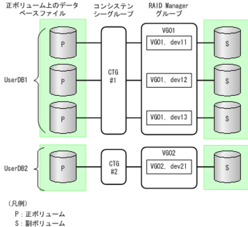
図 2-34 TrueCopy Async / Universal Replicator 構成で、UserDB1 と UserDB2 を同時にリストアする運用の場合
