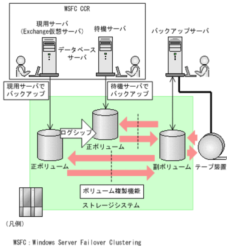
図 2-22 CCR 構成例（現用サーバと待機サーバで同じバックアップサーバを使用する場合）
