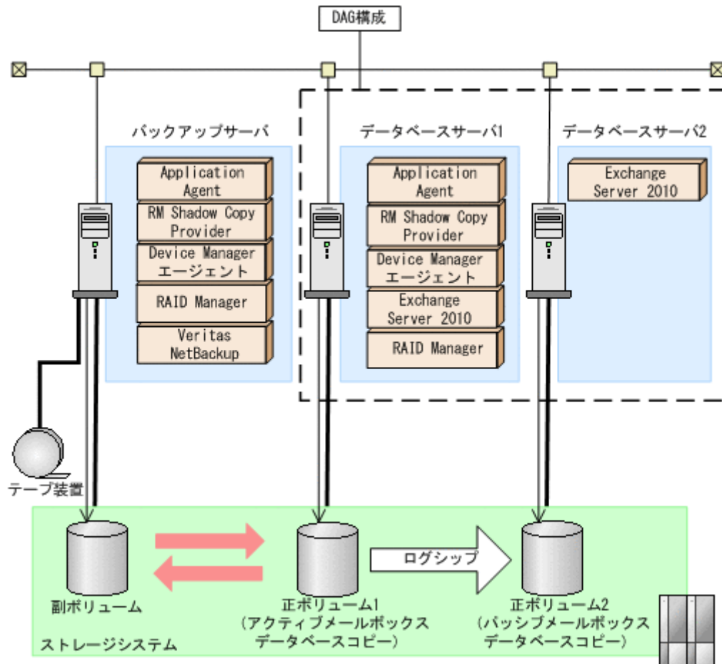
図 2-24 アクティブメールボックスデータベースコピーをバックアップおよびリストアする構成
