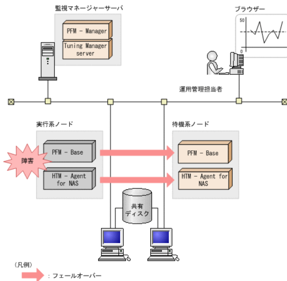
図 1-2 クラスタシステムの運用例 (HTM - Agent for NAS の場合)
