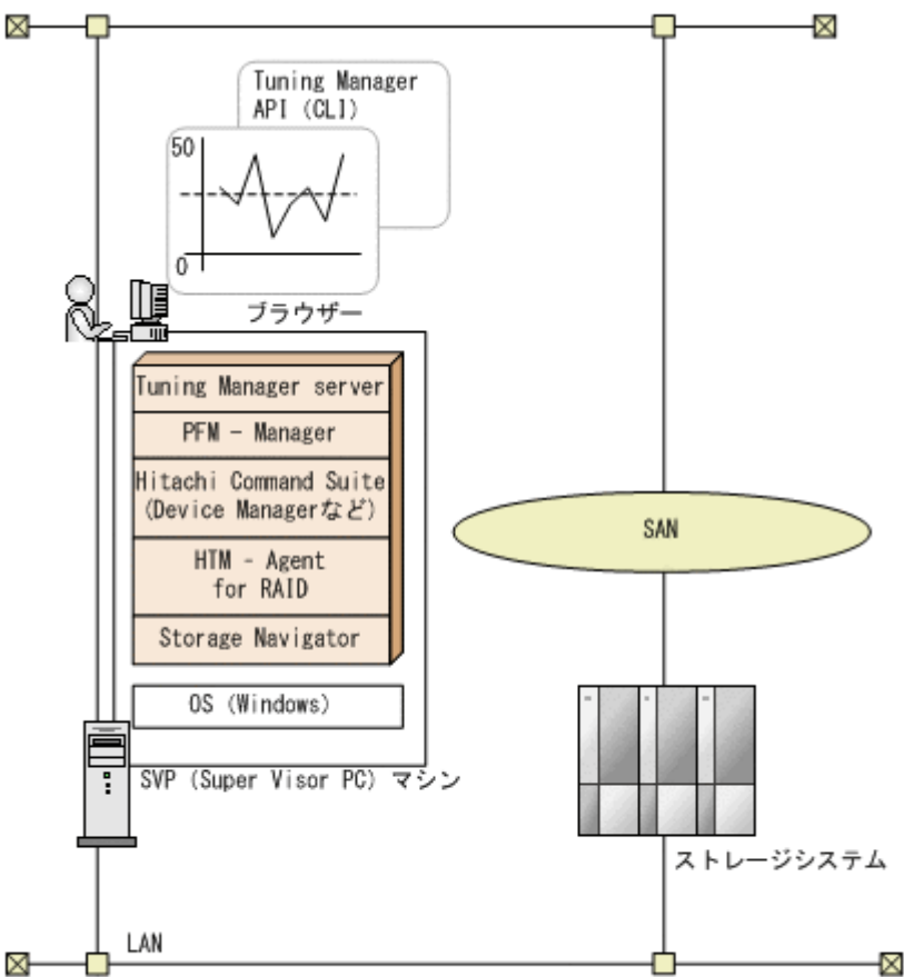
図 B-1 Tuning Manager シリーズのシステム構成例（機能を限定して省物理メモリー環境で Tuning Manager シリーズを運用する場合）
