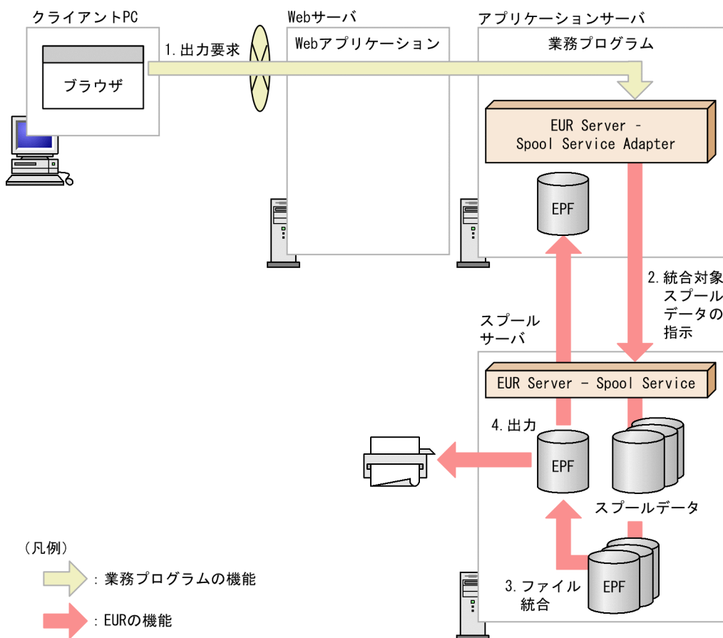
図 6-6 複数のスプールデータを統合出力する流れ
