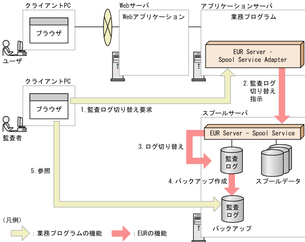
図 13-3 監査ログ参照の流れ（監査ログを業務プログラムで管理する場合）
