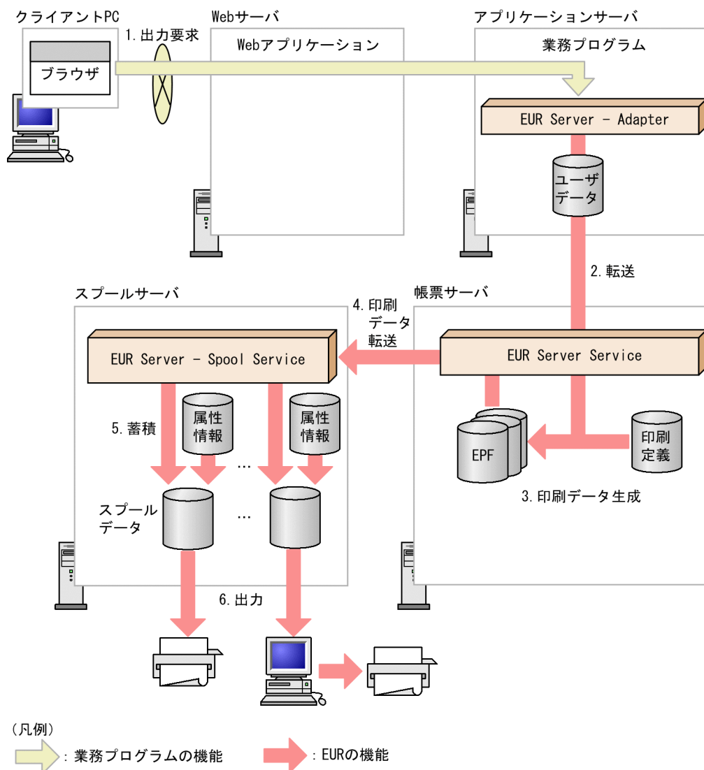
図 6-4 帳票を分割して出力する流れ
