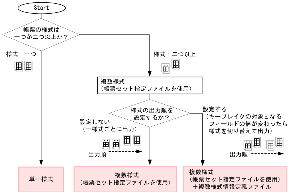
図 2-5 帳票様式を決定するまでの流れ
