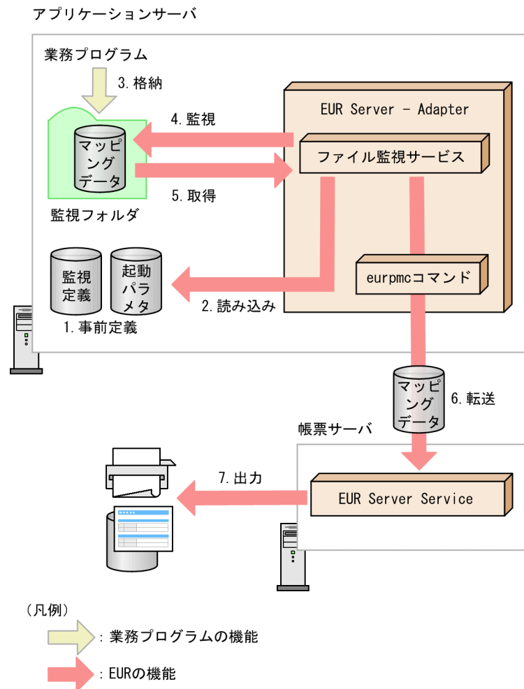
図 8-1 事前定義型の場合の帳票自動出力の流れ
