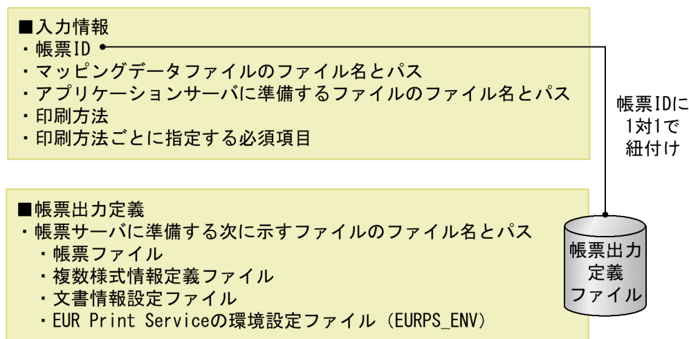
図 2-4 帳票出力時の起動部品の入力情報と帳票出力定義 (帳票 ID を使用する場合)
