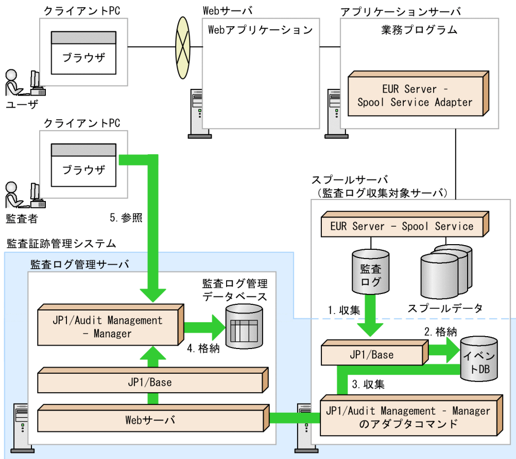
図 13-2 監査ログ切り替えの流れ（監査証跡管理システムと連携する場合）
