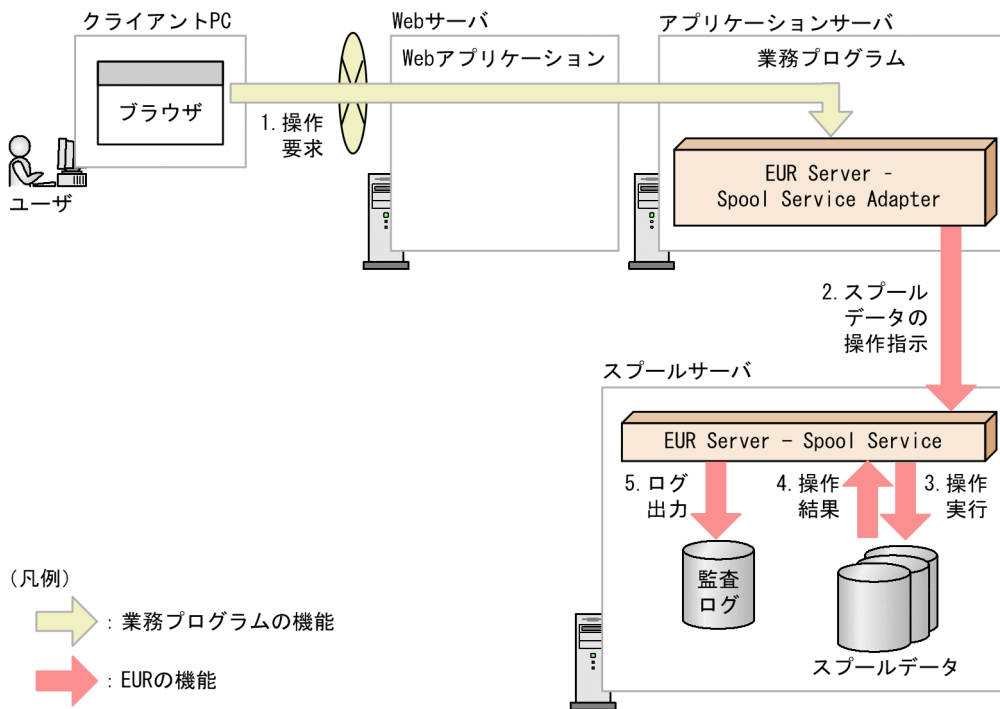
図 13-1 監査ログ出力の流れ
