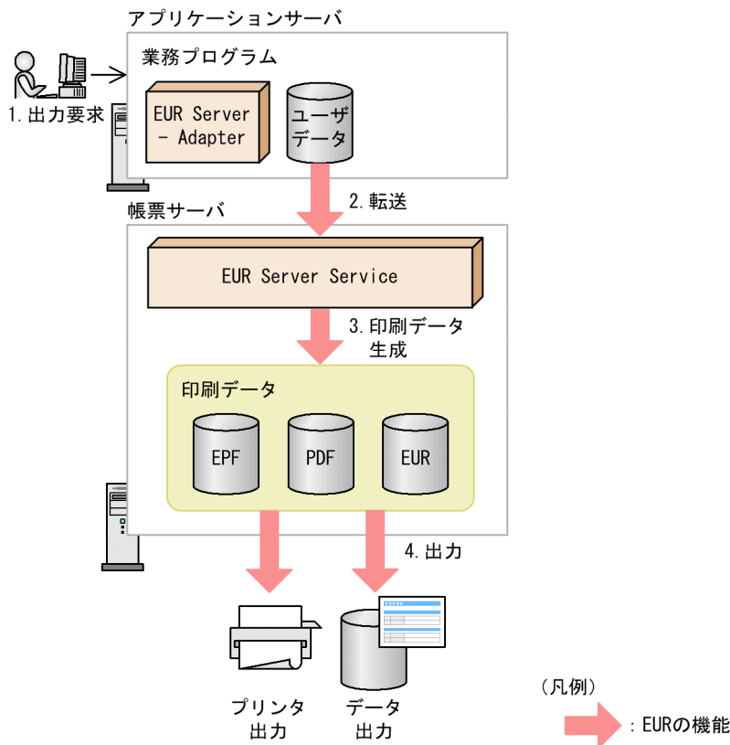
図 10-1 複数様式で帳票を出力する流れ
