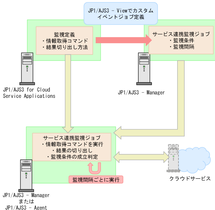
図 6-1 監視処理の実行の流れ
