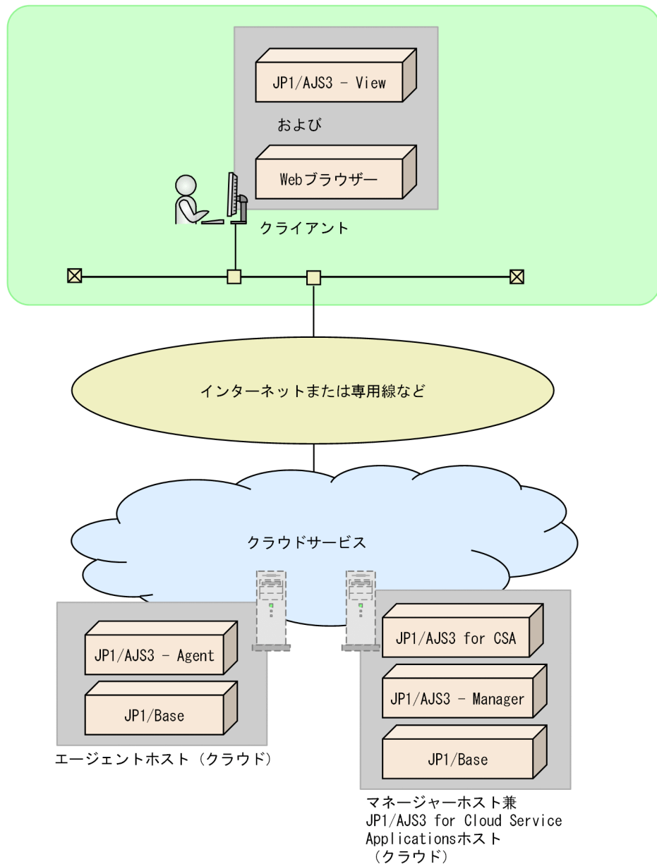
図 2-7 JP1/AJS3 for Cloud Service Applications を JP1/AJS3 - Manager と同一のクラウドホスト上に構築するシステム構成例
