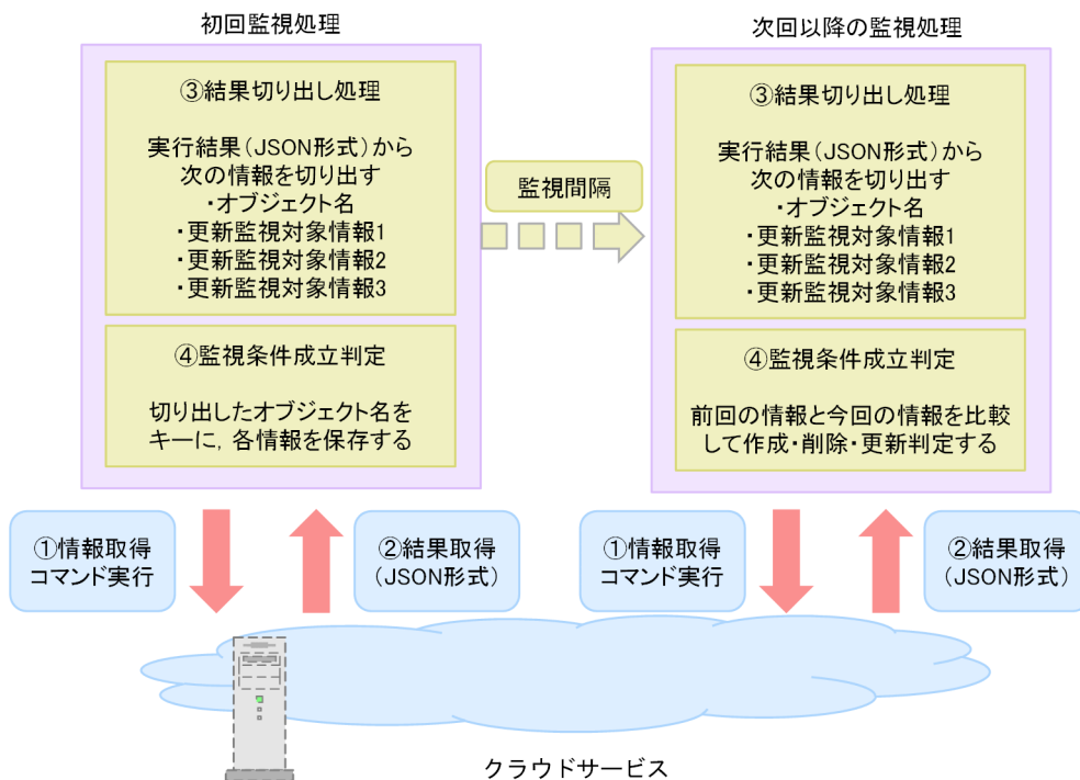
図 6-2 イベント検知処理の詳細
