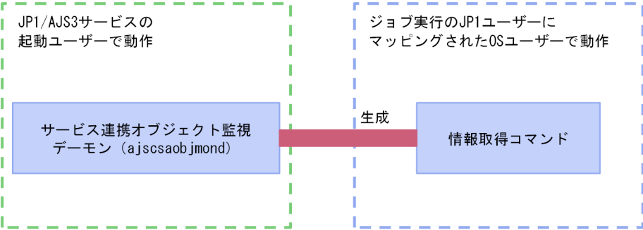
図 6-3 サービス連携オブジェクト監視ジョブの実行時の OS ユーザー
