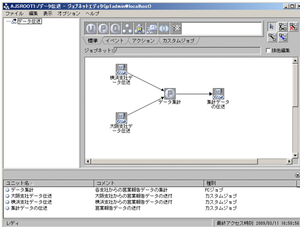
図 5-6 ジョブネット設定例
