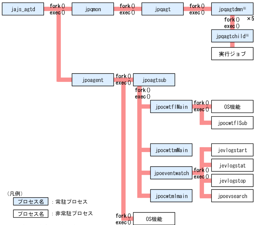
図 B-4 JP1/AJS3 のプロセス構成 (子プロセスおよび詳細プロセス) (3/3)
