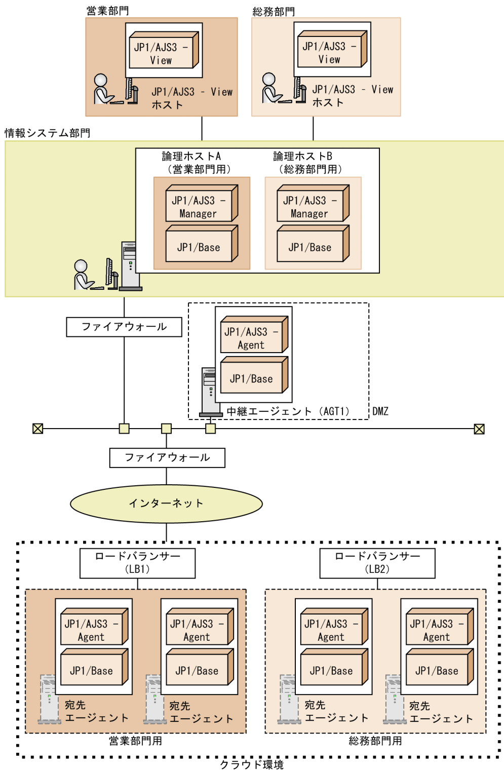
図 13-18 ジョブの実行環境をクラウド化した例
