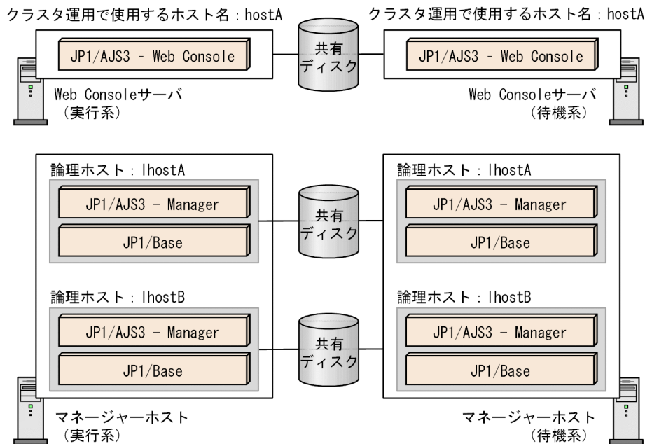
図 10-2 JP1/AJS3 - Web Console と JP1/AJS3 - Manager を異なるサーバにクラスタを構築する場合
