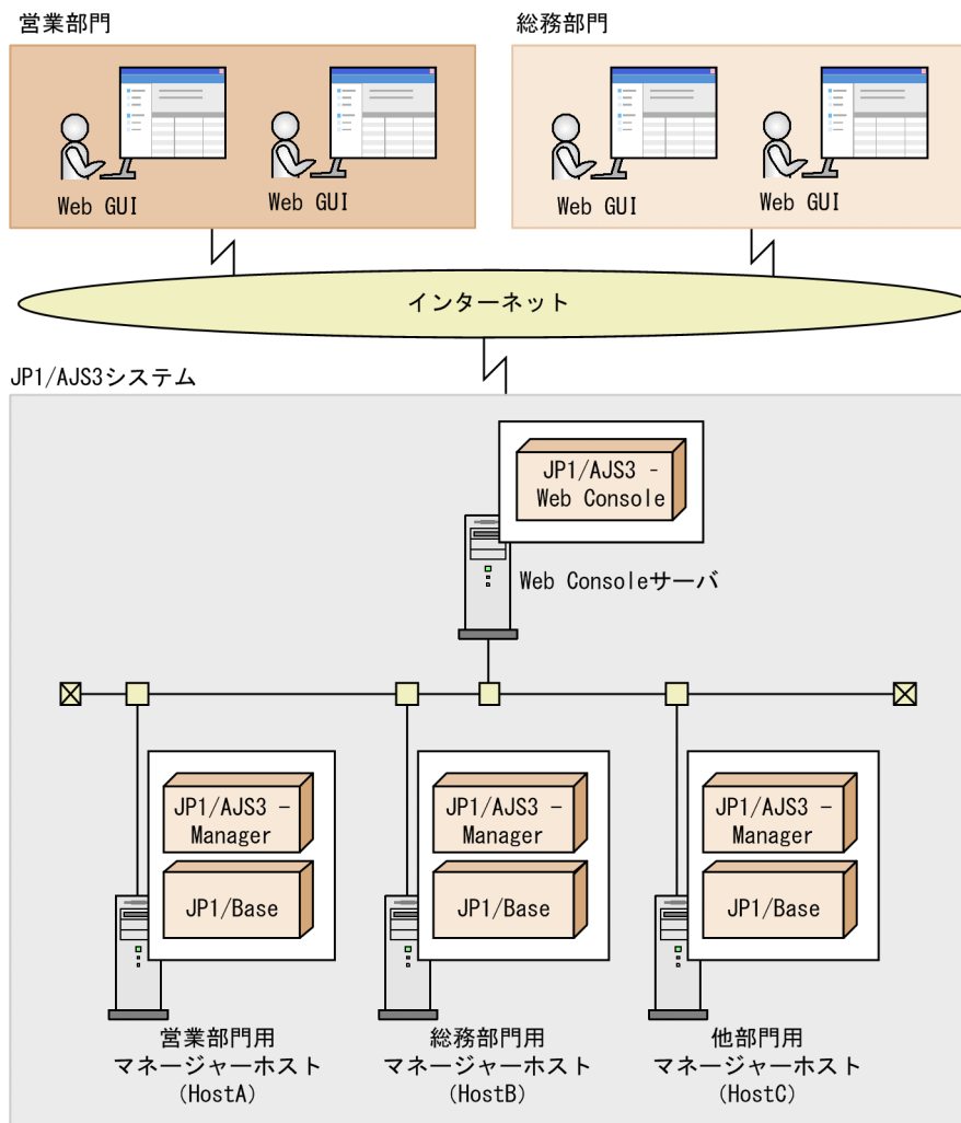
図 13-23 複数のユーザーが Web GUI (ジョブポータル) を使用して運用を監視している例
