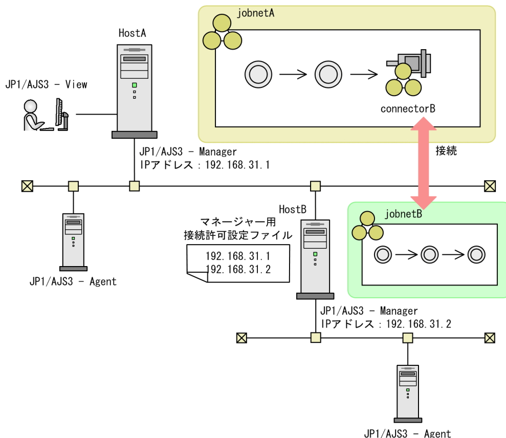
図 2-42 ジョブネットコネクタの例
