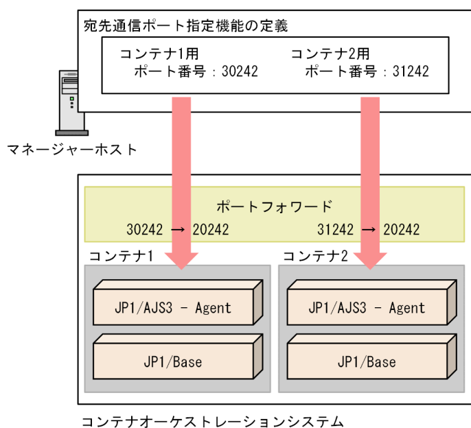
図 2-83 宛先通信ポート指定機能を使用したコンテナごとに異なるポート番号で通信する必要がある環境での接続の概要
