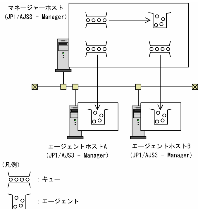
図 7-1 キュー・エージェント構成の例
