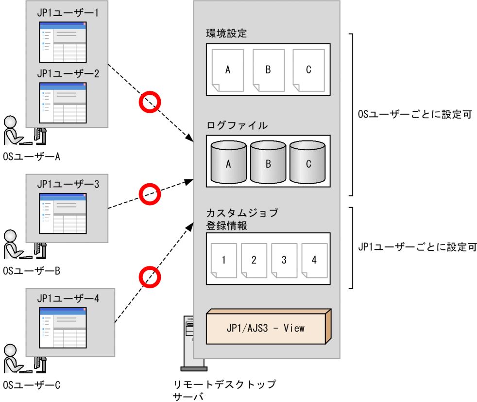
図 4-10 リモートデスクトップ複数接続機能を使用する場合のリモートデスクトップ複数接続の概要
