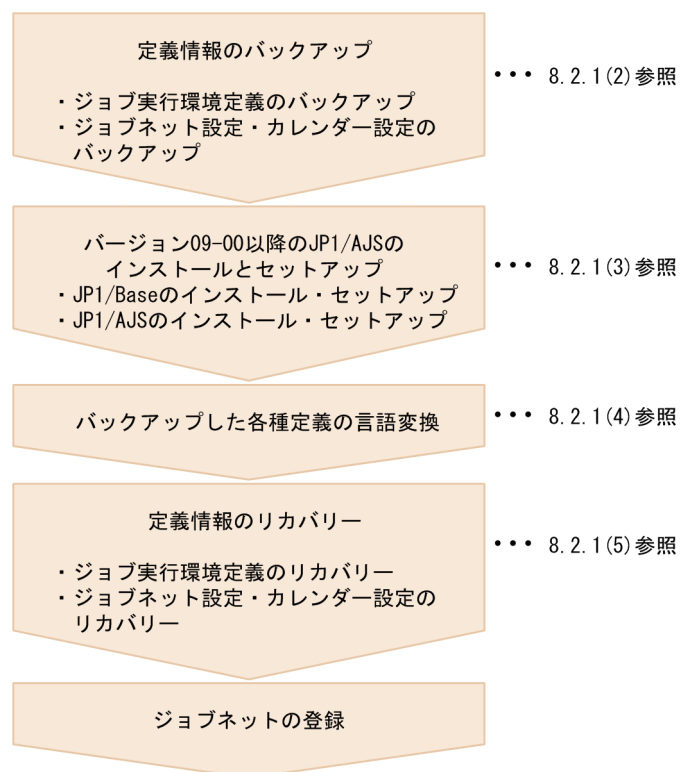
図 8-1 EUC 環境から UTF-8 環境への移行の流れ
