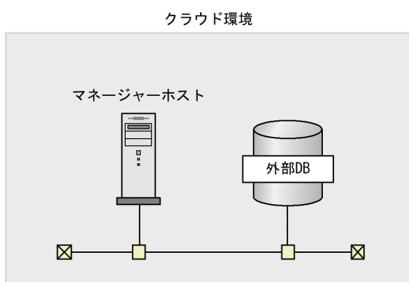
図 2-68 外部 DB を使用する場合のデータベース構成
