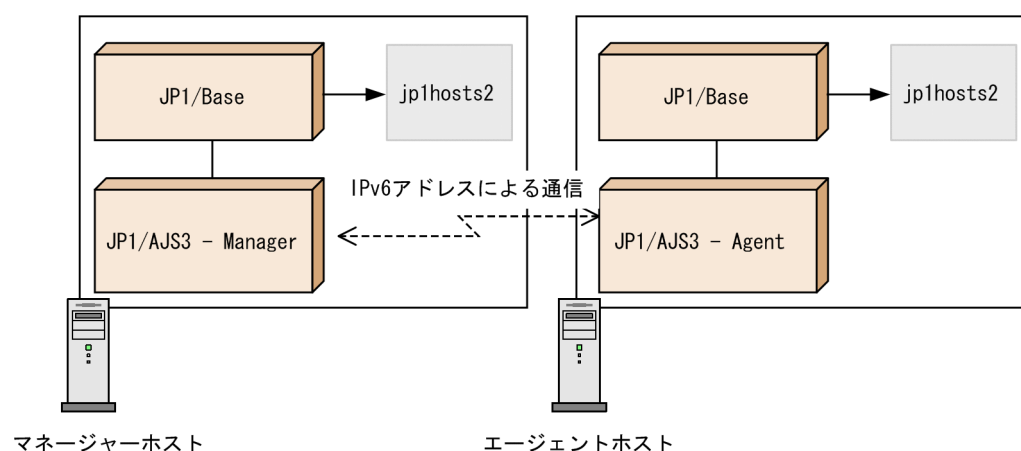
図 2-22 IPv6 アドレスで通信する場合の JP1/Base の通信基盤機能と JP1/AJS3 の関係
