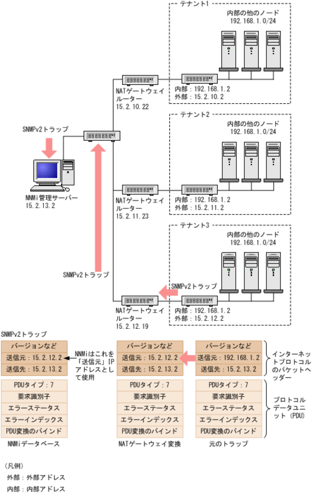
図 13-2 SNMPv2c の例
