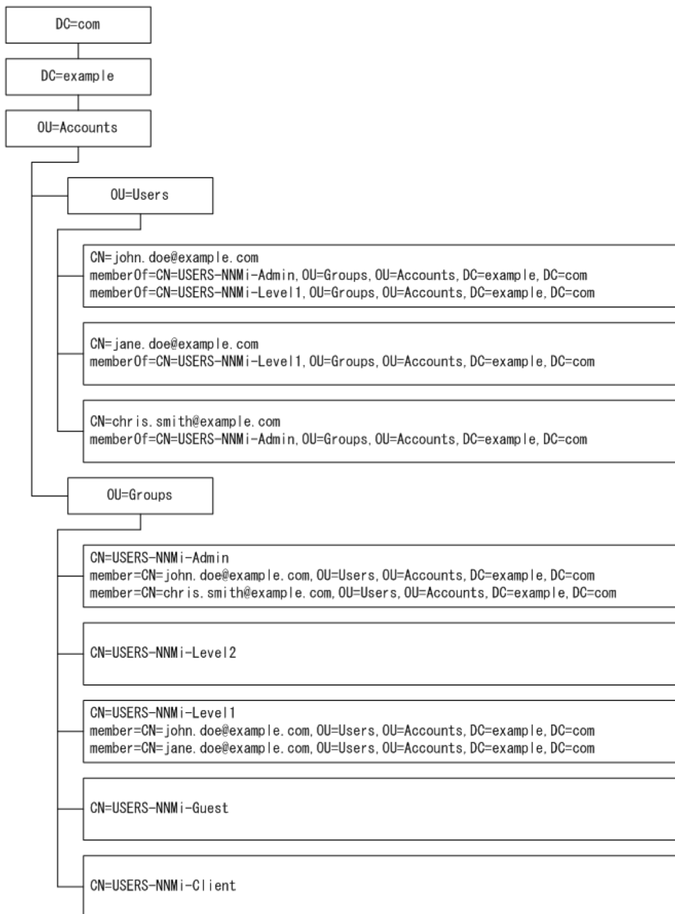
図 12-4 Active Directory のドメイン例
