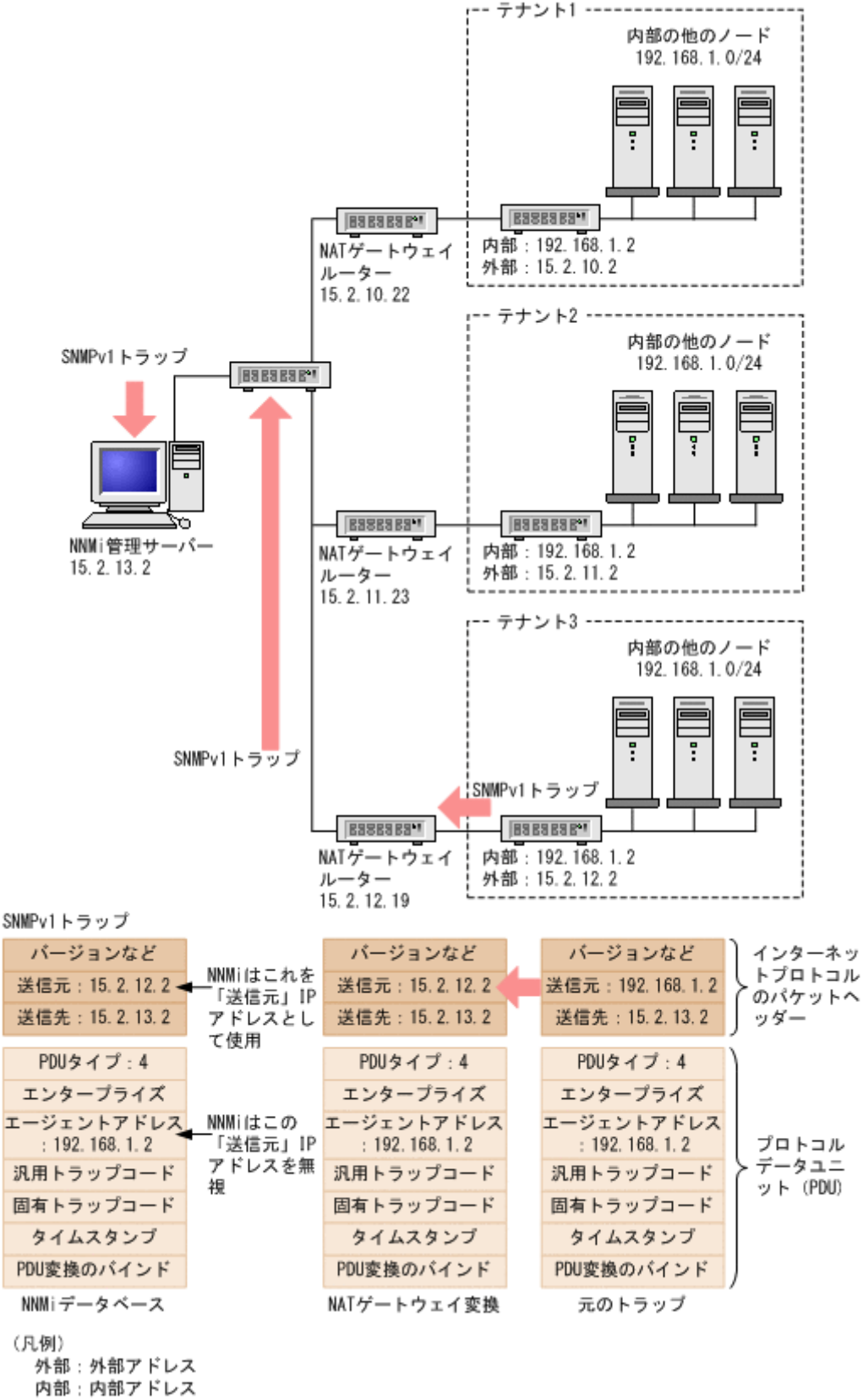
図 13-3 SNMPv1 の例
