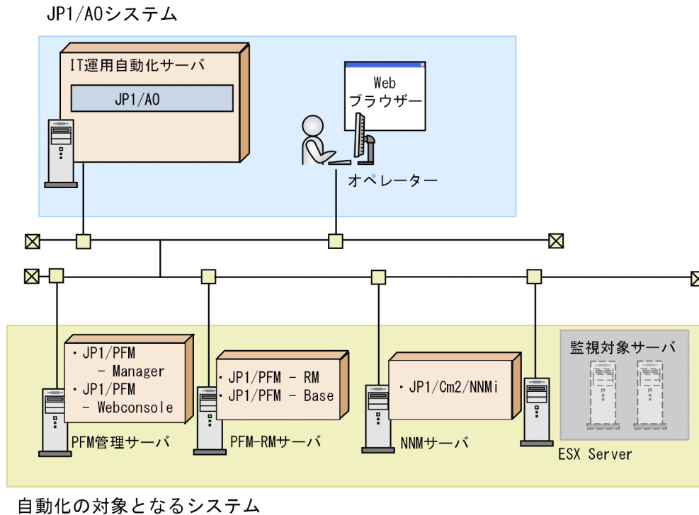
図 1-3 適用例のシステム構成
