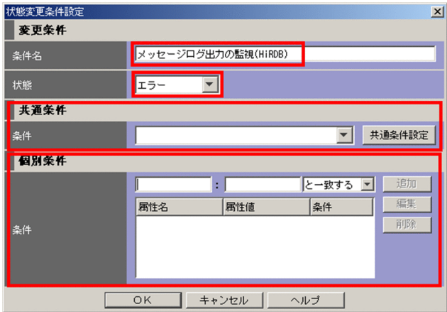
図 6-23 「状態変更条件設定」 画面
