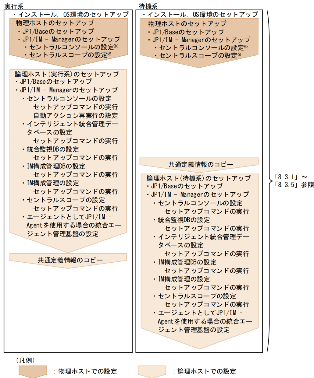
図 8-2 セットアップ作業の流れ（新規に環境設定する場合（JP1/IM - Manager））
