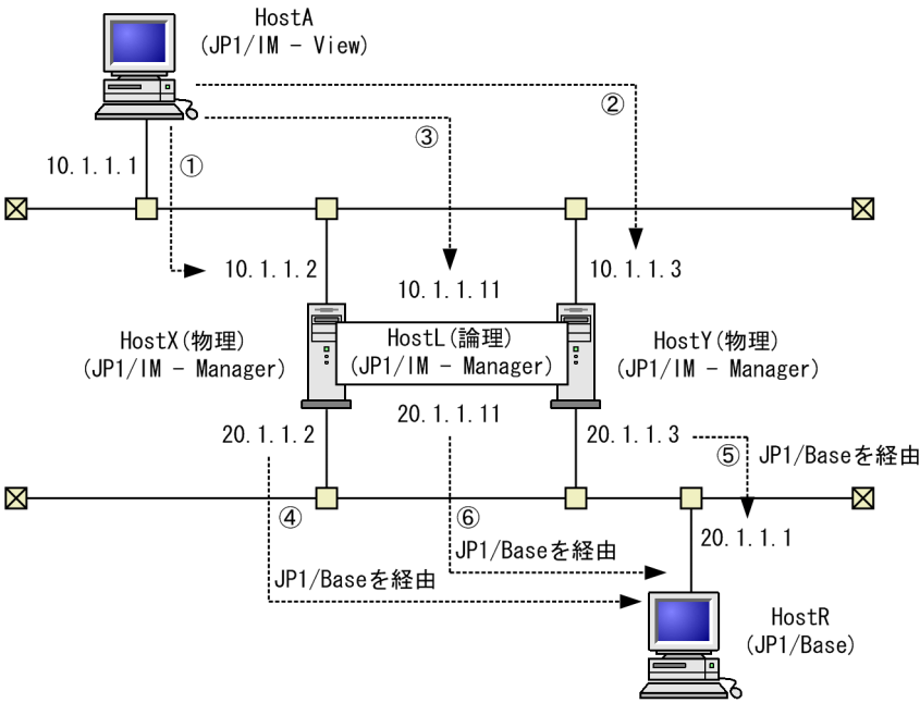
図 9-4 複数 LAN 環境でのコマンド実行 (クラスタ運用)
