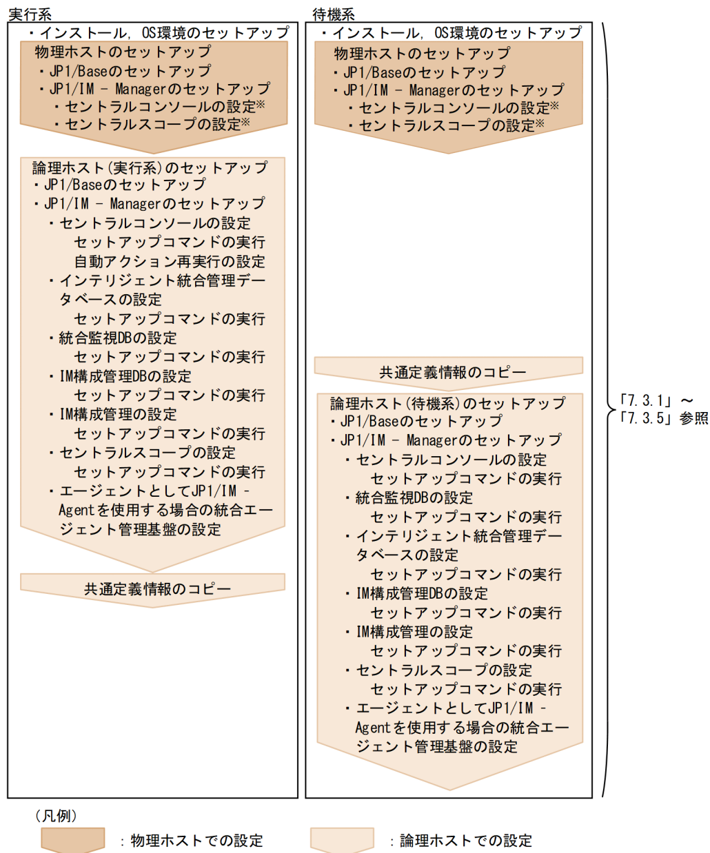
図 7-4 セットアップ作業の流れ（新規に環境設定する場合（JP1/IM - Manager））
