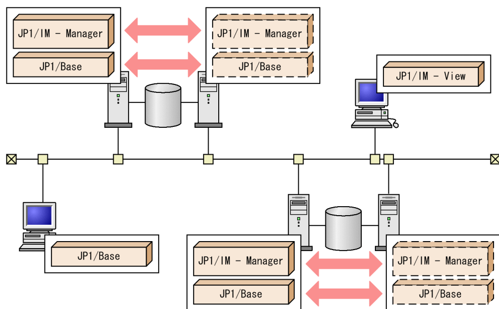
図 7-1 クラスタシステムでの JP1/IM の構成例
