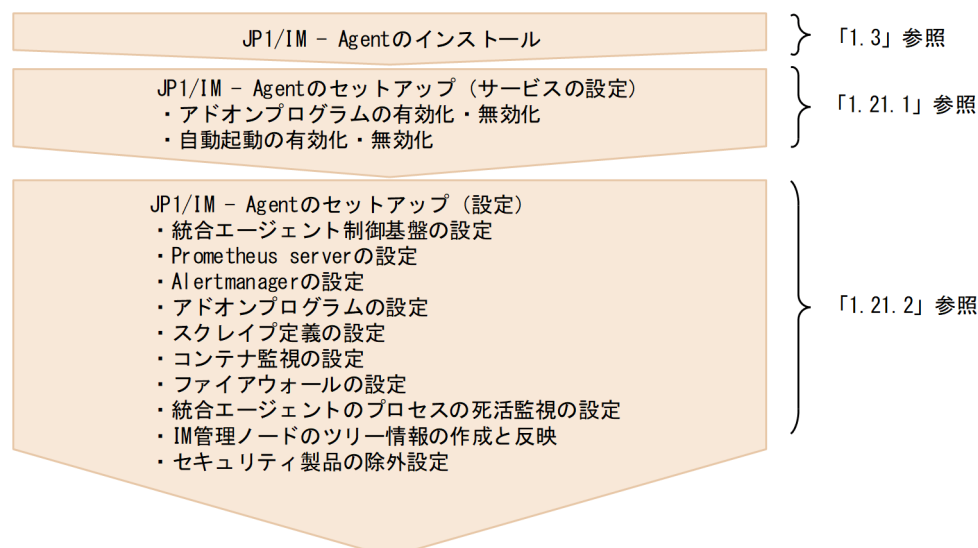
図 1-2 インストールとセットアップの作業の流れ（エージェント（JP1/IM - Agent））
