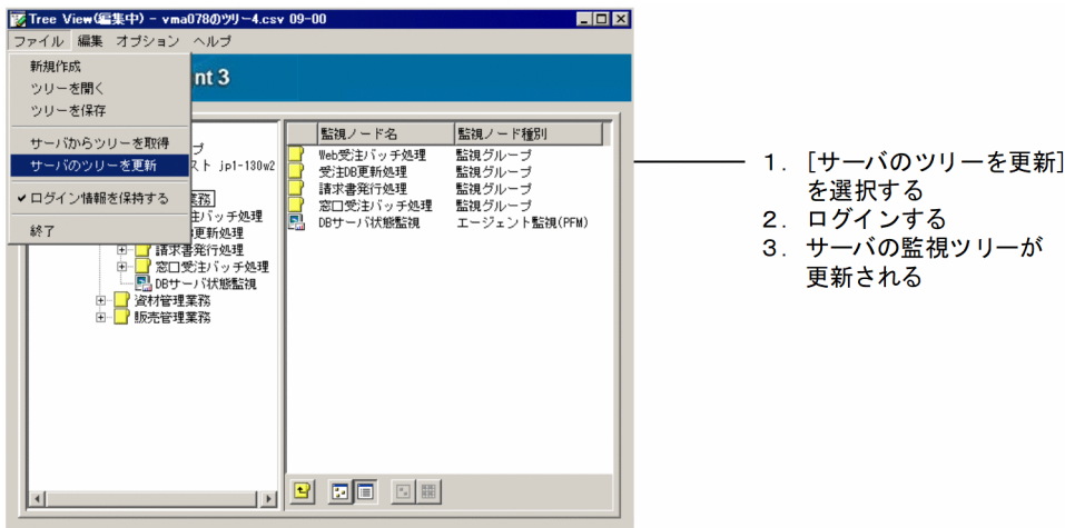
図 6-9 サーバのツリーを更新
