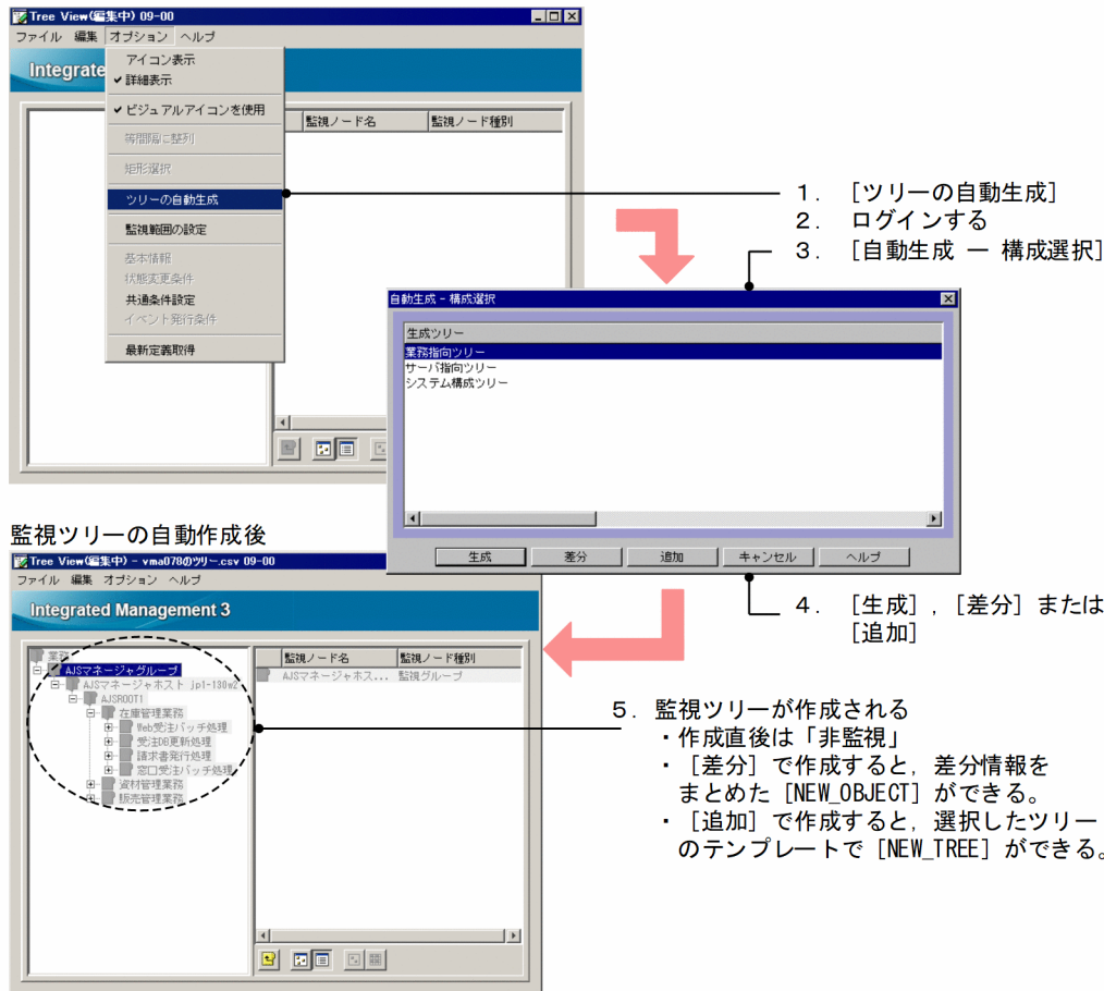
図 6-3 監視ツリーの自動生成の手順
