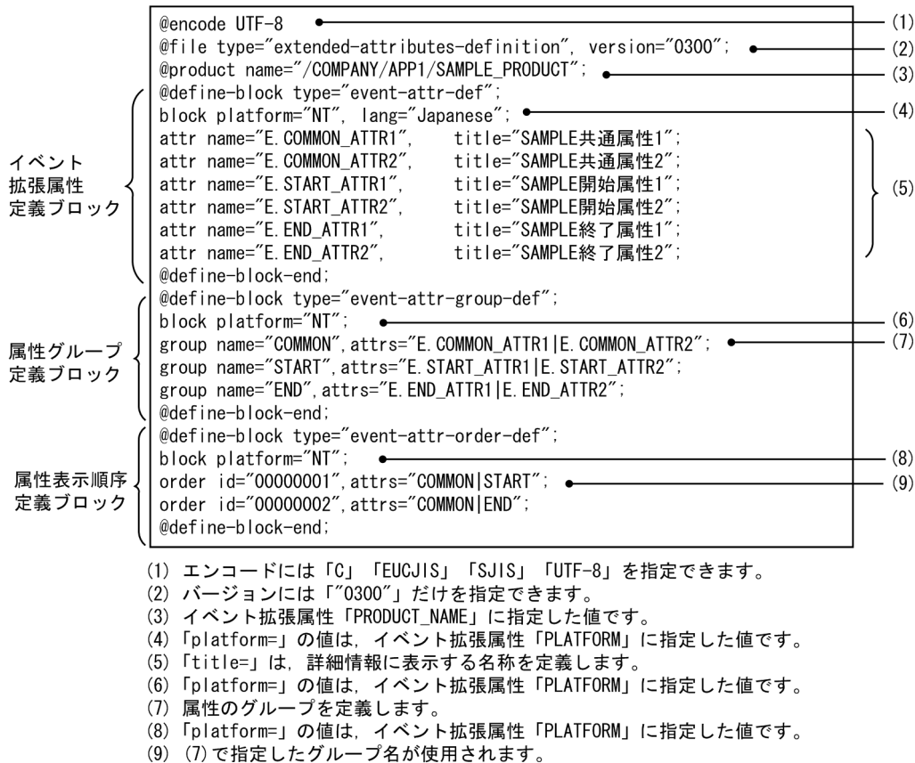
図 5-1 イベント拡張属性定義ファイルの定義例
