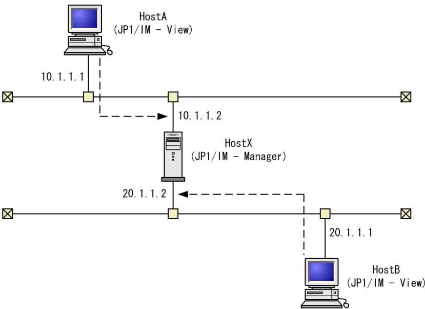
図 9-1 複数 LAN 環境での JP1/IM - View 接続（クラスタ運用なし）
