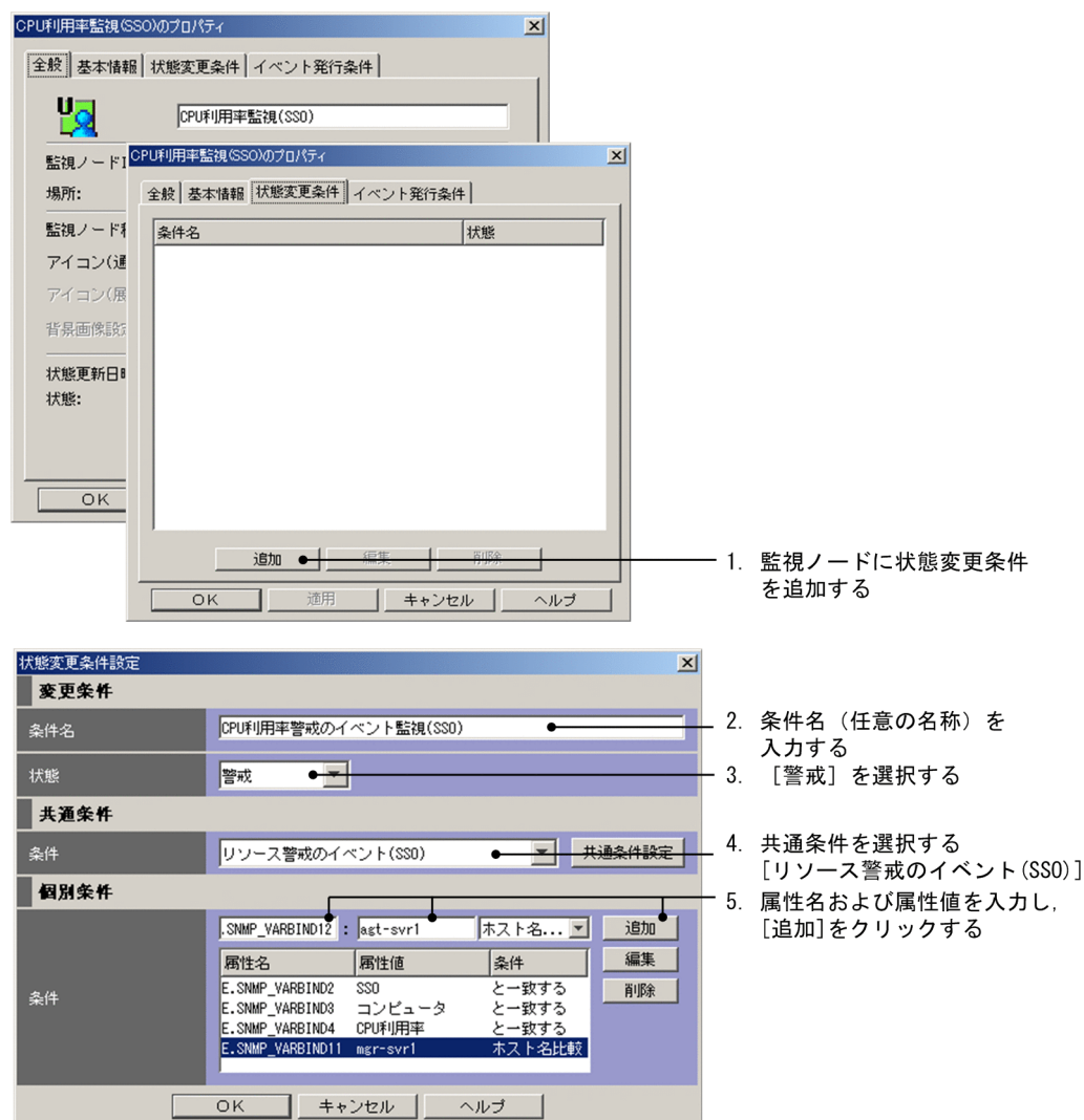
図 6-18 汎用監視オブジェクトの設定 (状態変更条件の追加 その 1)
