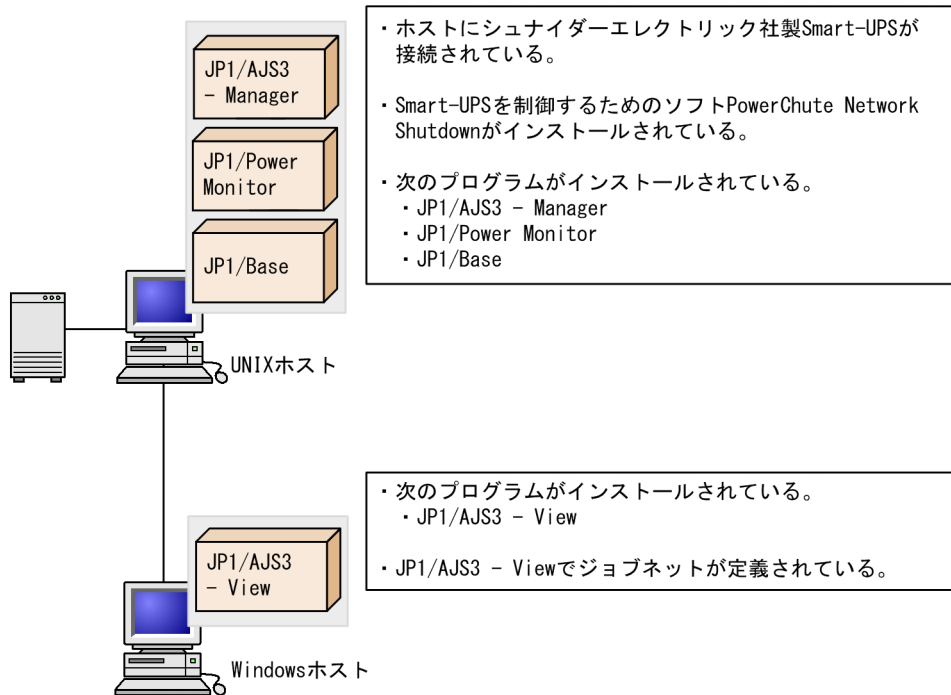
図 2-2 UNIXホストの電源を制御する構成例
