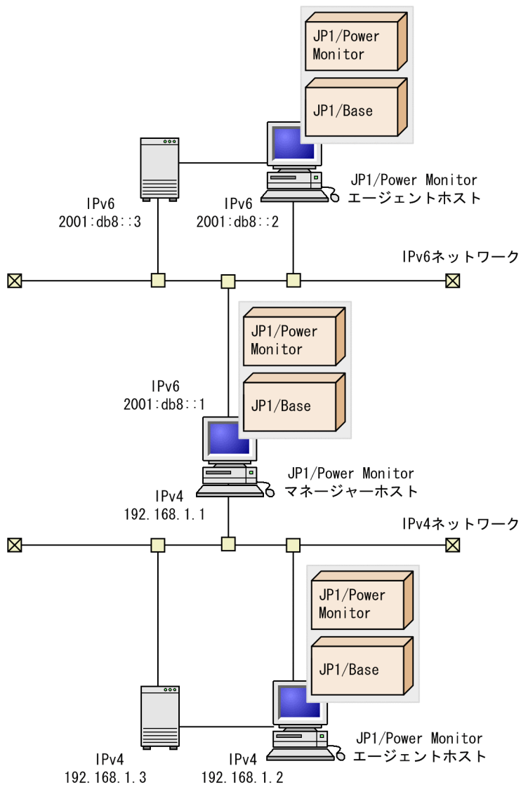
図 4-7 ネットワーク環境が IPv6 を使用する場合のシステム構成例
