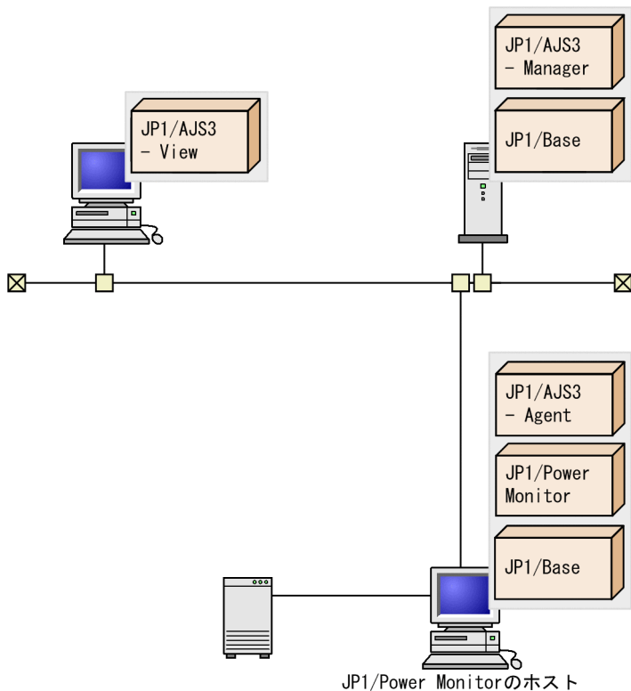
図 4-4 JP1/AJS3 と連携して自ホストを起動・終了する場合のシステム構成例
