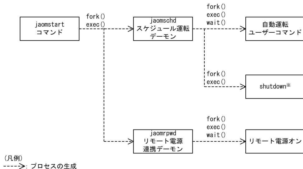
図 B-4 UNIX ホストで JP1/Power Monitor を実行する際のプロセス構成
