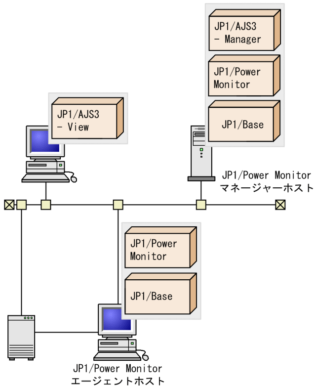
図 4-5 JP1/AJS3 と連携して他ホストを起動・終了する場合のシステム構成例
