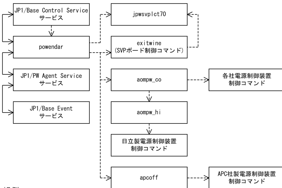
図 B-3 エージェントホストの場合のプロセス構成
