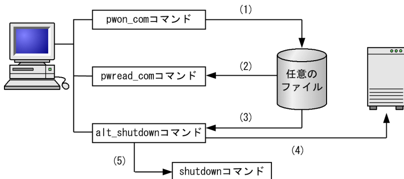
図 6-3 次回電源投入時刻をホスト終了時に設定できる電源制御装置の場合の命令の処理
