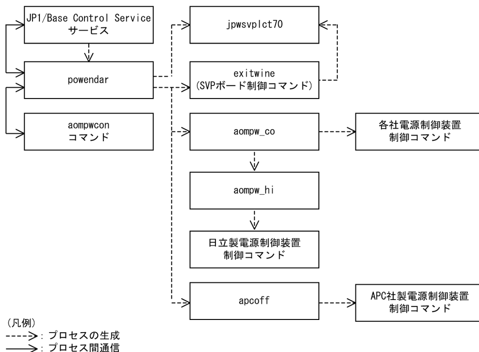
図 B-1 Windows ホストで自ホストを起動・終了する場合のプロセス構成
