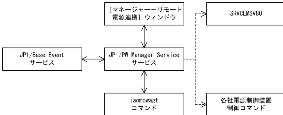
図 B-2 マネージャーホストのプロセス構成
