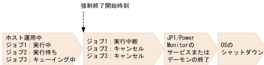
図 1-14 強制終了の流れ
