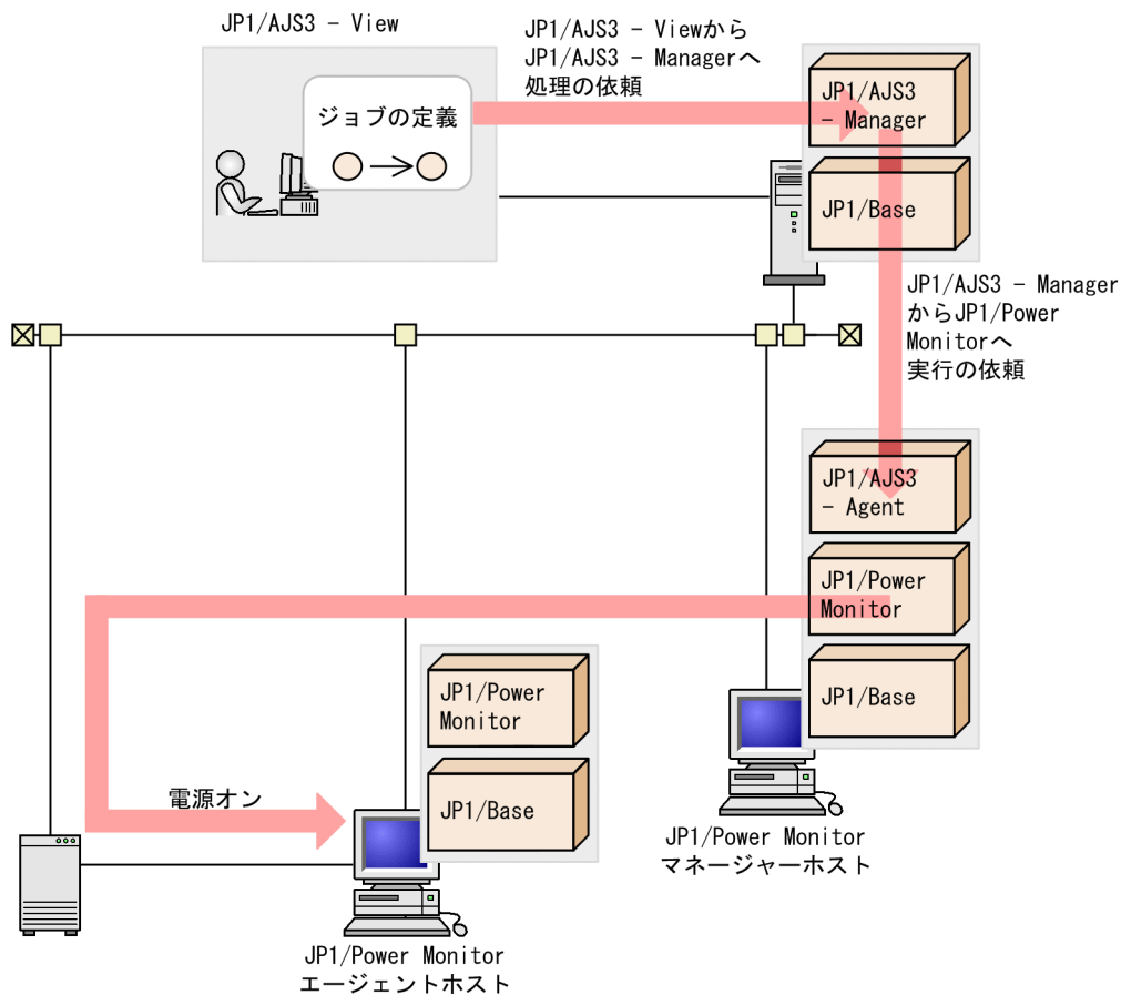
図 1-17 JP1/AJS3 が組み込まれたホストから別のホストを起動する
