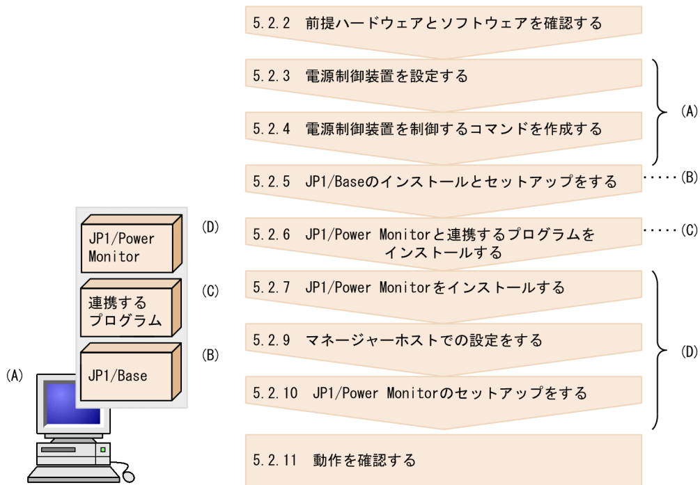
図 5-2 他ホストを制御する場合のマネージャーホストの設定の流れ
