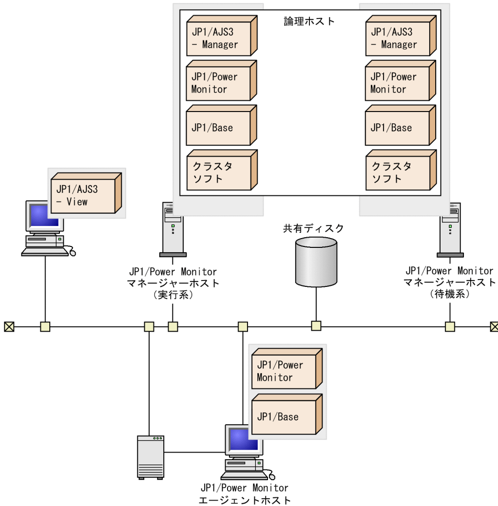
図 4-6 クラスタシステムで運用する場合のシステム構成例
