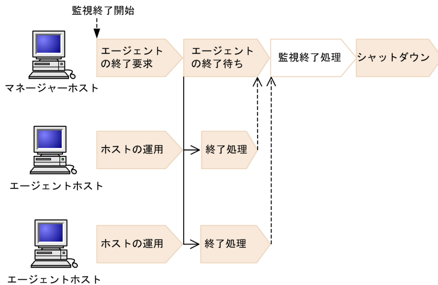
図 1-8 グループ化してホストを終了する流れ (UNIX の場合)
