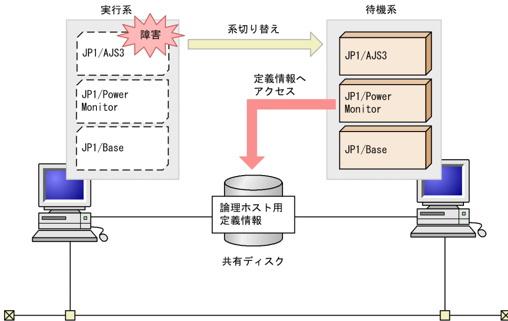
図 1-20 障害発生時の処理の流れ
