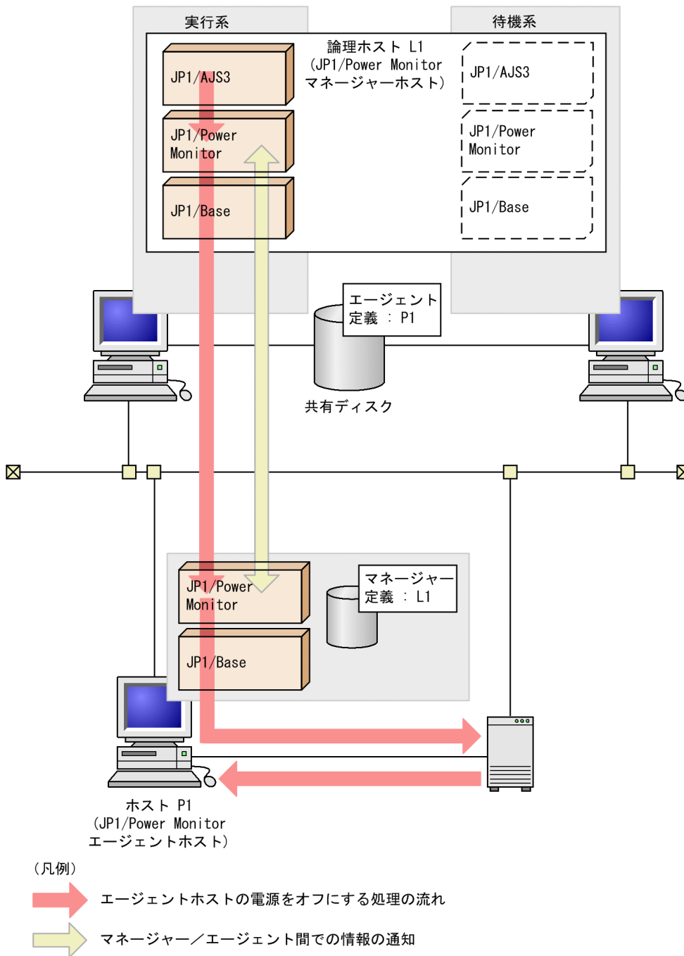
図 1-19 クラスタシステムでの処理の流れ
