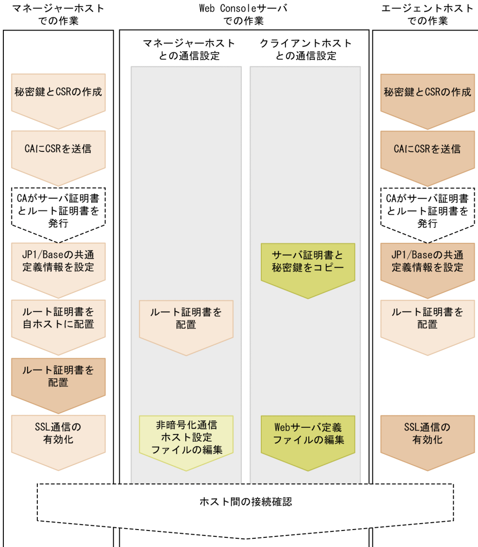
図 21-6 マネージャーホストのサーバ証明書を Web Console サーバで使用する場合の SSL 通信の設定作業の流れ
