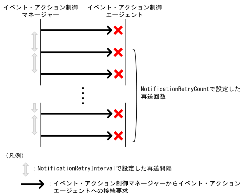
図 15-5 接続タイムアウト以外のエラーが発生した場合
