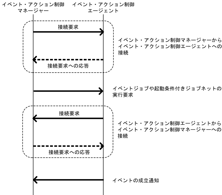
図 6-2 イベントジョブや起動条件付きジョブネットを実行するときの通信の様子
