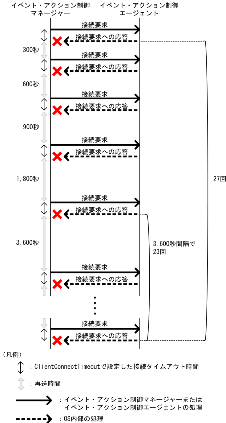
図 15-4 接続タイムアウトが発生した場合のイベント・アクション制御マネージャーとイベント・アクション制御エージェント間での通信の様子
