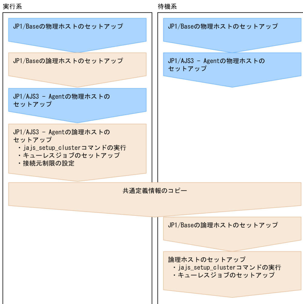
図 17-5 クラスタシステム的环境設定の手順 (JP1/AJS3 - Agent)
