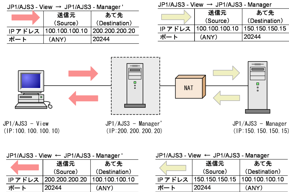
図 2-16 JP1/AJS3 の NAT の設定例
