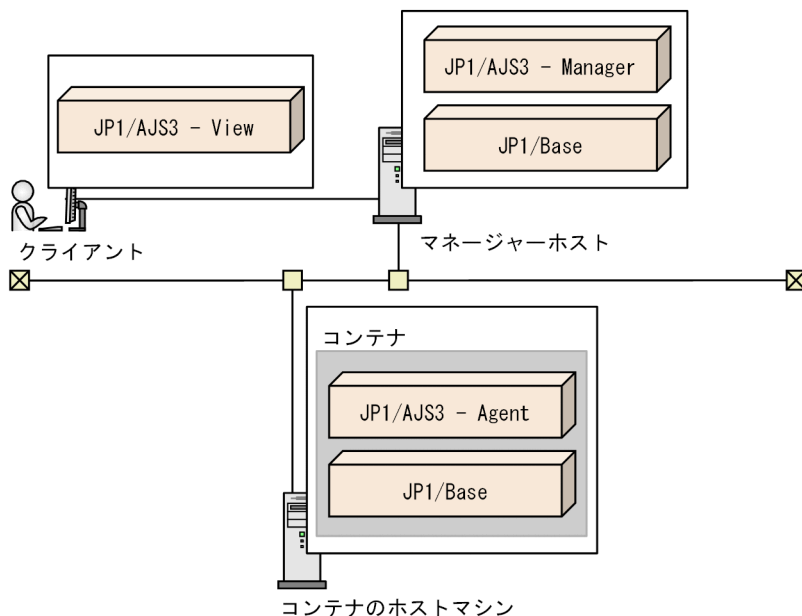
図 2-80 コンテナ環境における JP1/AJS3 のシステム構成 3 (マネージャーホストを用意し、コンテナのホストマシンのコンテナ内に JP1/AJS3 - Agent をインストールする場合)
