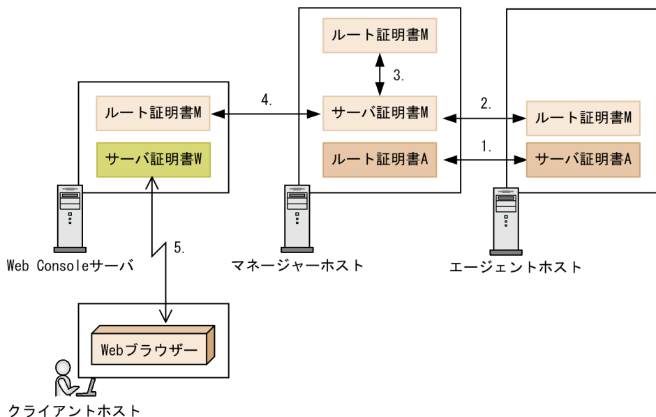
図 2-30 Web Console サーバとマネージャーホストを異なるホストに導入する場合のサーバ証明書とルート証明書の配置
