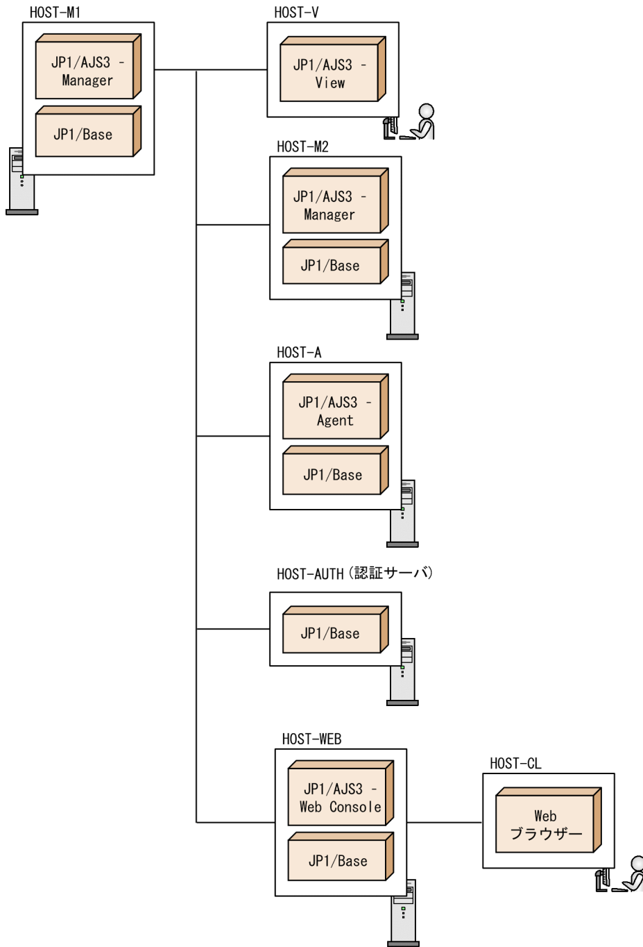
図 2-19 システム構成例
