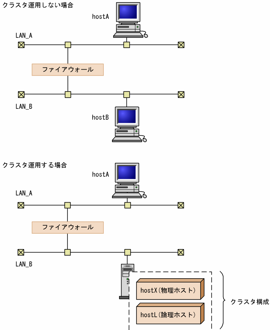
図 2-18 ファイアウォールを設定したシステム構成例
