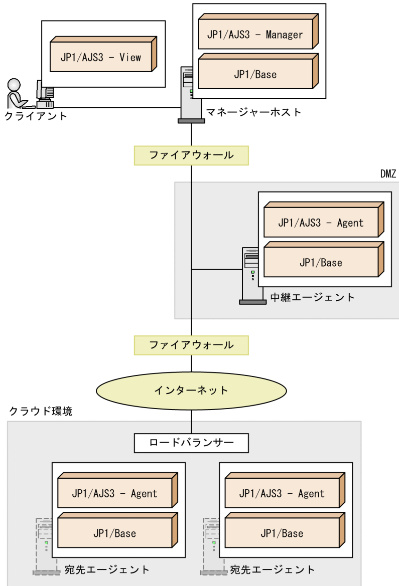
図 2-63 ロードバランサーおよび中継エージェントを使用したシステム構成例
