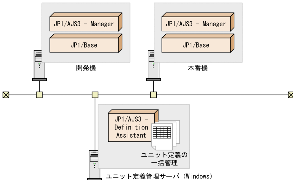
図 C-1 推奨する機器構成
