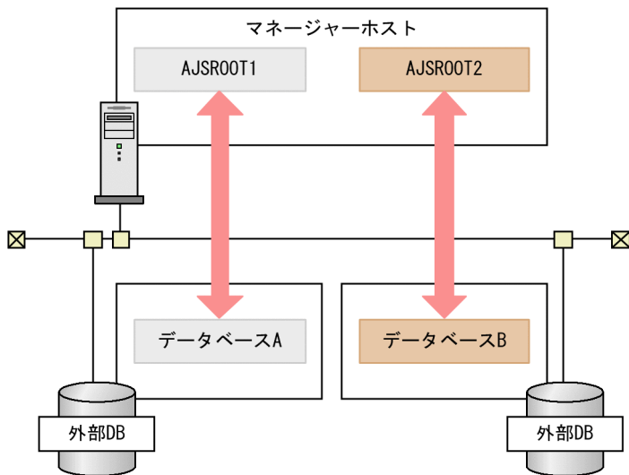
図 2-72 一つのマネージャーホストで、異なる外部 DB のインスタンスを利用する構成
