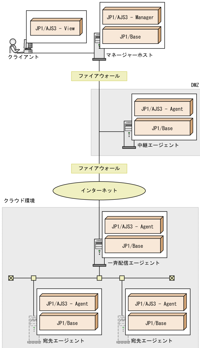
図 2-66 一斉配信エージェントを使用したシステム構成例
