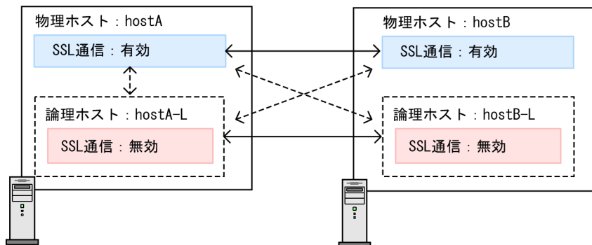
図 2-33 マネージャーホストまたは認証サーバを論理ホストとして導入する場合の例
