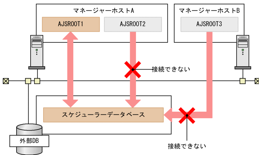
図 2-74 外部 DB のスケジューラーデータベースとスケジューラーサービスの接続関係
