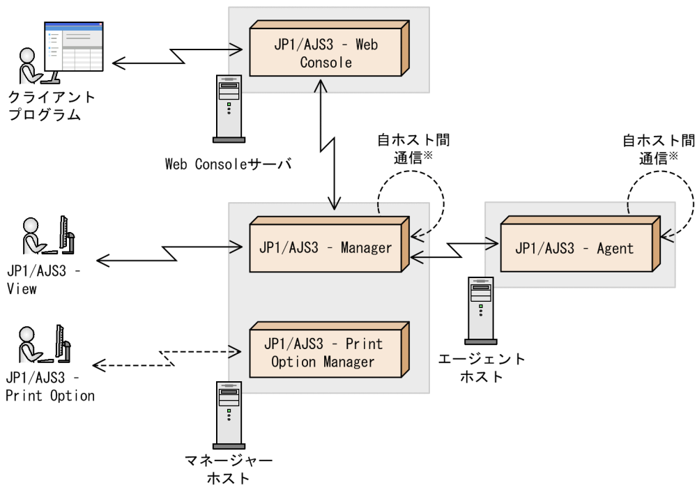
図 2-27 通信暗号化機能の対象となる通信
