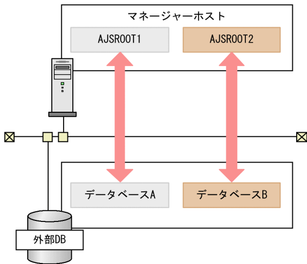
図 2-71 一つのマネージャーホストで、一つの外部 DB のインスタンスを利用する構成
