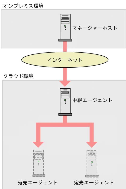
図 2-62 オンプレミス環境とクラウド環境を併用する例 2
