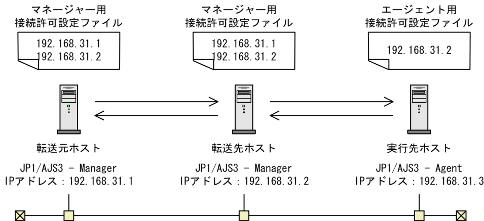
図 2-40 リモートジョブネットを実行する場合の設定例
