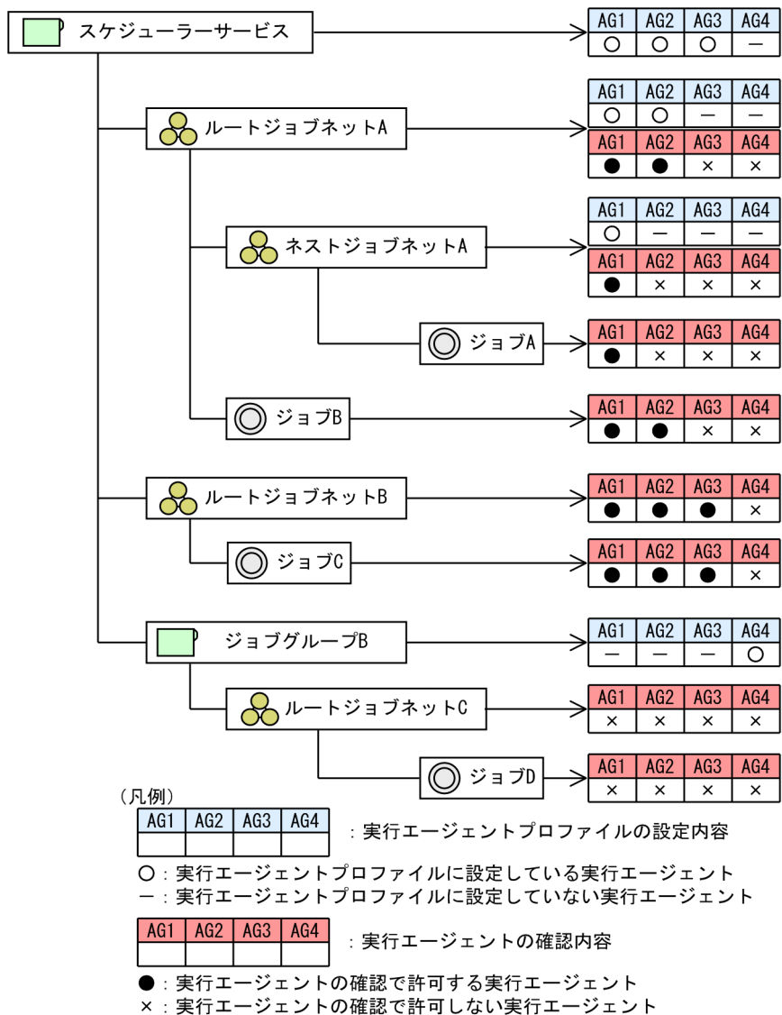
図 2-48 実行エージェントプロファイルの設定と許可する実行エージェント
