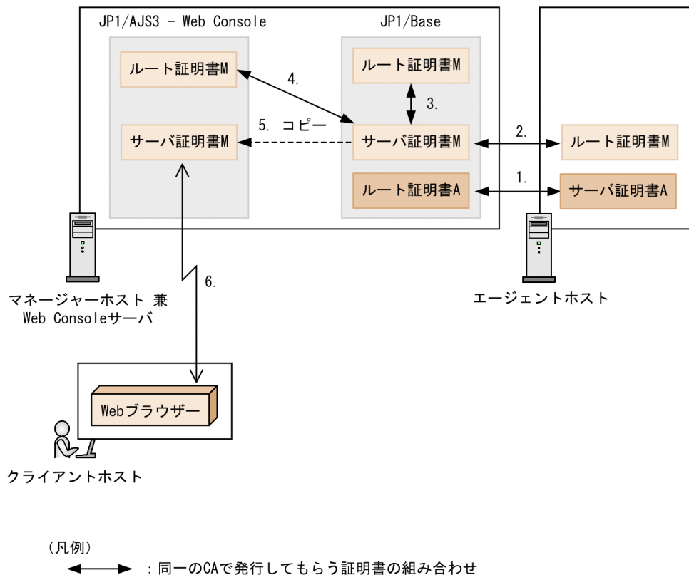
図 2-31 Web Console サーバとマネージャーホストを同一のホストに導入する場合 (JP1/Base を利用)
