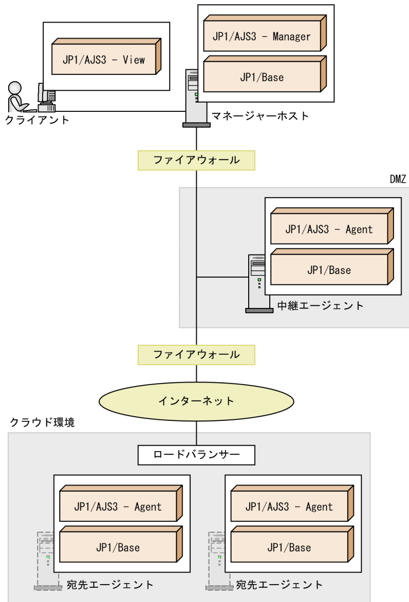
図 2-58 ロードバランサーおよび中継エージェントを使用したシステム構成例
