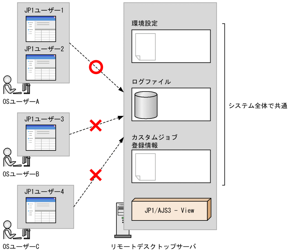
図 4-8 リモートデスクトップ複数接続機能を使用しない場合のリモートデスクトップ複数接続の概要
