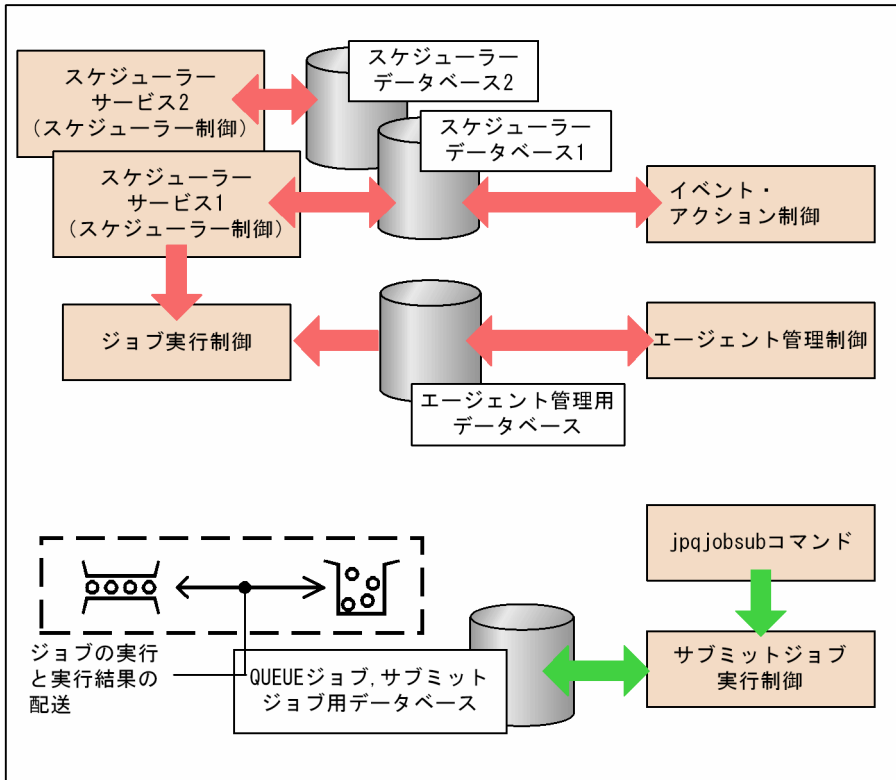
図 2-52 JP1/AJS3 のデータベース構成
