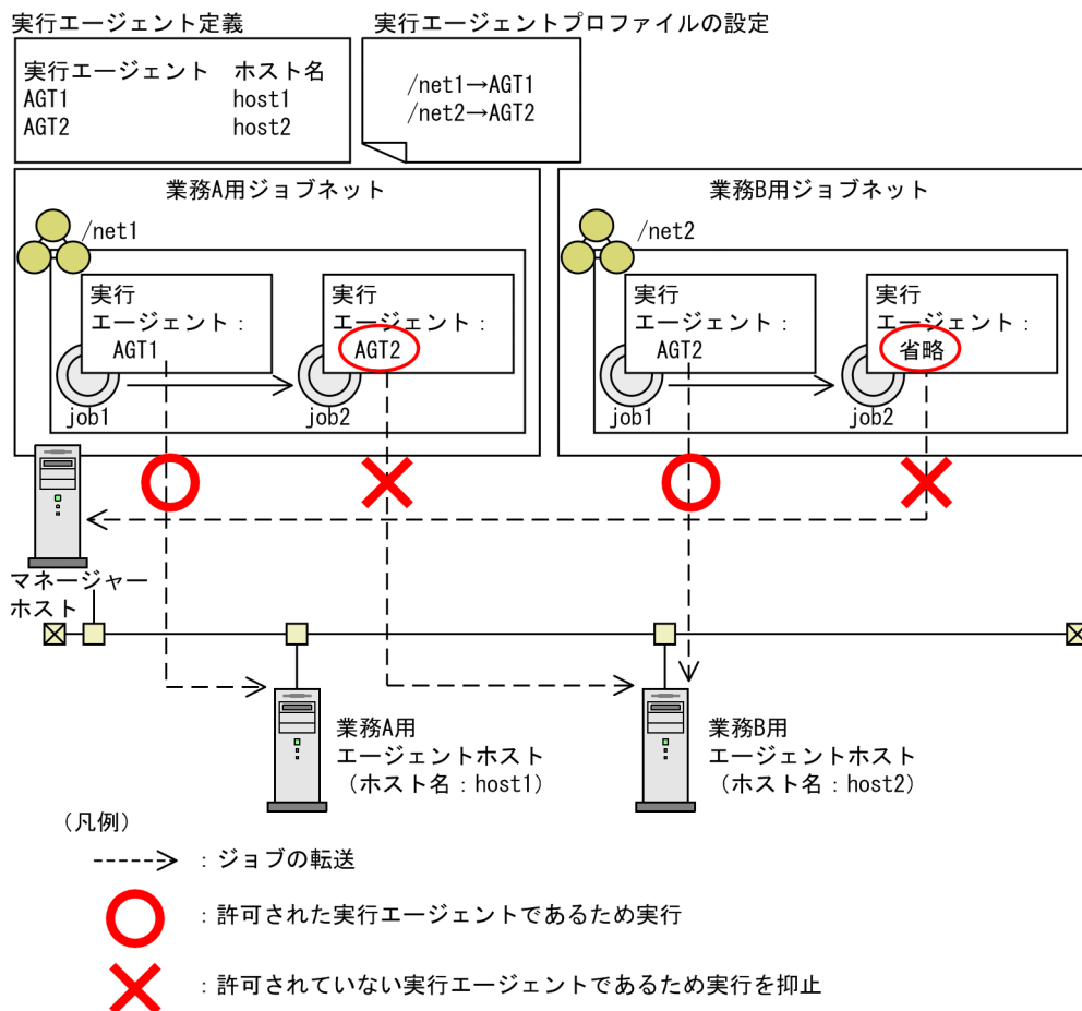
図 2-47 実行エージェント制限の使用例
