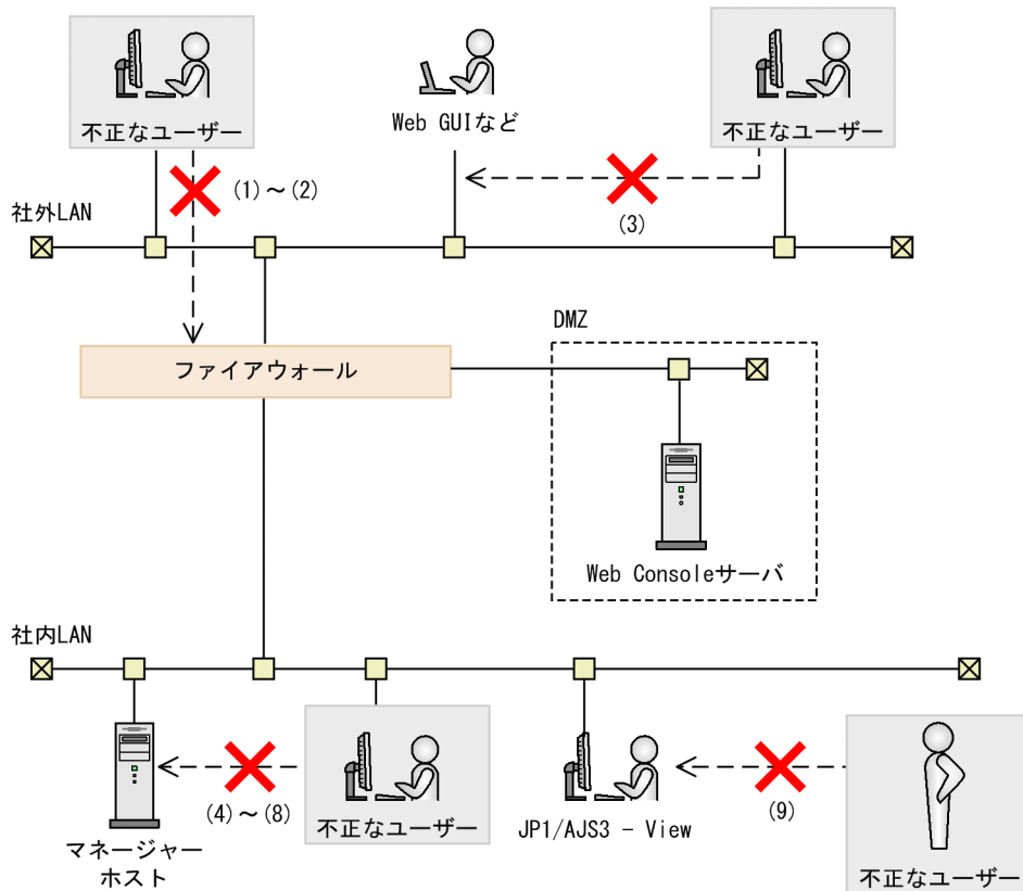
図 2-53 不正なユーザーからのアクセスへの対策
