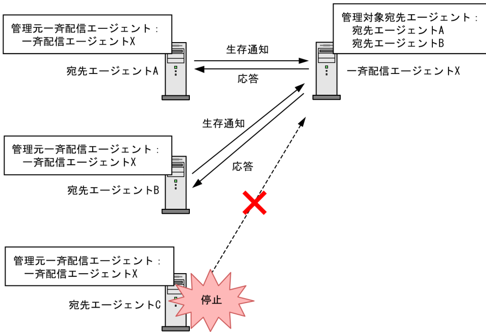
図 2-60 一斉配信エージェントが宛先エージェントを管理している例
