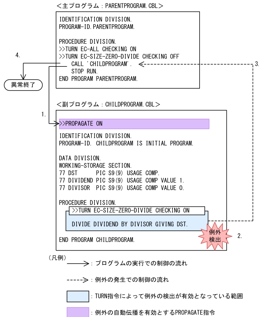
図 21-5 プログラム「CHILDPGRAM」から致命的な例外の伝播を実行するが、プログラム「PARENTPROGRAM」の例外チェックが無効な場合の動作例
