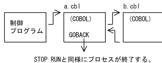
図 16-2 GOBACK 文による終了の例
