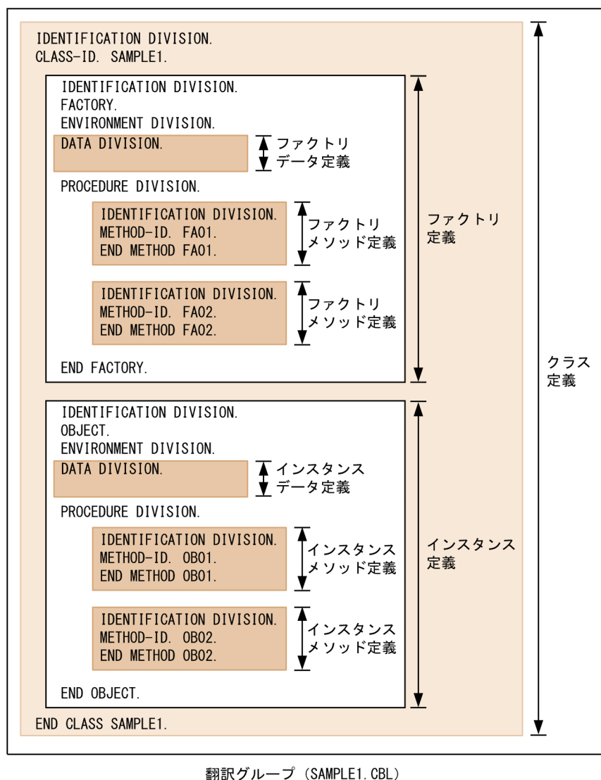
図 3-4 クラス定義
