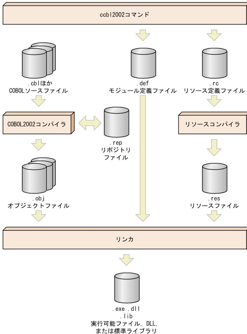
図 33-1 コンパイル時の入出力の流れ
