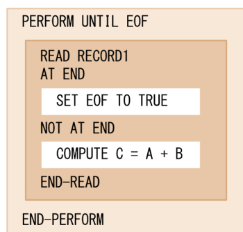
図 21-4 文の範囲
