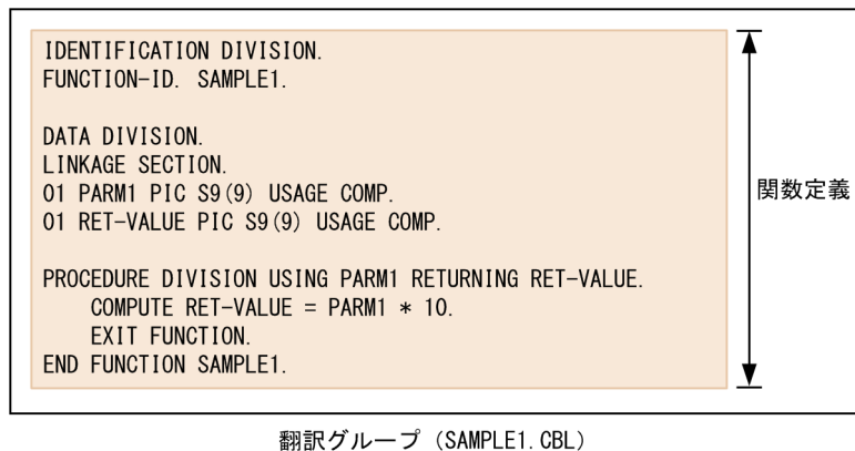
図 3-3 関数定義
