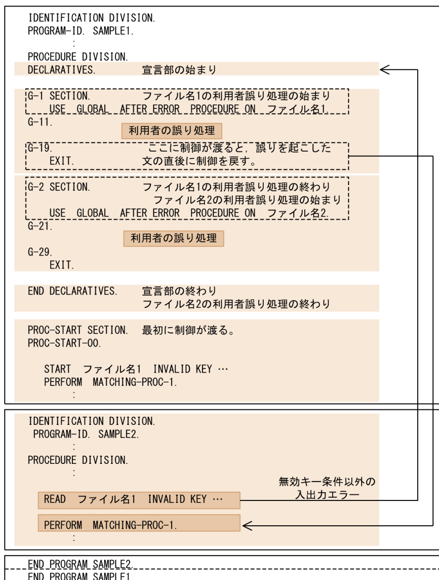
図 6-2 USE GLOBAL ERROR 手続き処理のコーディング例
