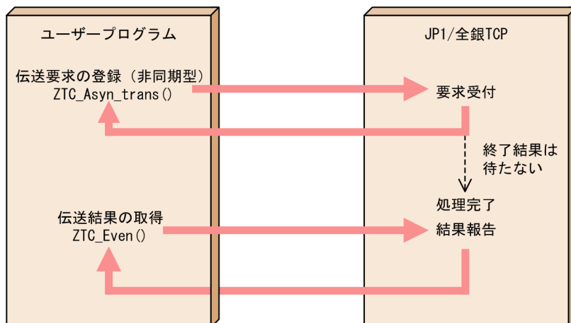
図 9-2 非同期型の伝送要求登録の場合
