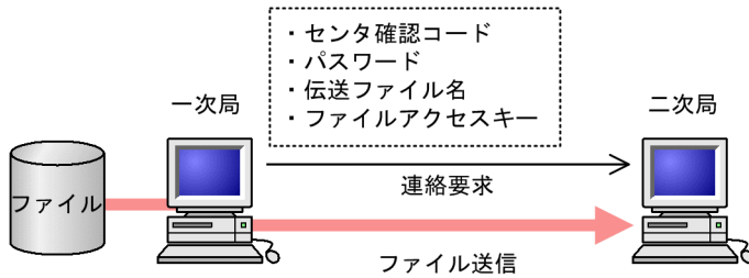
図 1-1 全銀協手順（TCP/IP）によるファイル伝送
