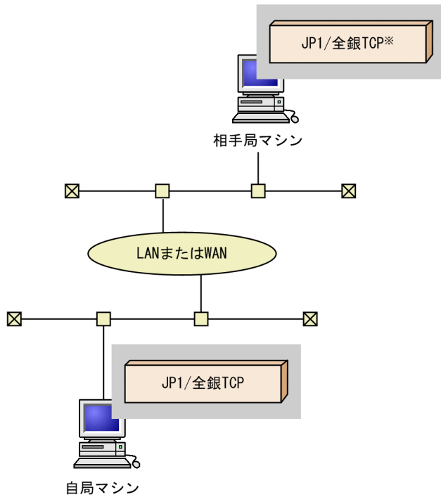
図 2-1 JP1/全銀 TCP のシステム構成
