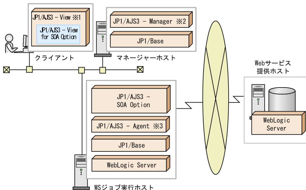
図 3-3 JP1/AJS3 - SOA Option および JP1/AJS3 - View for SOA Option の基本構成例 ( WebLogic Server を使用する場合 )
