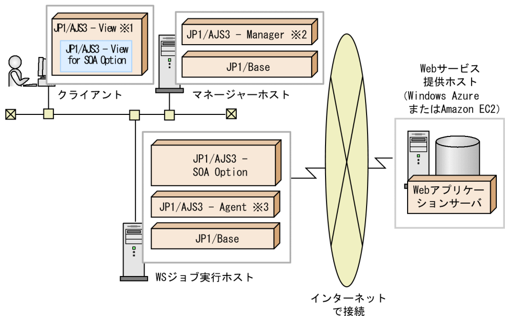
図 3-4 JP1/AJS3 - SOA Option および JP1/AJS3 - View for SOA Option の基本構成例 (クラウド上に Web サービス提供ホストを配置する場合 )
