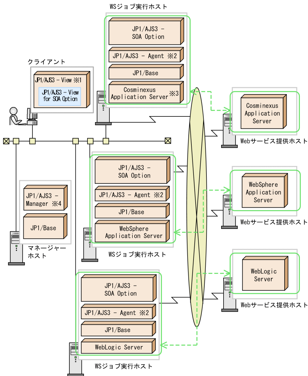
図 3-9 JP1/AJS3 - SOA Option および JP1/AJS3 - View for SOA Option のシステムの最大構成例
