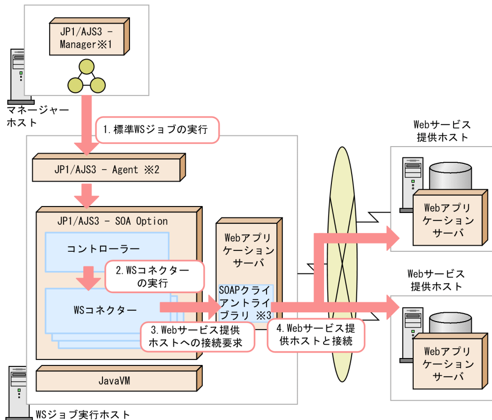
図 2-7 標準 WS ジョブが実行される仕組み
