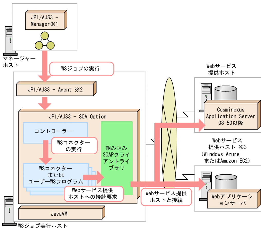
図 2-9 WS ジョブが実行される仕組み (組み込み SOAP クライアントライブラリを使用した場合)
