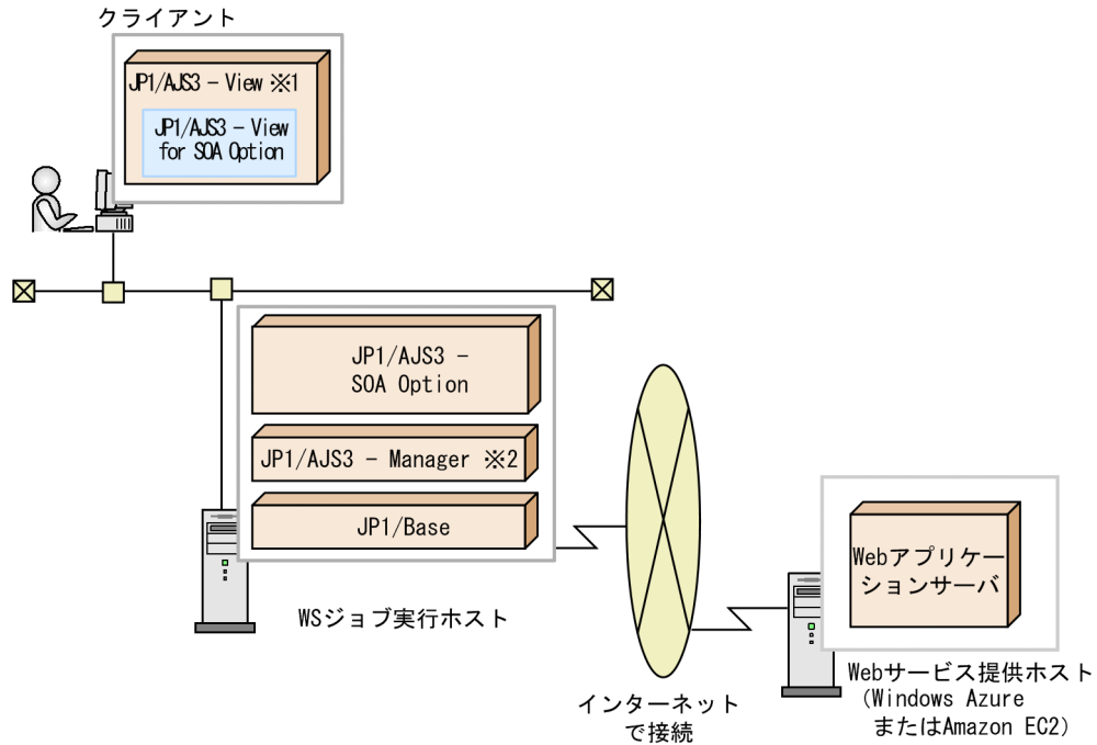
図 3-8 WS ジョブを JP1/AJS3 - Manager または JP1/AJS2 - Manager で実行する場合のシステム構成例 (クラウド上に Web サービス提供ホストを配置する場合)
