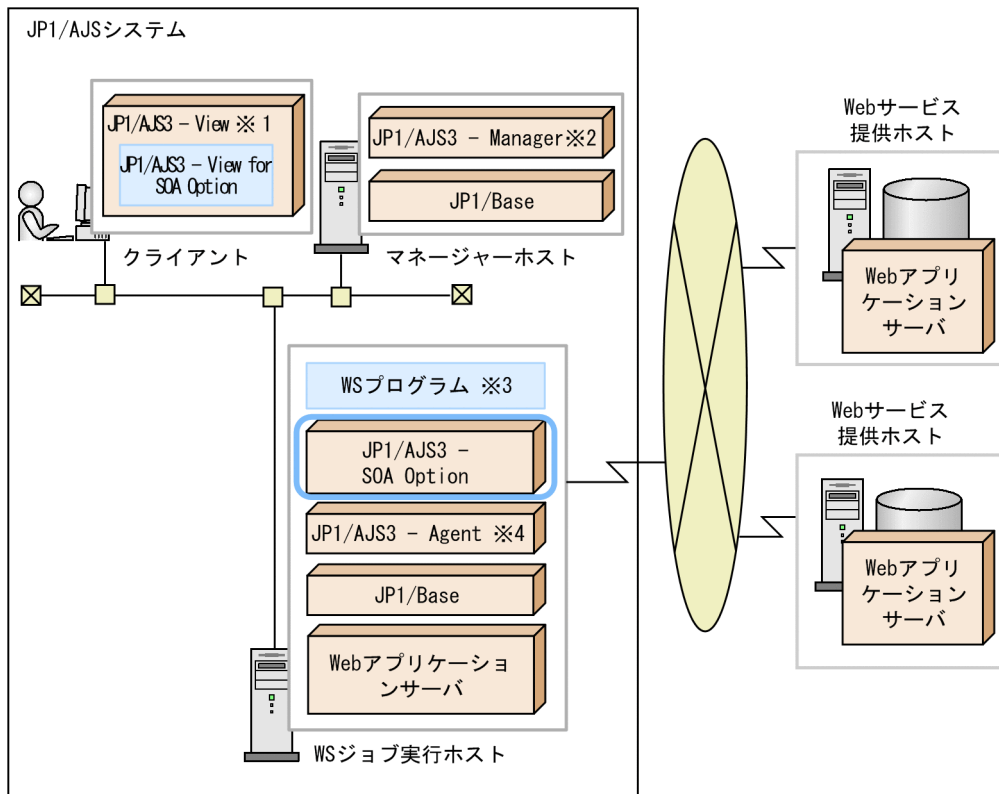
図 2-1 JP1/AJS3 - SOA Option のシステム全体像
