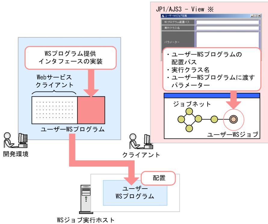
図 2-6 ユーザー WS ジョブを定義するイメージ
