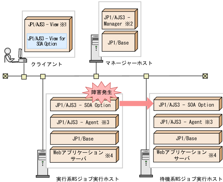
図 6-1 JP1/AJS3 - SOA Option にフェールオーバーが発生した場合の処理
