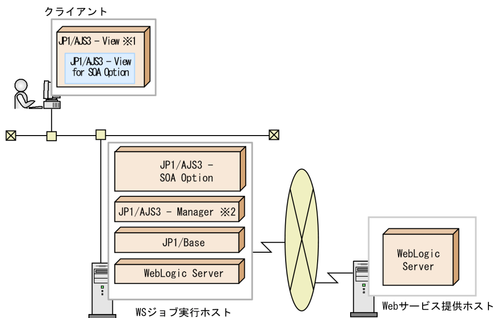
図 3-7 WS ジョブを JP1/AJS3 - Manager または JP1/AJS2 - Manager で実行する場合のシステム構成例 ( WebLogic Server を使用する場合 )
