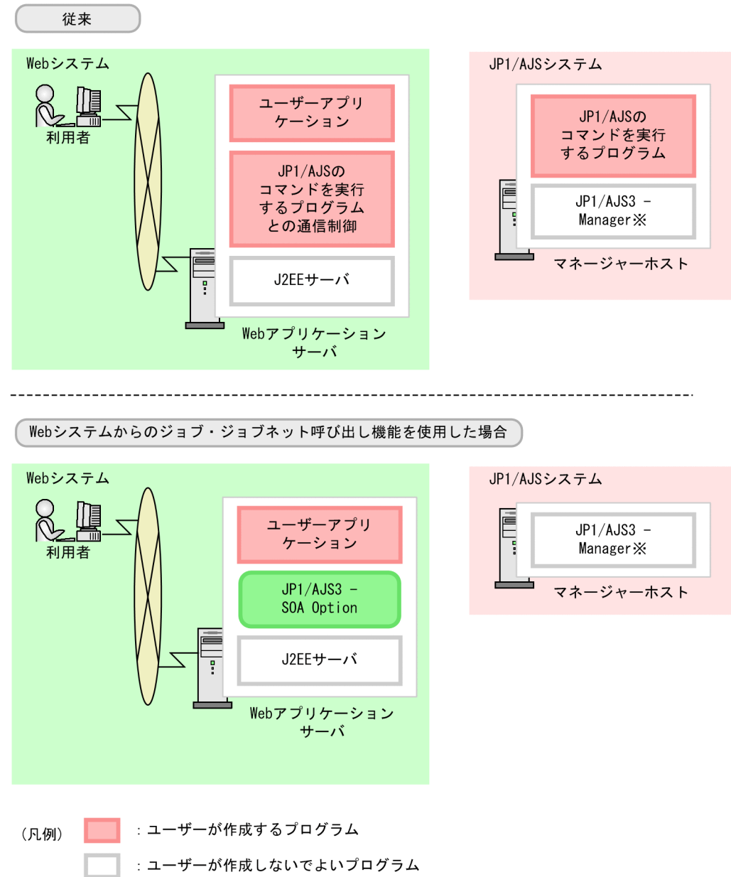
図 1-4 従来と Web システムからのジョブ・ジョブネット呼び出し機能を使用した場合との違い
