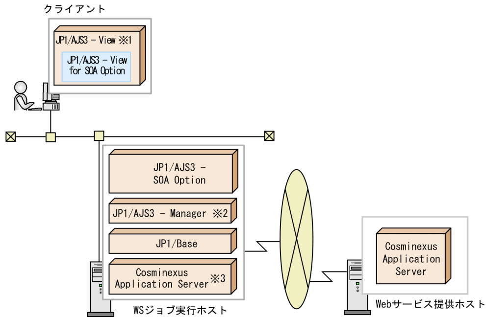
図 3-5 WS ジョブを JP1/AJS3 - Manager または JP1/AJS2 - Manager で実行する場合のシステム構成例 (Cosminexus Application Server を使用する場合)
