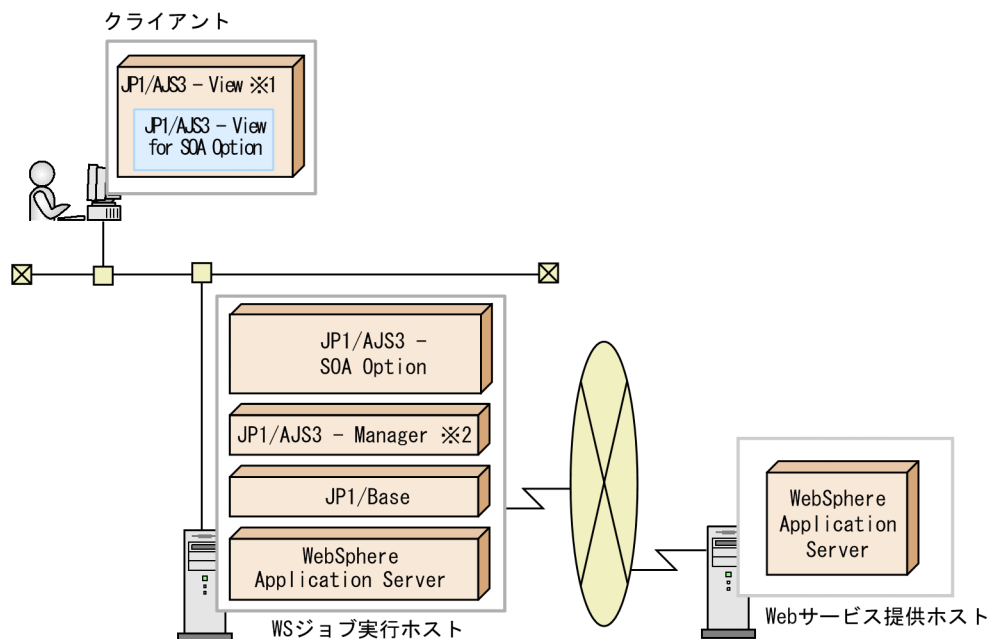
図 3-6 WS ジョブを JP1/AJS3 - Manager または JP1/AJS2 - Manager で実行する場合のシステム構成例 ( WebSphere Application Server を使用する場合 )
