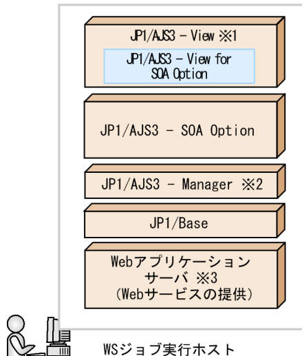
図 3-10 JP1/AJS3 - SOA Option および JP1/AJS3 - View for SOA Option のシステムの最小構成
