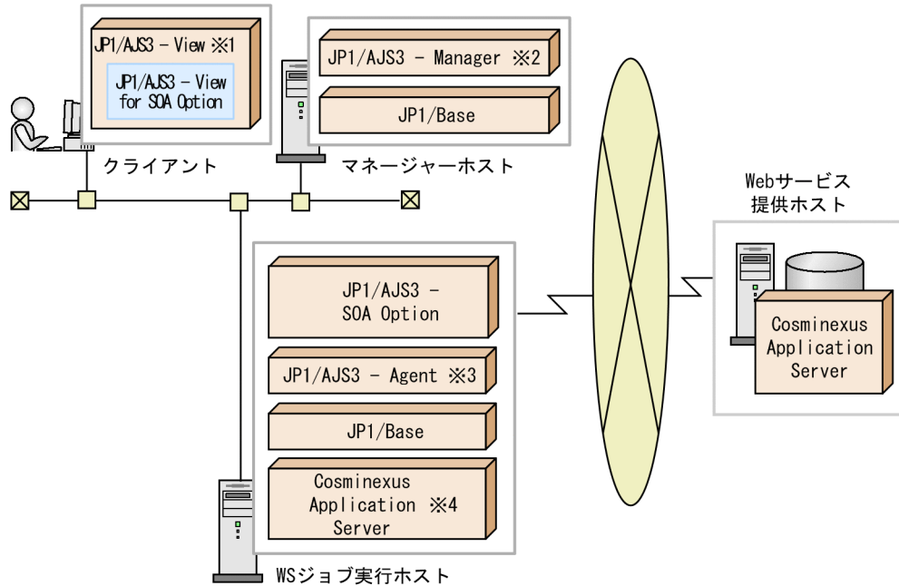
図 3-1 JP1/AJS3 - SOA Option および JP1/AJS3 - View for SOA Option の基本構成例 (Cosminexus Application Server を使用する場合)
