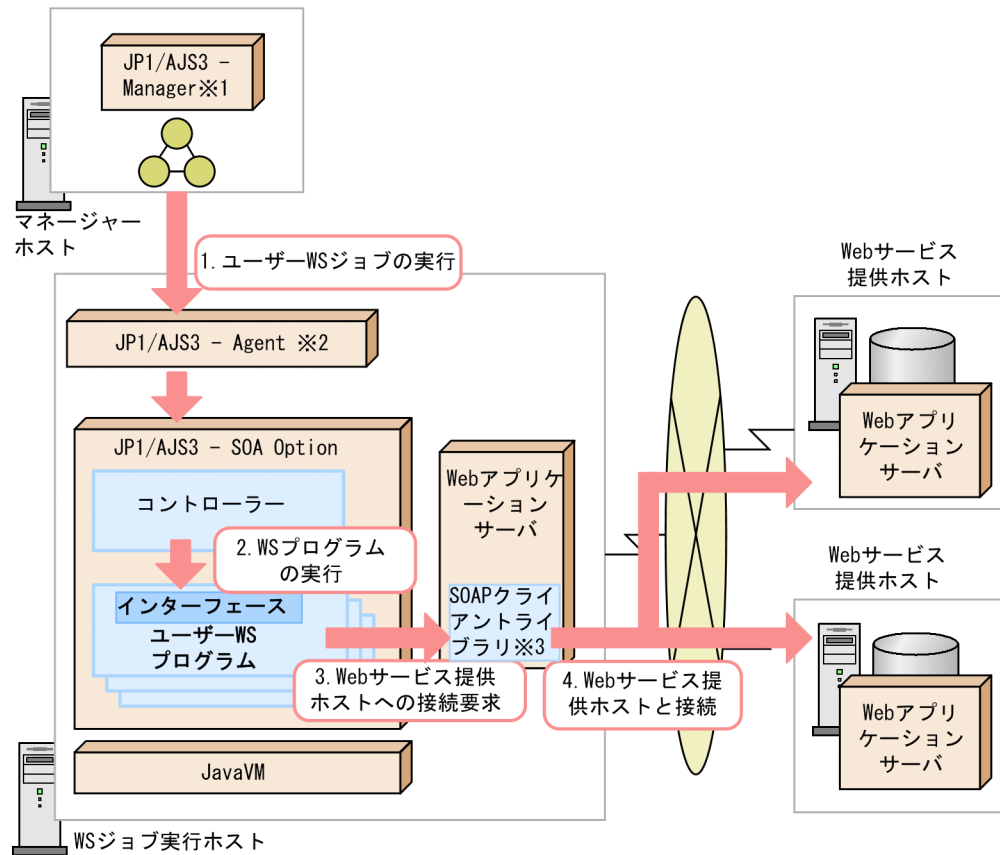
図 2-8 ユーザー WS ジョブが実行される仕組み
