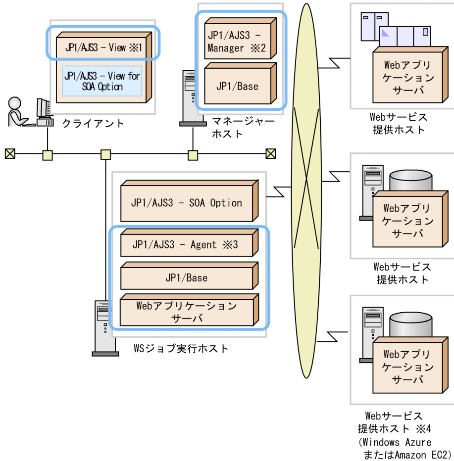
図 4-2 WS ジョブ実行ホストおよびクライアントを使用するために必要なアプリケーション
