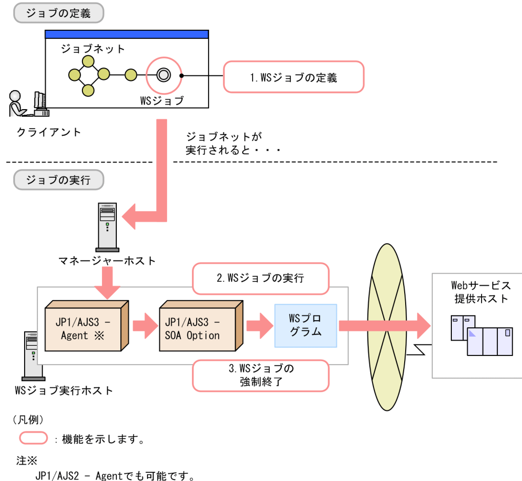
図 2-2 JP1/AJS からの Web システム呼び出し機能概要
