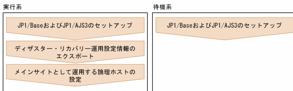
図 18-3 メインサイトのセットアップ手順
