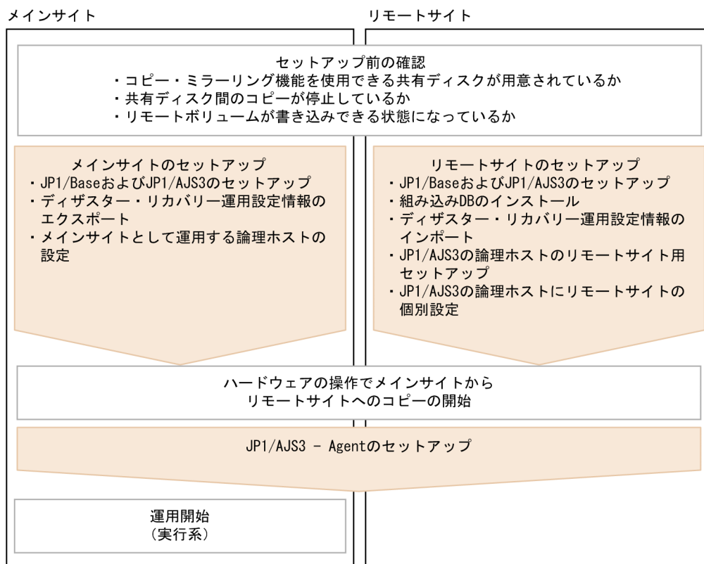
図 9-1 ディザスター・リカバリー運用のセットアップの流れ（メインサイトとリモートサイトの論理ホスト名を別名にする場合）
