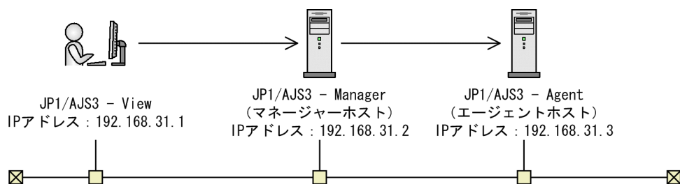
図 4-1 接続元制限の設定例
