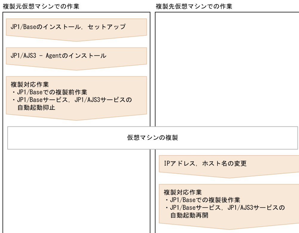
図 H-3 JP1/AJS3 - Agent のインストール後に仮想マシンを複製する場合の流れ
