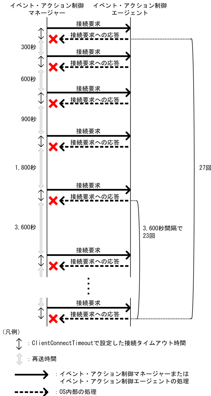
図 6-3 接続タイムアウトが発生した場合のイベント・アクション制御マネージャーとイベント・アクション制御エージェント間での通信の様子
