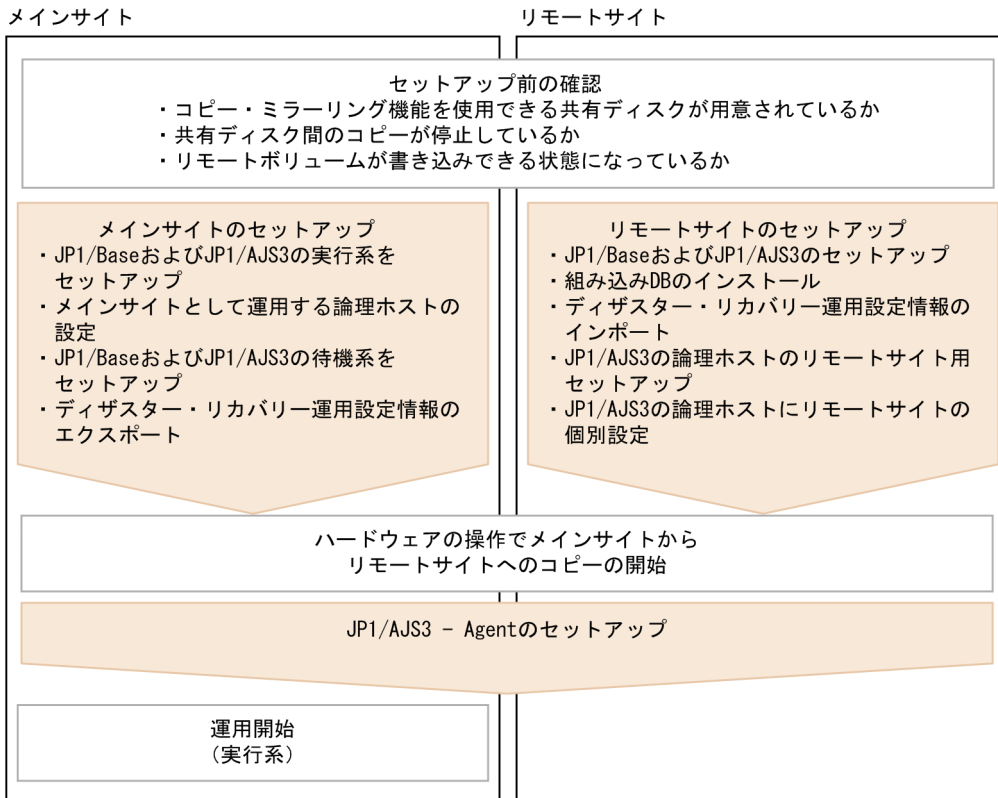
図 18-2 ディザスター・リカバリ運用のセットアップの流れ（メインサイトとリモートサイトの論理ホスト名を同一名にする場合）
