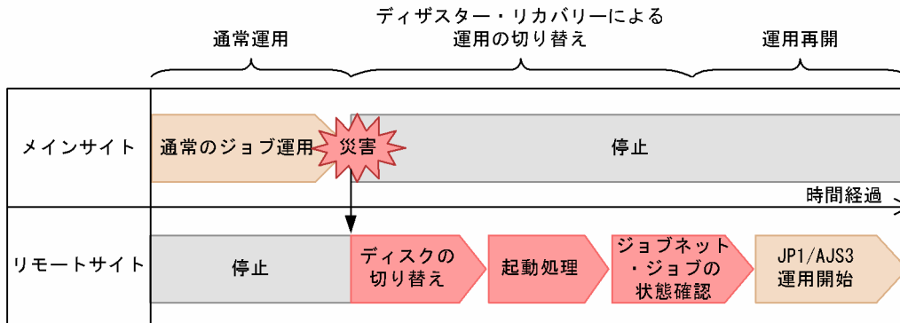
図 5-6 メインサイト停止からリモートサイトでの運用再開までの処理の内訳
