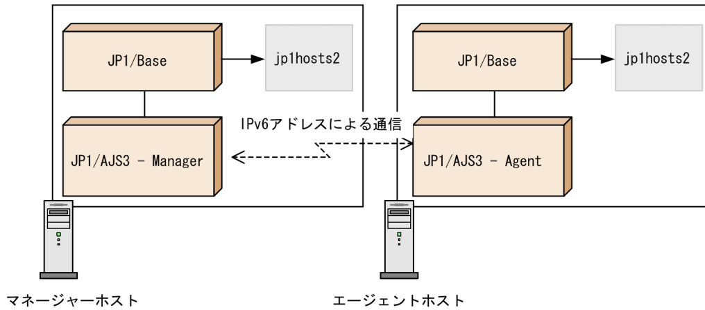
図 2-20 IPv6 アドレスで通信する場合の JP1/Base の通信基盤機能と JP1/AJS3 の関係
