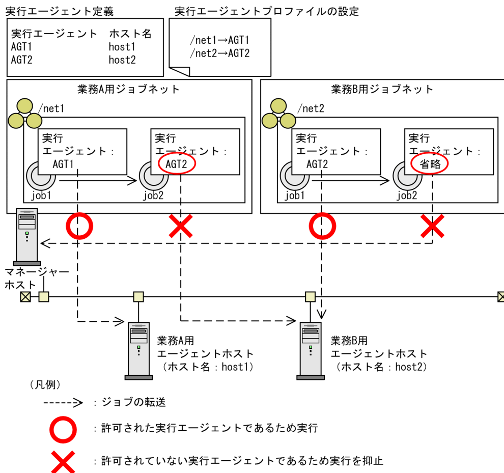
図 2-37 実行エージェント制限の使用例
