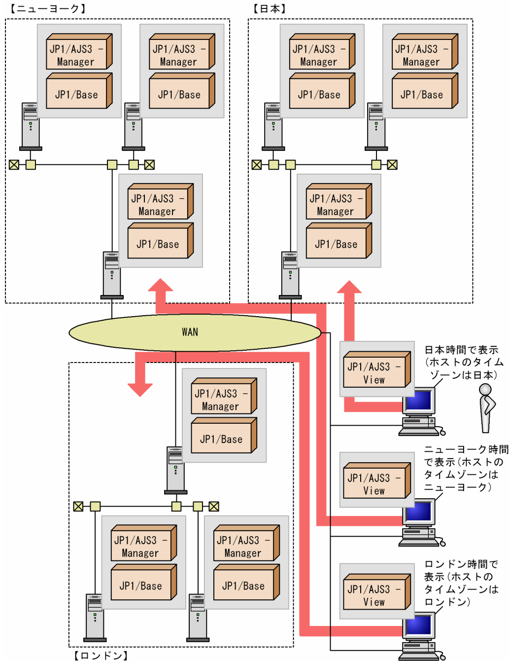
図 2-35 タイムゾーンが異なるマネージャーホストのジョブネットの実行状況を確認する場合のシステム構成例
