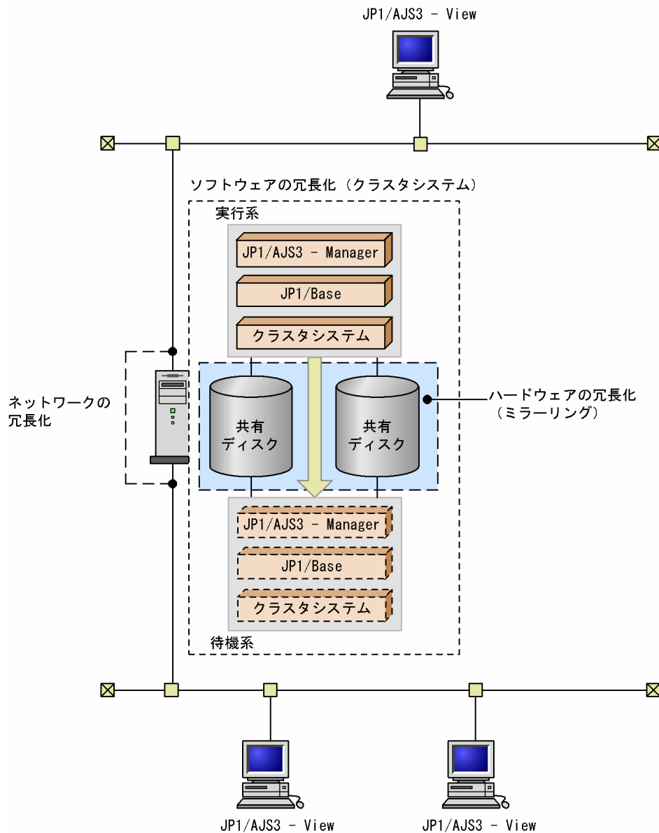
図 5-2 JP1/AJS3 でシステムを冗長化した場合の例
