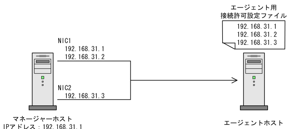
図 2-34 複数 NIC を使用している環境で接続を制限する例
