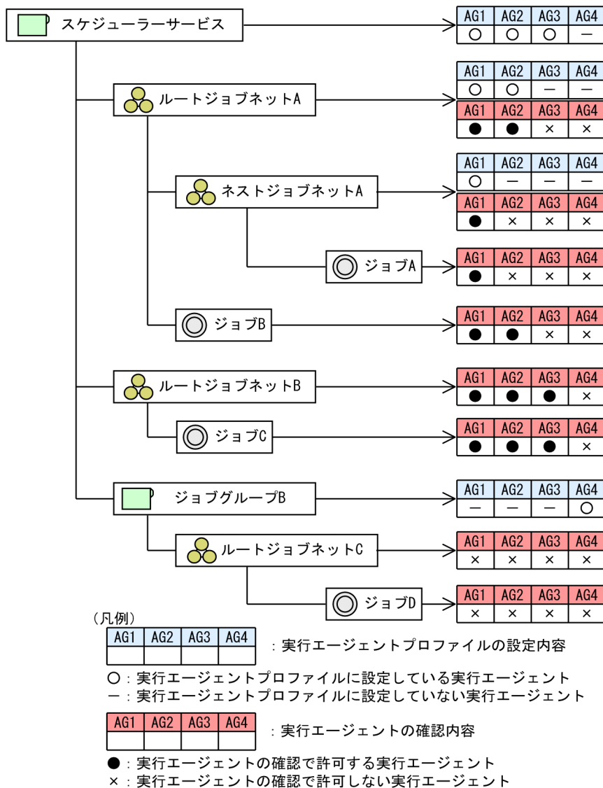
図 2-38 実行エージェントプロファイルの設定と許可する実行エージェント
