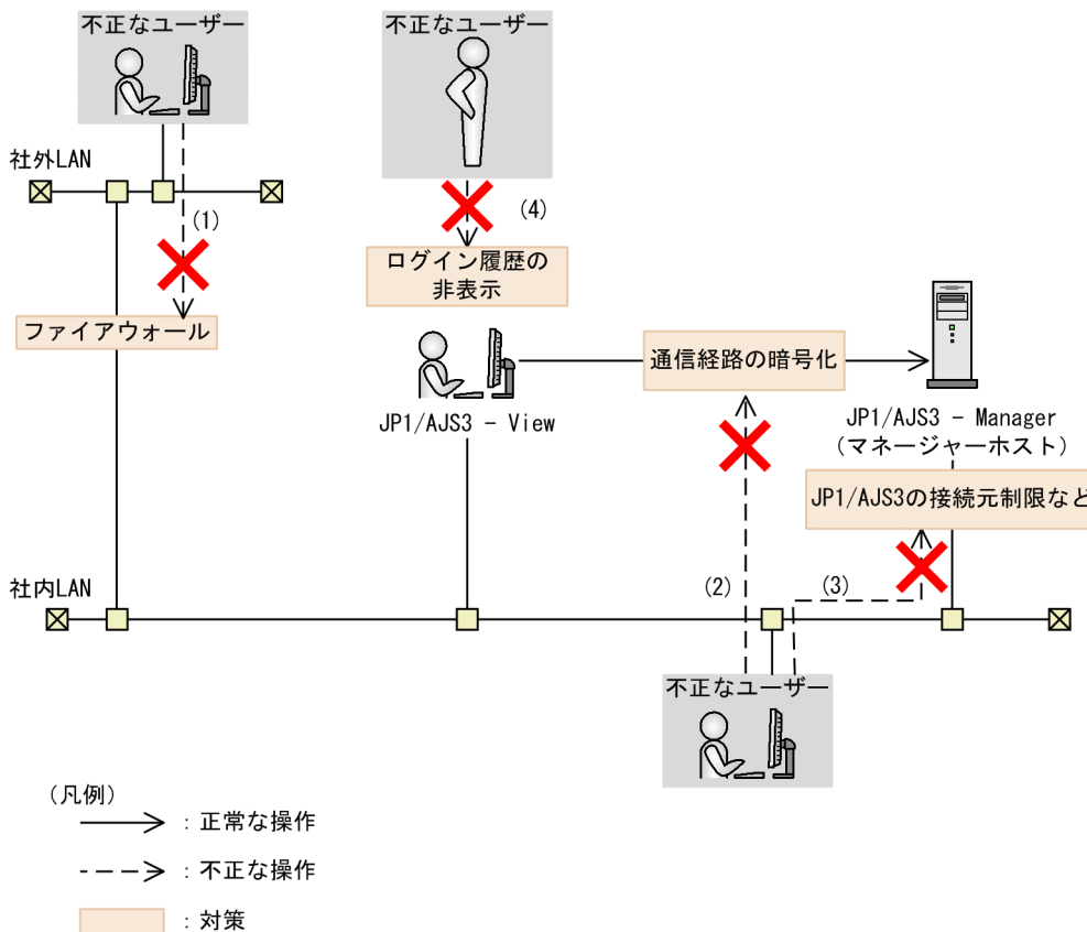
図 2-41 不正なユーザーからのアクセスへの対策
