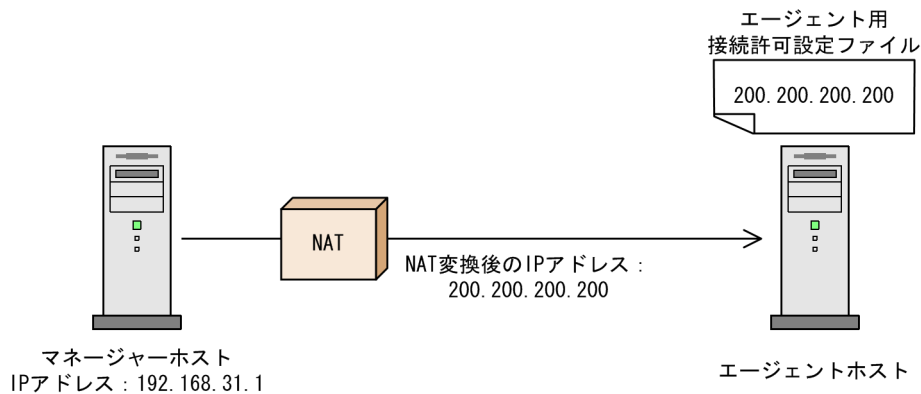
図 2-33 NAT 環境で接続を制限する例
