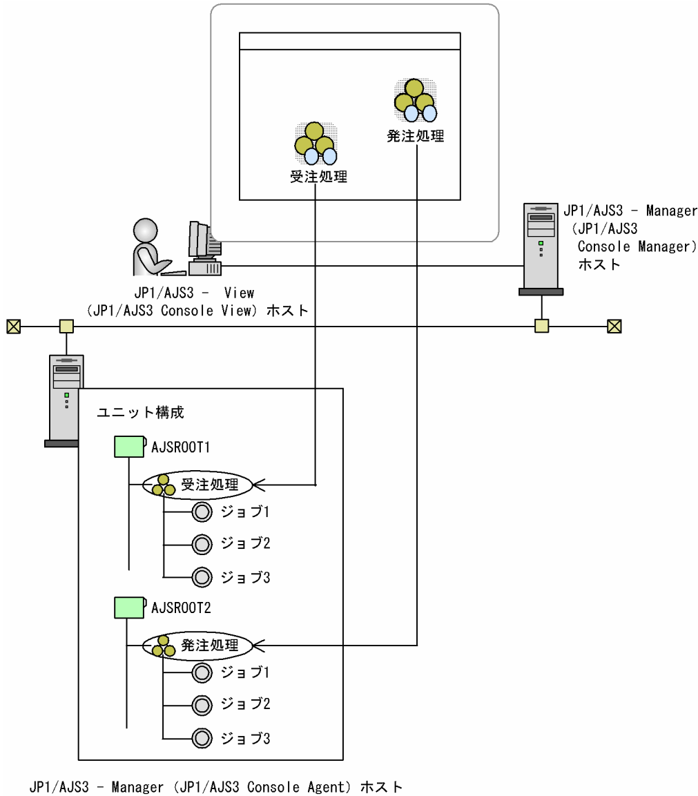
図 2-7 JP1/AJS3 Console での監視例 (1 台のマネージャーホストで管理する業務を監視する場合)
