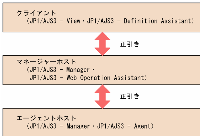
図 2-28 JP1/AJS3 各製品での正引きの解決について必要な設定
