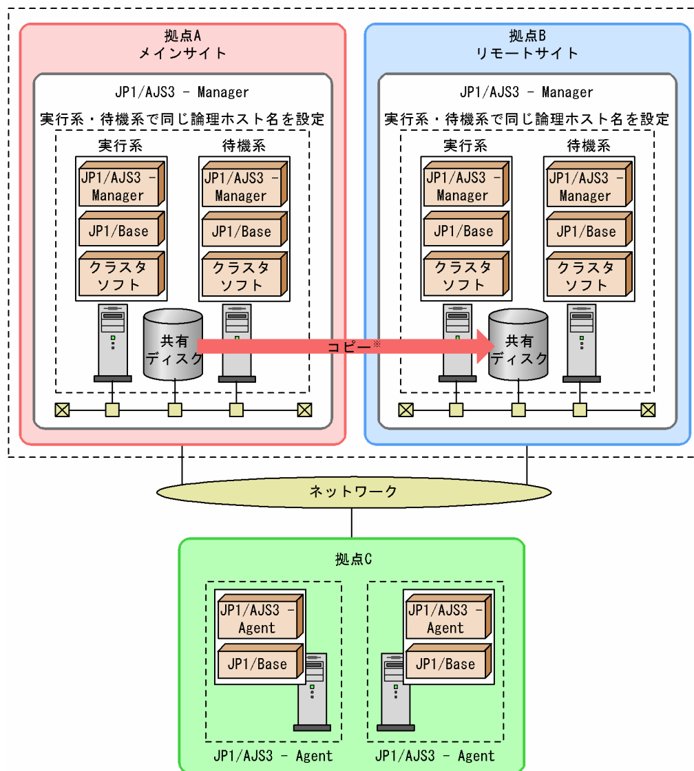
図 2-13 JP1/AJS3 が対応するディザスター・リカバリーのシステム構成例（クラスタ構成・エージェント共有型）
