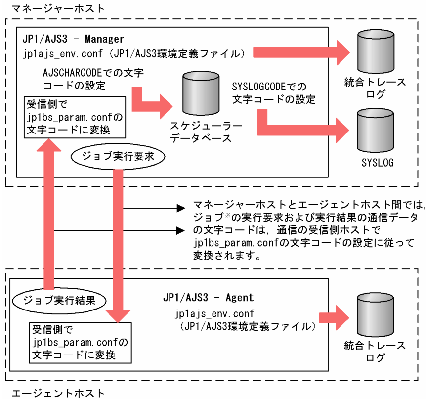
図 2-36 文字コード種別の変更時の影響範囲
