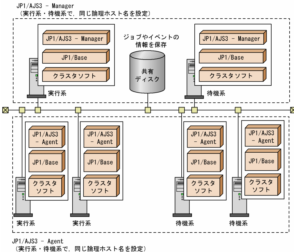
図 2-12 クラスタ運用時のシステム構成例
