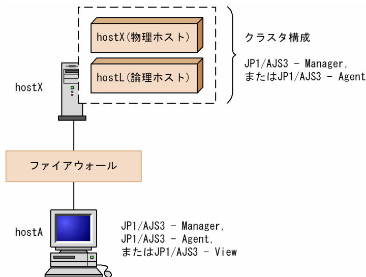
図 2-27 クラスタ運用する場合のファイアウォール構成例
