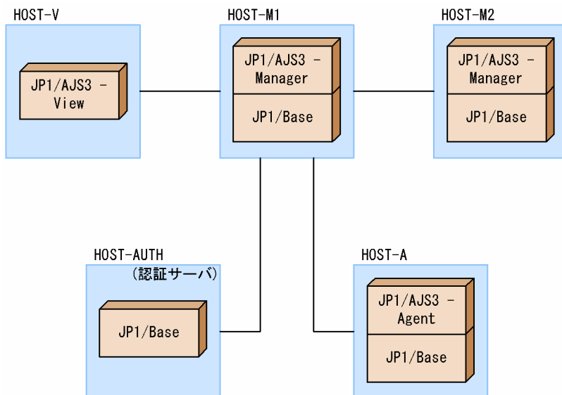
図 2-19 システム構成例
