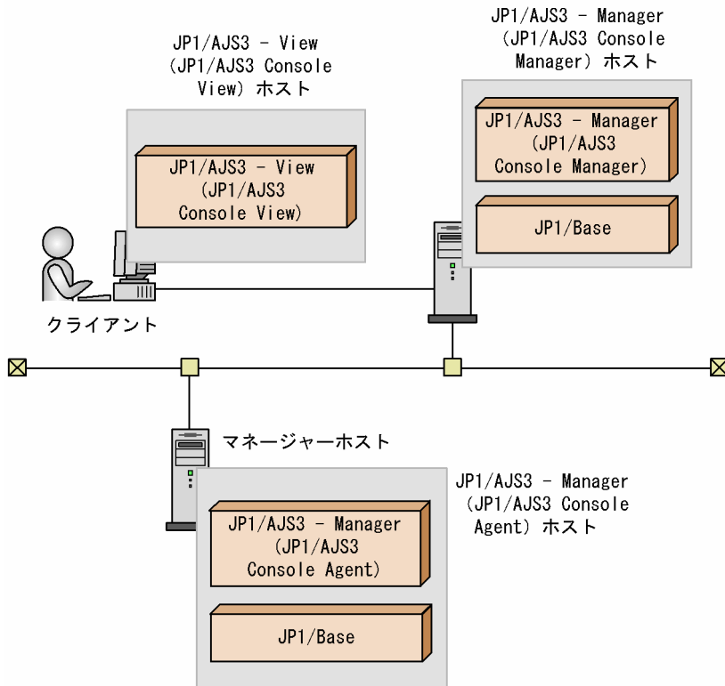
図 2-6 1 台のマネージャーホストで管理する業務を監視する場合のシステム構成
