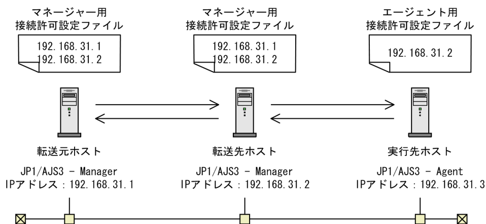
図 2-31 リモートジョブネットを実行する場合の設定例
