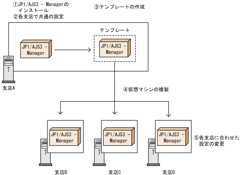
図 F-2 JP1/AJS3 - Manager をセットアップした仮想マシンを複製する運用例
