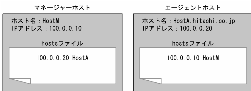
図 2-11 hosts ファイルでホスト名をショート名で定義している例
