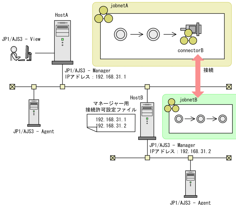
図 2-32 ジョブネットコネクタの例
