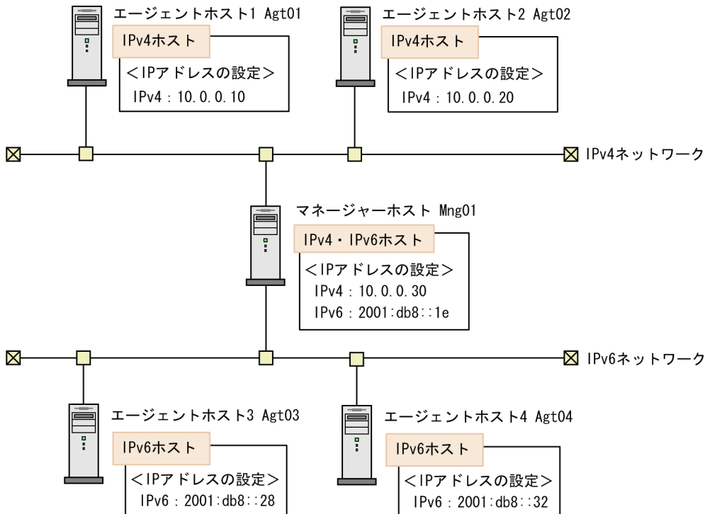
図 2-24 IPv6 アドレスを使用した環境の構成例
