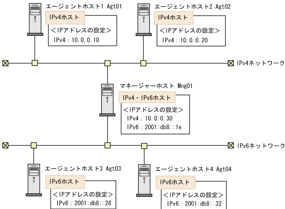
図 2-21 IPv6 環境でのシステム構成例
