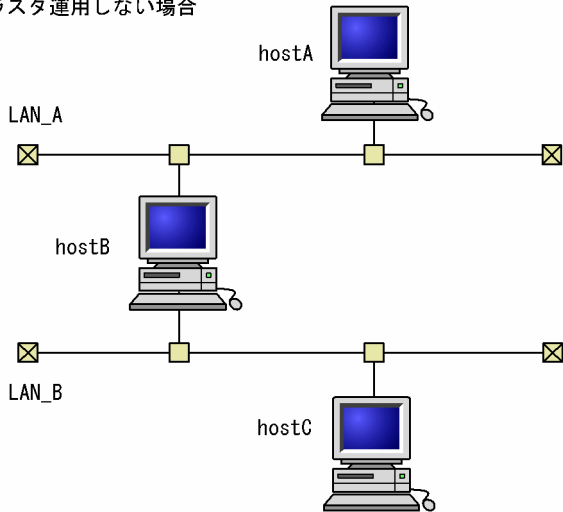
図 2-15 複数の LAN に接続したシステム構成例
