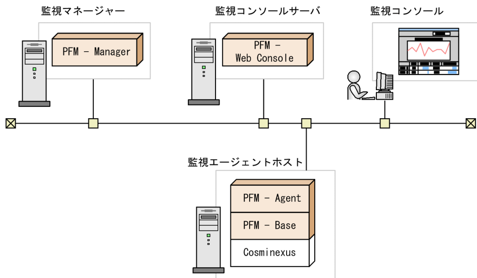
図 2-2 プログラムの構成
