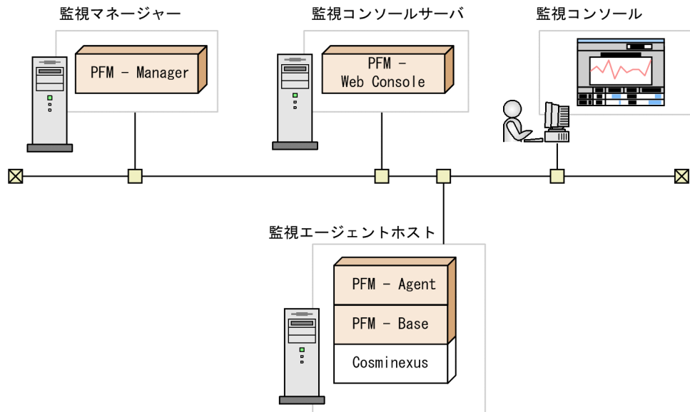
図 3-2 プログラムの構成
