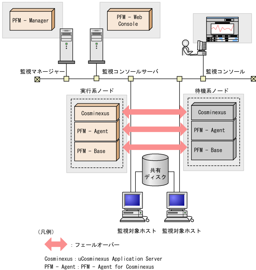
図 4-1 HA クラスタシステムでの PFM - Agent for Cosminexus の構成例
