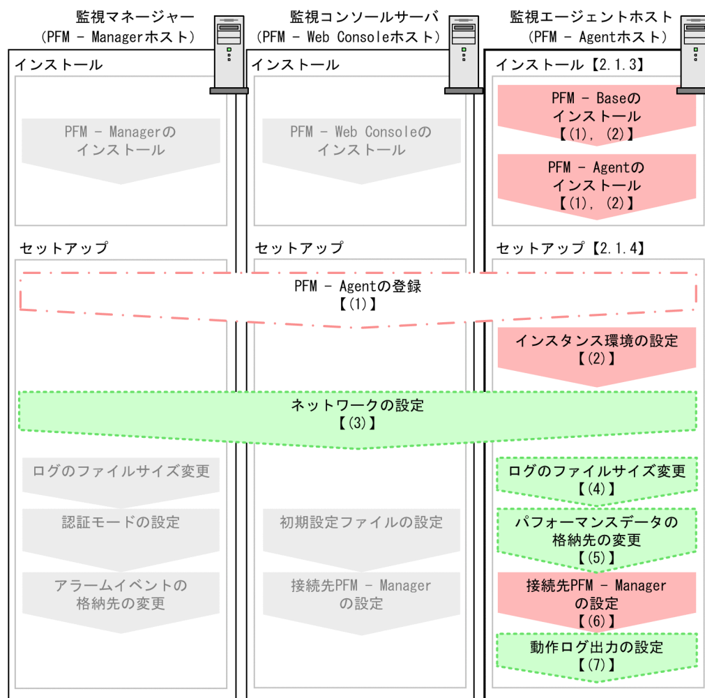
図 2-1 インストールとセットアップの流れ (Windows の場合)
