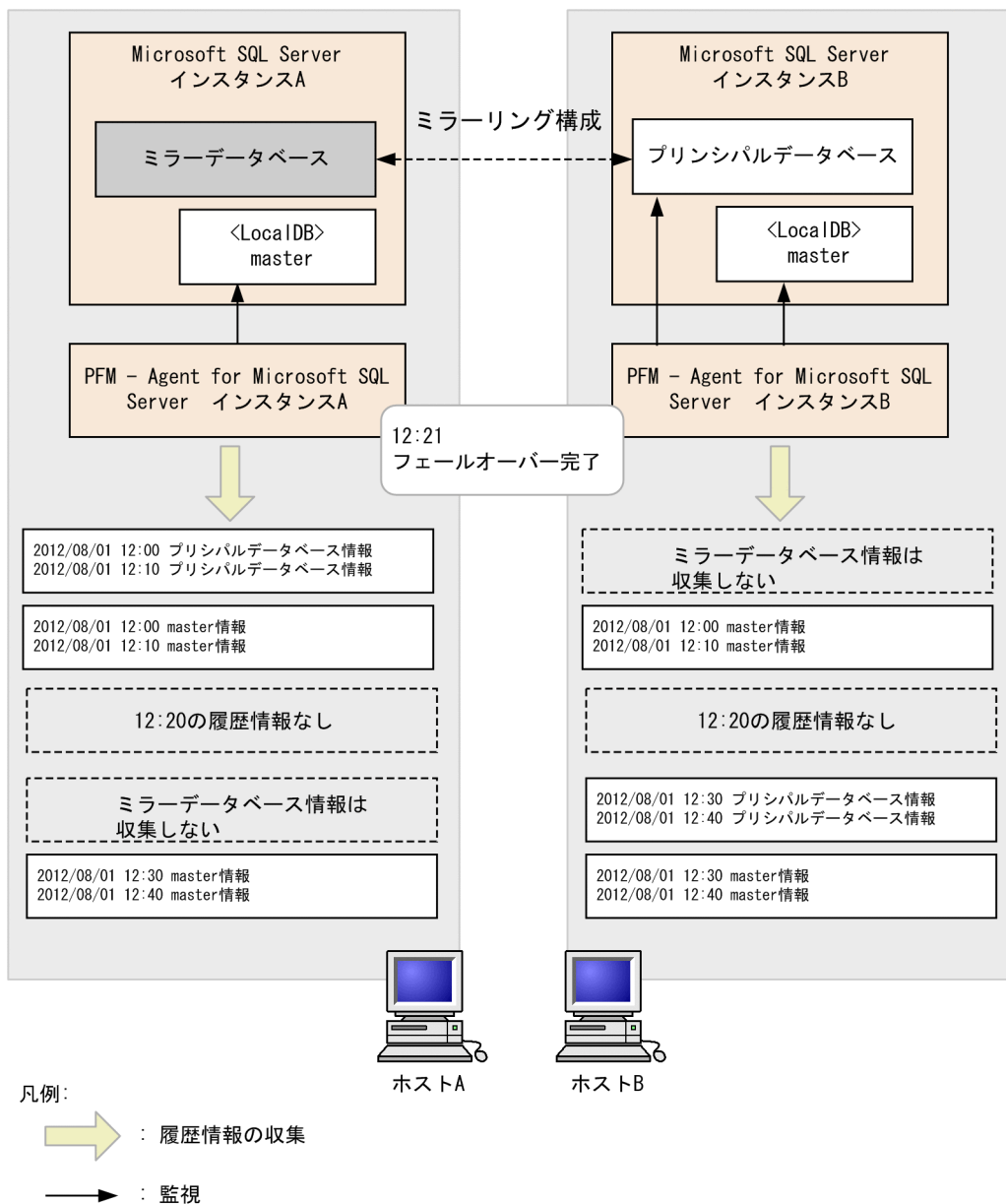
図 2-7 フェールオーバー後の監視
