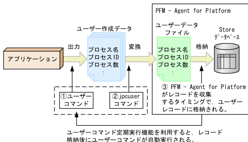
図 6-1 ユーザー独自のパフォーマンスデータを収集する仕組み
