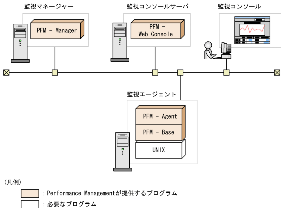
図 4-2 プログラムの構成図
