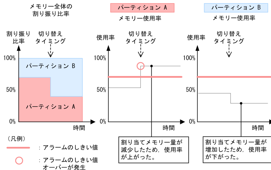
図 2-6 メモリリソースをアラームに組み込んだときのケース
