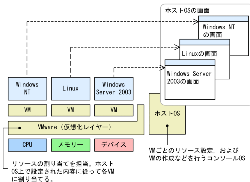
図 2-13 VMware の構造
