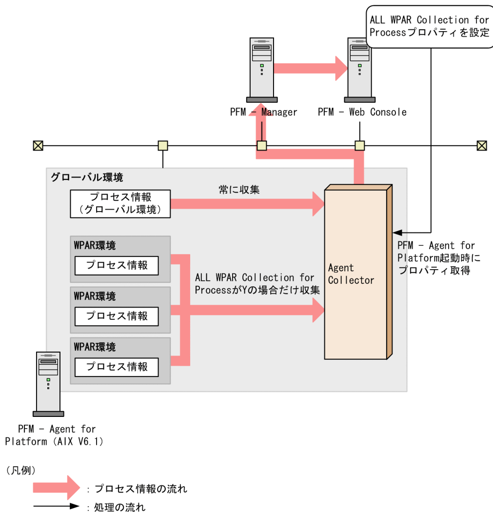
図 2-14 グローバル環境上で収集するプロセス情報
