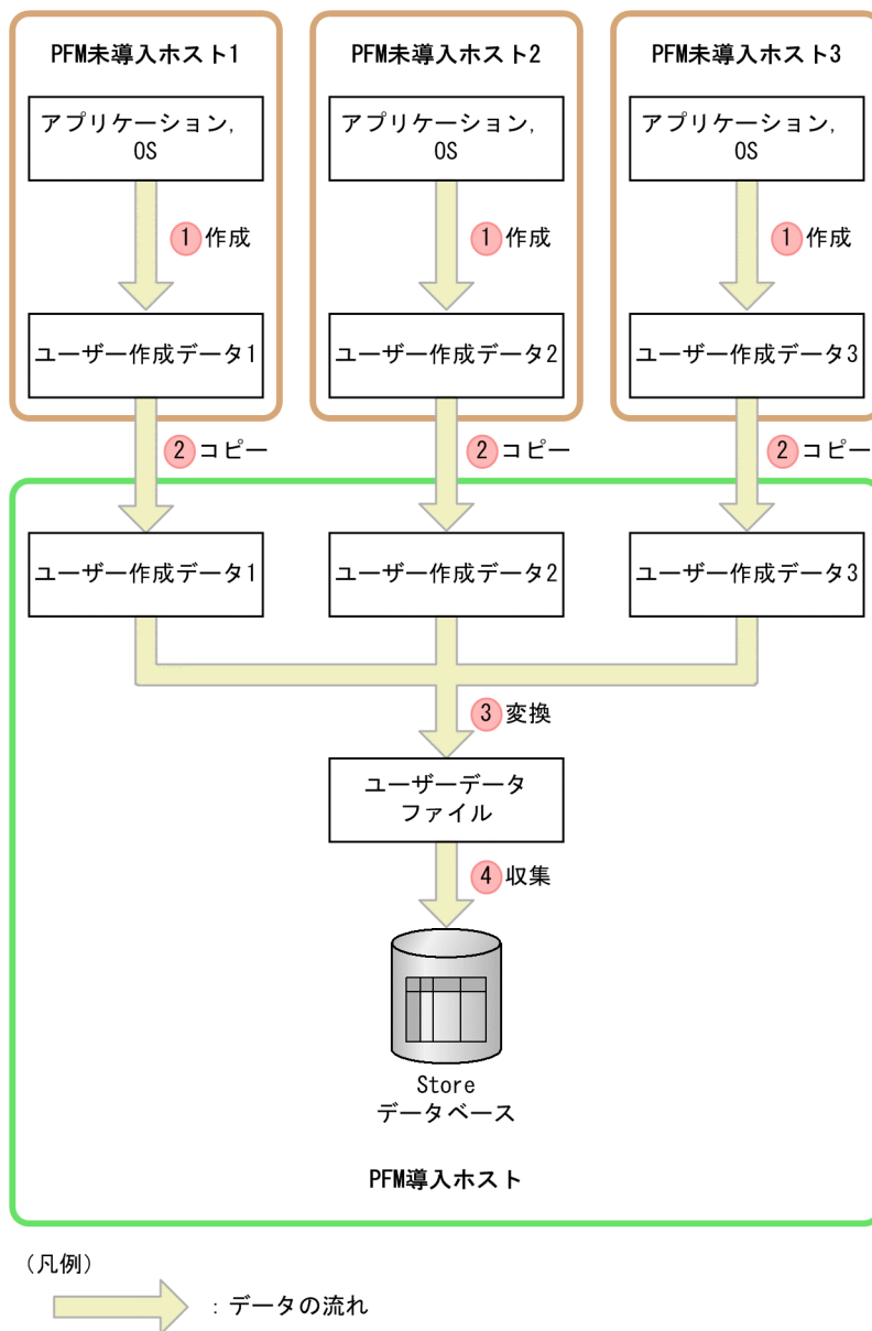
図 3-5 PFM 製品が導入されていないホストのデータ収集の流れ
