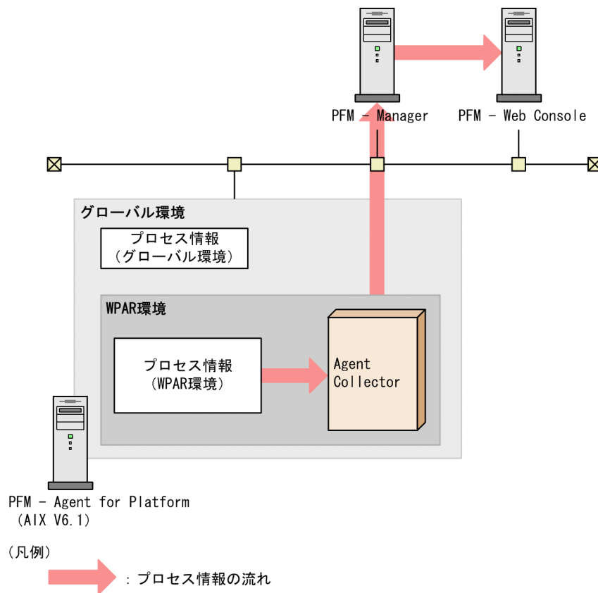
図 2-15 System WPAR 環境上で収集するプロセス情報
