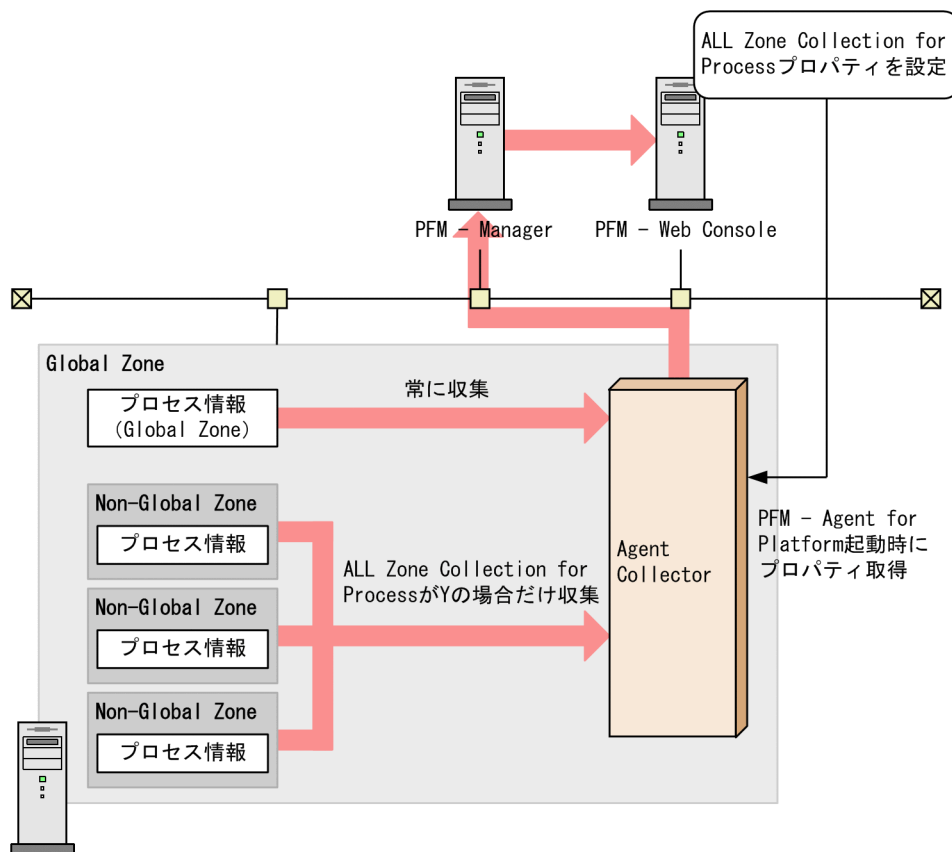
図 2-9 Global Zone 上で収集するプロセス情報
