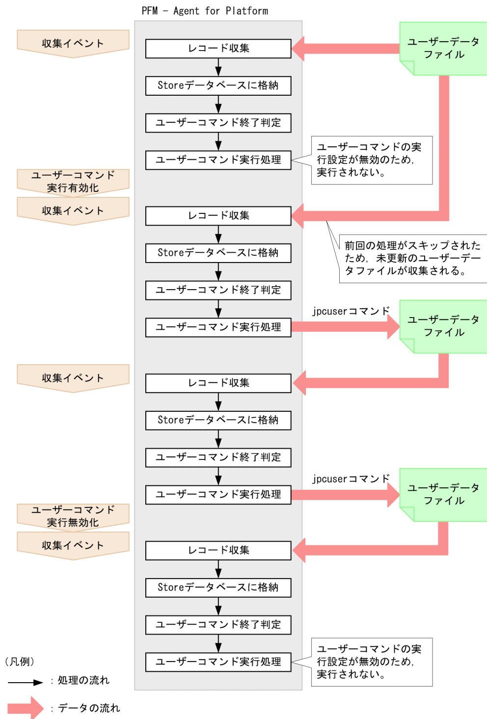
図 6-2 ユーザーコマンド定期実行機能の処理の流れ
