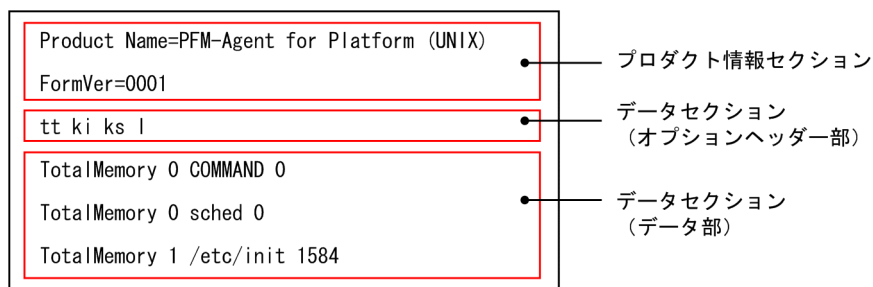
図 6-4 ユーザー作成データの構成例
