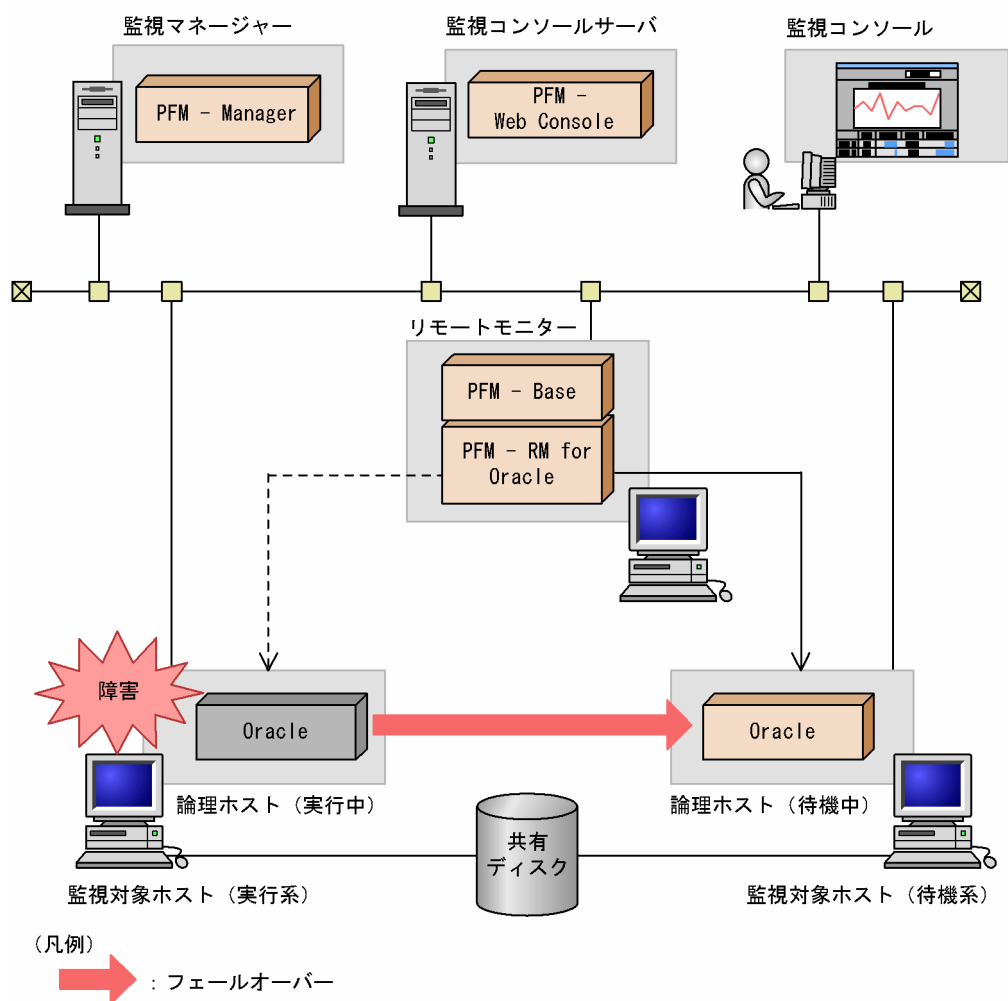
図 1-1 Oracle Database がクラスタシステムの場合に PFM - RM for Oracle を運用する場合の運用例
