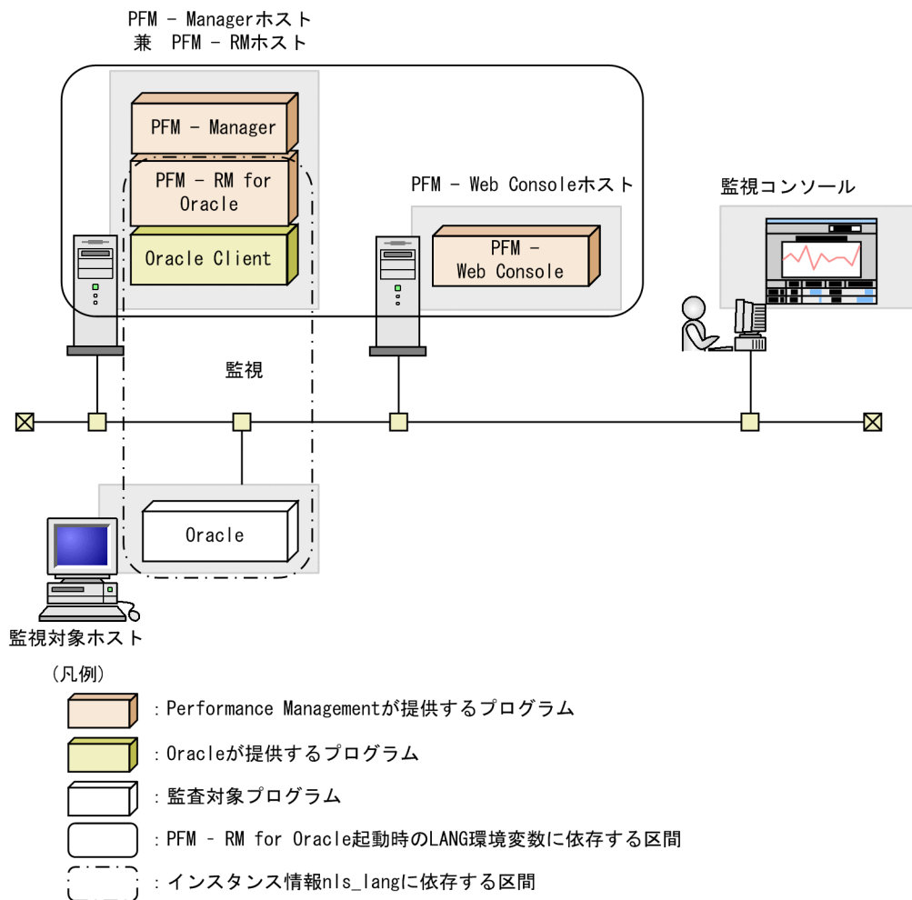
図 2-10 データと設定値との関係
