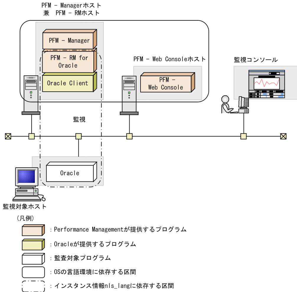
図 2-11 データと設定値との関係
