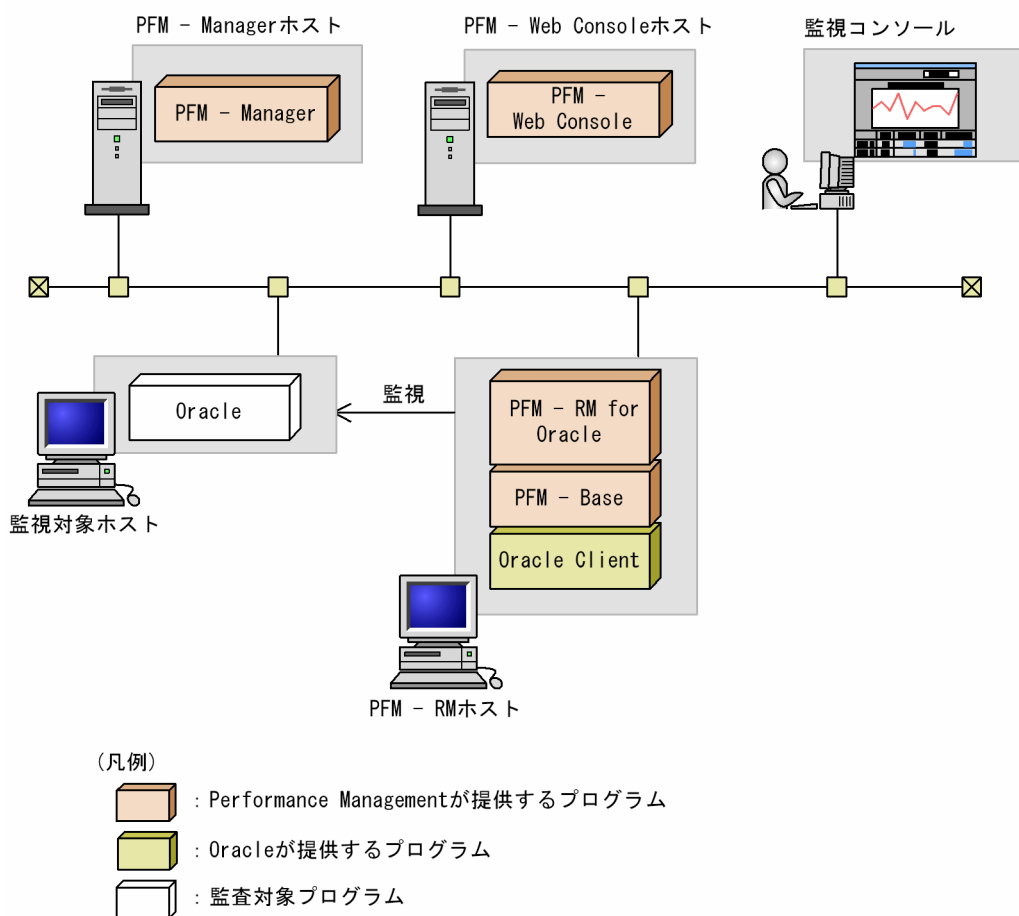
図 2-2 プログラムの構成 (PFM - Base, および Oracle Client と同一ホストに PFM - RM for Oracle をインストールする場合 (Windows の場合))
