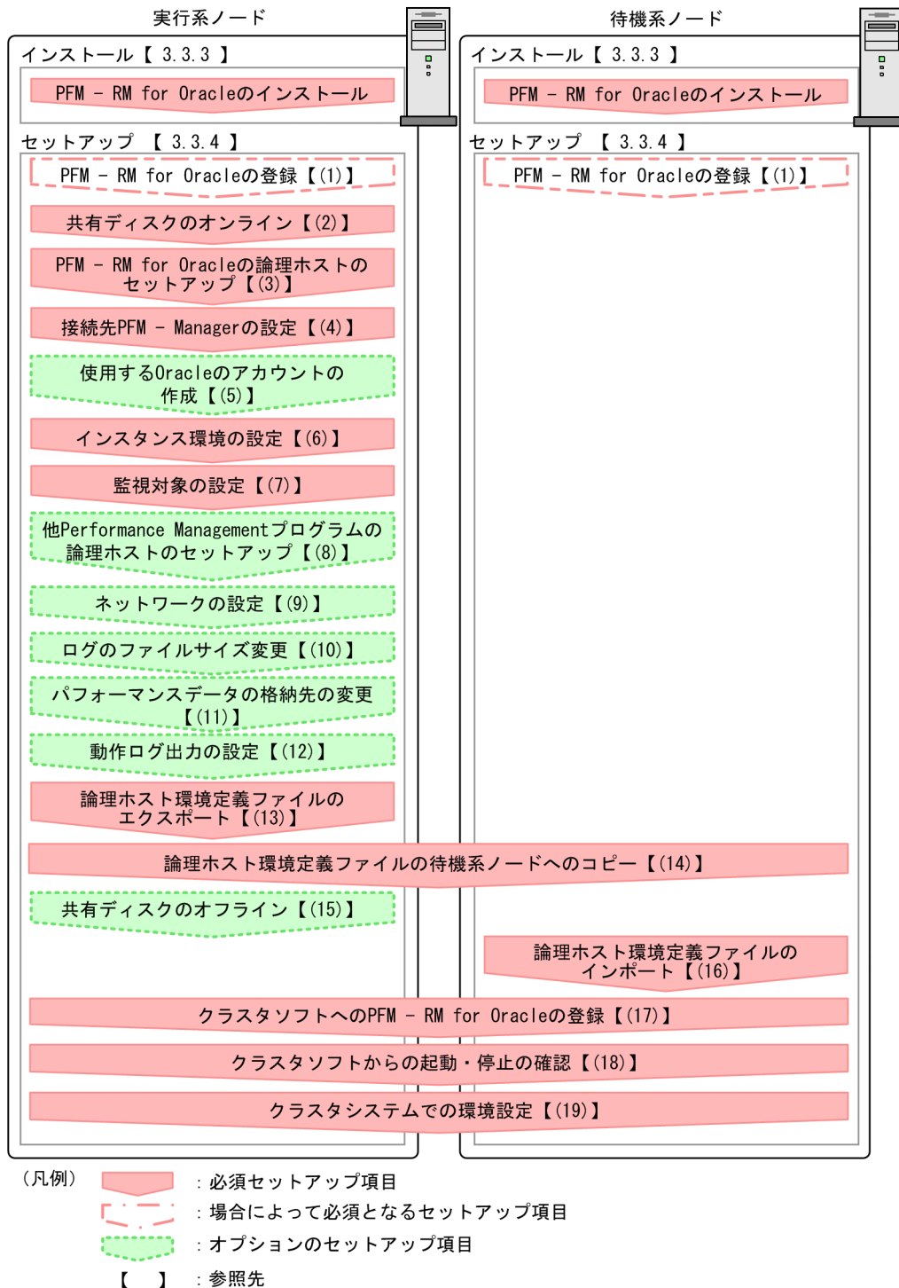
図 3-6 クラスタシステムで論理ホスト運用する PFM - RM for Oracle のインストールおよびセットアップの流れ (Windows の場合)
