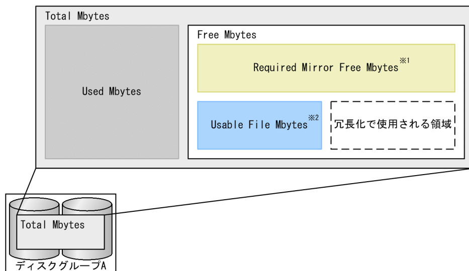
図 5-1 ASM Disk Group Interval (PI_PIDG) レコードの空き容量に関するフィールド構成
