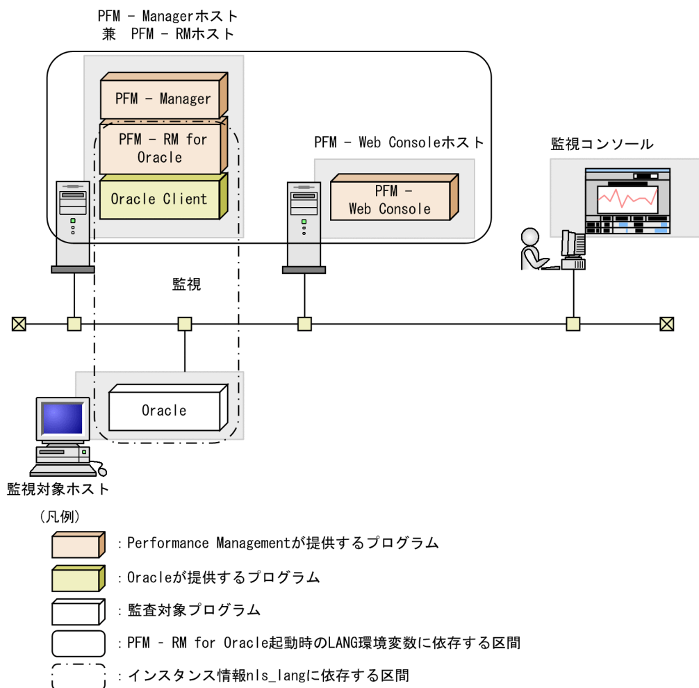
図 2-12 データと設定値との関係
