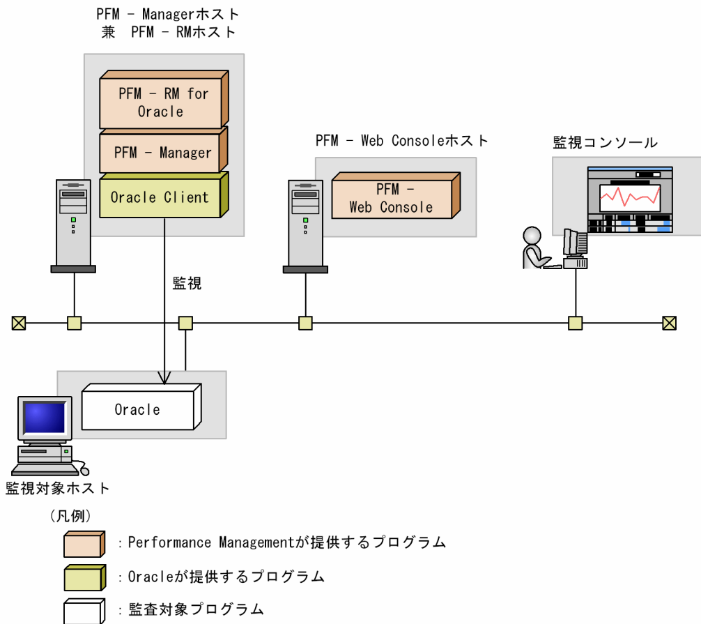
図 2-6 プログラムの構成 (PFM - Manager と同一ホストに PFM - RM for Oracle をインストールする場合 (UNIX の場合))
