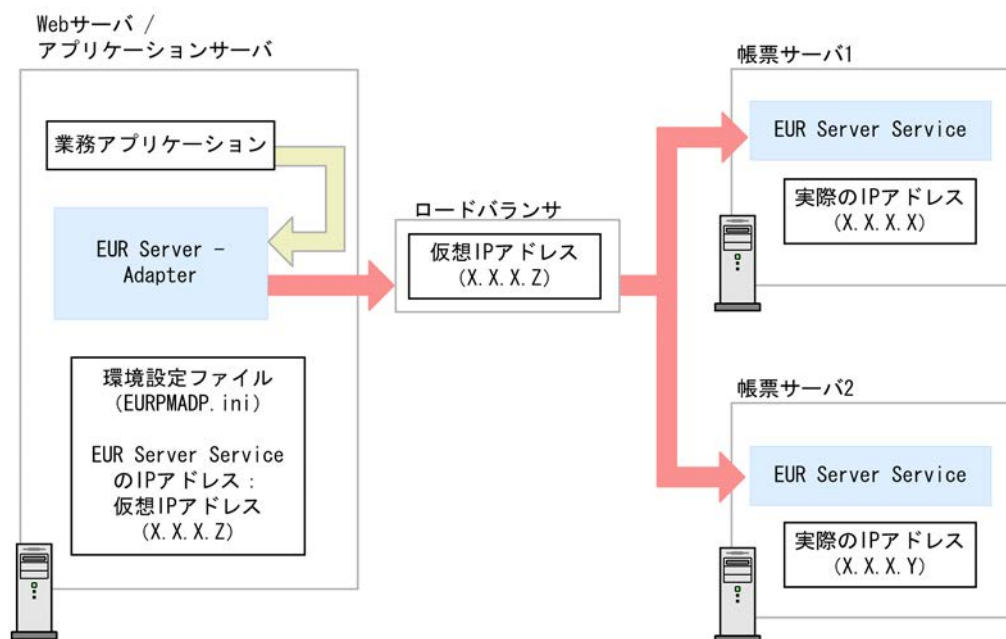
図 2-1 ロードバランサを使用した構成例
