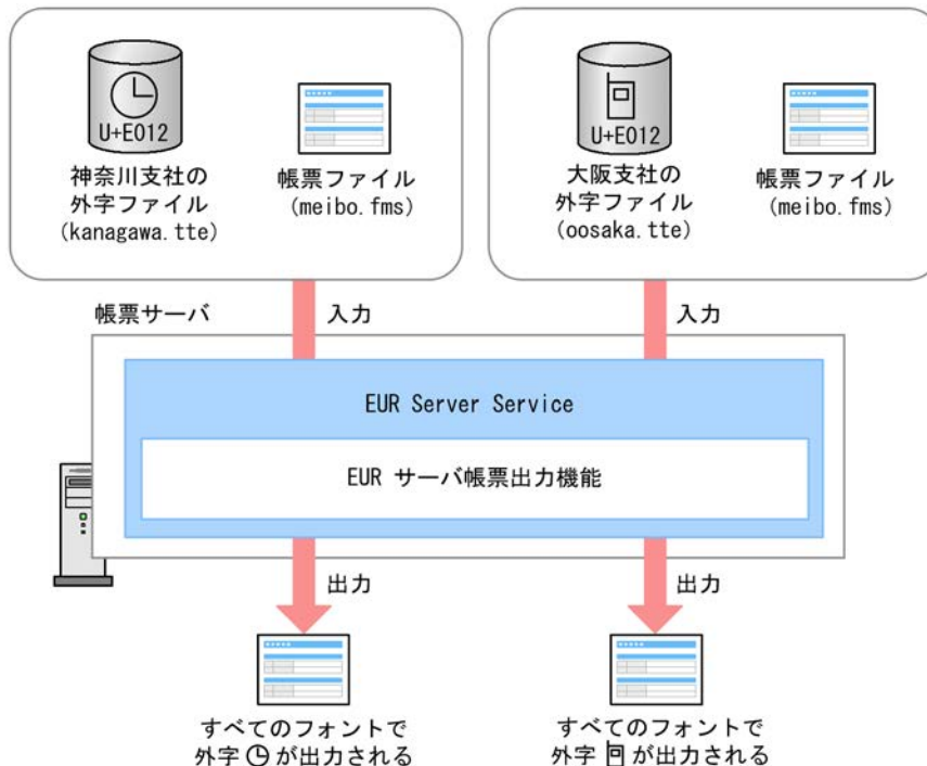
図 4-1 同じ帳票に別の外字を出力するイメージ
