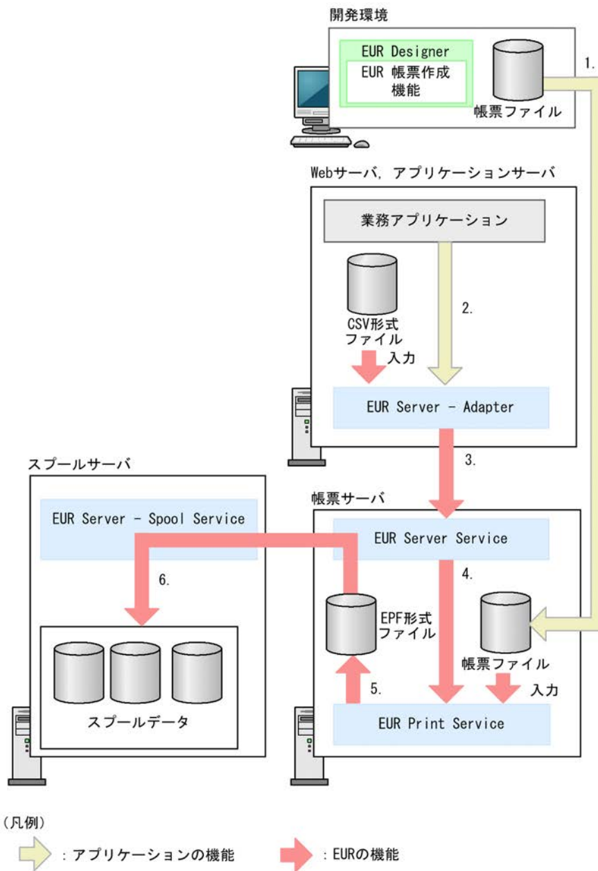
図 1-8 帳票を蓄積するときのデータの流れ
