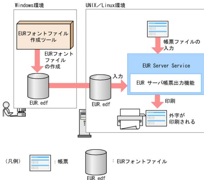
図 4-3 EUR フォントファイルを使用した外字の出力
