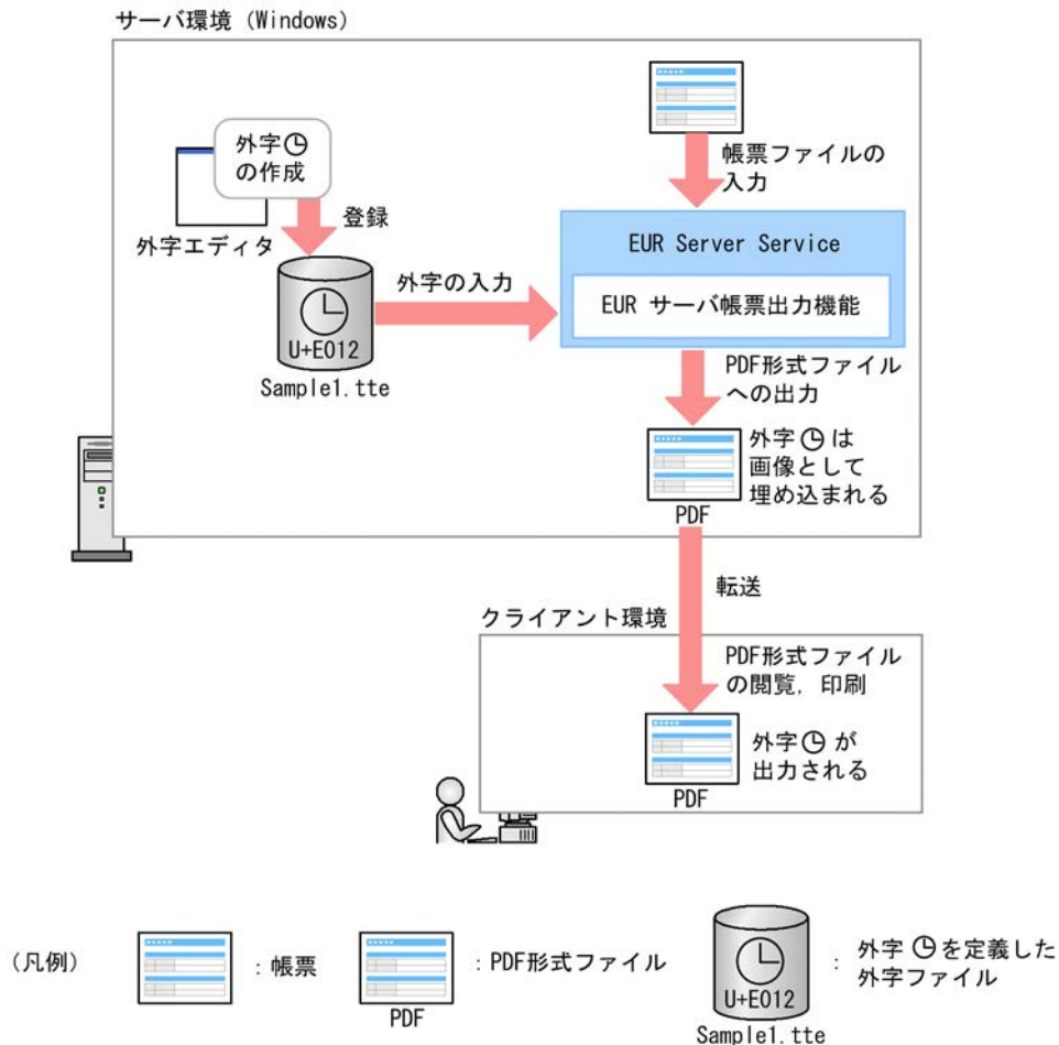
図 4-2 Windows 環境での外字を含む帳票の PDF 形式ファイル出力
