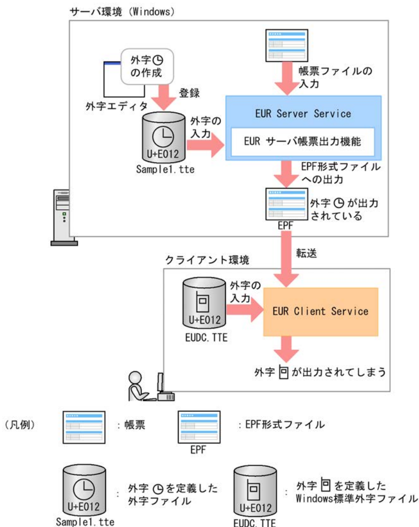
図 4-4 帳票を EPF 形式ファイルに出力する場合（クライアント環境の Windows 標準外字ファイル（EUDC.TTE）に別の外字が定義されたとき）
