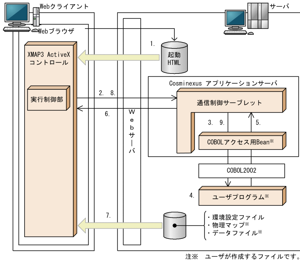
図 3-4 Cosminexus ベースのシステムの動作 (COBOL)
