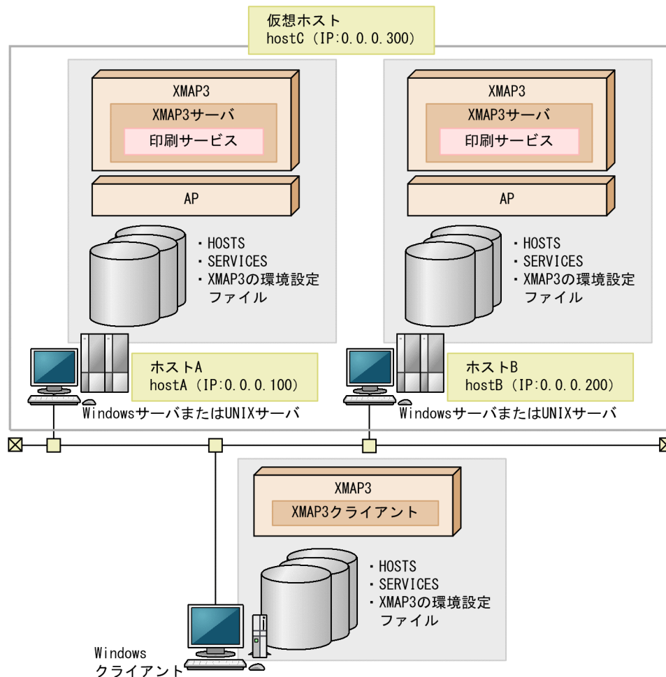
図 6-6 クラスタ構成の例
