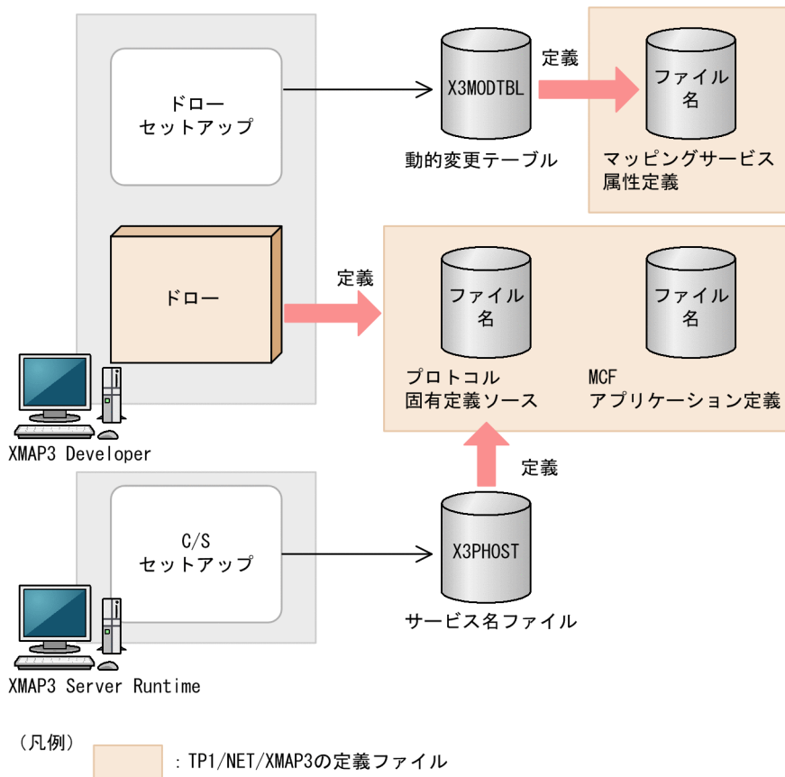
図 11-2 OLTP サーバ構成の環境セットアップの概要
