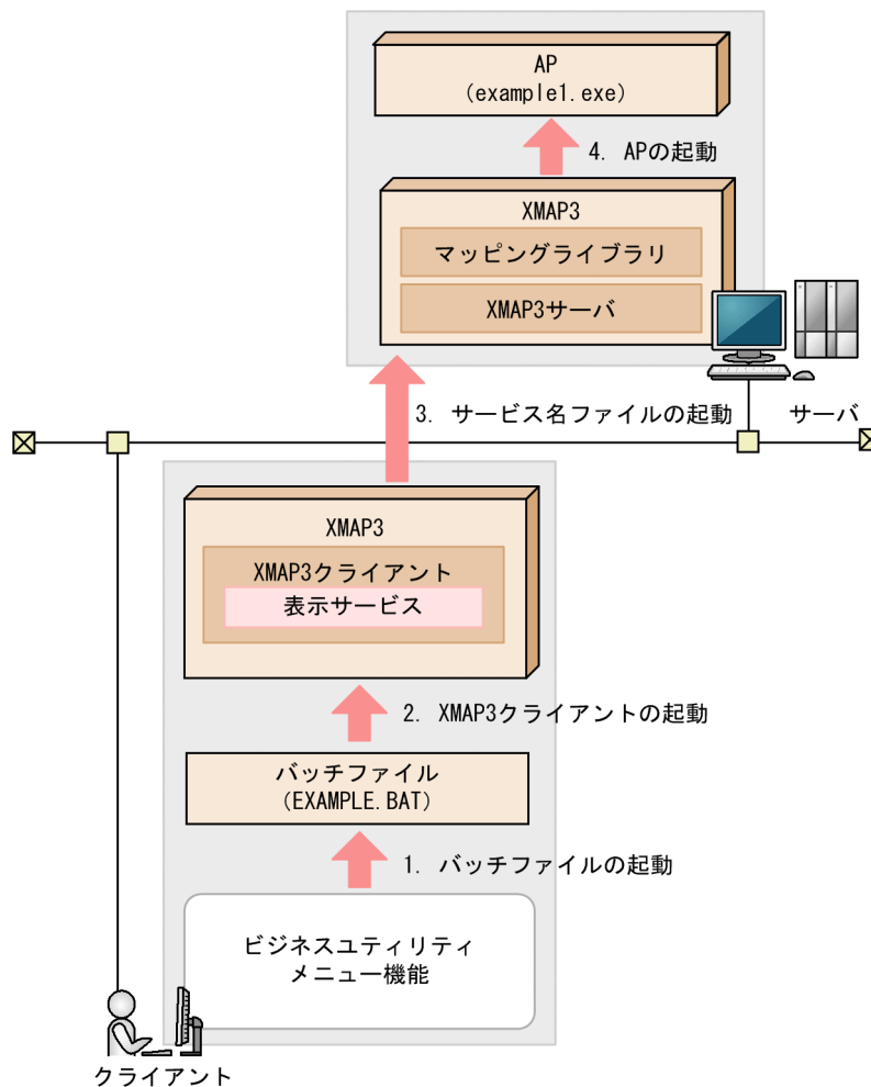
図 6-7 XMAP3 とビジネスユティリティの連携
