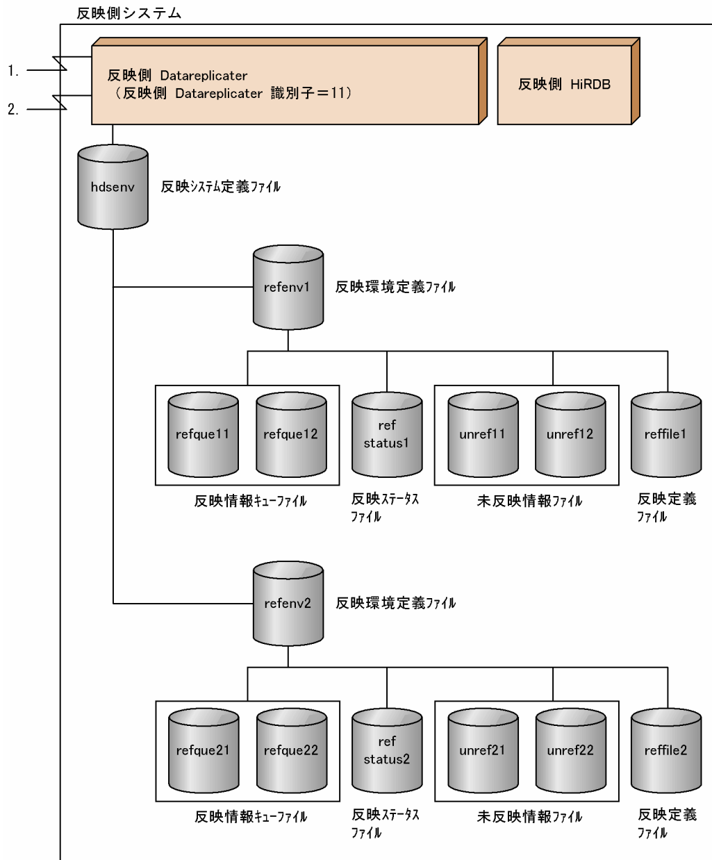
図 5-14 システムの対応とファイルの構成例 2
