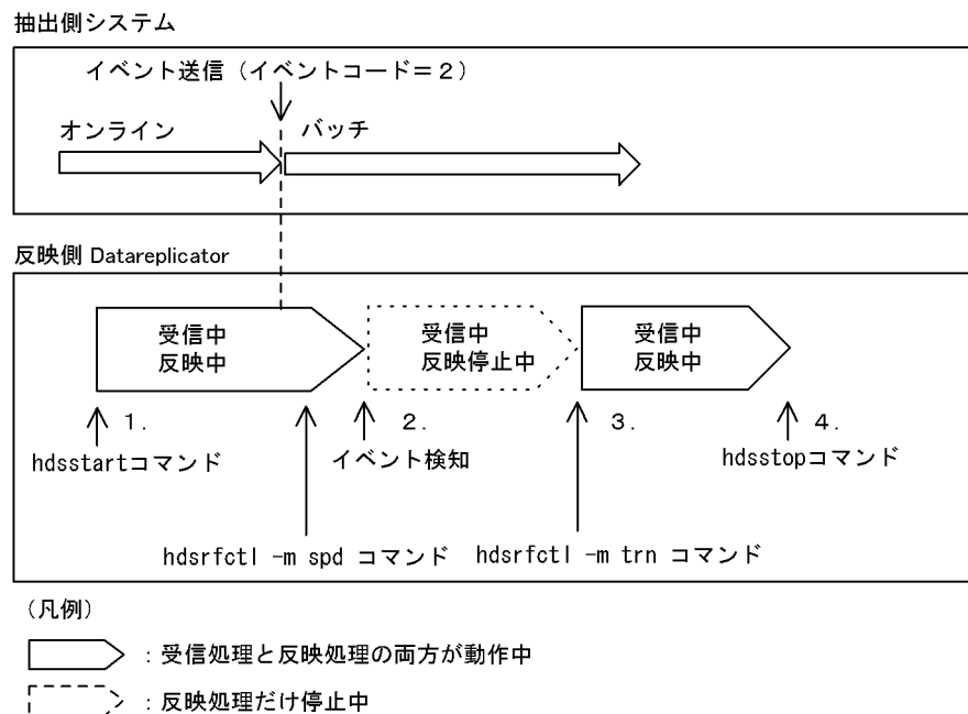
図 6-20 反映処理方式の切り替えの運用例
