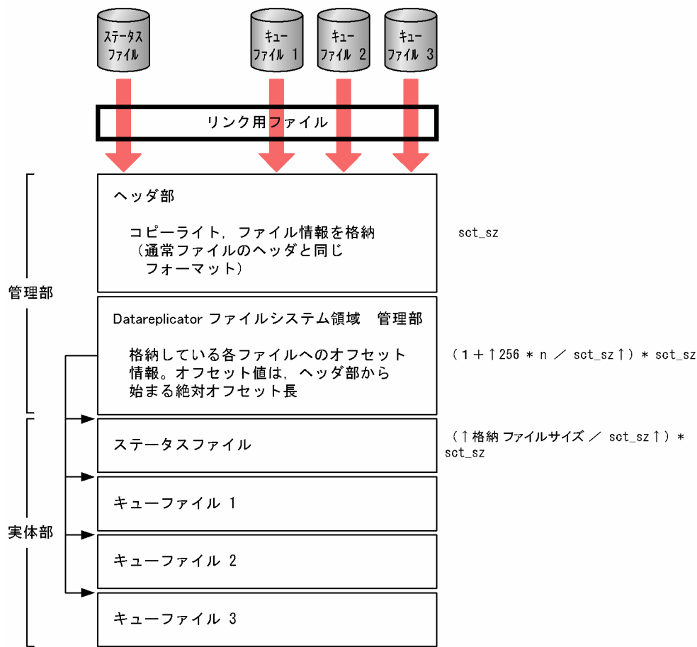
図 3-29 Datareplicator ファイルシステム領域の構造
