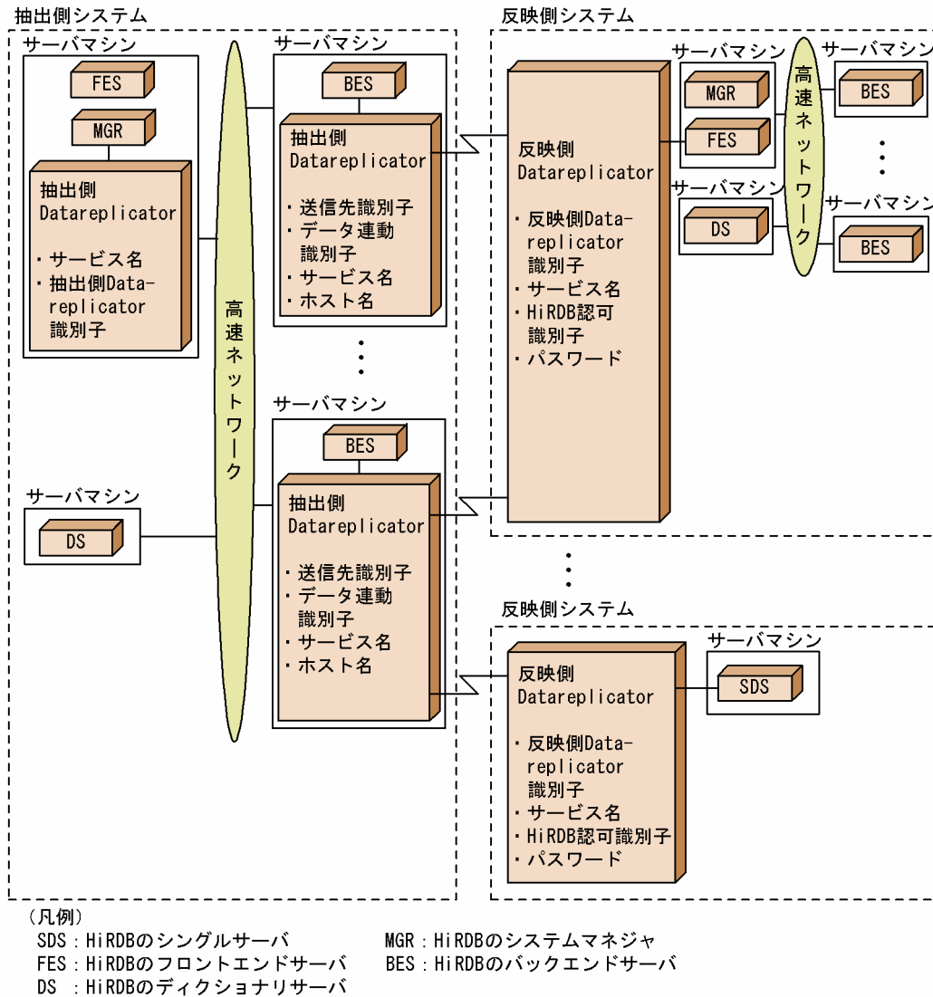
図 4-17 HiRDB から HiRDB へデータ連動する場合の、抽出側システムと反映側システムとの対応（抽出側 HiRDB が平行サーバの場合）
