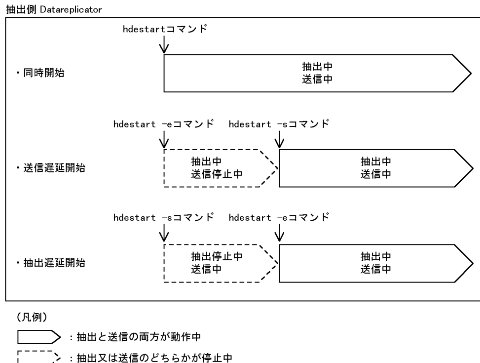
図 4-36 抽出処理の開始方式と開始タイミングの関係
