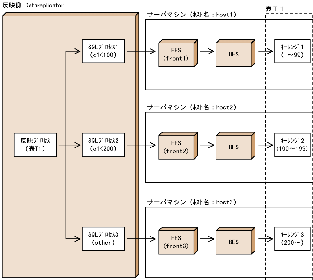
図 4-42 キーレンジ単位分割方式でマルチ FES 機能を使う例
