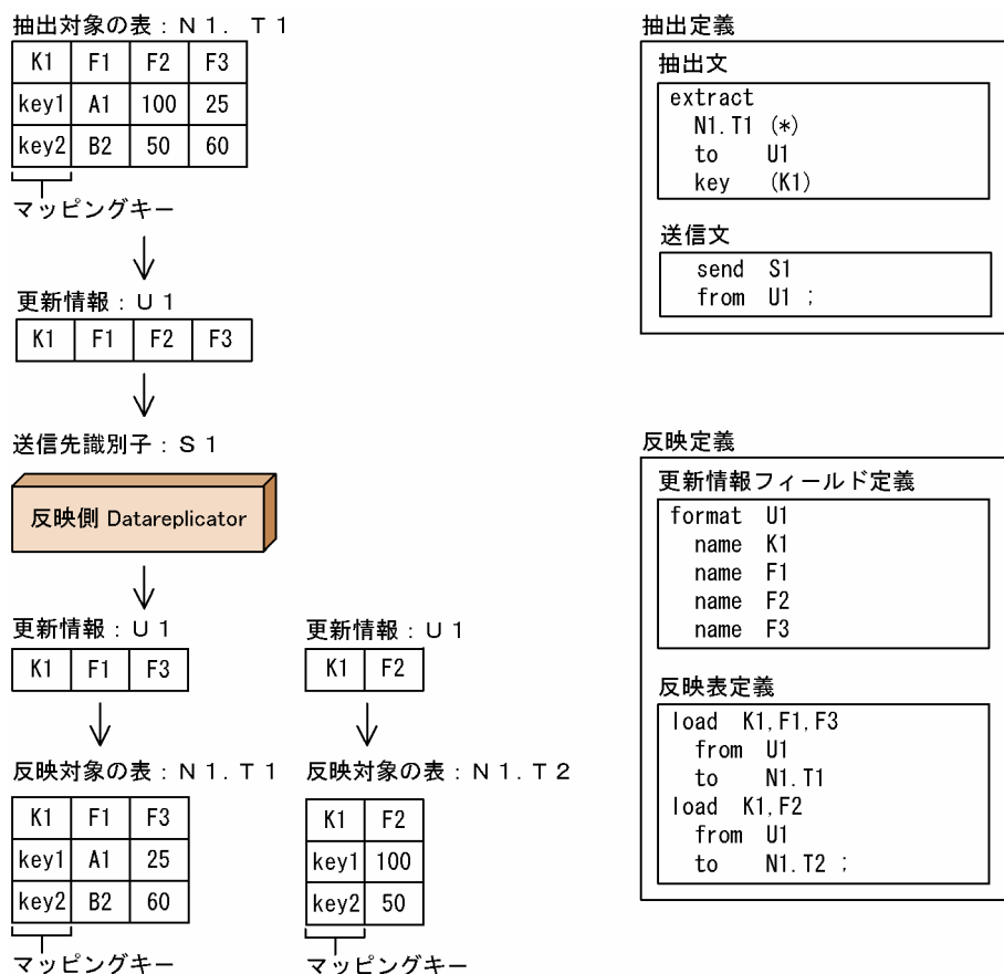
図 4-11 一つの抽出対象表を反映側で複数に分割して反映する例
