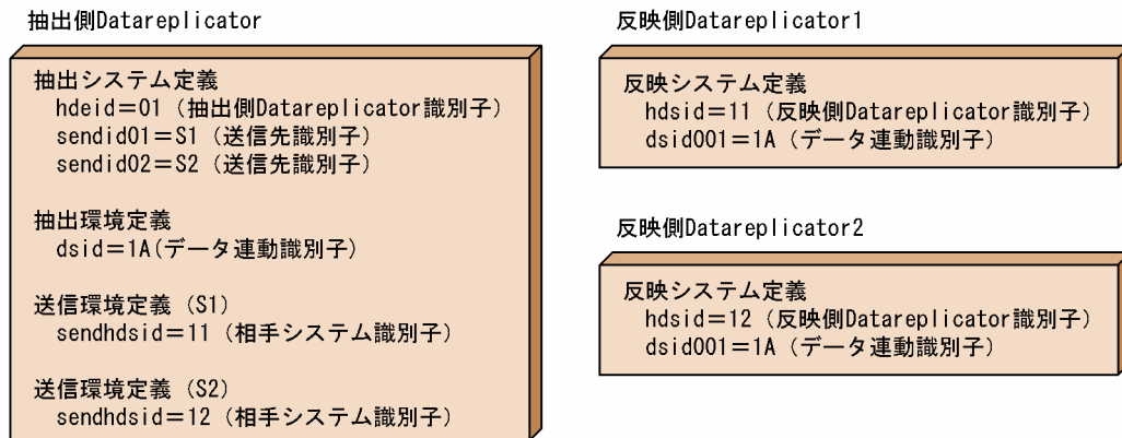
図 4-18 識別子の定義例
