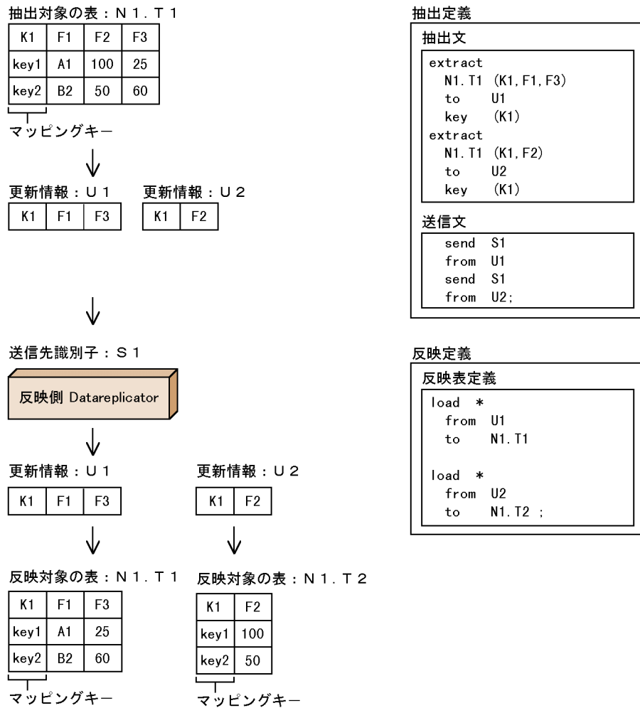
図 4-9 抽出側で 1 表を n 表に分割して抽出して一つの反映側システムで反映する例
