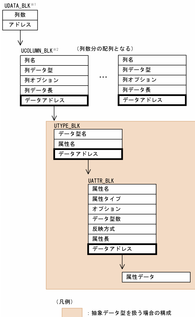
図 8-5 抽象データ型の列データ構造
