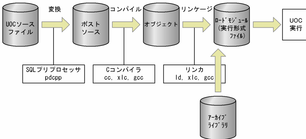
図 8-3 反映情報編集 UOC の実行手順
