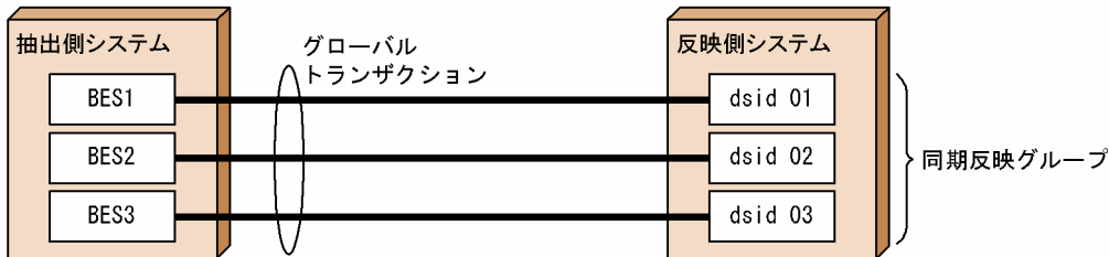
図 3-36 反映トランザクション同期機能を使用する場合の構成例
