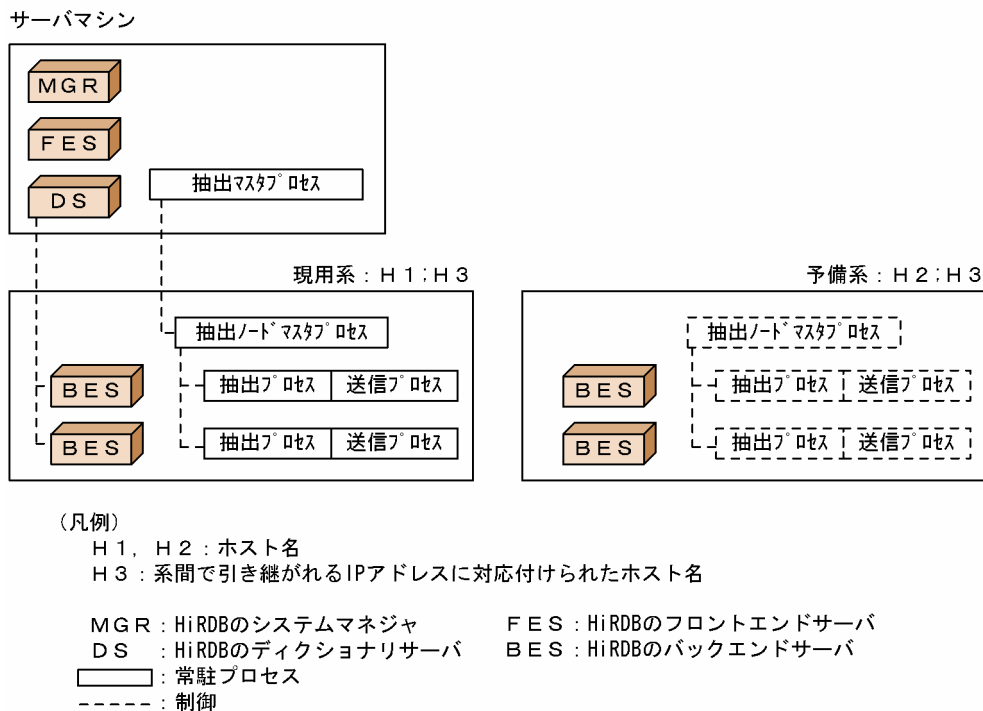
図 6-29 抽出側システムのサーバと主要なプロセスの関係
