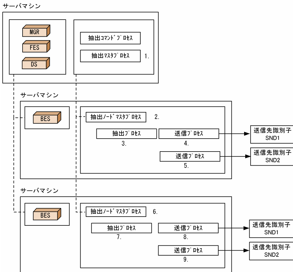
図 7-1 抽出側 HiRDB がパラレルサーバの場合の、hdestart コマンドによる動作
