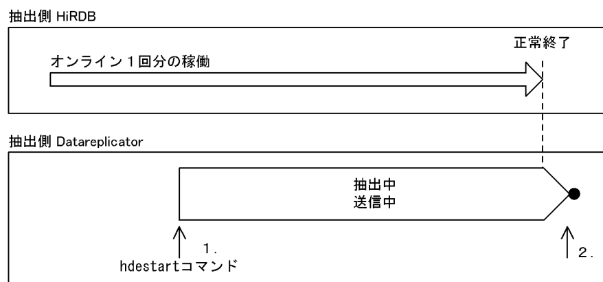
図 6-5 抽出側 Datareplicator の同時開始の運用例
