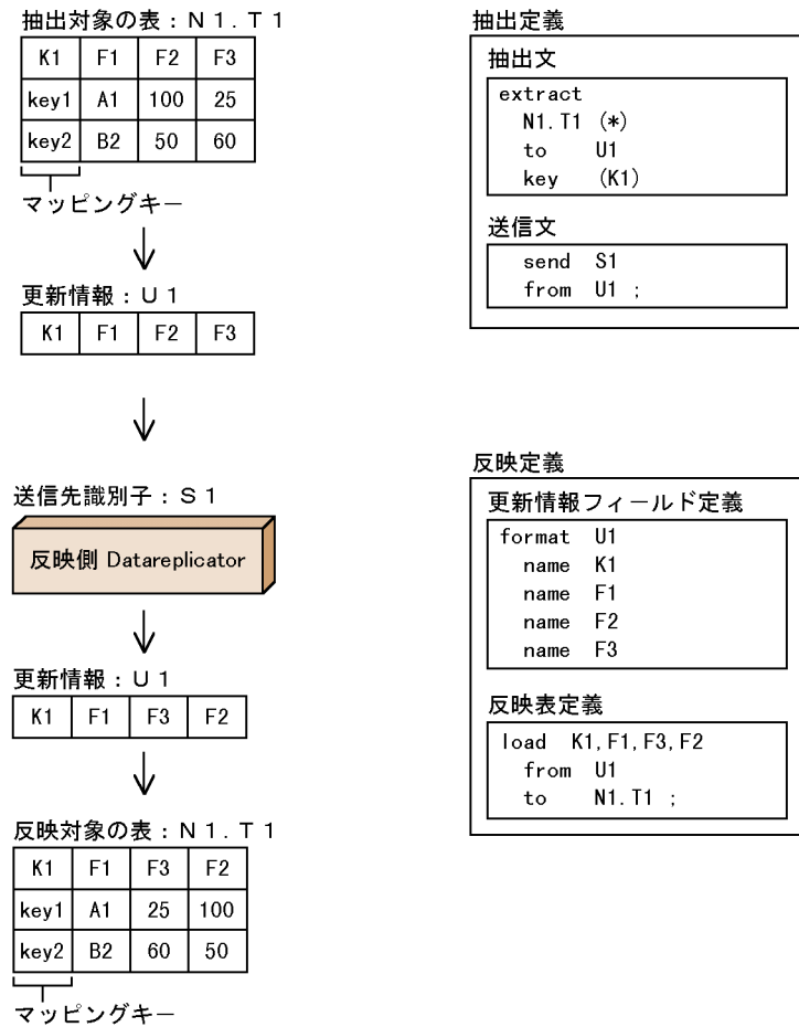
図 4-5 反映側で列を並べ替えて反映する例
