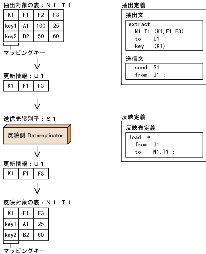
図 4-6 抽出側で列の一部を選択して抽出して反映する例
