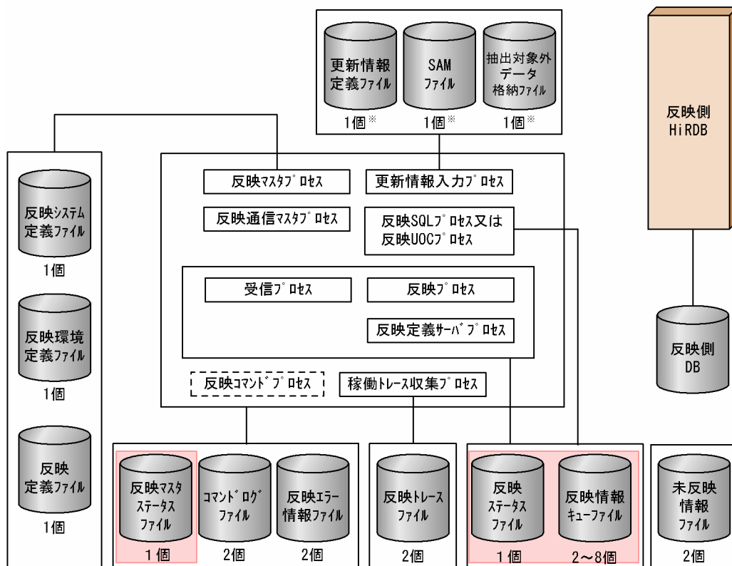
図 4-40 反映側 Datareplicator のファイル構成
