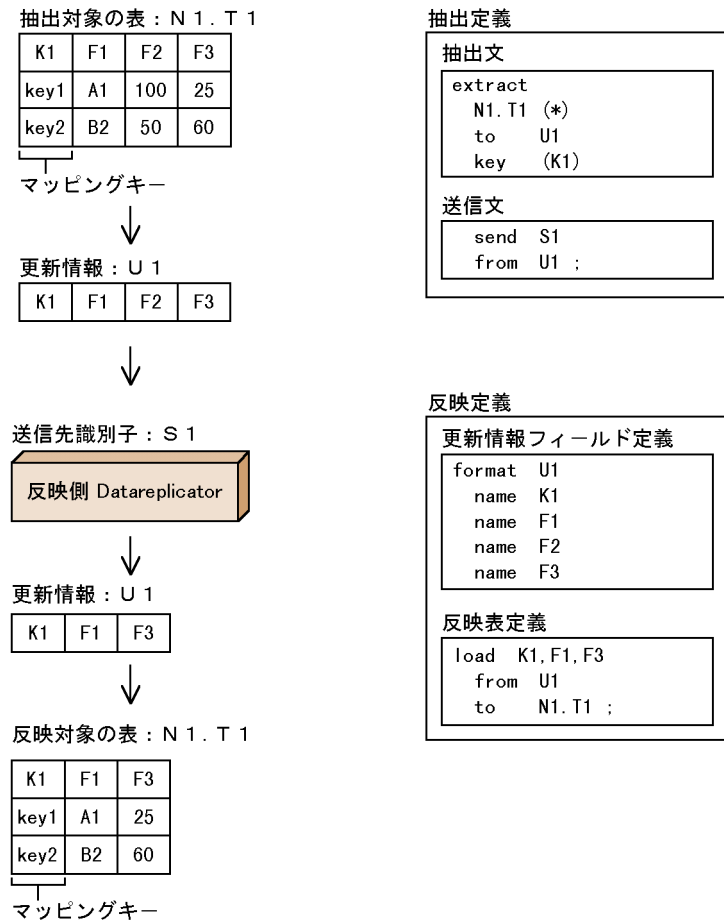
図 4-7 反映側で列の一部を選択して反映する例
