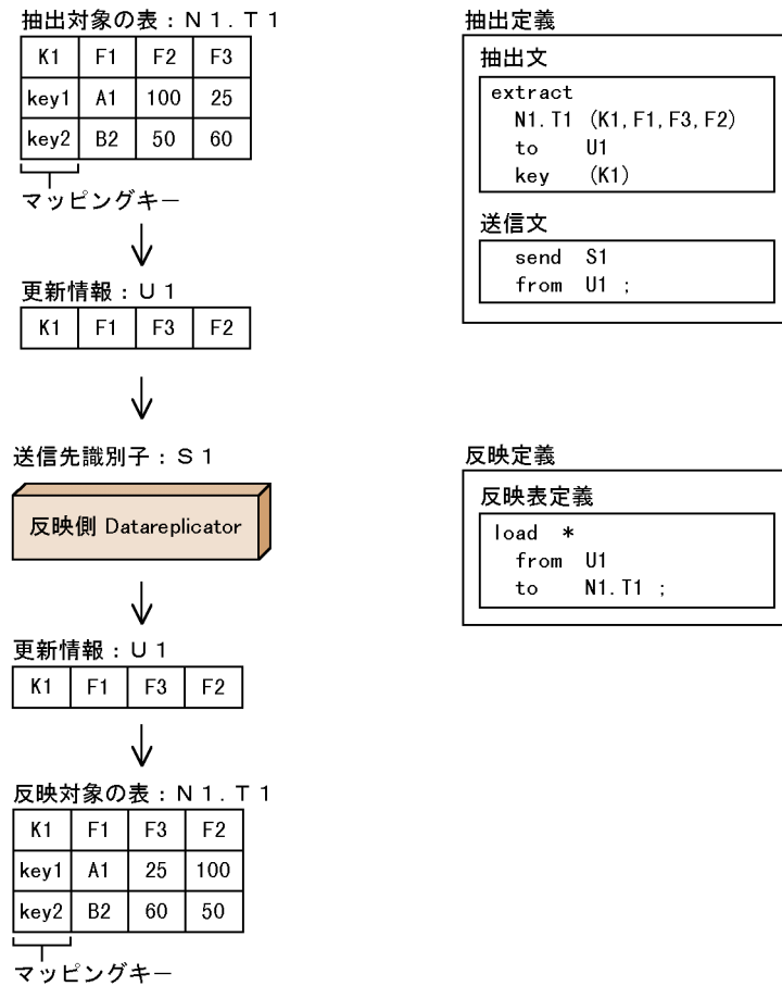
図 4-4 抽出側で列を並べ替えて抽出して反映する例
