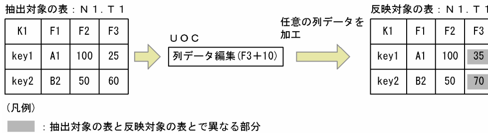
図 3-10 UOC で列を加工して反映する例
