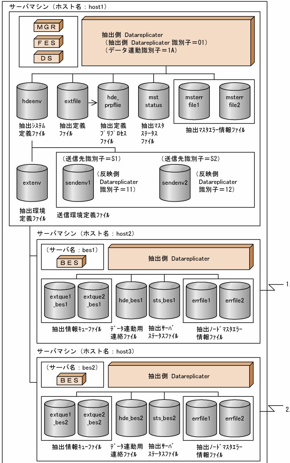
図 5-13 システムの対応とファイルの構成例 1
