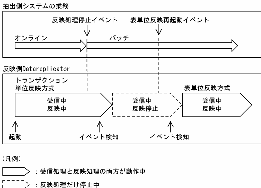
図 4-46 反映処理方式の切り替えの設計例
