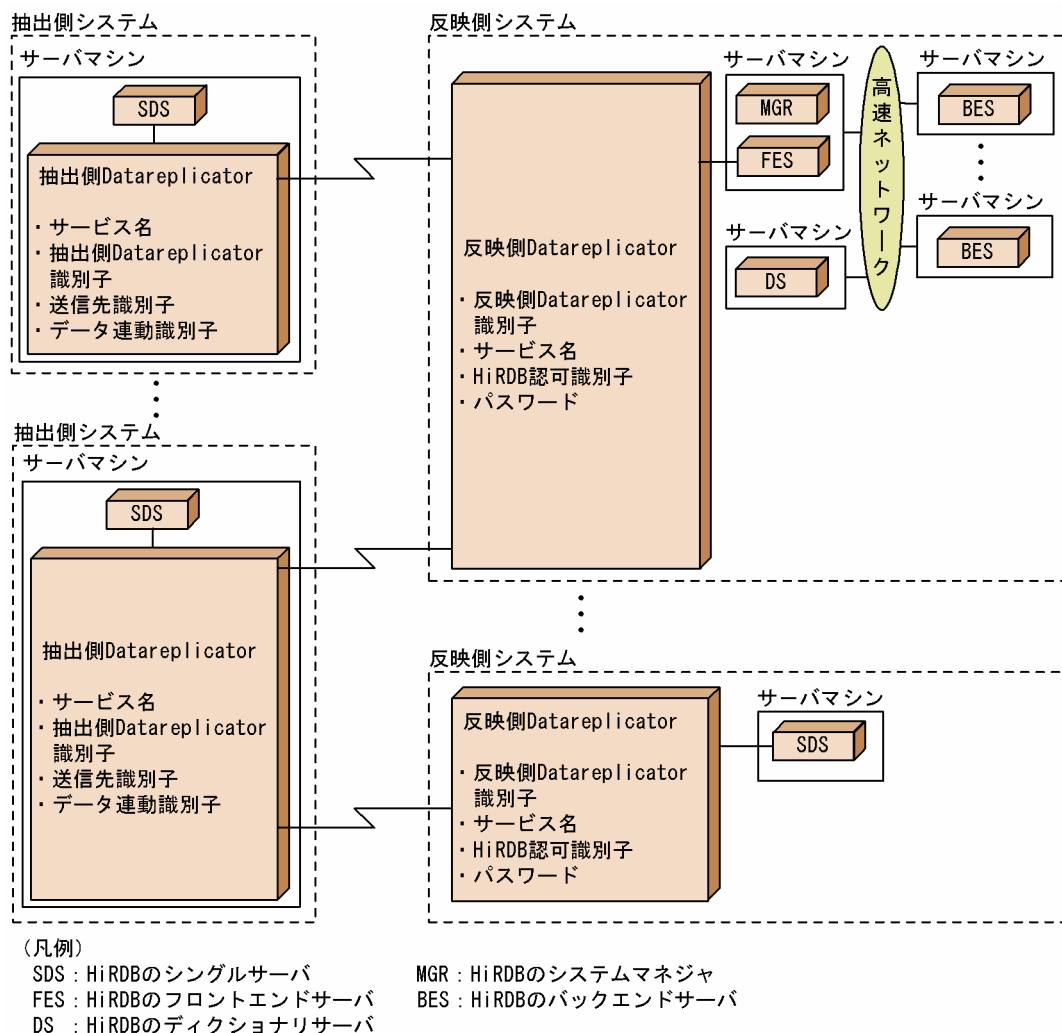
図 4-16 HiRDB から HiRDB へデータ連動する場合の、抽出側システムと反映側システムとの対応（抽出側 HiRDB がシングルサーバの場合）
