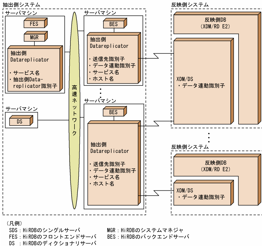
図 4-20 HiRDB からメインフレーム側 DB へデータ連動する場合の、抽出側システムと反映側システムとの対応（抽出側 HiRDB がパラレルサーバの場合）
