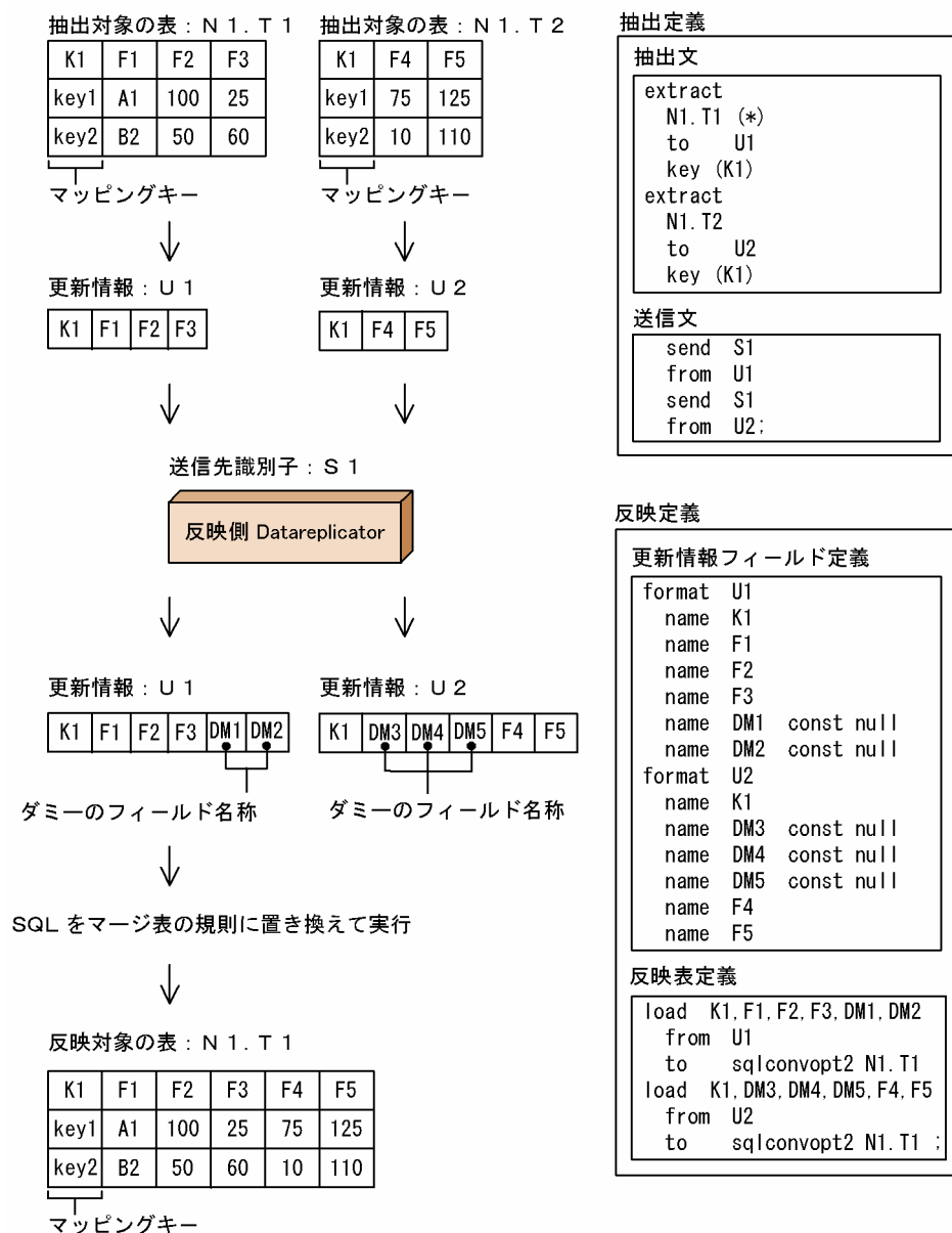
図 4-12 マージ表を使って、複数の抽出対象表を反映側で一つにまとめて一つの表に反映する例
