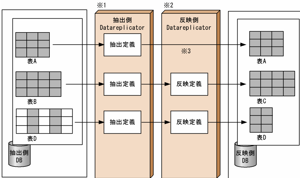
図 1-8 リレーショナル型からリレーショナル型へのデータ連動の概念
