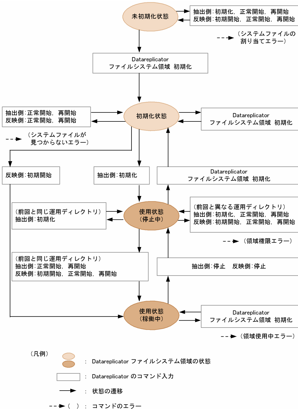
図 3-28 Datareplicator ファイルシステム領域の状態遷移
