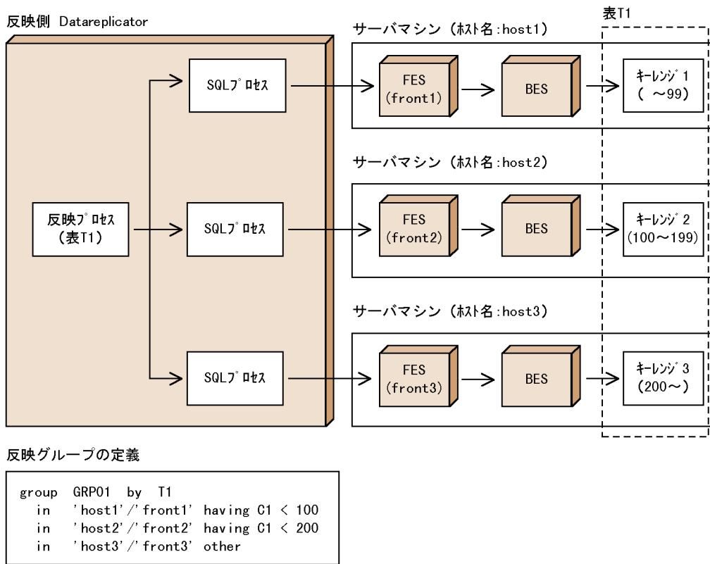
図 5-30 反映グループ定義の例 (キーレンジ単位分割方式)
