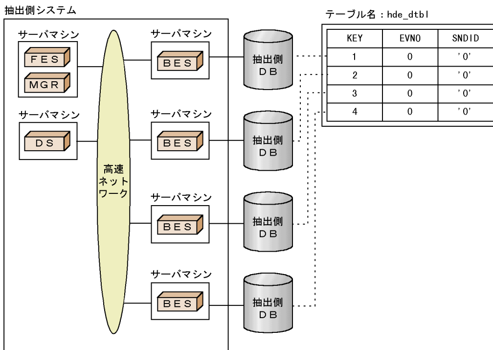
図 4-39 抽出側 HiRDB がパラレルサーバの場合のイベント制御用テーブルの例
