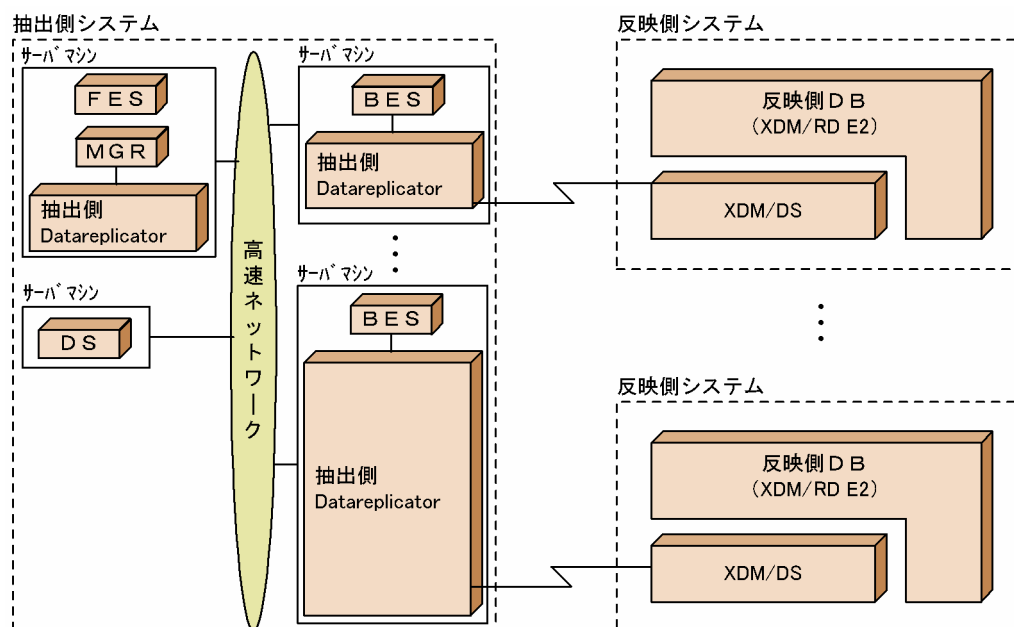
図 1-14 HiRDB からメインフレーム側 DB へデータ連動する場合の抽出側システムと反映側システムの形態
