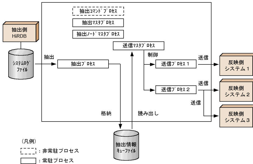
図 3-17 送信プロセスの制御の概要
