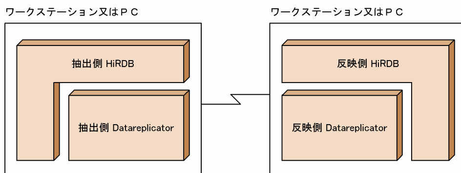
図 1-10 HiRDB から HiRDB へデータ連動する場合のソフトウェア構成
