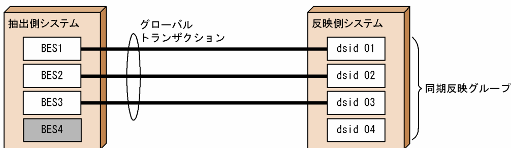
図 3-37 同期を待ち続ける構成の例
