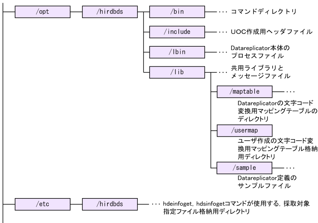
図 2-1 Datareplicator に関連するディレクトリとファイル
