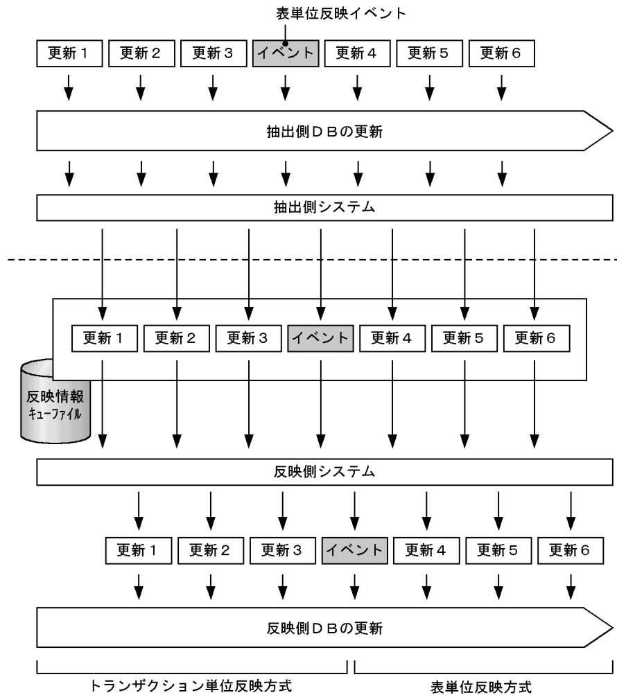
図 3-43 イベント機能の動作例
