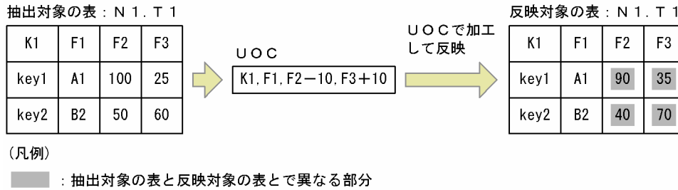
図 3-9 UOC で更新情報を加工して反映する例
