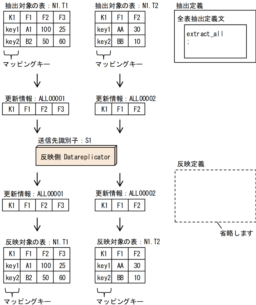
図 4-3 すべての表を抽出対象とし、すべて同一の表に反映する例
