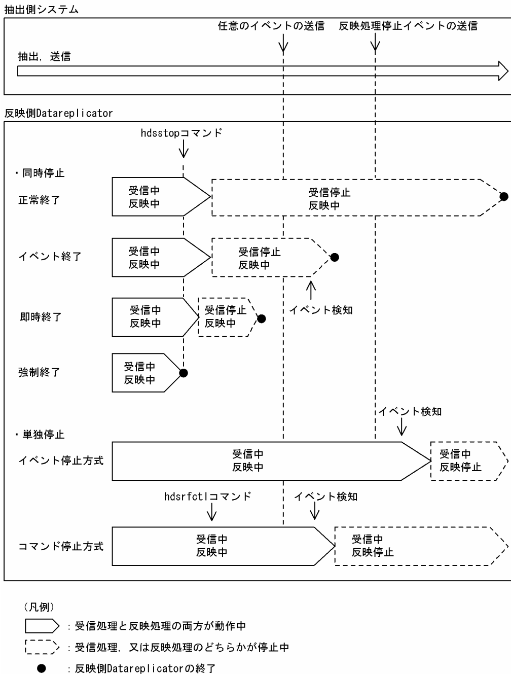
図 4-45 反映処理の停止方式と停止タイミングの関係
