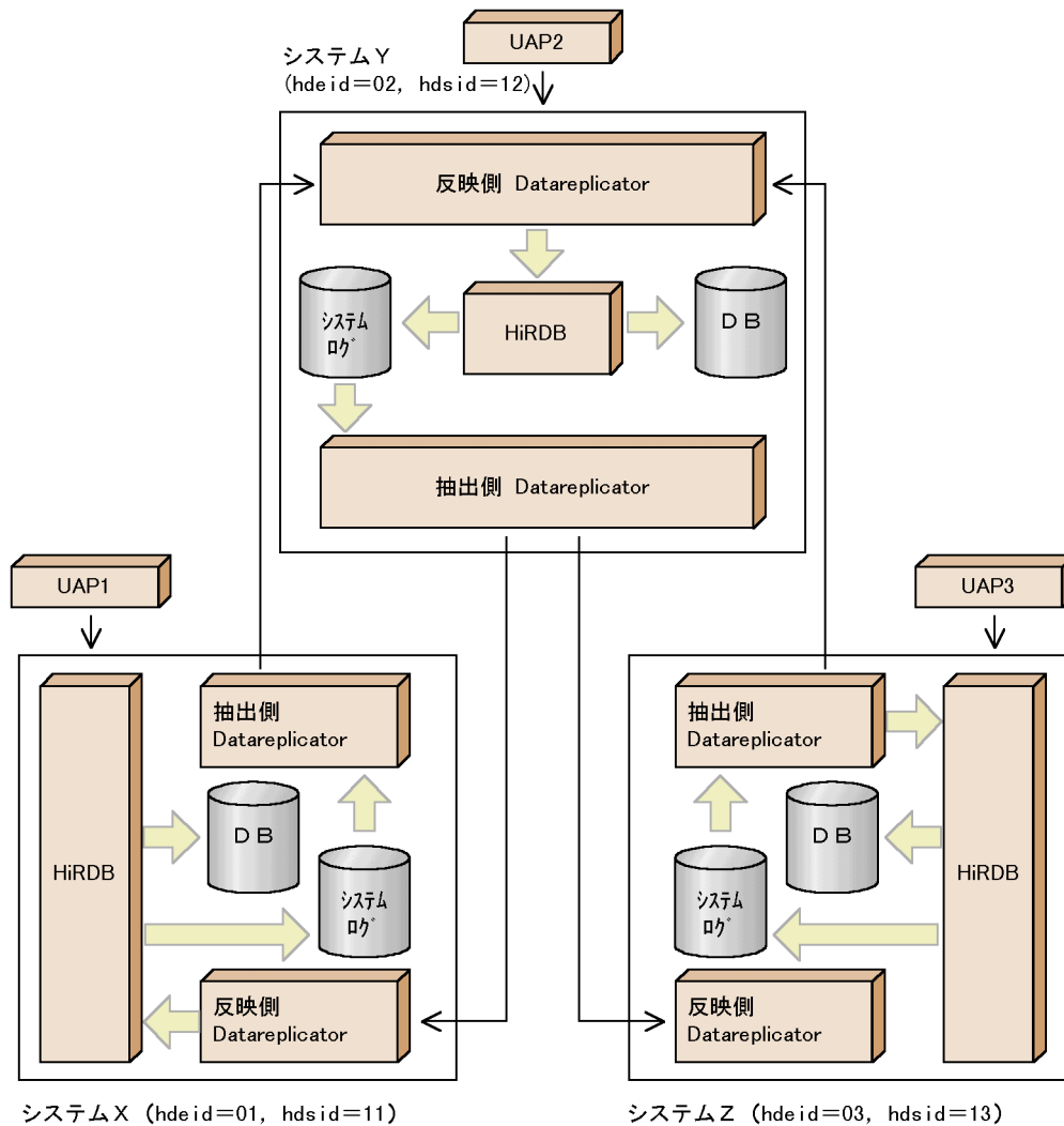
図 4-28 ループバックを抑止する双方向更新システムの形態の例
