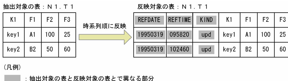
図 3-11 更新情報のほかに反映日付、反映時間などを時系列順に取得する例
