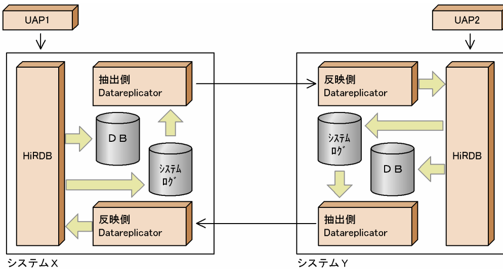
図 4-24 双方向更新システムの例
