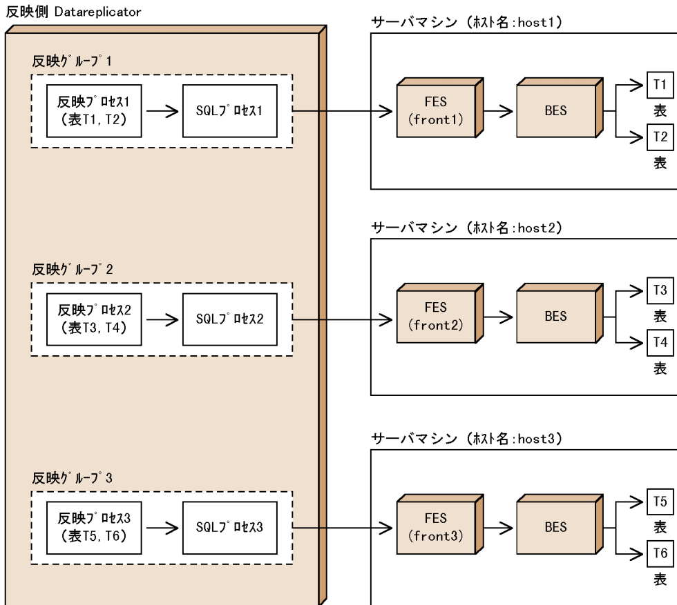
図 4-41 表単位分割方式でマルチ FES 機能を使う例
