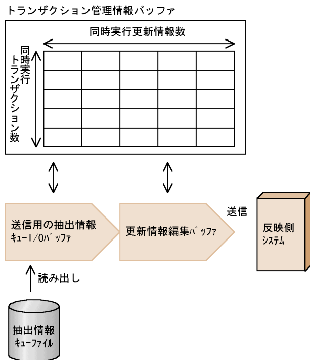
図 4-33 送信方法の概要
