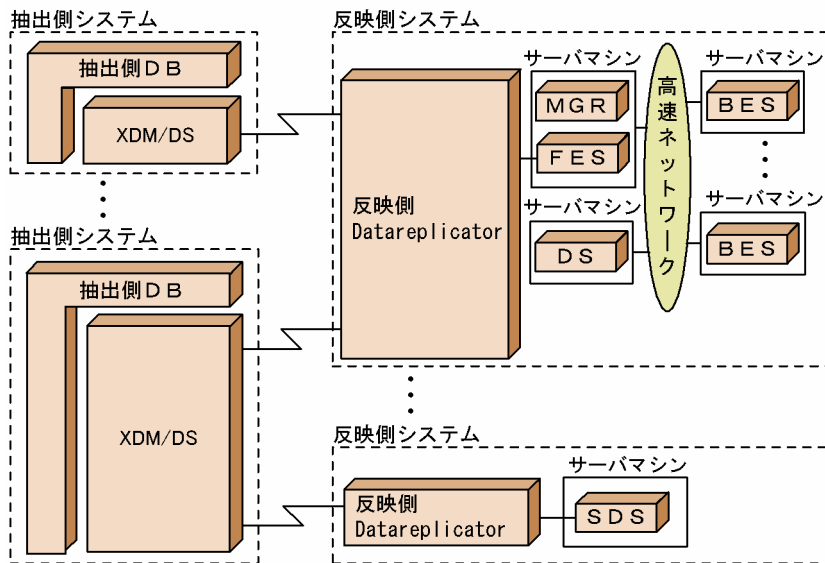
図 1-16 メインフレーム側 DB から HiRDB ヘデータ連動する場合の抽出側システムと反映側システムの形態
