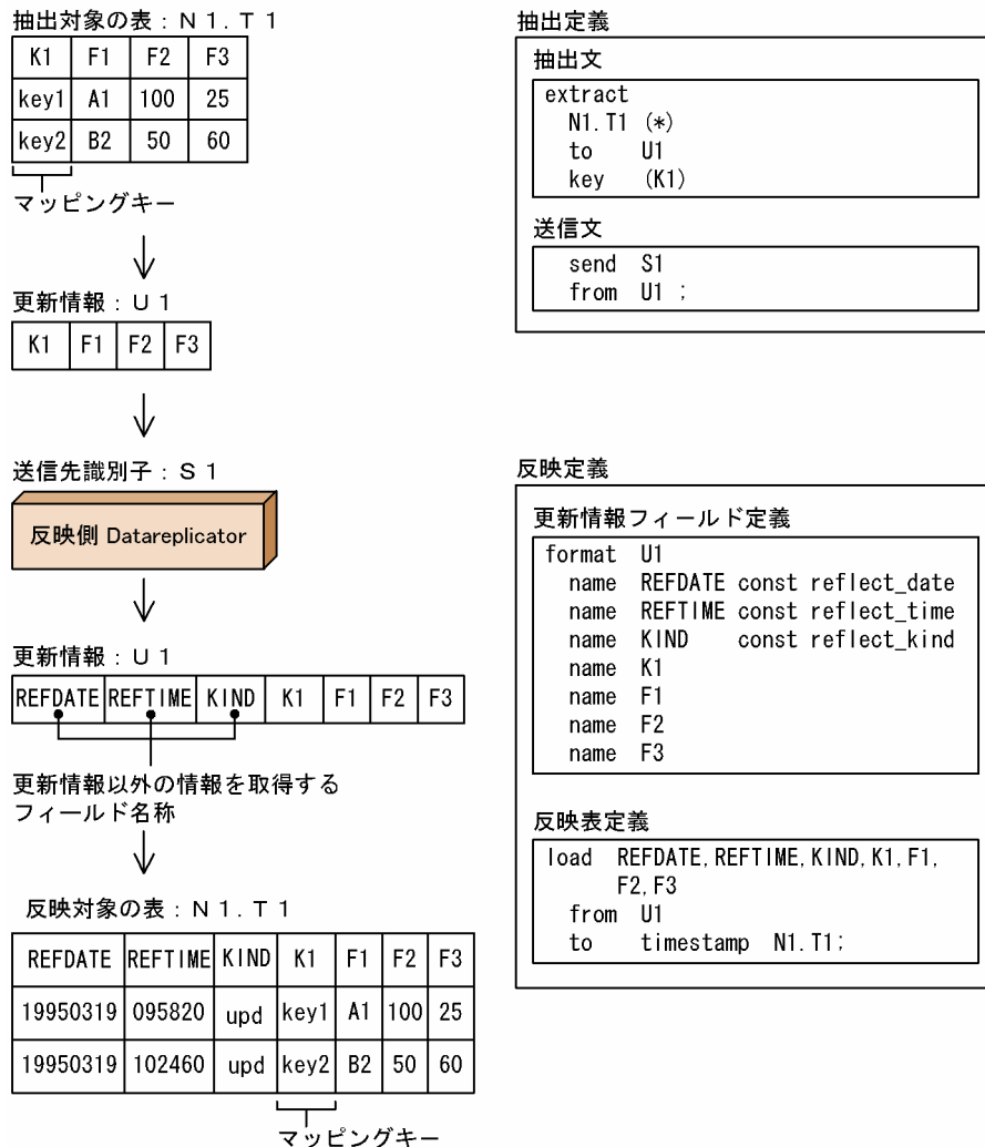
図 4-15 更新情報のほかに反映日付、反映時間などを時系列順に取得する例
