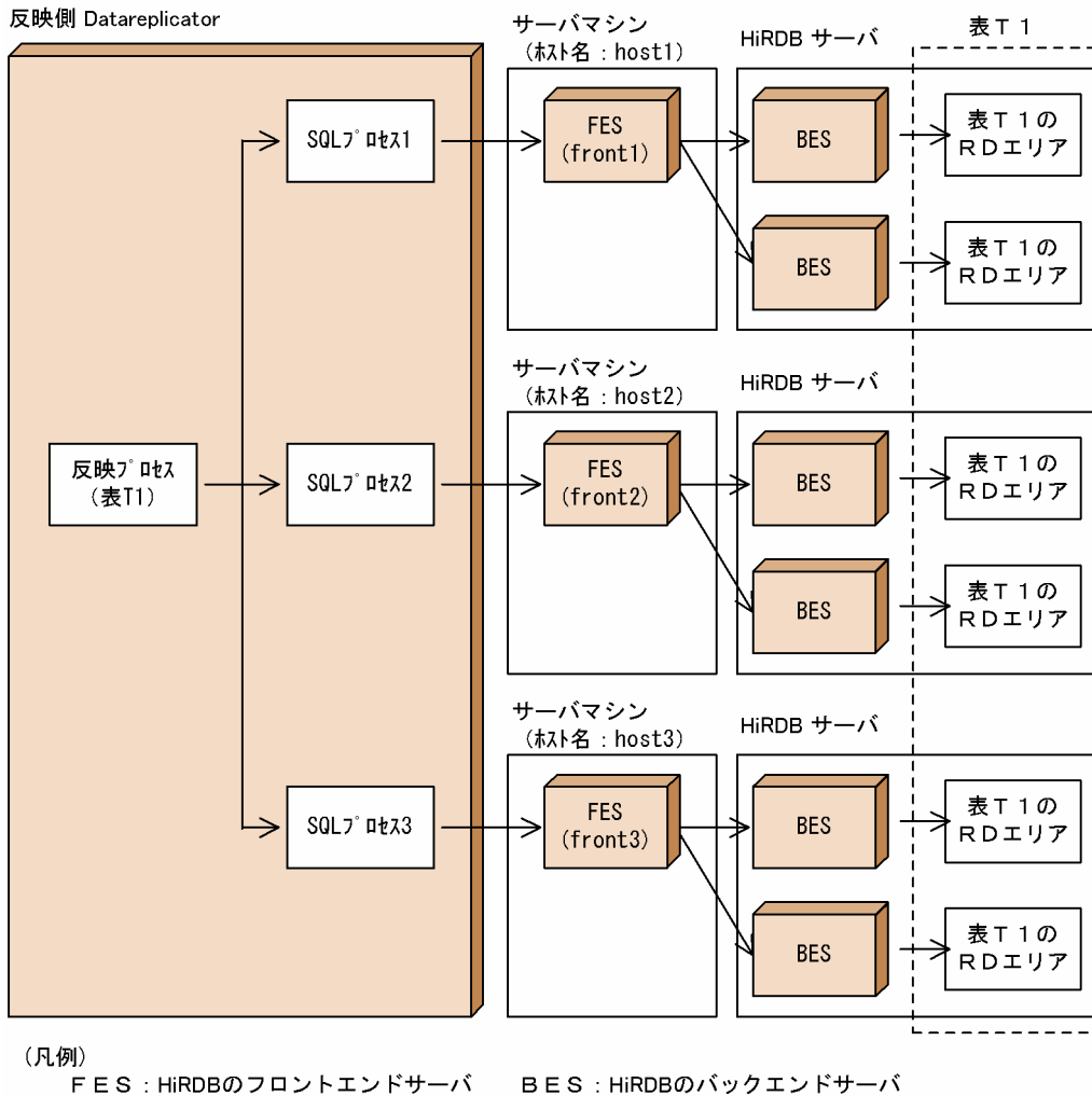
図 4-43 ハッシュ分割方式でマルチ FES 機能を使う例
