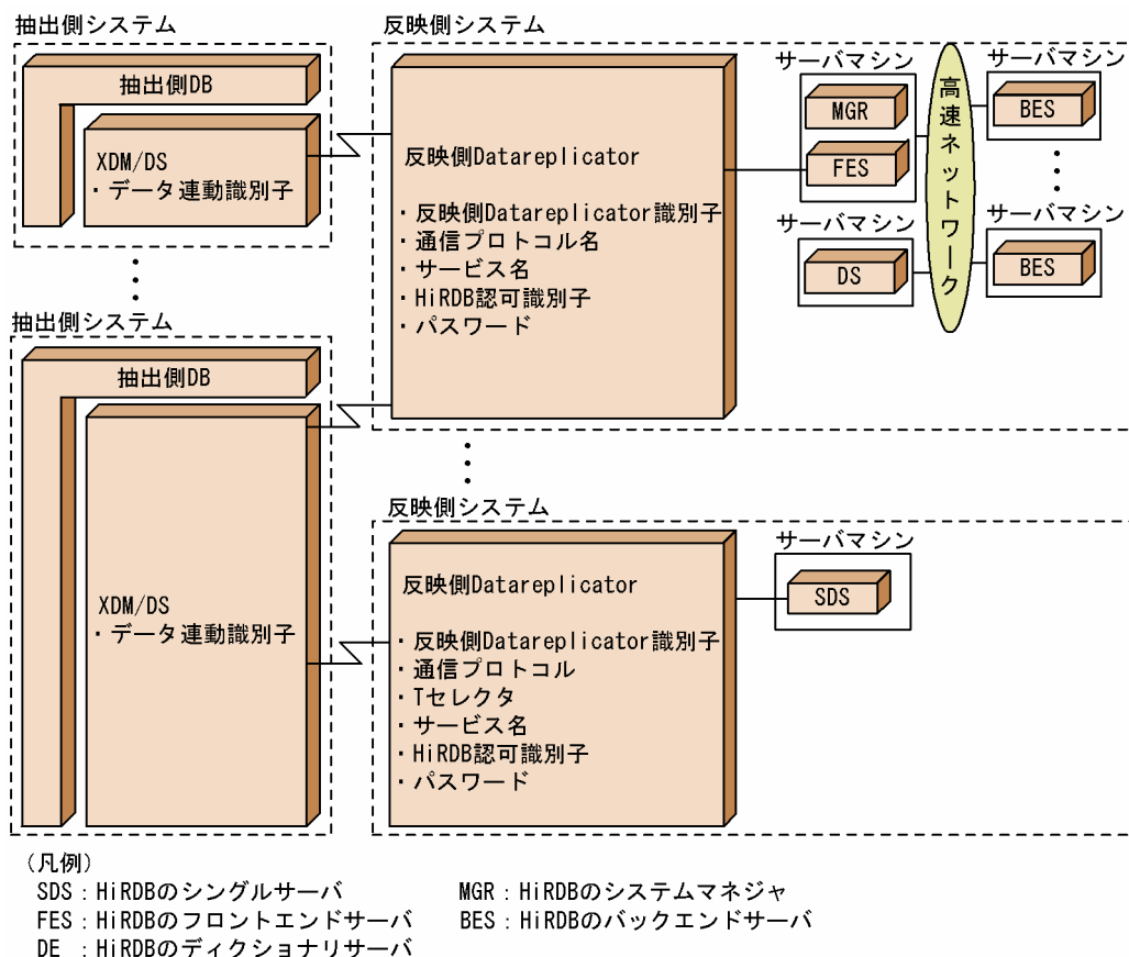
図 4-21 メインフレーム側 DB から HiRDB へデータ連動する場合の、抽出側システムと反映側システムとの対応
