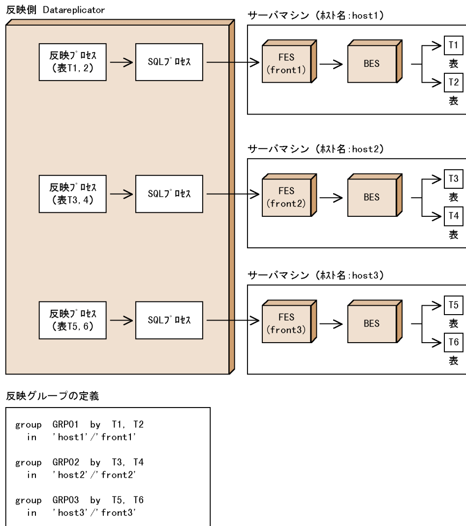
図 5-29 反映グループ定義の例 (表単位分割方式)
