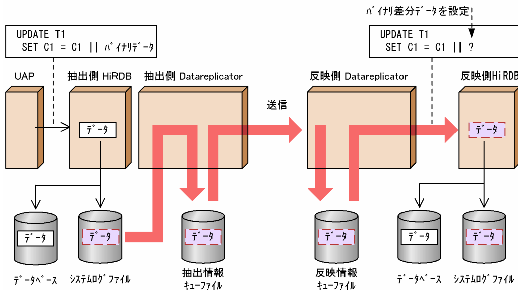
図 3-18 連結演算の更新データのデータ連動
