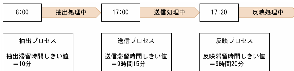
図 5-9 送信処理を遅らせて開始する場合の運用例
