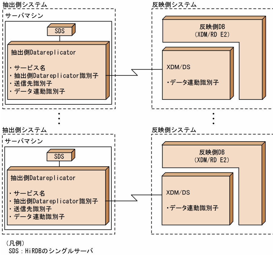
図 4-19 HiRDB からメインフレーム側 DB へデータ連動する場合の、抽出側システムと反映側システムとの対応（抽出側 HiRDB がシングルサーバの場合）
