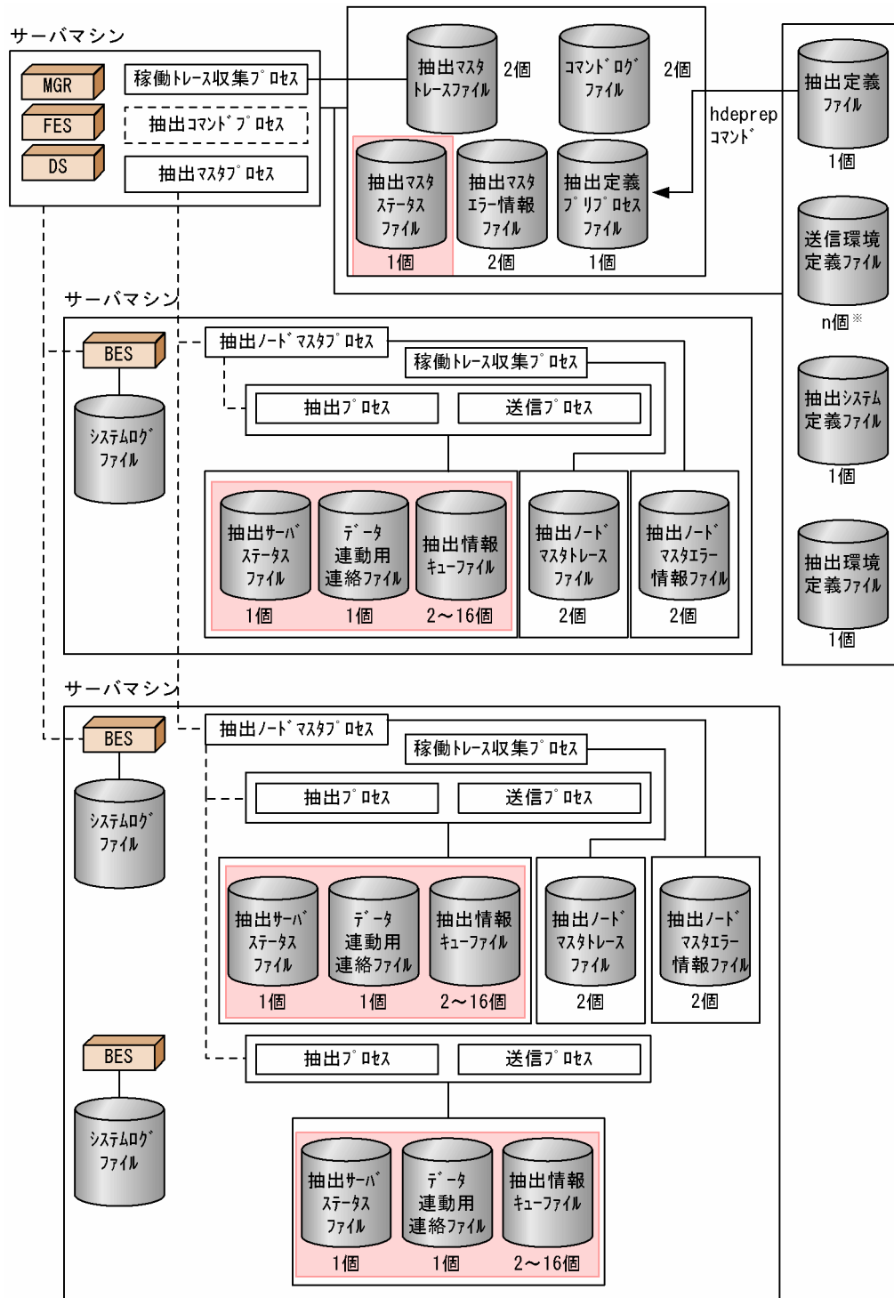
図 4-31 抽出側 HiRDB がパラレルサーバの場合の抽出側 Datareplicator のファイル構成
