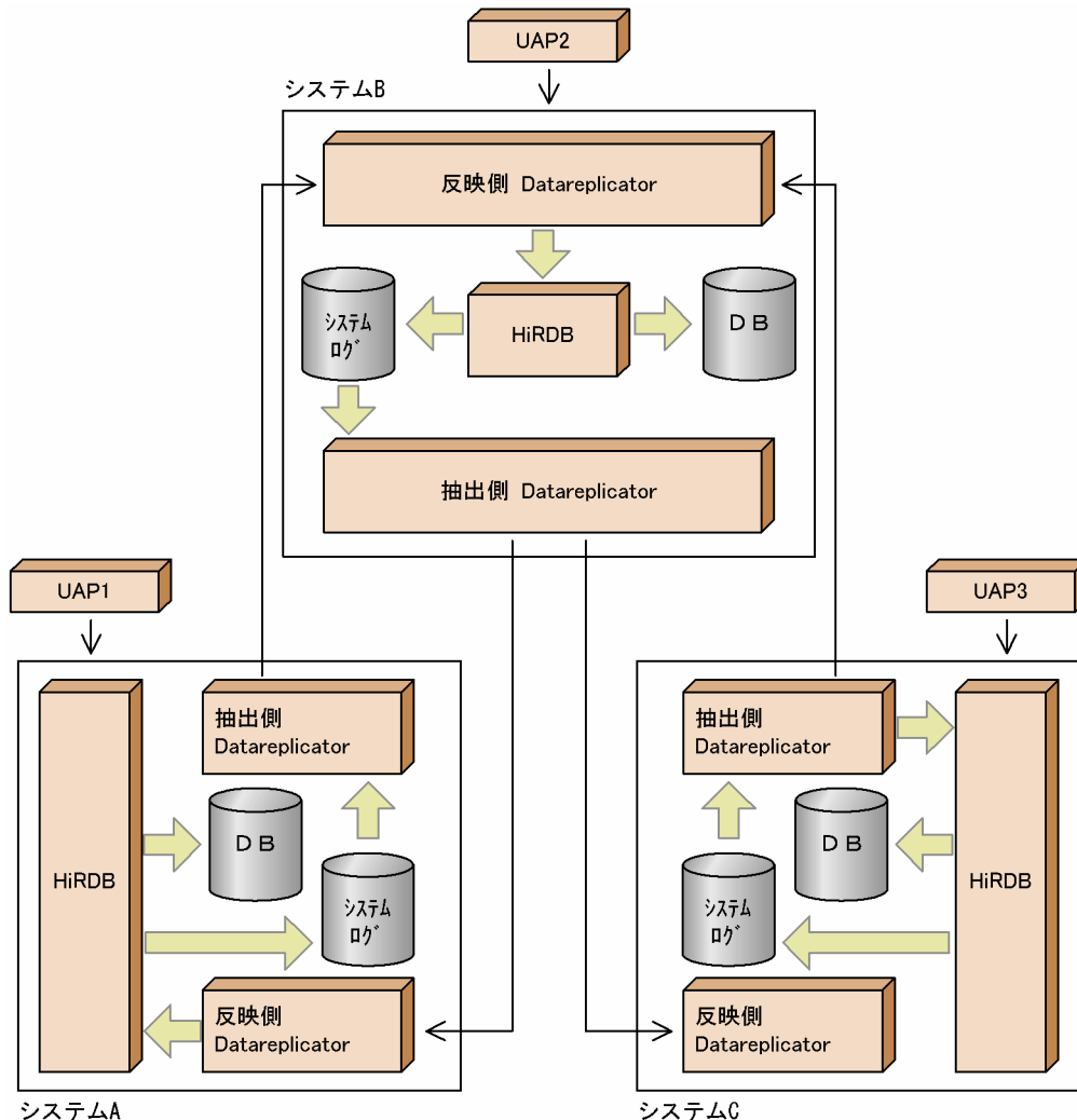
図 4-27 複数のシステムを一つの線をつないだシステムの例
