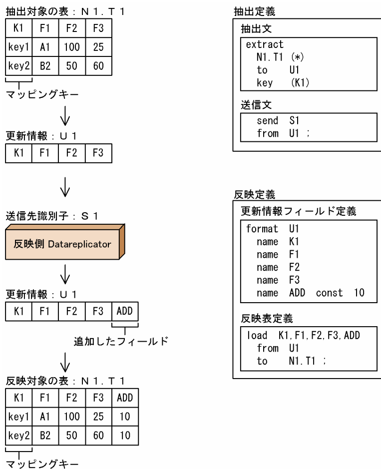
図 4-8 反映側で固定値の列を追加して反映する例
