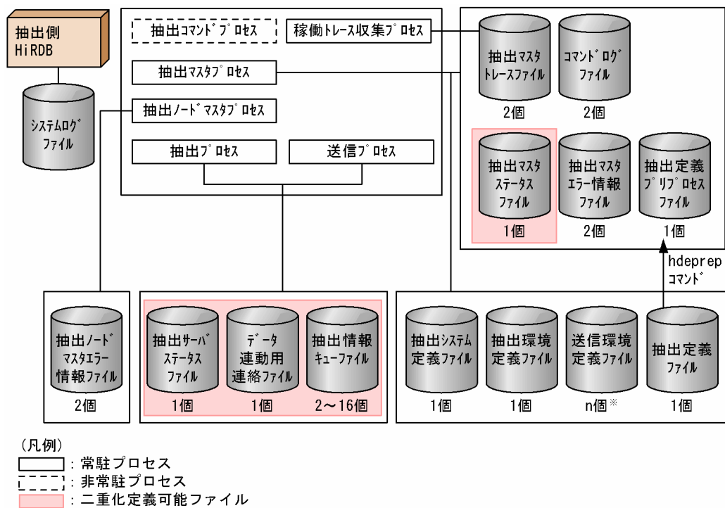
図 4-30 抽出側 HiRDB がシングルサーバの場合の抽出側 Datareplicator のファイル構成
