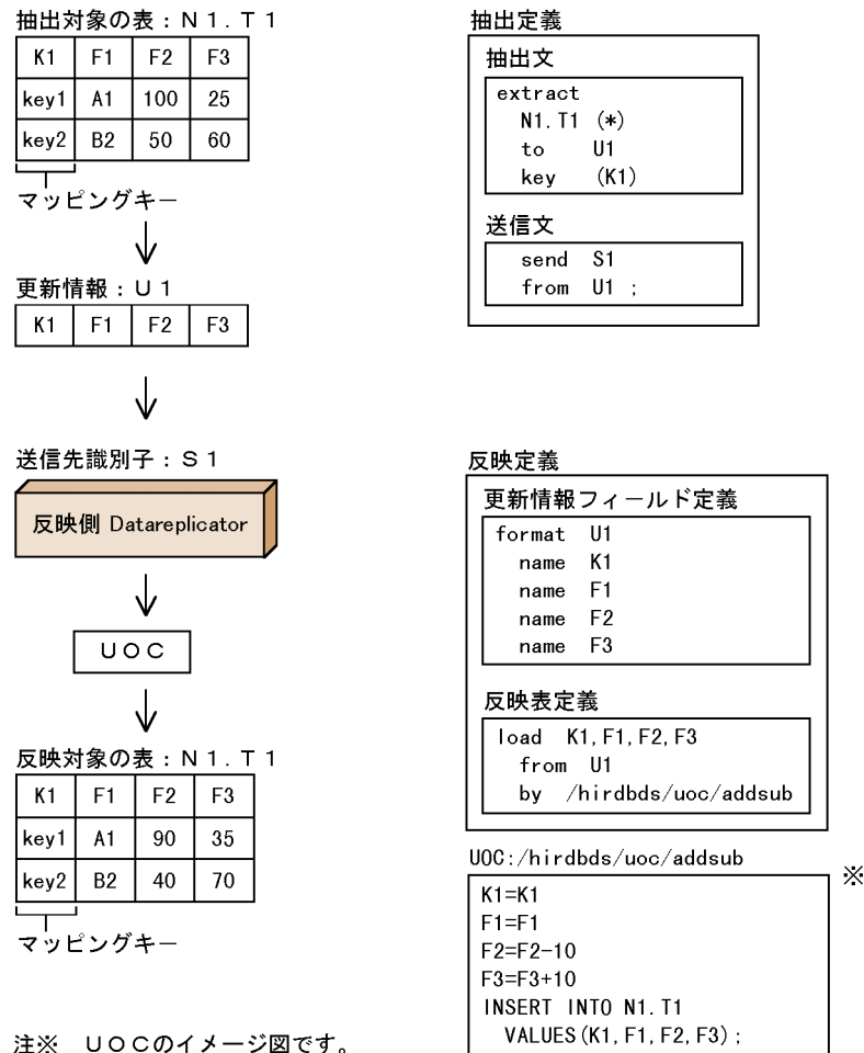
図 4-14 反映側の UOC を使って任意に加工して反映する例
