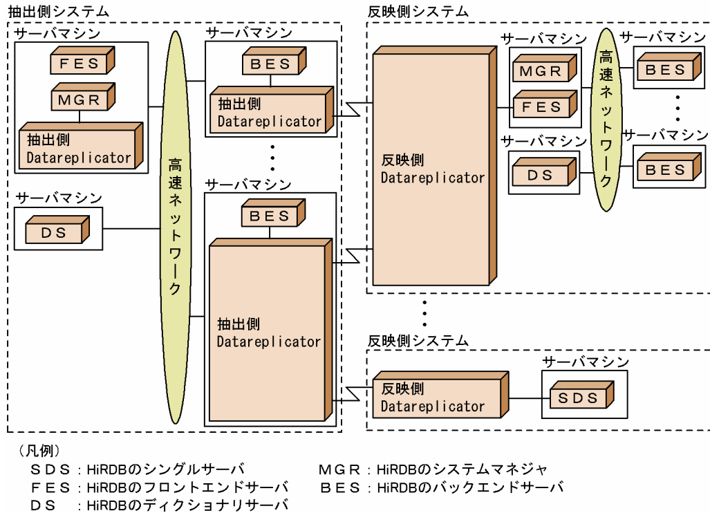
図 1-12 HiRDB から HiRDB へデータ連動する場合の抽出側システムと反映側システムの形態 (抽出側 HiRDB がパラレルサーバの場合)
