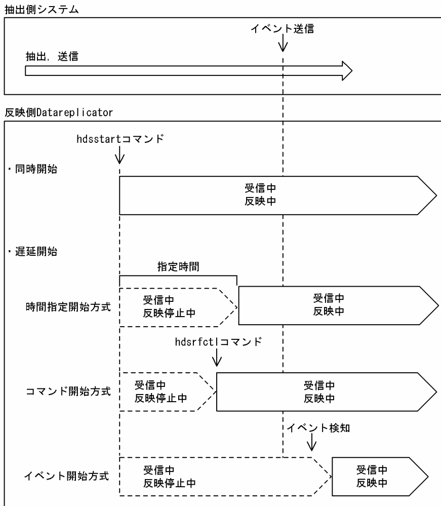
図 4-44 反映処理の開始方式と開始タイミングの関係
