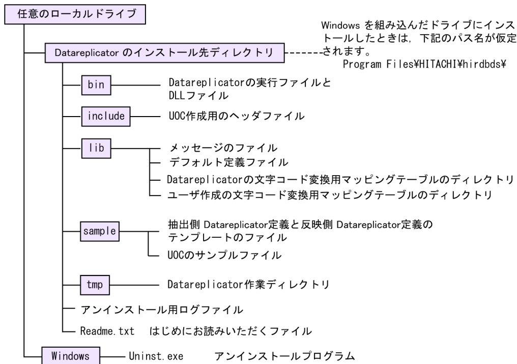
図 2-4 Datareplicator に関連するディレクトリとファイル
