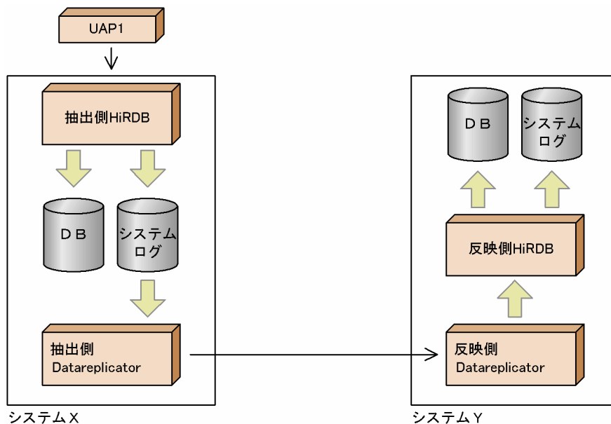
図 4-23 単一方向更新システムの例
