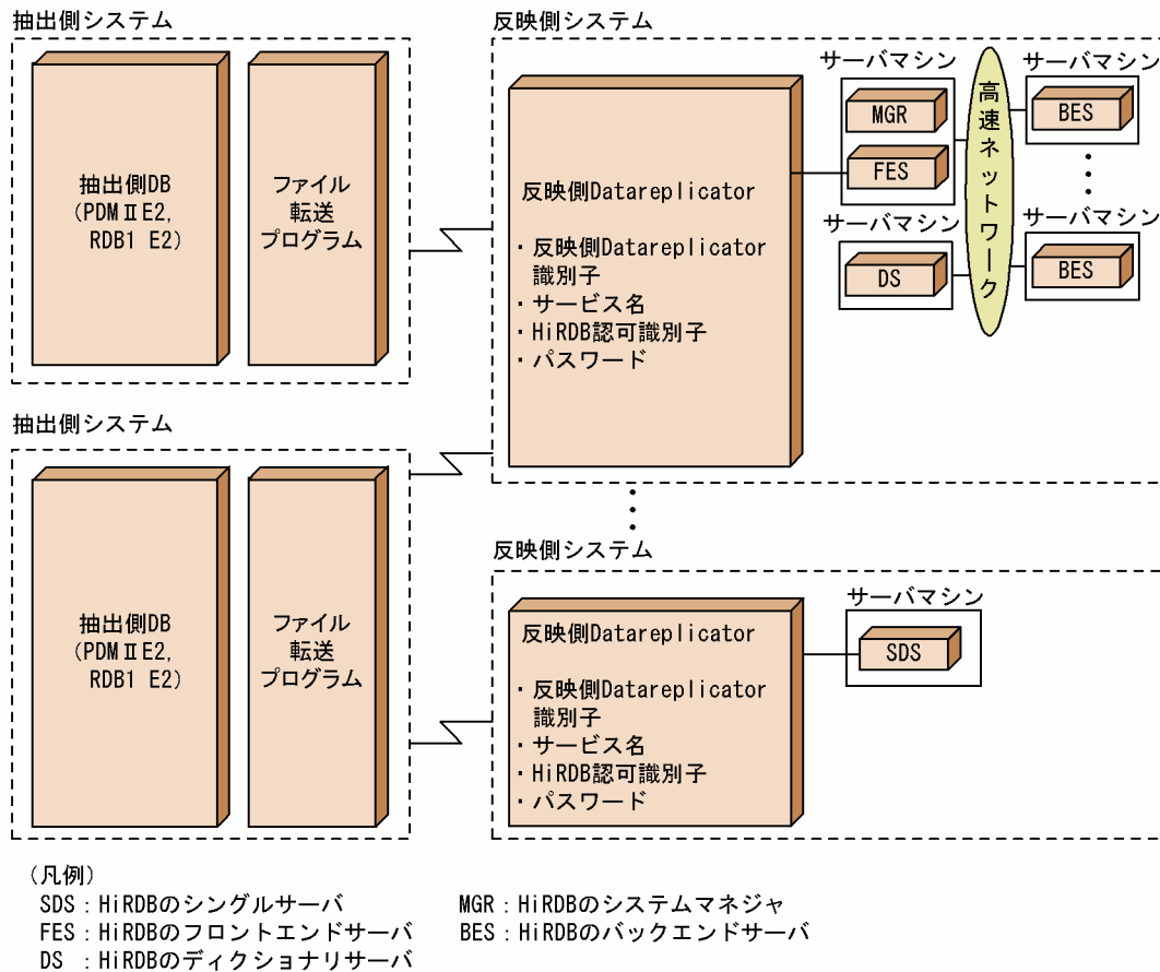
図 4-22 メインフレーム側 DB (PDMII E2, RDB1 E2) から HiRDB へデータ連動する場合の、抽出側システムと反映側システムとの対応
