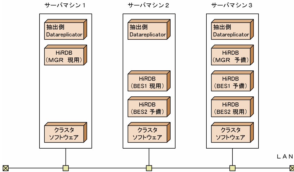
図 6-31 抽出側 HiRDB がパラレルサーバで相互系切り替えの形態の例
