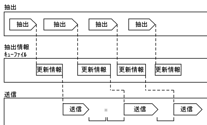
図 4-34 抽出処理の送信間隔の概要
