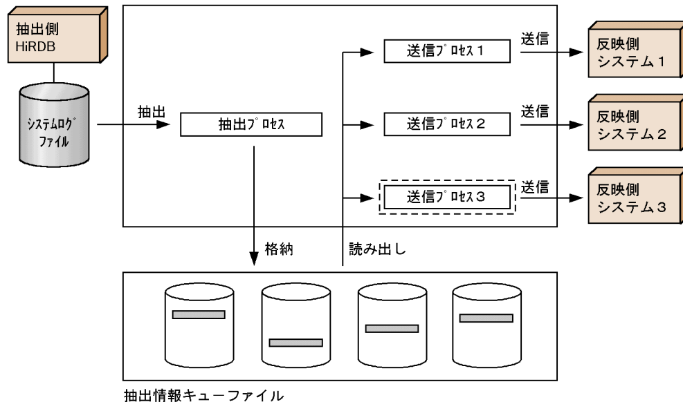
図 4-35 送信処理の縮退の概念
