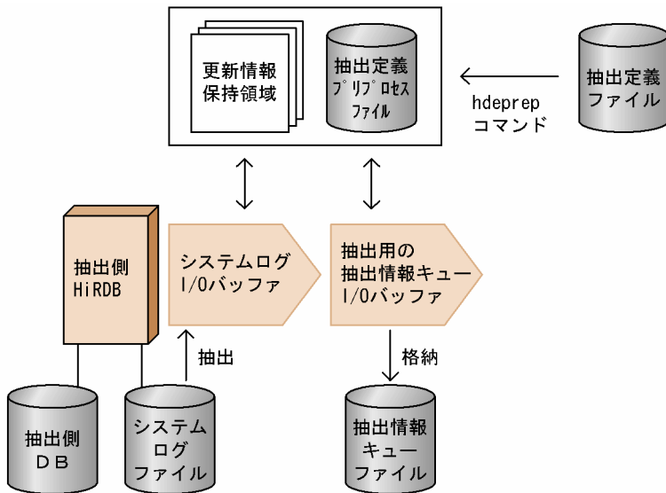
図 4-32 抽出方法の概要
