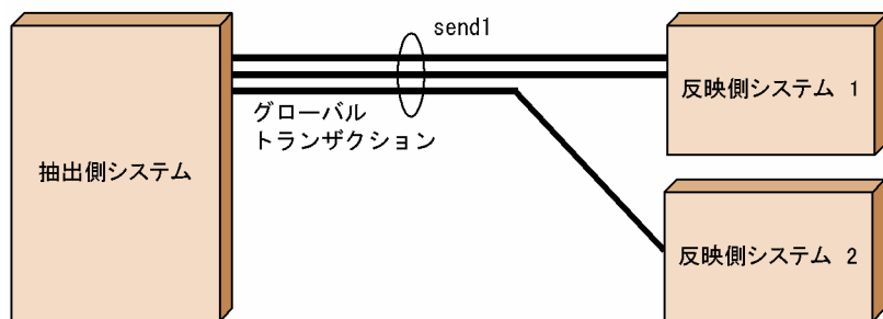
図 3-40 同期できない構成の例
