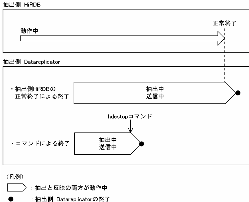
図 4-37 抽出処理の停止方式と停止タイミングの関係
