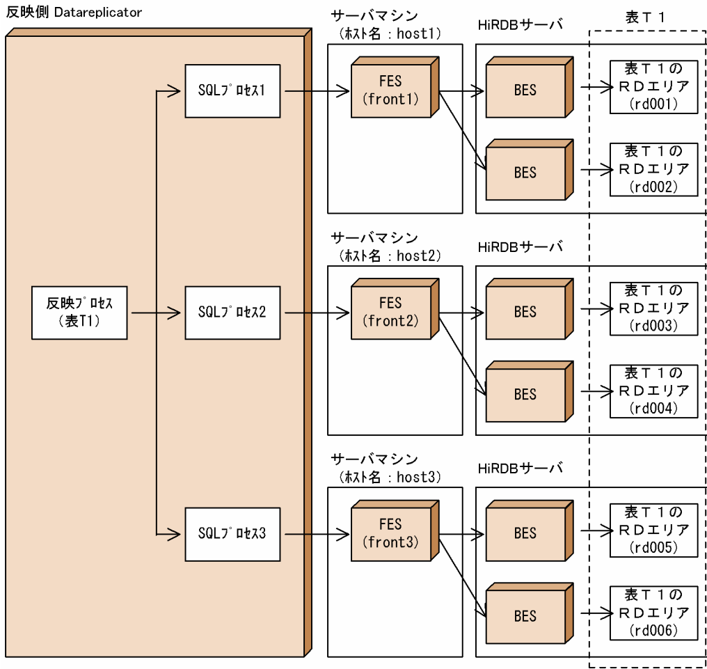
図 5-32 反映グループ定義の例 (ハッシュ分割方式で FES を指定する場合)
