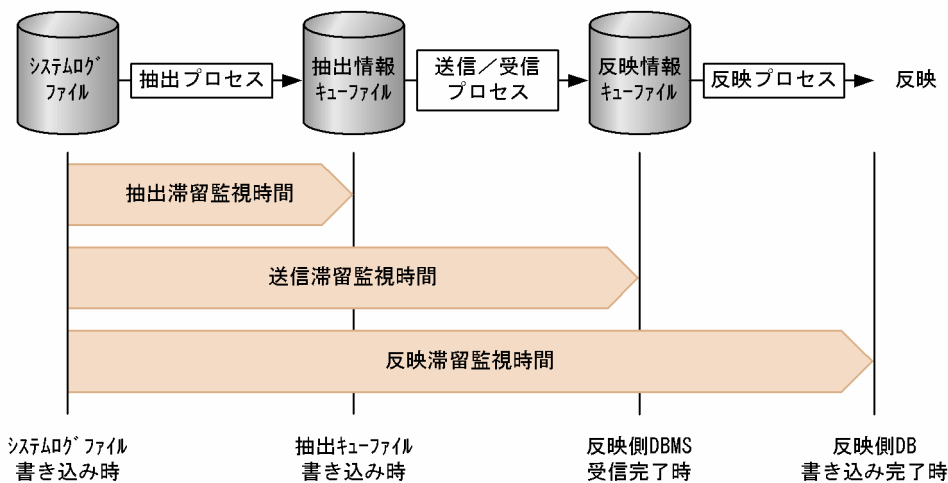
図 3-32 滞留監視機能の概念
