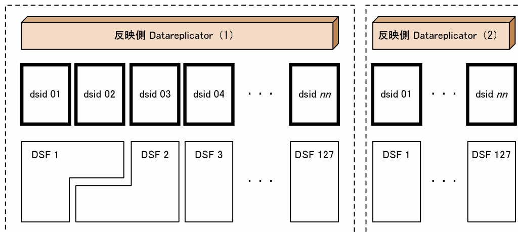
図 3-31 反映側システムでの Datareplicator ファイルシステム領域への格納例
