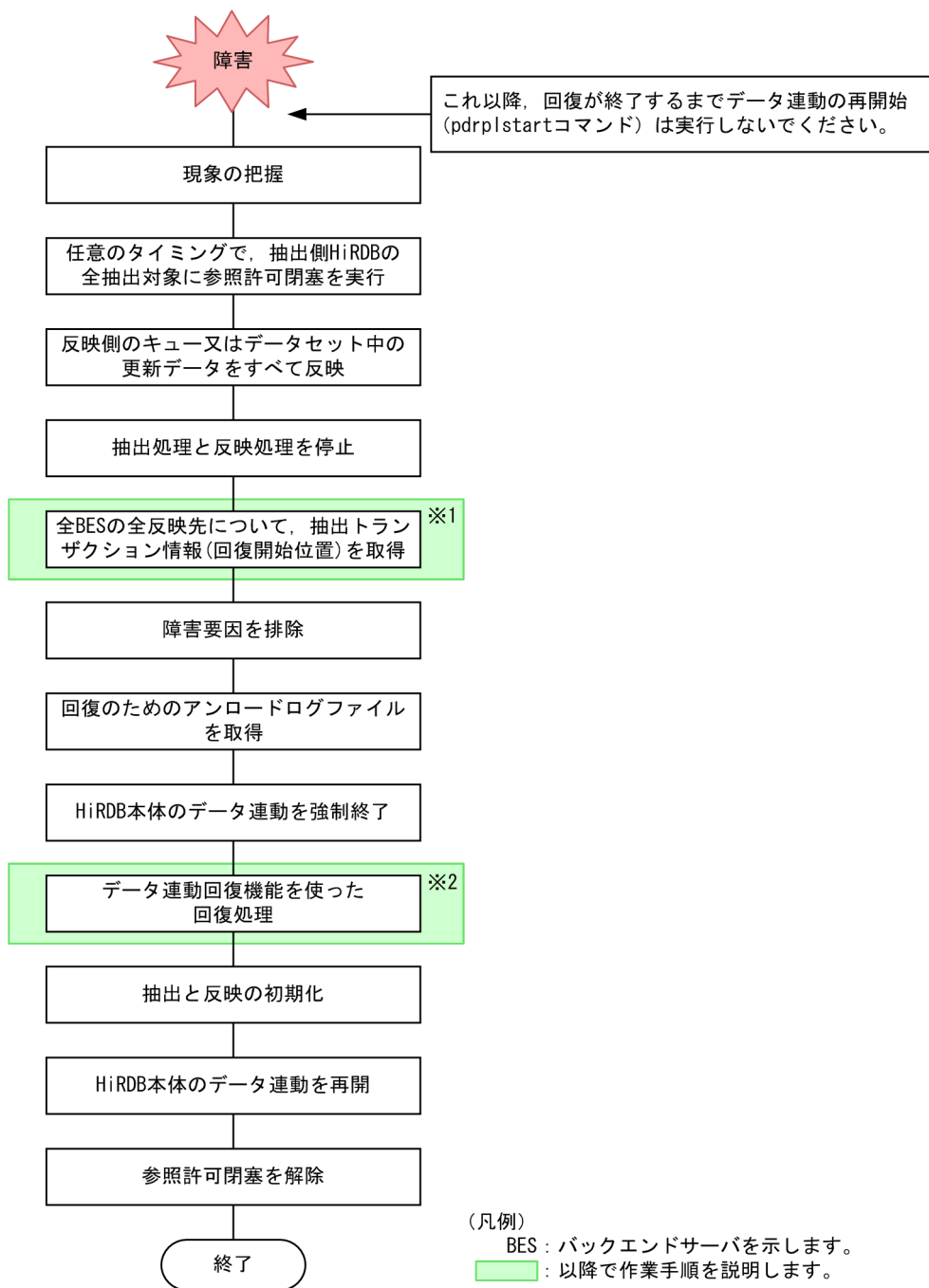
図 9-8 アンロードログファイルによる回復手順の概要
