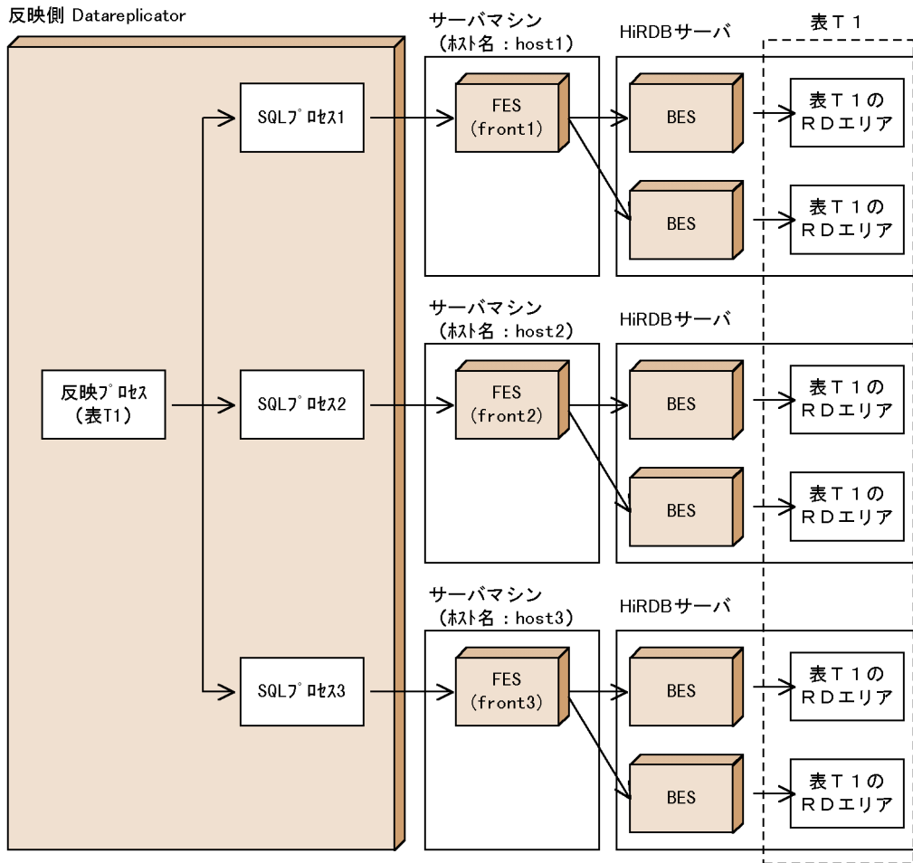
図 5-31 反映グループ定義の例 (ハッシュ分割方式)
