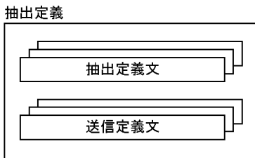
図 5-7 抽出定義の構造
