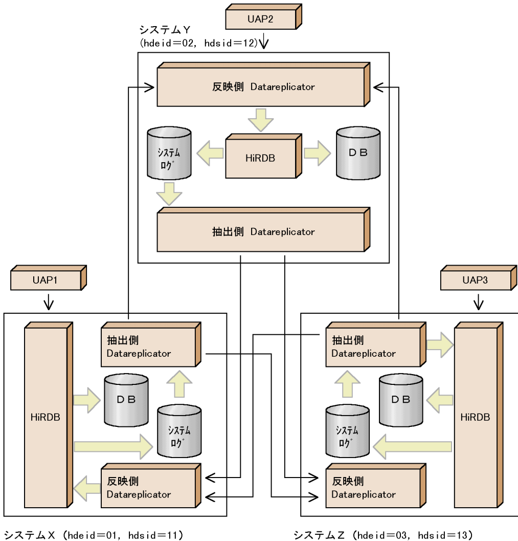
図 4-29 三つ以上のシステムの間で双方向更新をする例
