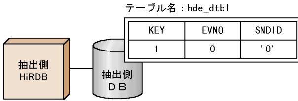
図 4-38 抽出側 HiRDB がシングルサーバの場合のイベント制御用テーブルの例
