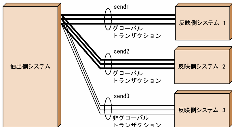
図 3-39 抽出側システムと反映側システムの構成例 2
