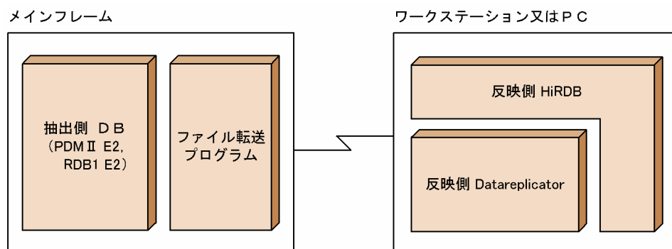
図 1-17 SAM ファイルを使って、メインフレーム側 DB から HiRDB ヘデータ連動する場合のソフトウェア構成
