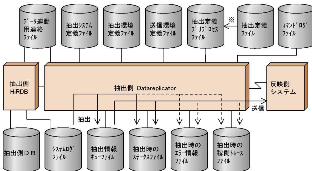
図 3-12 抽出処理の概要
