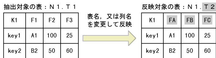
図 3-2 表名、又は列名を変更して反映する例
