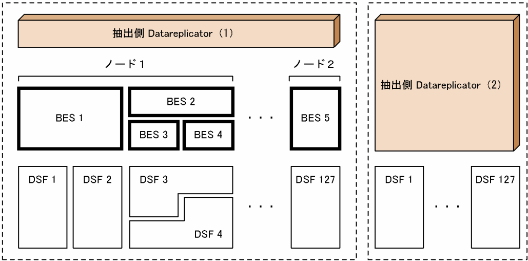
図 3-30 抽出側システムでの Datareplicator ファイルシステム領域への格納例
