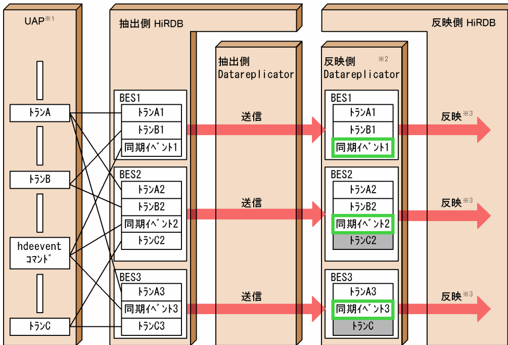
図 3-41 反映トランザクション同期機能の処理の流れ
