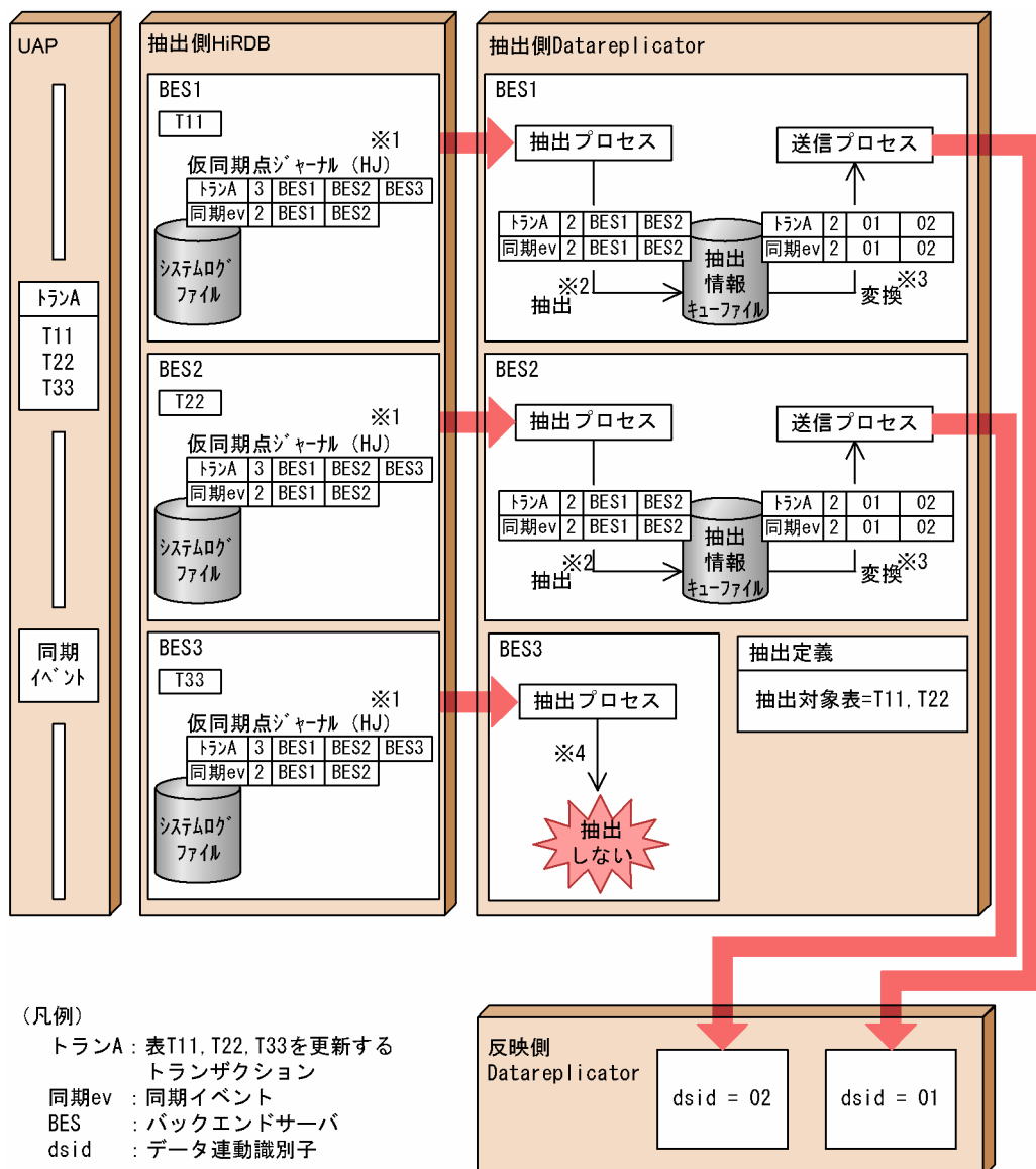
図 3-42 トランザクションブランチ情報の連動
