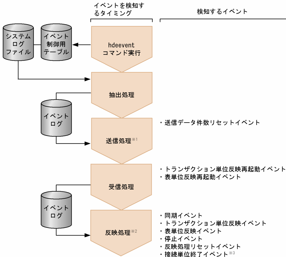
図 3-44 イベントを検知するタイミング
