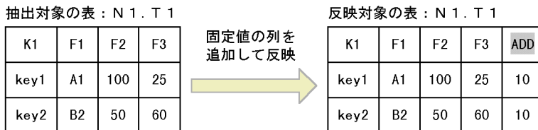
図 3-5 固定値の列を追加して反映する例
