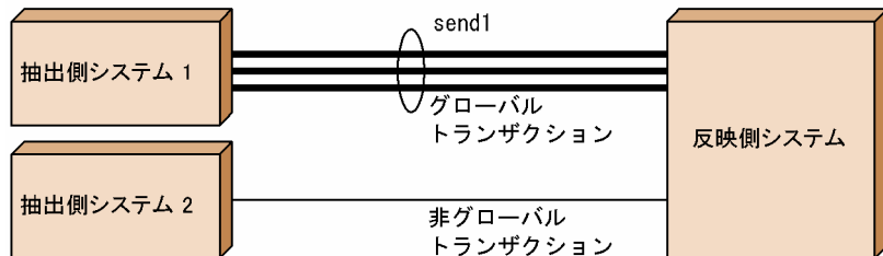
図 3-38 抽出側システムと反映側システムの構成例 1
