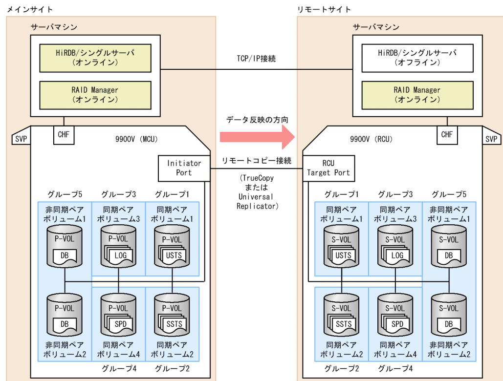
図 2-5 ハイブリッド方式のシステム構成例 (HiRDB/シングルサーバの場合)
