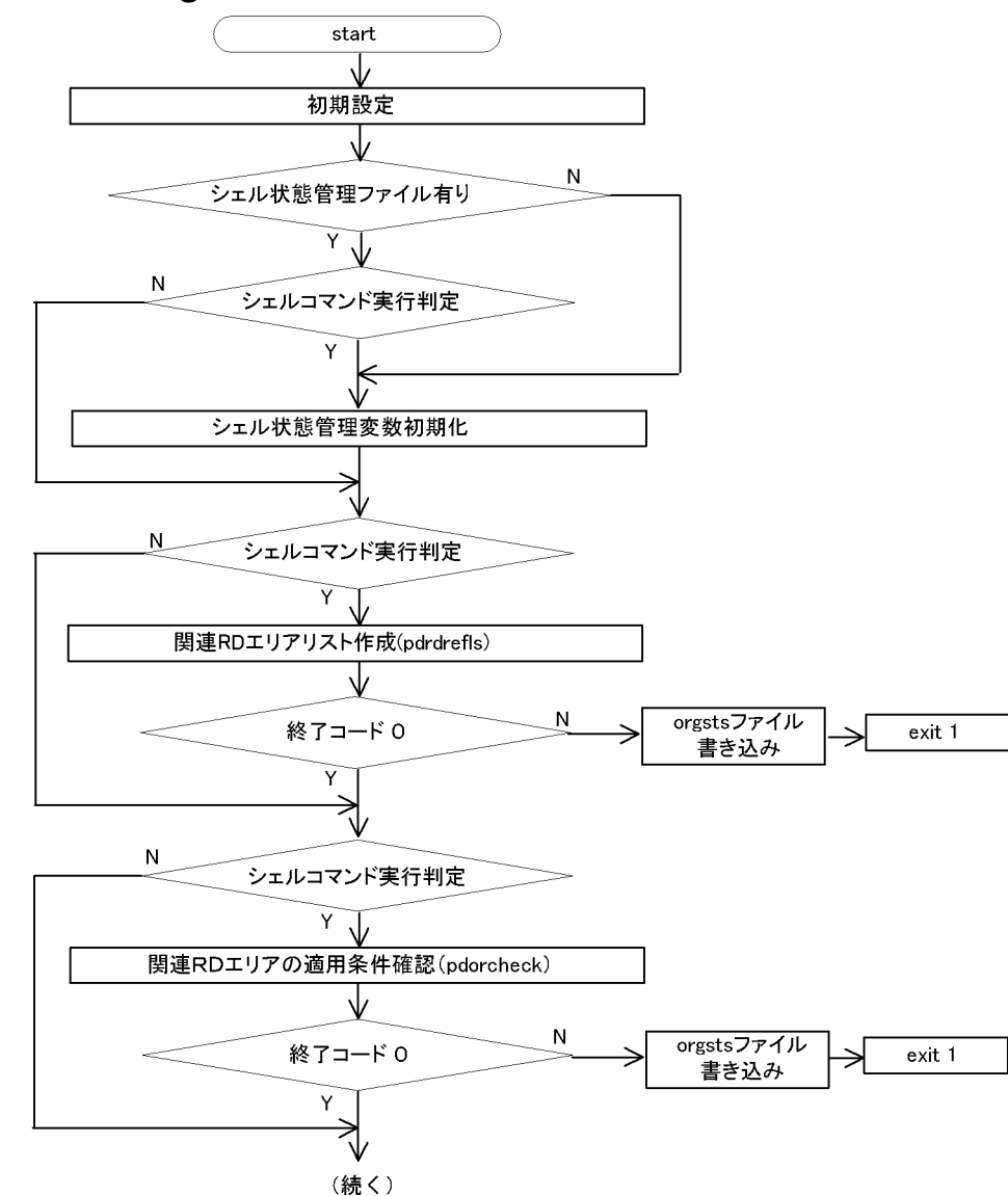
図 E-4 org1_ [OS 名] .sh のフローチャート
