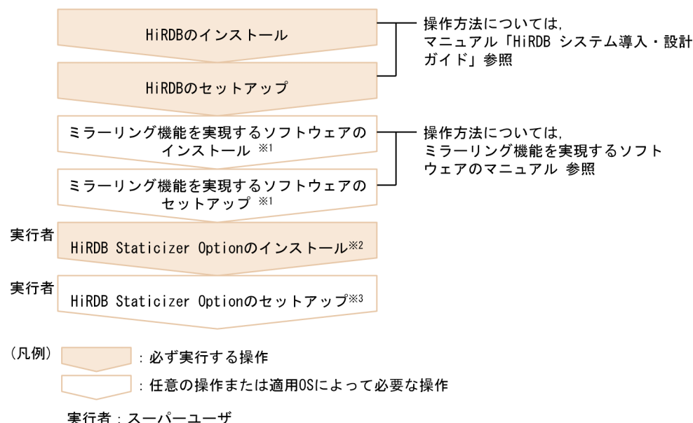
図 2-2 HiRDB と HiRDB Staticizer Option のインストールとセットアップ手順
